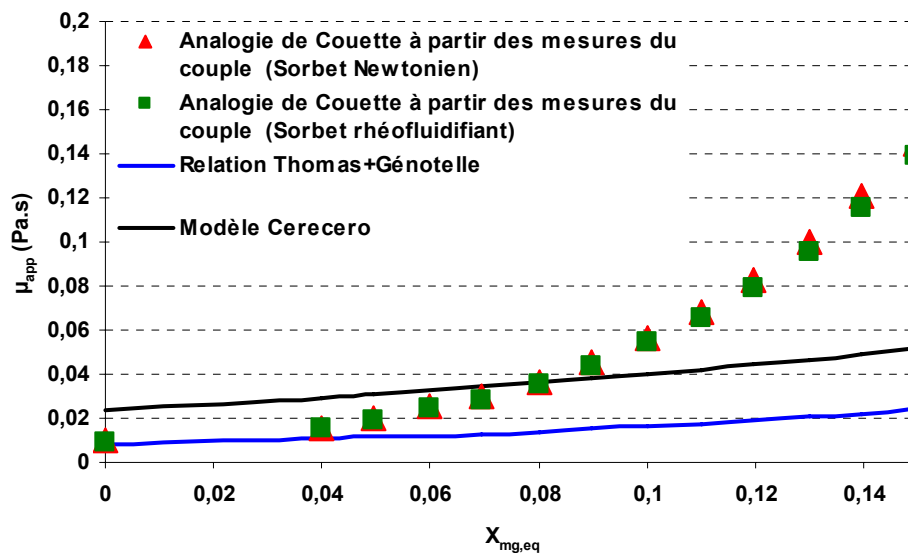
Figure III-7. Comparaison entre les viscosités apparentes déterminées par l'analogie de Couette à partir des mesures du couple (début de la congélation : X_{\text{mg,eq}} < 15\% ) et celles calculées avec les modèles de Thomas et de Cerecero (solution de 30% de sucre et à T_b = -20^\circ\text{C} , N_{\text{rac}} = 300 \text{ tr/min} , N_{\text{mob}} = -100 \text{ tr/min} ).
