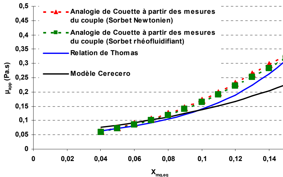
Figure III-17. Comparaison entre les viscosités apparentes déterminées par l'analogie de Couette à partir des mesures du couple et celles calculées avec les modèles de Thomas et de Cerecero à X_{mq,eq} < 15\% (solution de 45% de sucre et à T_b = -20^\circ\text{C} , N_{rac} = 300 \text{ tr/min} , N_{mob} = -100 \text{ tr/min} ).
