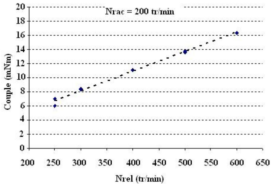
Figure II-11. Mesures du couple avec le mobile hélice dans le cas d'une huile de 4,87 Pa.s et pour une vitesse du racleur de 200 tr/min.
