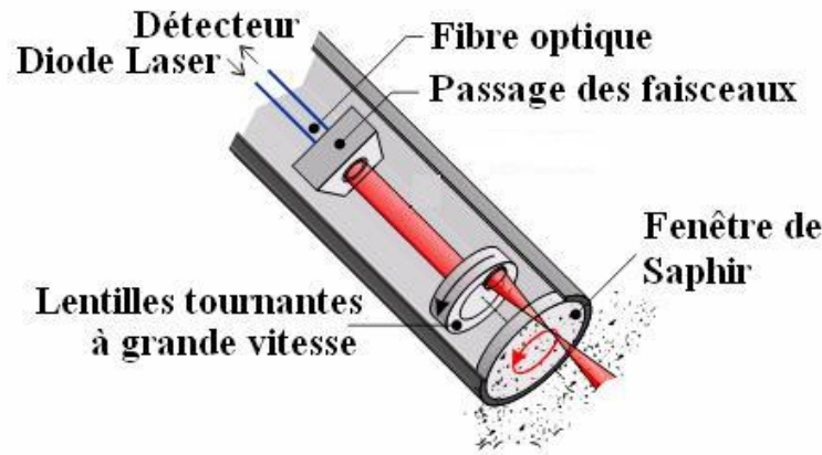
Figure I-11. Sonde FBRM
