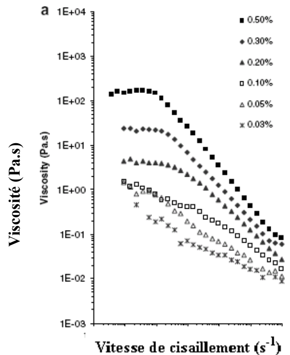
Figure III-18. Viscosité apparente des suspensions de Xanthane à différentes fractions massiques et à différentes vitesses de cisaillement (Sereno et al, 2007).
