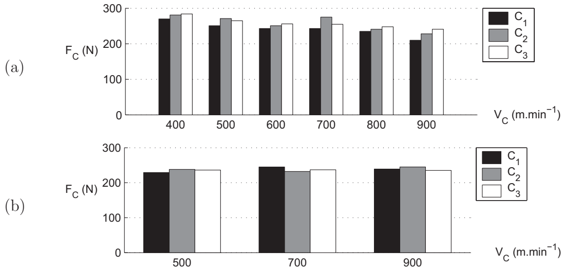
Figure 3.2 – Evolution de l'effort de coupe en fonction de la vitesse de coupe, pour une avance f = 0,3mm.tr^{-1} et différents matériaux (a) CMM_5 , (b) CMM_{15} .
