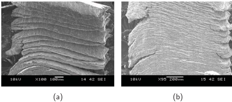
Figure 4.2 – Observation des copeaux obtenus lors de la coupe du CMM_{25} (a) et du CMM_{25ST} (b) par l'outil C_1 .
