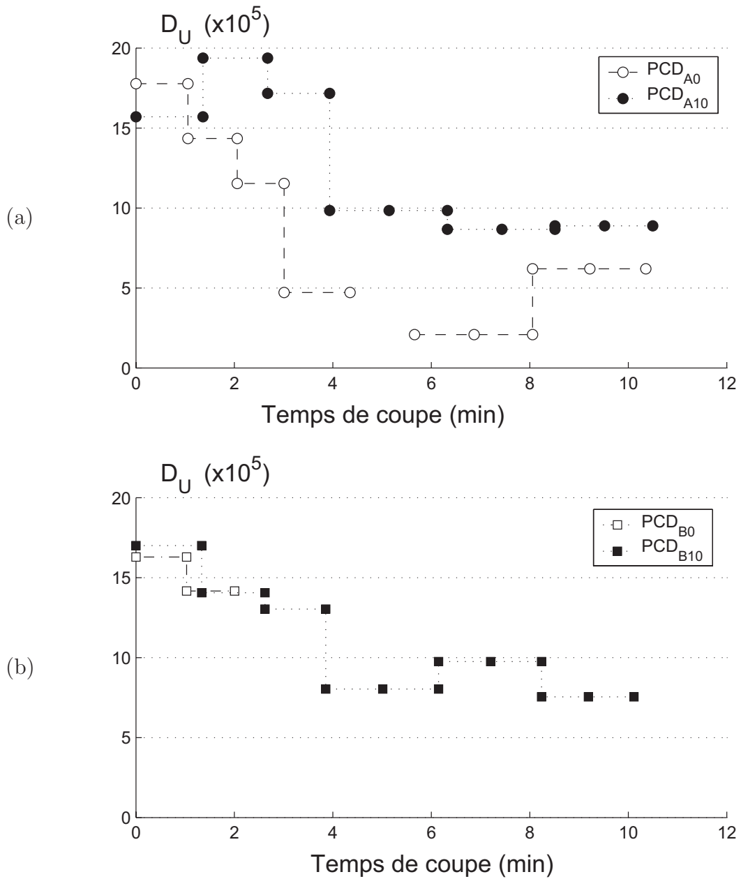
Figure 4.16 – Evolution du Dust Unit ( D_U ) lors des essais de coupe du CMM_{15} avec les outils PCD_A (a) et PCD_B (b).
