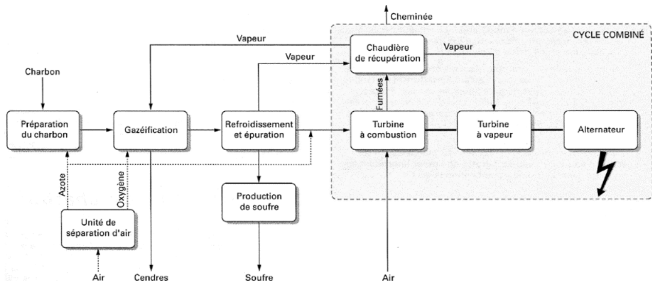
Figure 17 : Schéma simplifié du fonctionnement d'une IGCC, d'après Klaeyl et Nandjee (1997)
