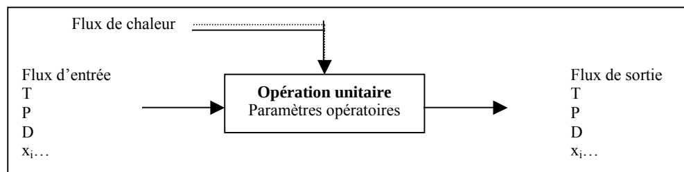
Figure 21 : Représentation d'un module d'opération unitaire
