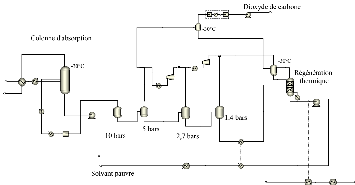
Figure 57 : Schéma de la séparation du CO 2 .
