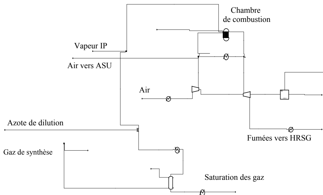
Figure 38 : Turbine à combustion
