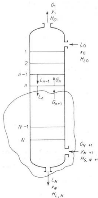
Figure 23 : Absorbeur
