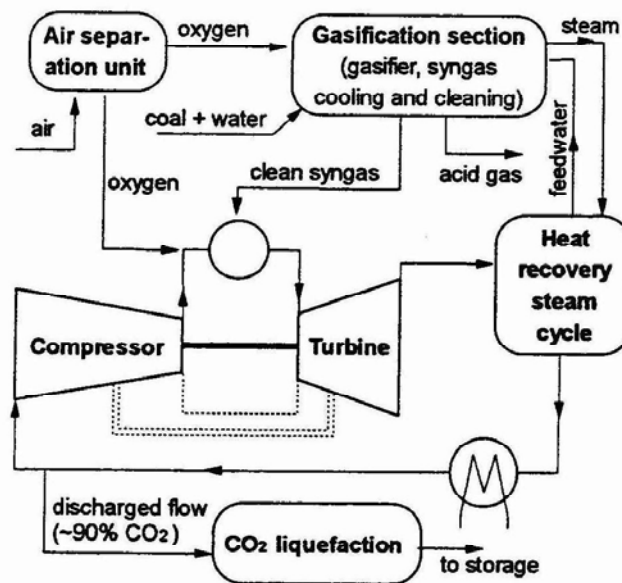
Figure 18 : Séparation du dioxyde de carbone cycle \text{O}_2/\text{CO}_2 , Chiesa et Lozza (1999)
