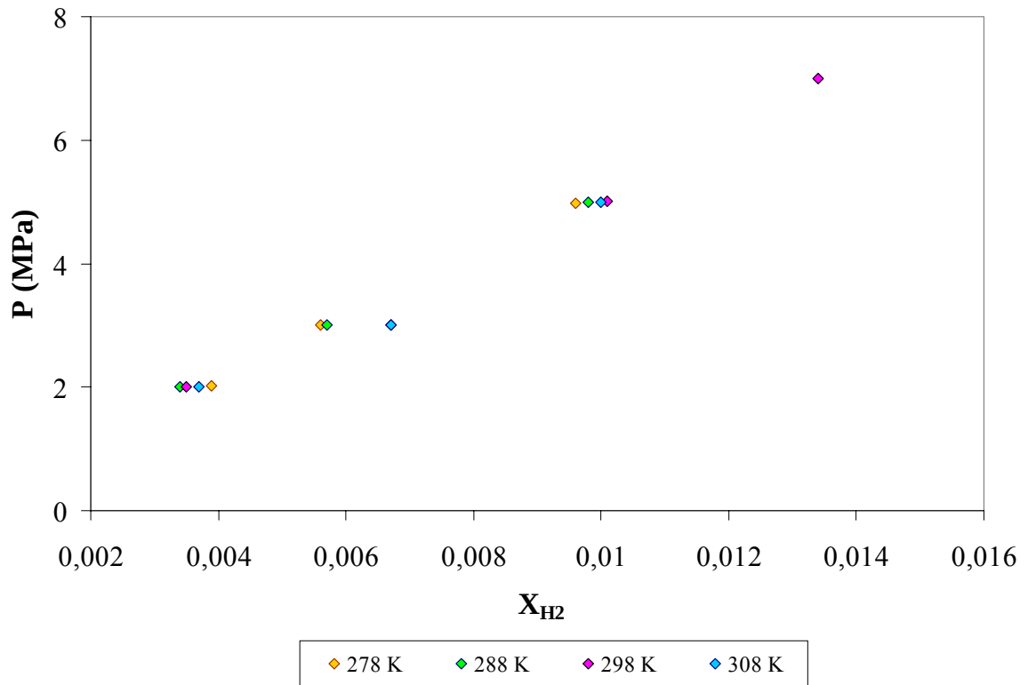
Figure 58 : Solubilité de l'hydrogène dans le méthanol, d'après Bezanehtak et al. (2002)
