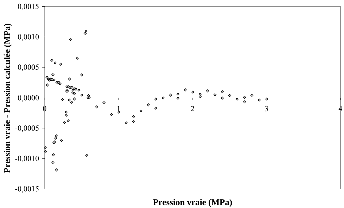
Figure 65 : Écarts absolus sur les mesures de pression de la cellule, capteur 2,5 MPa.
