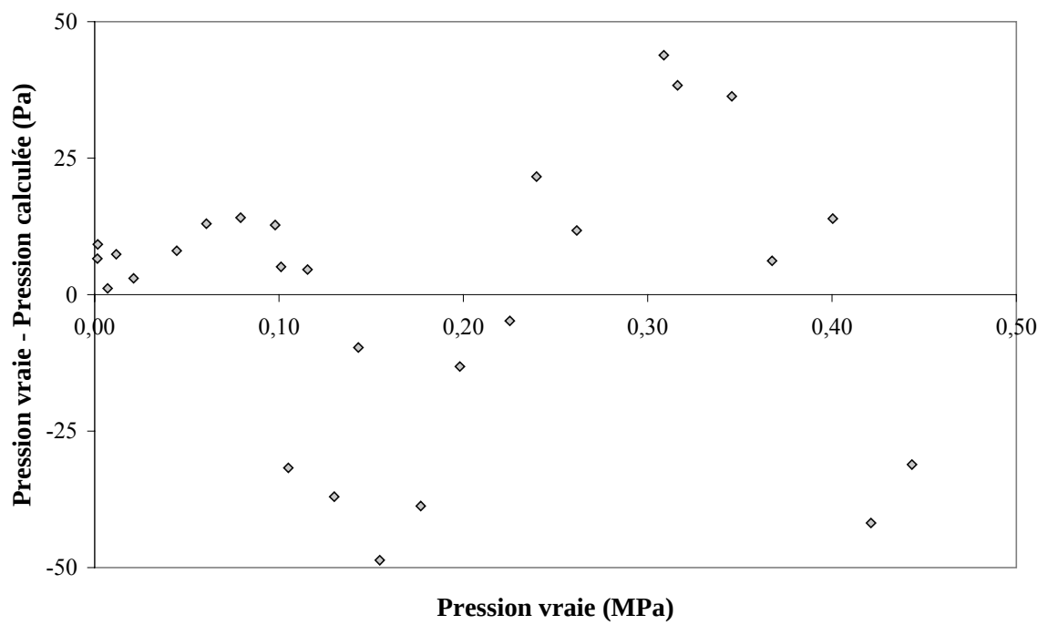
Figure 66 : Écarts absolus sur les mesures de pression de la cellule, capteur 0,25 MPa.
