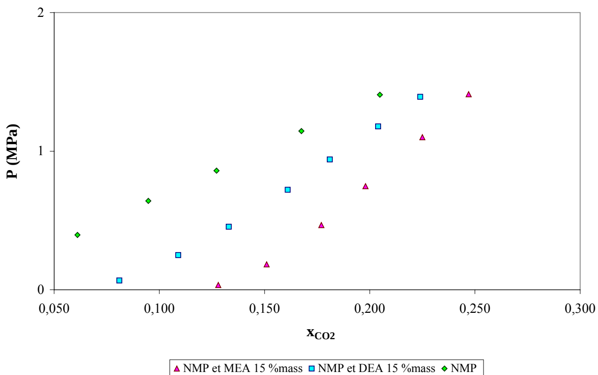
Figure 11 : Solubilité du CO_2 dans les mélanges NMP et MEA ou DEA à 298 K, Murietta-Guevara et al. (1992)
