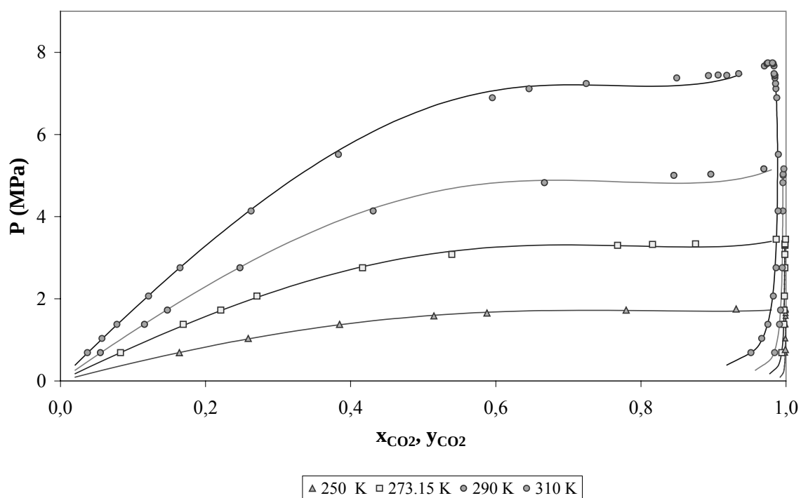
Figure 44 : Équilibres liquide vapeur CO 2 méthanol, Hong et Kobayashi (1988) et calcul avec le modèle thermodynamique.
