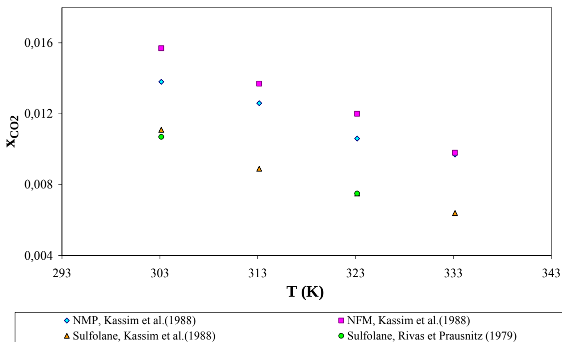
Figure 7 : Solubilité du CO 2 à 0,1 MPa
