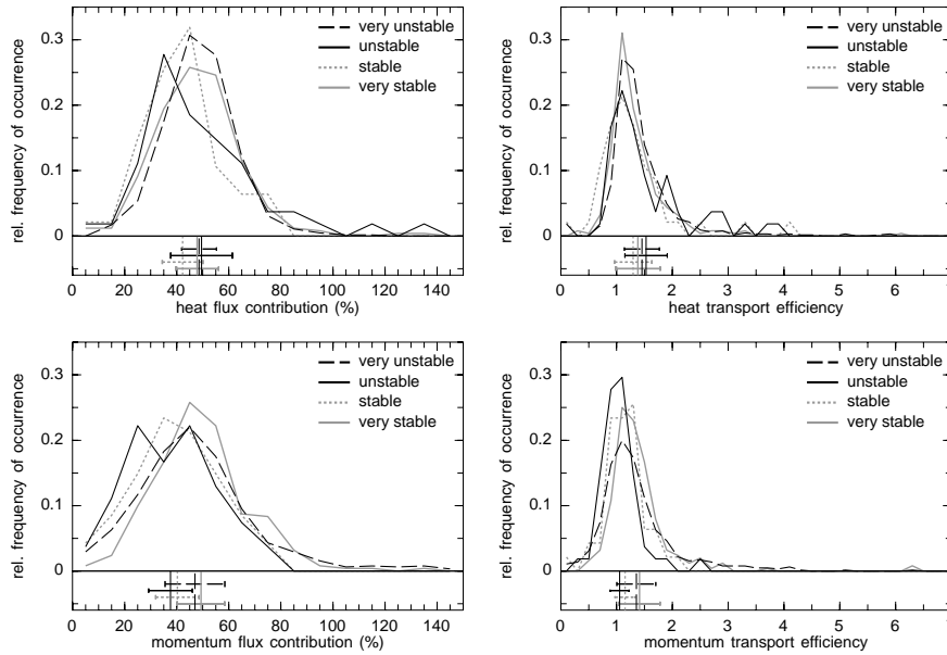
FIG. 4.5 – Distributions de probabilité de la contribution des structures cohérentes aux flux et de l'efficacité du transport à 10 m. Les distributions des contributions aux flux ont été calculés par pas de 10%.
