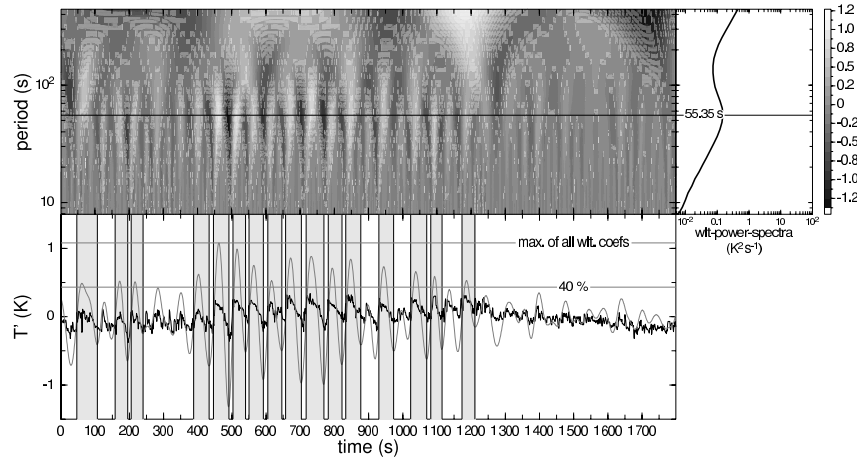
FIG. 2.9 – Idem figure 2.6, mais pour les fluctuations de température en condition stable du 31 Mai 2005 (2000-2030 UTC) à l’observatoire du SIRTA.
