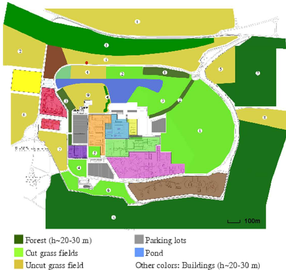
FIG. 2.3 – Carte de l’Ecole Polytechnique. Les couleurs correspondent à différents types de terrain (forêt, champ d’herbe, bâtiments...). Le point rouge localisé sur le champ d’herbe représente le mât instrumenté du Sirta.
