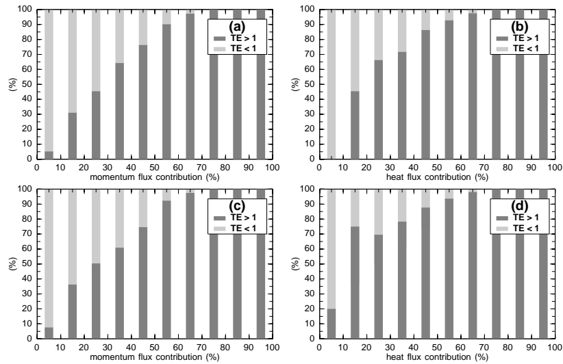
FIG. 4.9 – Variation de l’efficacité du transport en fonction de la contribution au flux à 30 m (a;b) et 10 m (c;d).
