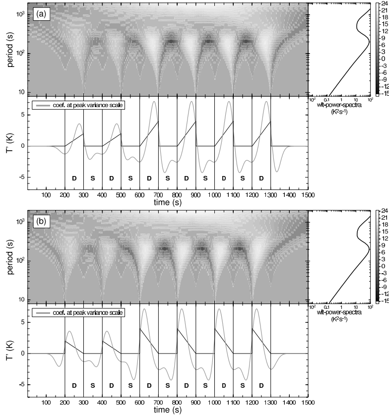
FIG. 2.6 – Exemples de transformation en ondelette en conditions instable (a) et stable (b). Chaque sous-figure représente les coefficients d’ondelette W_n(s) (en haut) de la série temporelle artificielle (en bas, ligne noire), les coefficients d’ondelette à l’échelle où le spectre global d’ondelette atteint son maximum (en bas, ligne grise) et le spectre global d’ondelette \overline{W}(s) (en haut à droite).
