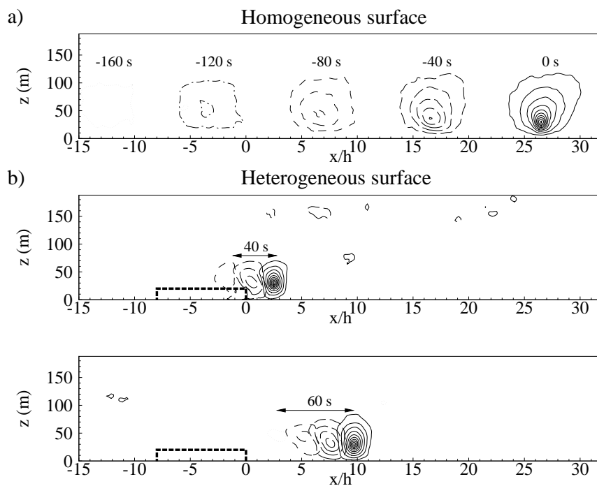
FIG. 6.8 – Identification de la trajectoire des structures cohérentes à partir des contours de la fonction d’auto-correlation espace-temps pour la composante verticale du vent R_{33\Delta t} en terrains homogène (a) et hétérogène (b), pour des points de référence localisés au temps t_0 = 0 s à z = 30 m et x = 26.5h pour (a), et à x = 2.5h et 9.5h pour (b). Les contours varient de 0.1 à 1.0 avec un pas de 0.1. La ligne noire en pointillés indique le contour de la canopée.
