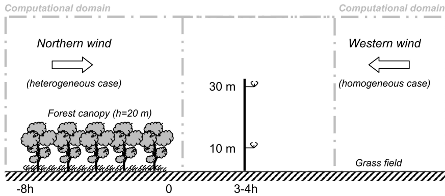
FIG. 2.5 – Représentation schématique du site expérimental pour les deux secteurs de vent, nord et ouest, qui nous intéressent dans cette étude. Nous en tirons deux cas, le cas hétérogène et le cas homogène, associés à deux domaines de calcul représentés respectivement par des rectangles pointillé-point et pointillé-point-point
