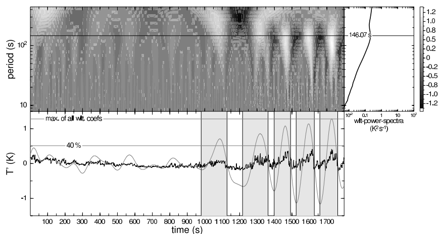
FIG. 2.8 – Idem figure 2.6, mais pour les fluctuations de température en condition instable du 28 Novembre 2005 (1100-1130 UTC) à l'observatoire du SIRTA.
