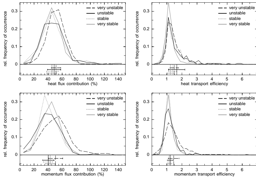
FIG. 4.6 – Distributions de probabilité de la contribution des structures cohérentes aux flux et de l'efficacité du transport à 30 m.
