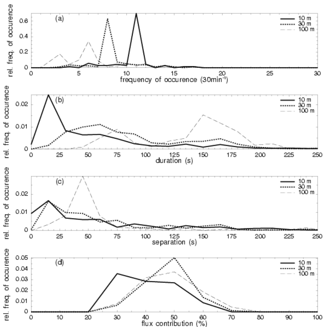
FIG. 6.4 – Distribution de probabilité de la fréquence d'occurrence (a), de la durée des structures (b), du temps de séparation entre deux structures consécutives (c) et de la contribution relative au flux de quantité de mouvement (d) à z = 10, 30 et 100 m, en terrain homogène.
