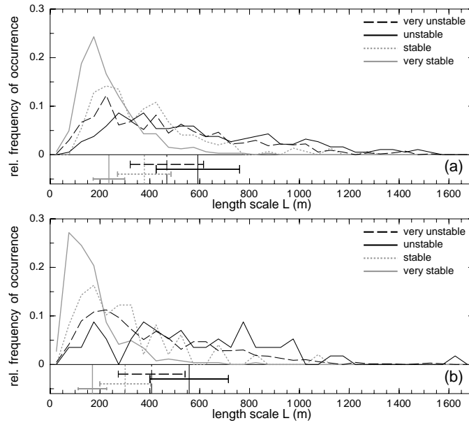
FIG. 4.3 – Distribution de probabilité de la taille caractéristique L à 30 m (a) et 10 m (b). Même légende que la figure 4.1.
