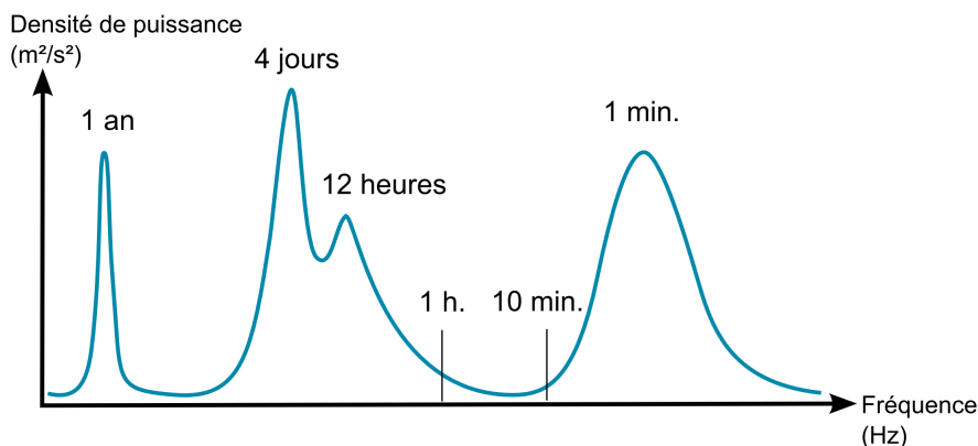
FIG. 1.1 – Schéma représentant les différentes échelles du vent à 100 m d'altitude (Van der Hoven, 1957).
