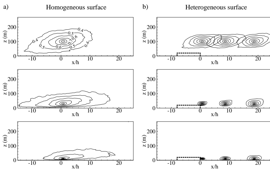
FIG. 6.6 – Contours des fonctions d'auto-corrélation spatiales pour la composante longitudinale de la vitesse du vent R_{110} en terrains homogène (a) et hétérogène (b), avec des points de référence localisés à z = 10, 30 et 100 m de bas en haut, respectivement, et à x = 1h pour (a) et à x = 1h, 9h et 19h pour (b). Les contours varient de 0.4 à 1.0 comme indiqué sur la figure en haut à gauche. La ligne en pointillés indique le contour la canopée.
