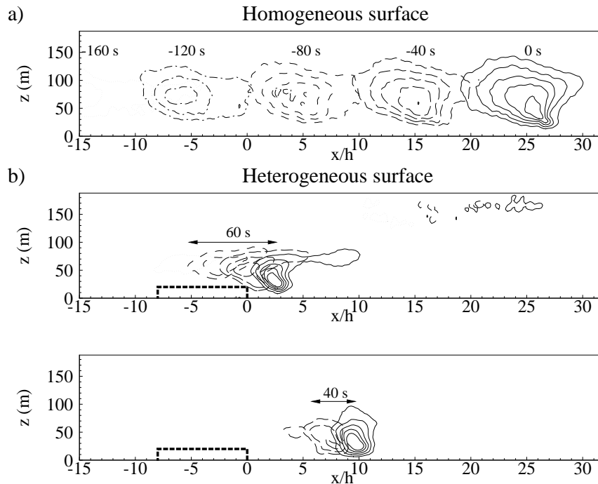
FIG. 6.9 – Identification de la trajectoire des structures cohérentes à partir des contours de la fonction de corrélation espace-temps croisée pour les composantes longitudinale et verticale de la vitesse du vent R_{13\Delta t} en terrains homogène (a) et hétérogène (b), avec des points de de référence localisés au temps t_0 = 0 s à z = 30 m et x = 26.5h pour (a), et x = 2.5h et 9.5h pour (b). Les contours varient de -0.15 à -0.35 avec un pas de 0.05 . La ligne noire en pointillés indique le contour de la canopée.
