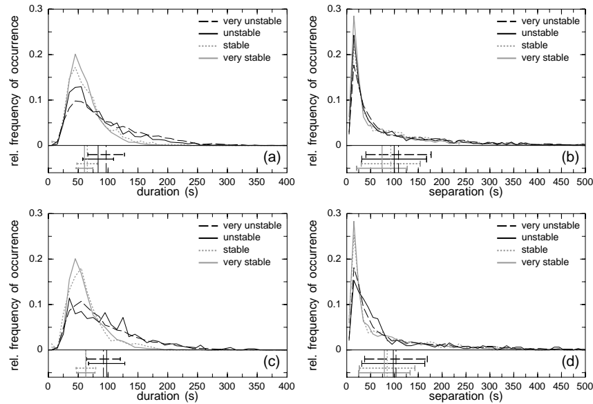
FIG. 4.2 – Distribution de la durée et de la séparation des structures cohérentes à 30 m (a;b) et 10 m (c;d). Même légende que la figure 4.1.
