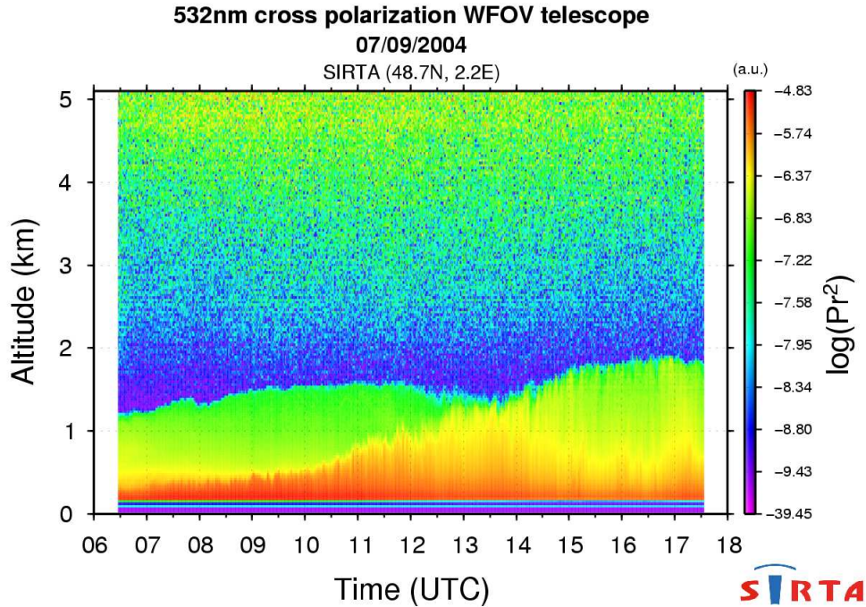
FIG. 2.2 – Evolution temporelle de la hauteur de CLA ( z_i ) au SIRTA entre 6h00 TU et 18h00 TU.
