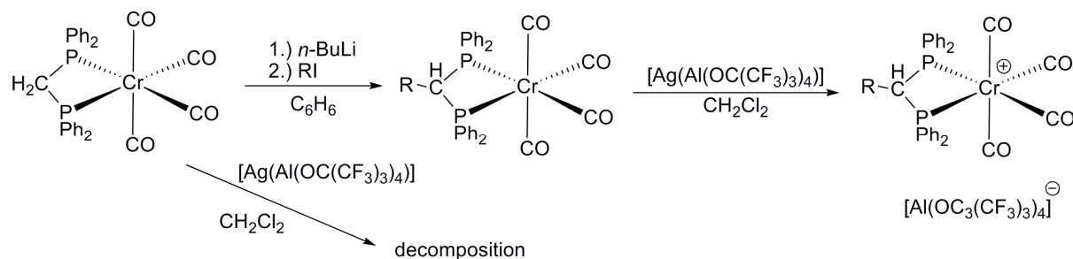
Scheme 28.
