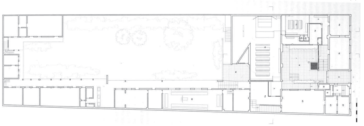
P0: Plan de rez-de-chaussée
