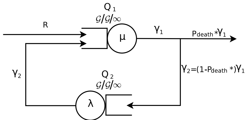
Figure A.12: Réseau de files d'attente modélisant le stockage d'un objet.
