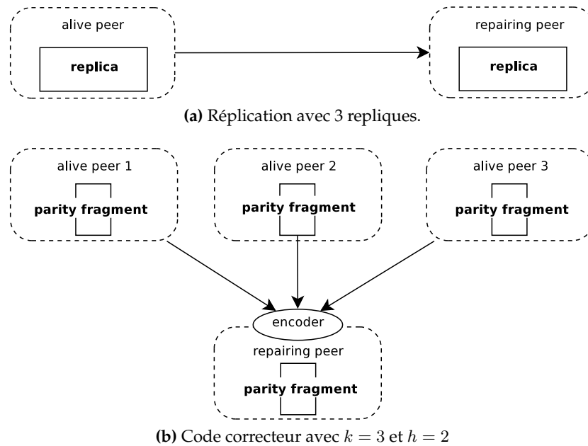
Figure A.5: Schémas de redondance : Réparation des données.
