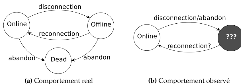
Figure A.3: Automate fini modélisant le comportement d'un pair.
