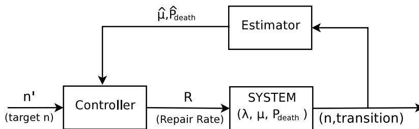
Figure A.11: Le schéma de contrôle adaptatif
