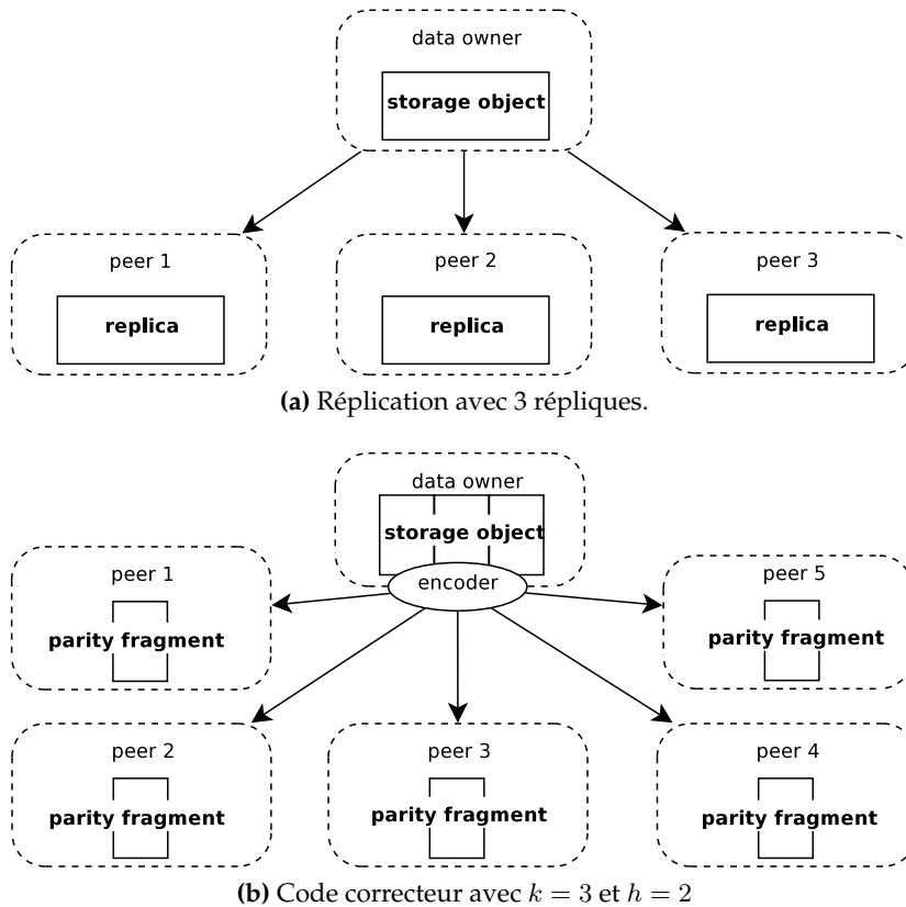
Figure A.4: Schémas de redondance : Insertion des données.
