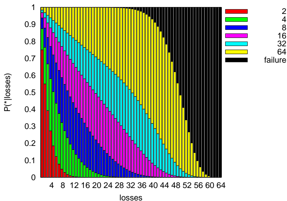
(a) Hierarchical Code A.
