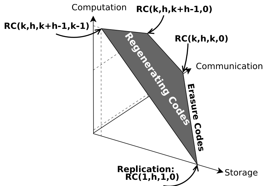
Figure A.10: Illustration du trade-off posé par le "Regenerating Codes".
