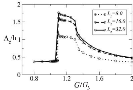
FIGURE 5.11 – Longueur de pénétration \Lambda_z calculée avec le modèle DJS pour un contraste de viscosité de \eta = 0.05 pour des rapports d'aspect, ou encore largeur renormalisée par la hauteur w/h = L_z = 8, 16, 32 .
