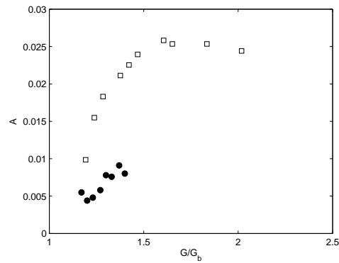
FIGURE 5.20 – Amplitude du mode dominant issue de l’expérience (carrés) et de l’analyse non-linéaire avec le modèle DJS (cercles pleins) pour w/h = L_z = 2 .
