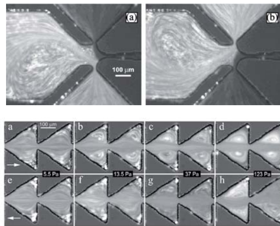
FIGURE 2.3 – Résistance anisotrope [54] et commutateur microfluidique [62] utilisant les non-linéarités visco-élastiques en circuit microfluidique.
