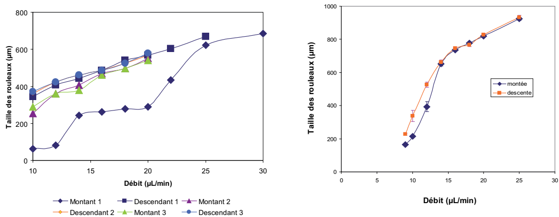
FIGURE C.6 – Diamètre mesuré de rouleaux stables à l'entrée d'une constriction G2 en fonction du débit pour du PEO 5 MDa 1000 ppm lors de cycle successifs de montée et de descente sans retrouver l'état laminaire (exploration de la branche sous-critique après déclenchement en haut), et valeur moyenne en retrouvant l'état laminaire (exploration de l'hystérésis).
