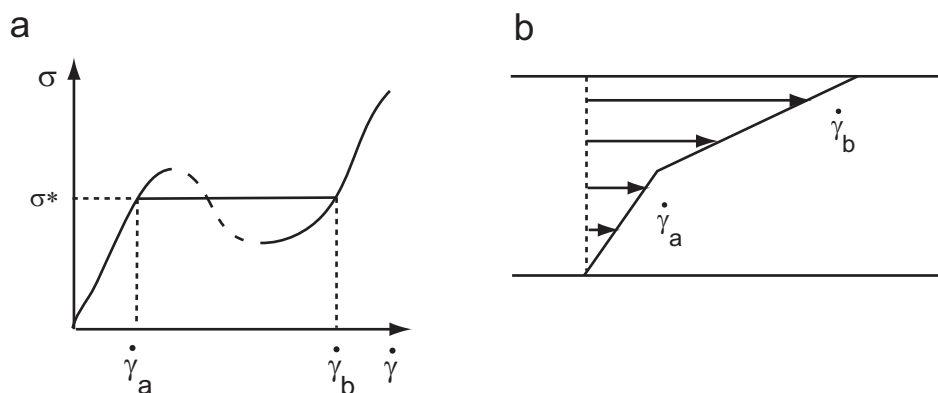
FIGURE 4.2 – (a) Relation constitutive non monotone donnant lieu à un écoulement en bandes de cisaillements (en Couette plan ici).
