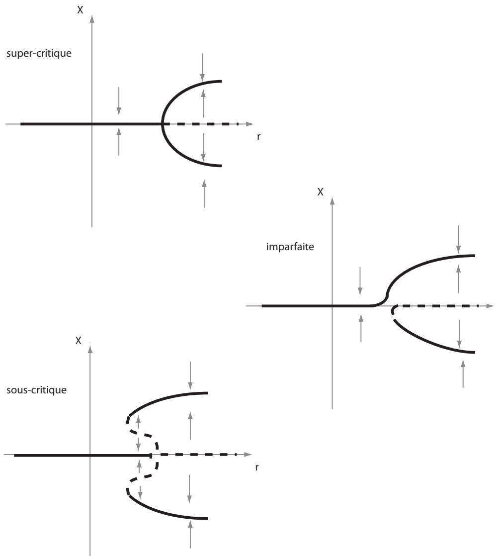
FIGURE 5.1 – Bifurcations super-critique, sous-critique et imparfaite de paramètre de contrôle r et de paramètre d'ordre X . Les branches pleines indiquent les valeurs d'équilibre stables de X et les branches pointillées les valeurs d'équilibre instable. La connaissance de la stabilité est issue de l'analyse de petite perturbation au voisinage de la valeur d'équilibre, perturbations qui sont soit atténuées soit amplifiées exponentiellement, selon le sens donné par les flèches.
