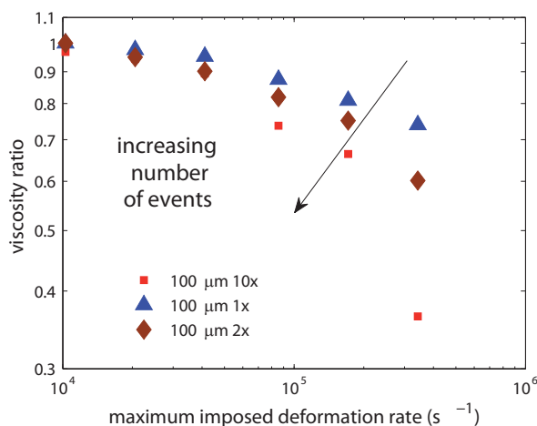
FIGURE 3.17 – Baisse de viscosité induite par le passage en constrictions répétées d’une solution de PEO 5 MDa 4000 ppm.
