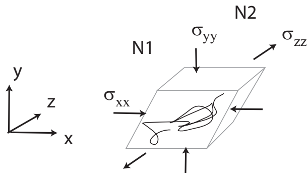
FIGURE 1.7 – Contribution des forces normales non nulles dans le cas du cisaillement d’un objet anisotrope tel un polymère. Les composantes N_1 et N_2 sont chacune la somme de leur deux flèches adjacentes.
