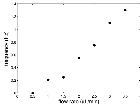
FIGURE C.7 – Fréquence d’oscillation entre deux rouleaux à l’entrée de la géométrie G6 pour une solution de PEO 5MDa 1000 ppm.
