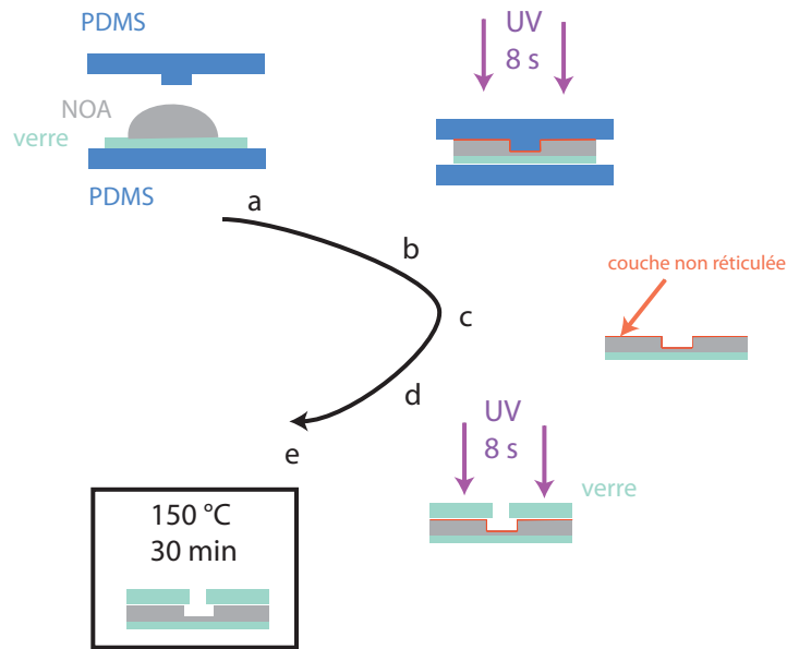
FIGURE 2.6 – Protocole de fabrication d’un circuit résistant à des pressions élevées. (a) Le moule en PDMS est apporté en contact avec une goutte de NOA 81 disposée sur une lamelle de verre, elle-même posée sur un support planaire en PDMS. (b) Exposition sous lampe UV ( 20\text{ mW.cm}^2 ) et réticulation en volume de la NOA. Les surfaces en contact avec le PDMS restent non réticulée sur une certaine épaisseur dépendant du temps d’insolation. (c) Démoulage du PDMS. (d) Mise en contact avec une lame de verre, préalablement percée pour les connectiques, avec la surface non réticulée. Adhésion mécanique puis ré-insolation pour l’adhésion par réticulation. (e) Recuit au four au-dessus de la T_g pour une adhésion maximale.
