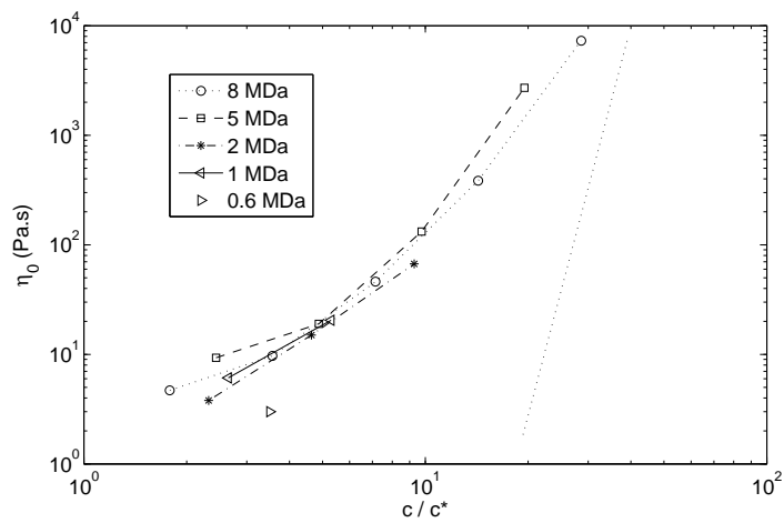
FIGURE B.5 – \eta_0 pour des solutions de différentes tailles moyenne en fonction de la concentration renormalisée par les valeurs de c^* déduites de la Fig. ??.
