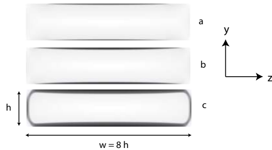
FIGURE 5.9 – Module du taux de déformation local calculé avec le modèle DJS dans un canal de section rectangulaire pour G/G_b = 1.08, 1.18, 1.4 (de haut en bas) et un rapport d'aspect de 8.
