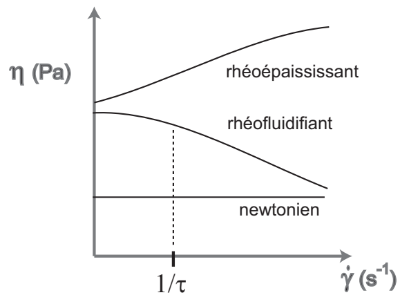
FIGURE 1.6 – Courbes schématiques de viscosité non-linéaire pour des fluides rhéofluidifiants, newtonien et rhéoépaississant (l’allure des courbes correspond typiquement à une représentation logarithmique).
