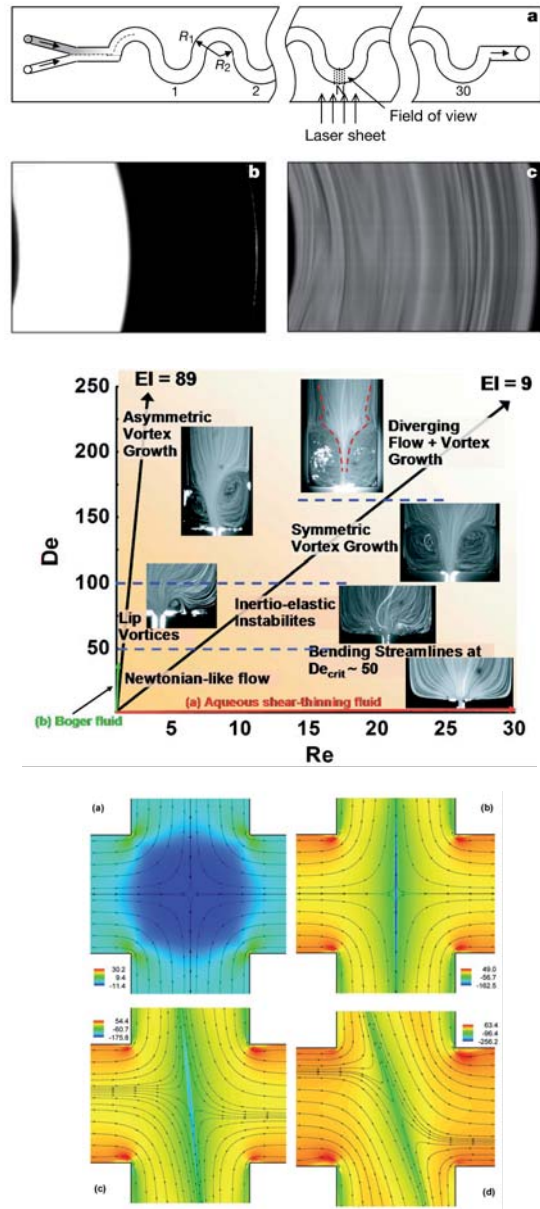
FIGURE 2.2 – Etudes fondamentales d’instabilités viscoélastiques en canaux microfluidiques. Les deux figures du haut représentent la géométrie en serpentin et l’effet de mélange mesuré dû à la présence de recirculations déclenchées par la courbure (tiré de [21]). Le diagramme du milieu répertorie les comportements de recirculations à l’entrée d’une constriction plane (tiré de [58]). Bas : champs de déformation et de contrainte d’une instabilité spécifique en cross-slot (tiré de [60]).
