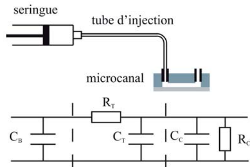
FIGURE 2.5 – Montage microfluidique et sa correspondance en terme électrocinétique.
