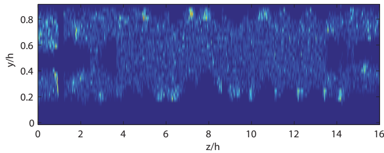
FIGURE 5.23 – Carte du flux de traceurs de 3 \mu m à travers une section de canal à \Delta p = 1.95 \text{ bars} en x = 4 \text{ cm} . Les zones bleu foncé sont complètement déplétées en traceurs et la frontière de cette zone déplétée correspond à l'interface entre les deux phases. On observe près des bords latéraux d'autres zones de déplétion sans doute liées à l'effet de bord commenté au 5.3.
