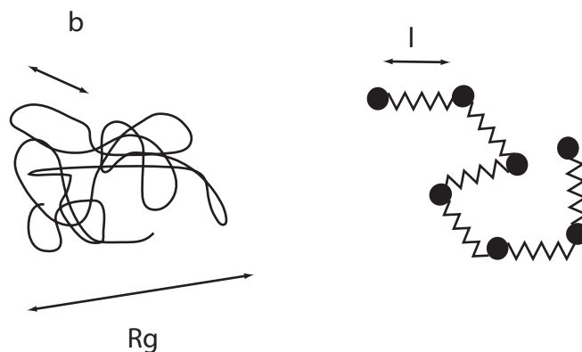
FIGURE 1.9 – Représentations d’une chaîne de polymère. A gauche une chaîne de conformation aléatoire ayant une longueur de persistance b définissant un segment de Kuhn et un diamètre effectif R_g , le rayon de gyration. A droite la représentation d’une chaîne gaussienne sous forme de billes reliées par des ressorts, renfermant l’information sur la force entropique d’un segment de longueur l ayant lui-même une configuration aléatoire.
