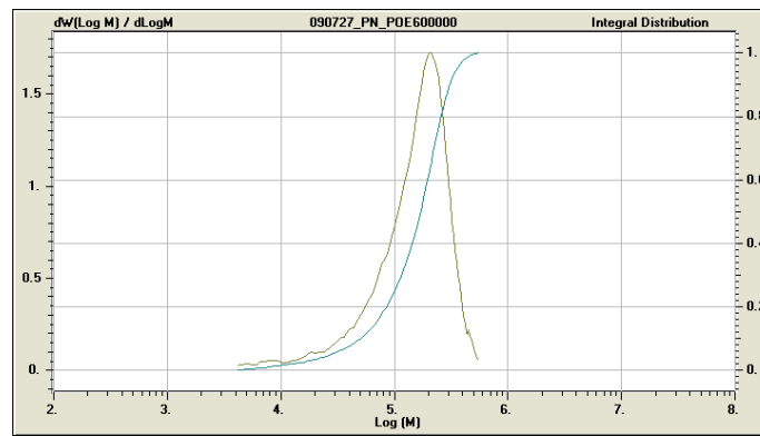
FIGURE B.6 – GPC effectuée sur un échantillon de PEO de masse moyenne 0.6 MDa de Sigma-Aldrich indiquant un indice de polydispersité de 2.
