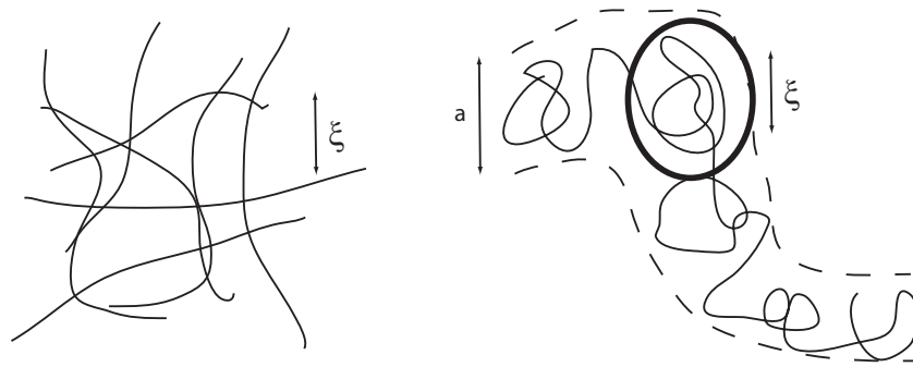
FIGURE 1.10 – Chaînes en régime enchevêtré ( c > c^* ). A gauche, réseau formé par les chaînes a une taille caractéristique de maille \xi qui correspond à la longueur de corrélation des fluctuations de concentration. A droite, une chaîne donnée voit l’environnement des autres chaînes comme un "tube" de diamètre a contraignant son mouvement de diffusion. Dans ce cadre, les interactions internes à la chaînes sont écartées sur une échelle supérieure à \xi , ce qui lui confère un caractère gaussien similaire à une chaîne isolée. Les sous-parties de chaîne de diamètre \xi sont nommées "blobs" (partie cerclée).
