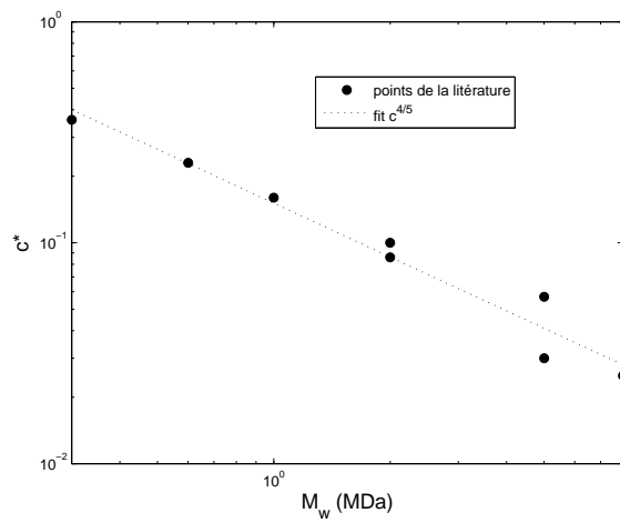
FIGURE B.4 – Valeurs de c^* en fonction de la masse pour des PEO, extraites des références [138, 139].
