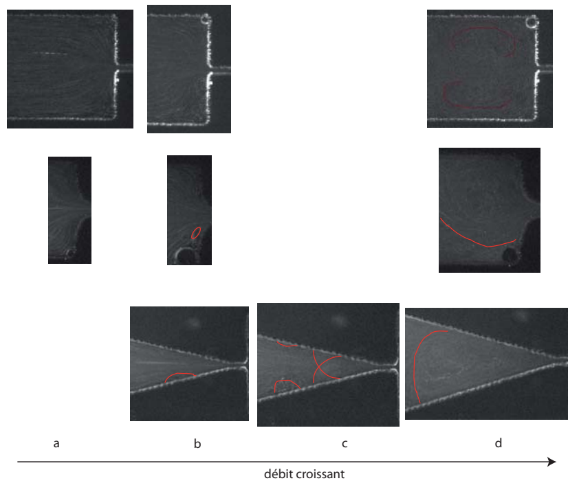
FIGURE C.2 – Morphologies de recirculations en amont de différentes constrictions pour du PEO 5 MDa 1000 ppm : (a) régime laminaire; (b) "lip vortex" ou rouleau intermittent accroché à la paroi; (c) parfois plusieurs localisations instationnaires des "lip vortices"; (d) rouleau permanent. Le régime instationnaire à plus haut débit n'est pas représenté.
