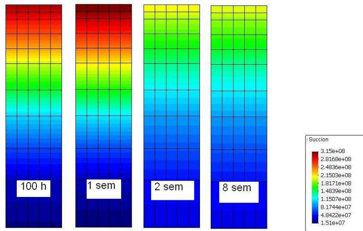
FIGURE 16.28 – Evolution de la succion à la fin de l'essai de Pintado et al. [161]
