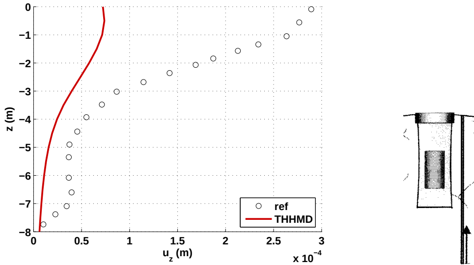
FIGURE 17.84 – Déplacements verticaux dans le massif granitique, à proximité de la barrière ouvragée, après la phase de chauffage (au bout de 8 mois et demi).
