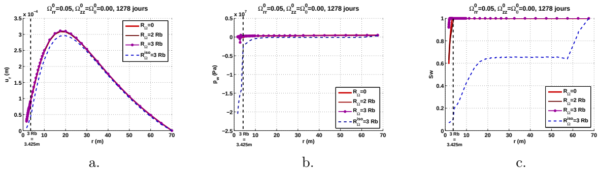
FIGURE 17.73 – Test in situ FEBEX. Influence de la présence d'un endommagement initial radial de 5 pour cent dans une zone d'étendue variable sur le comportement du massif granitique. Etat de la barrière géologique après la phase de refroidissement (1278 jours). a. Déplacement radial. b. Pression d'eau interstitielle. c. Degré de saturation.
