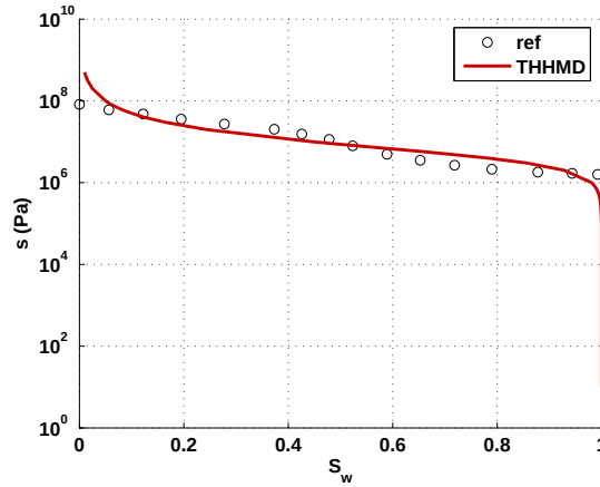
FIGURE 17.77 – Courbe de rétention adoptée dans la simulation du test de chauffage de Kamaishi. Calage des paramètres de Van Genuchten d’après les données expérimentales [173] : \alpha_{VG} = 2 \cdot 10^{-7} \text{ Pa}^{-1} , n_{VG} = 2 .
