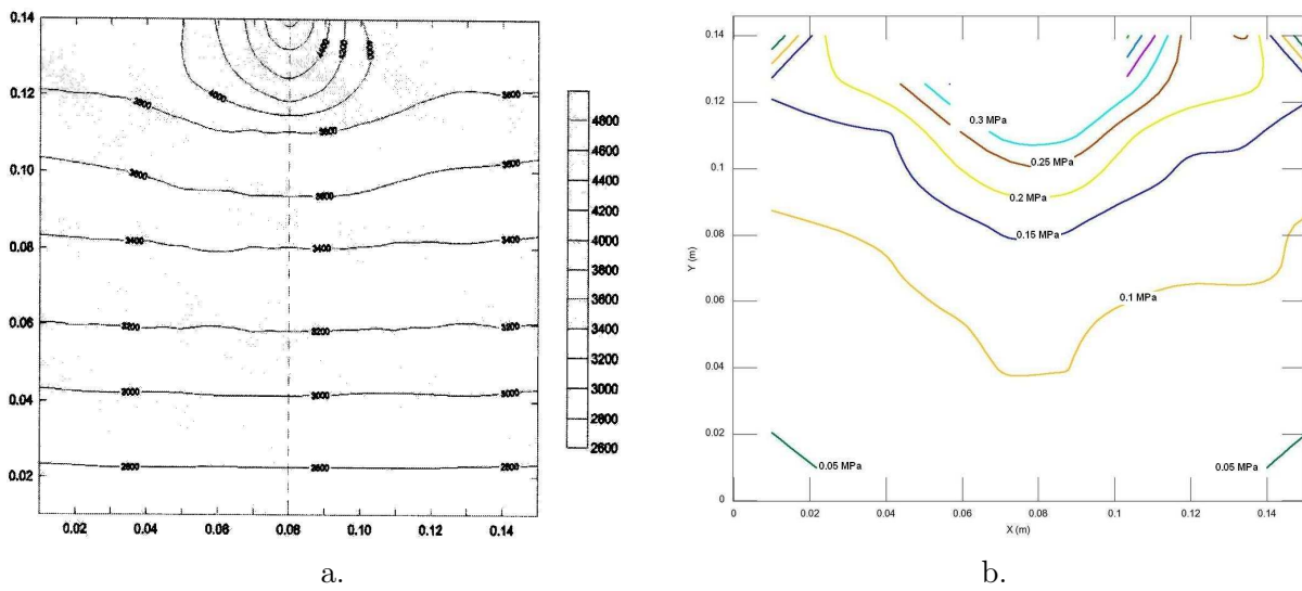
FIGURE 16.43 – Distribution spatiale de la succion après 2h de chauffage. a. Modèle à surfaces d'état [102]. b. Modèle THHMD.
