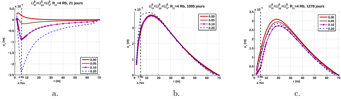
FIGURE 17.55 – Test in situ FEBEX. Influence de la présence d'endommagement initial isotrope dans la zone Rb \leq r \leq 4Rb . Evolution du déplacement radial dans le massif granitique. a. Fin de l'accroissement de température (21 jours). b. Après le plateau de température (1095 jours). c. Après refroidissement (1278 jours).
