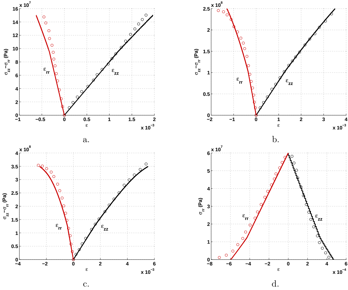
FIGURE 16.2 – Essais mécaniques sur le granite de la Vienne : comparaison des résultats numériques (lignes continues) aux mesures expérimentales (points) [93]. a. Compression triaxiale, p_c = 0 \text{ MPa} . b. Compression triaxiale, p_c = 5 \text{ MPa} . c. Compression triaxiale, p_c = 20 \text{ MPa} . d. Extension latérale, p_c^{\text{init}} = 60 \text{ MPa} .
