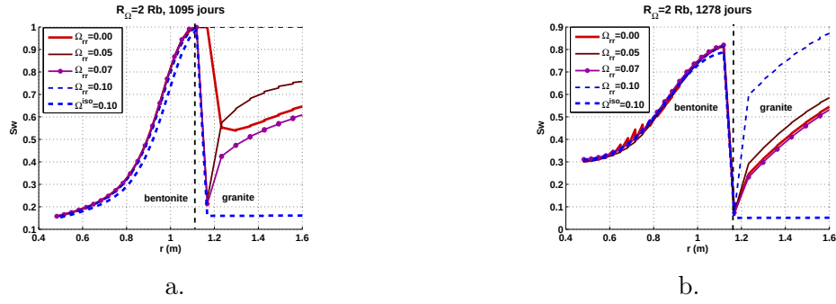
FIGURE 17.72 – Test in situ FEBEX. Influence de la présence d'un endommagement initial radial entre r = Rb et r = 2Rb sur le degré de saturation de la barrière ouvragée en bentonite. a. Après le plateau de température (1095 jours). b. Après refroidissement (1278 jours).
