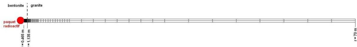
FIGURE 17.44 – Géométrie et maillage adoptés pour la simulation du test in situ FEBEX [79].
