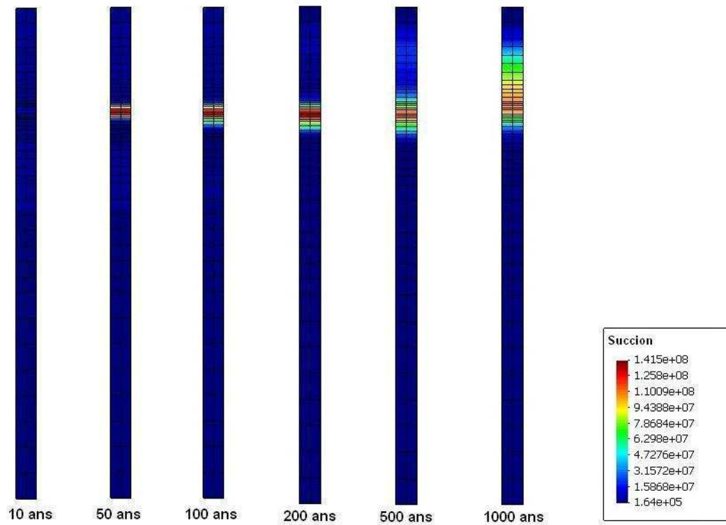
FIGURE 17.32 – Evolution spatio-temporelle de la succion avec le modèle THHMD dans le problème de Pollock [163].
