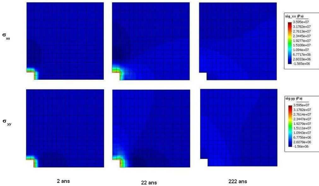
FIGURE 17.16 – Evolution spatio-temporelle des contraintes dans le problème de stockage des déchets radioactifs [32] traité en déformations planes.
