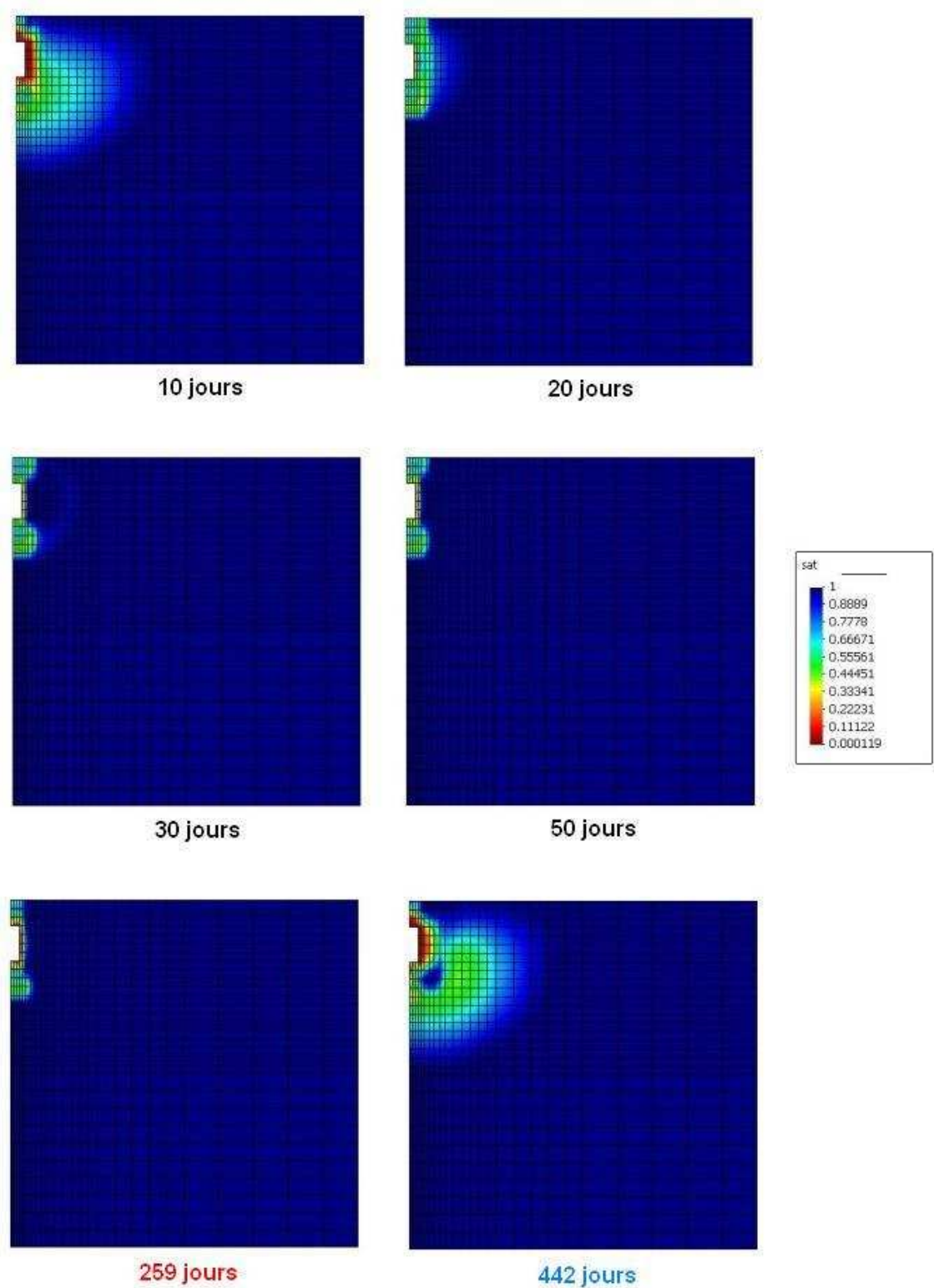
FIGURE 17.92 – Evolution spatio-temporelle du degré de saturation dans la simulation du test de Kamaishi. Cas n^{\circ} 2 (un plan de fissuration horizontal d’une étendue de 10 mètres).
