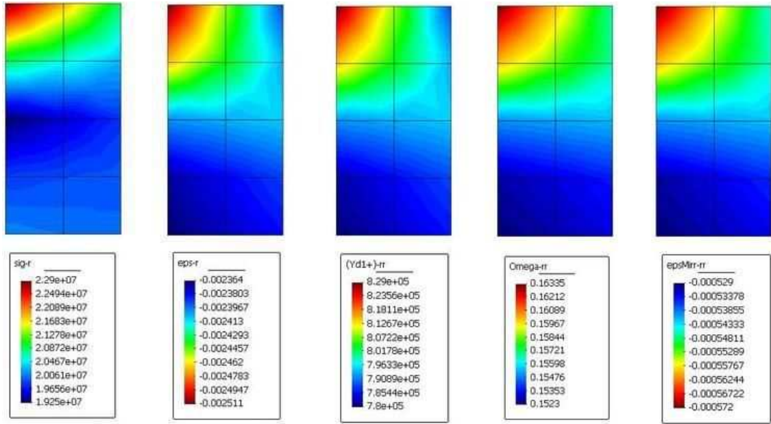
FIGURE 16.4 – Caractérisation de l'état mécanique de l'échantillon de granite de la Vienne à la fin de l'essai de compression triaxiale ( p_c = 20\text{MPa} ).
