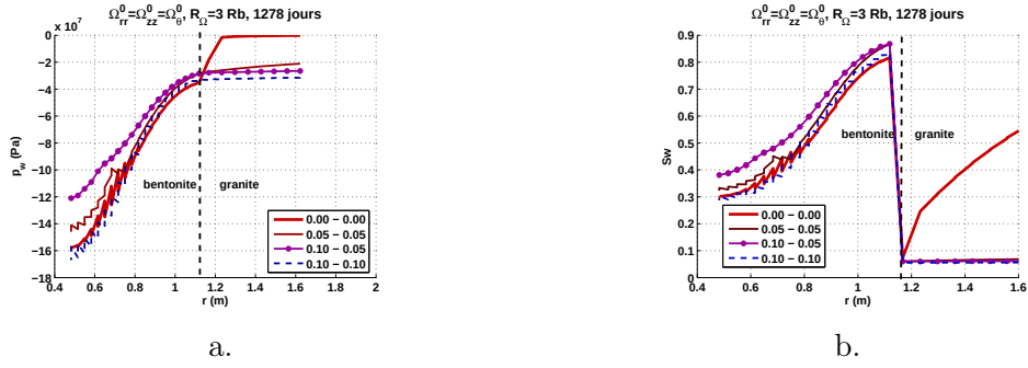
FIGURE 17.64 – Test in situ FEBEX. Influence de la présence d’endommagement initial isotrope dans la zone Rb \leq r \leq 3Rb , avec deux zones d’endommagement : Rb \leq r \leq 2Rb et 2Rb \leq r \leq 3Rb . Observations au voisinage de la frontière entre les barrières ouvragée (en bentonite) et géologique (en granite) après une phase de refroidissement (1278 jours). a. Pression d’eau interstitielle. b. Degré de saturation.
