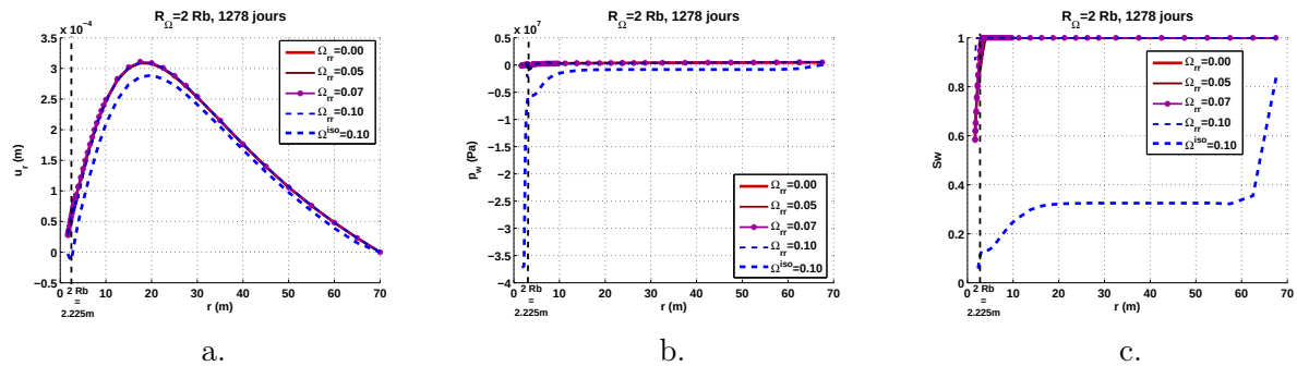
FIGURE 17.70 – Test in situ FEBEX. Influence de la présence d'un endommagement initial radial entre r = Rb et r = 2 Rb sur le comportement du massif granitique. Etat de la barrière géologique après la phase de refroidissement (1278 jours). a. Déplacement radial. b. Pression d'eau interstitielle. c. Degré de saturation.
