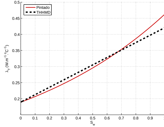
FIGURE 16.20 – Comparaison des modèles de conductivité thermique. \lambda_s = 0.3 W.m^{-1}.^{\circ}C^{-1} dans le modèle THHMD.
