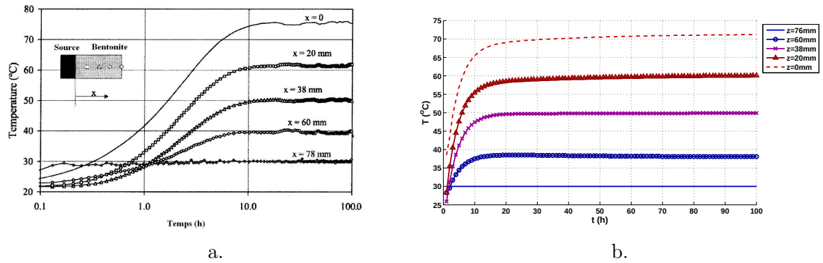
FIGURE 16.23 – Evolutions temporelles de quelques températures nodales lors de l'essai de Pintado et al. a. Mesures expérimentales [161]. b. Résultats numériques.
