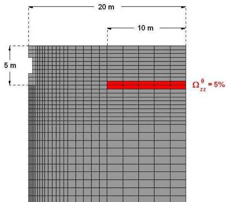
FIGURE 17.86 – Etude du problème de stockage de Kamaishi avec un massif granitique initialement endommagé. Cas n^o 2 : un plan de fissuration horizontal d’une étendue de 10 mètres.
