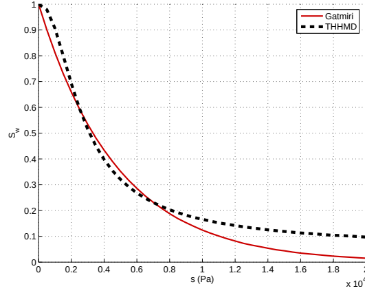
FIGURE 16.36 – Calage de la courbe de rétention du modèle THHMD ( S_{w,r} = 0 , \alpha_{VG} = 5 * 10^{-4} Pa^{-1} , n_{VG} = 2.3 ) sur celle du modèle élastique à surfaces d'état de Gatmiri ( a_s = 1 , b_s = 0 et c_s = -2.08855 Pa^{-1} ).
