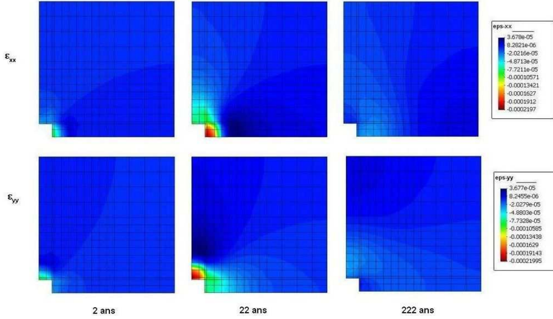
FIGURE 17.17 – Evolution spatio-temporelle des déformations dans le problème de stockage des déchets radioactifs [32] traité en déformations planes.
