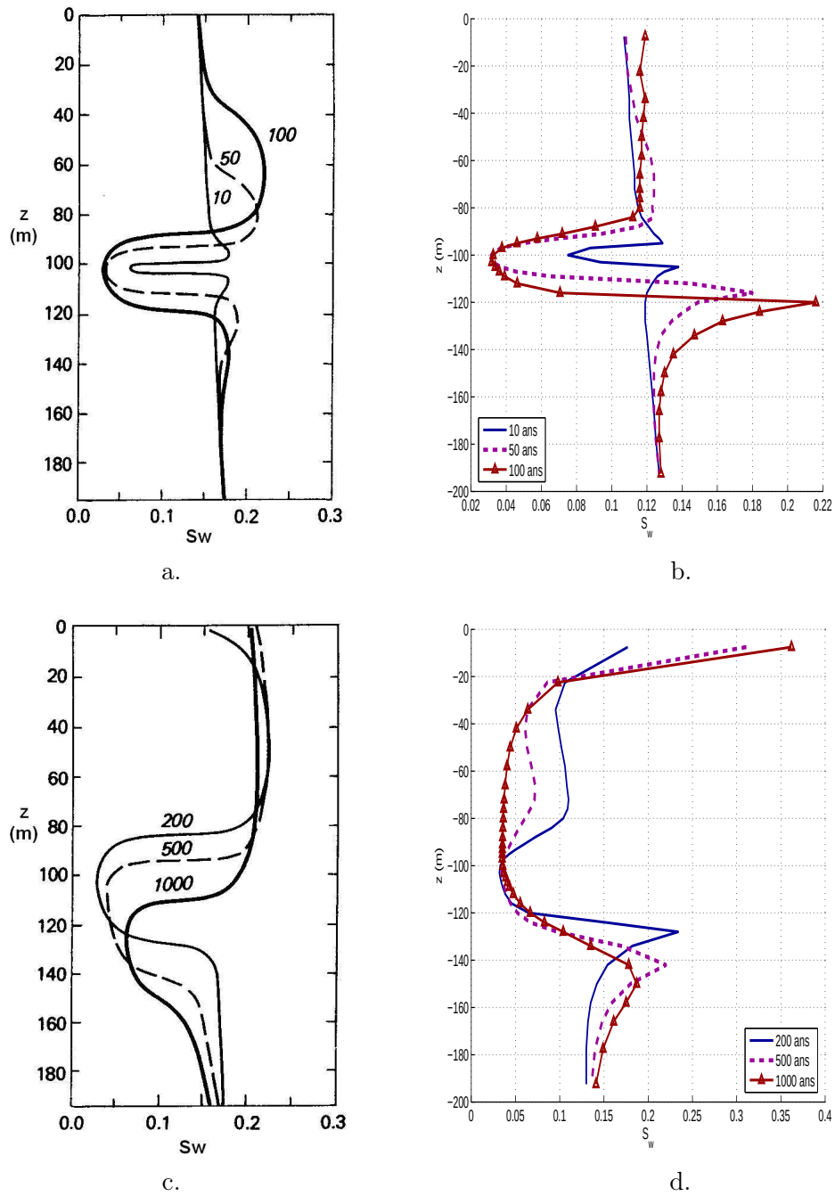
FIGURE 17.31 – Evolution spatio-temporelle du degré de saturation. a,c. Résultats de Pollock [163]. b,d. Résultats obtenus dans le domaine élastique du modèle THHMD.
