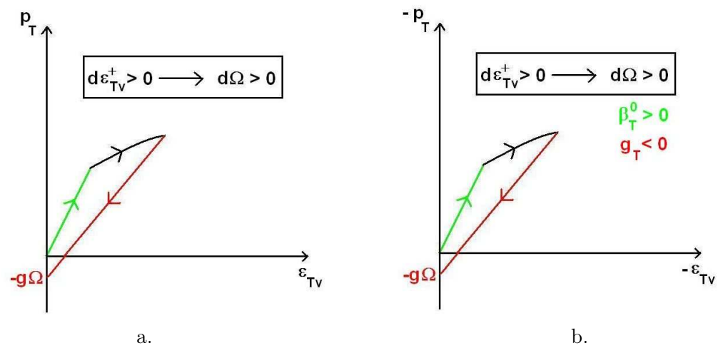
FIGURE 7.3 – Degré de rigidité thermique. a. MMC. b. Mécanique des sols.
