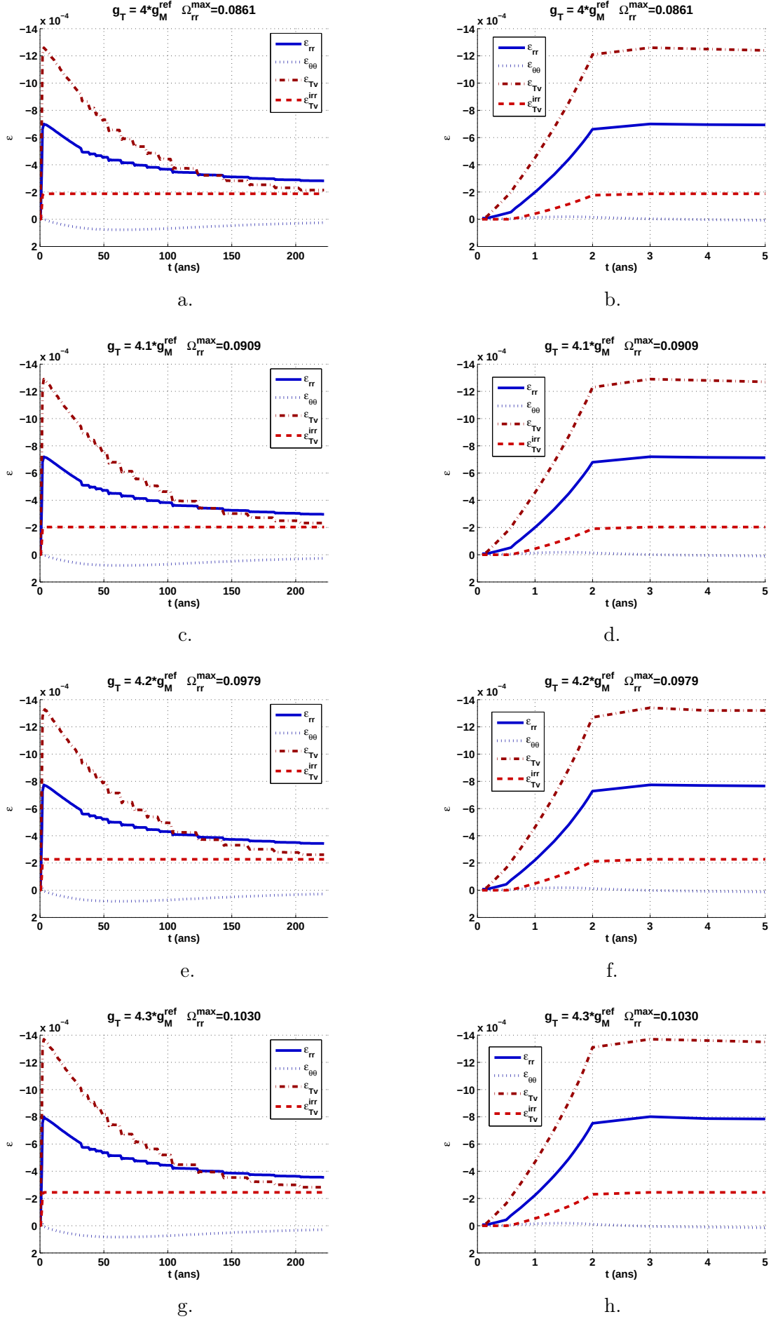
FIGURE 17.19 – Etude axisymétrique du comportement thermo-mécanique fragile d'un massif granitique. Evolution temporelle des déformations calculées sur un élément jouxtant le paquet radioactif, pour g_T = 4 * g_M^{ref} (a,b), g_T = 4.1 * g_M^{ref} (c,d), g_T = 4.2 * g_M^{ref} (e,f) et g_T = 4.3 * g_M^{ref} (g,h).
