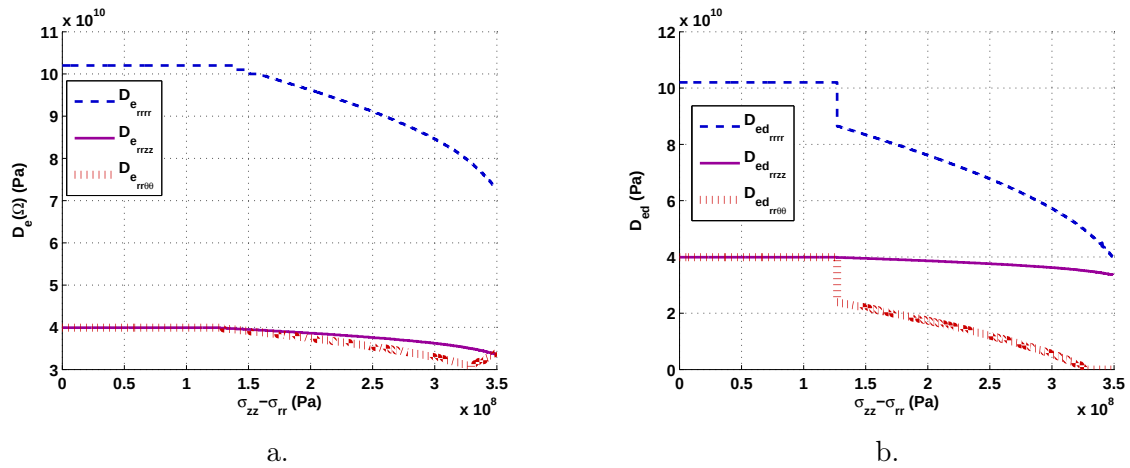
FIGURE 16.5 – Dégradation de quelques coefficients des rigidités mécaniques du granite de la Vienne pendant l'essai de compression triaxiale ( p_c = 20\text{MPa} ). a. Rigidité élastique ( \mathbf{D}_e(\Omega) ). b. Rigidité élasto-fragile ( \mathbf{D}_{ed} ).
