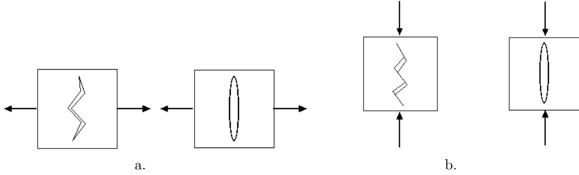
FIGURE 4.3 – Types de ruptures représentées dans le modèle THHMD. a. Traction, “splitting effects” [150]. b. Compression, “crossing effects” [150].
