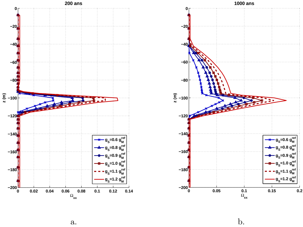
FIGURE 17.41 – Influence de la rigidité g_S sur le développement de l'endommagement dans le problème de stockage des déchets radioactifs traité par Pollock [163]. g_T = 0 . a. Endommagement généré au bout de 200 ans de stockage ( \Omega_{xx} = \omega yy ). b. Endommagement généré au bout de 1000 ans de stockage ( \Omega_{xx} = \omega yy ).
