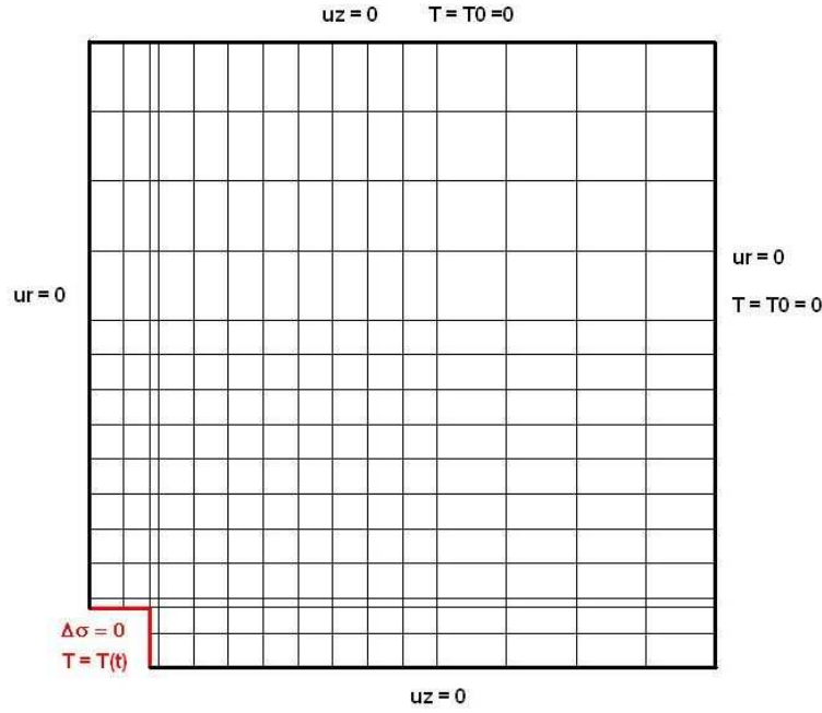
FIGURE 17.11 – Maillage et conditions aux limites pour le problème de stockage de déchets radioactifs dans un massif rocheux sec [32]. Analyse en déformations planes.
