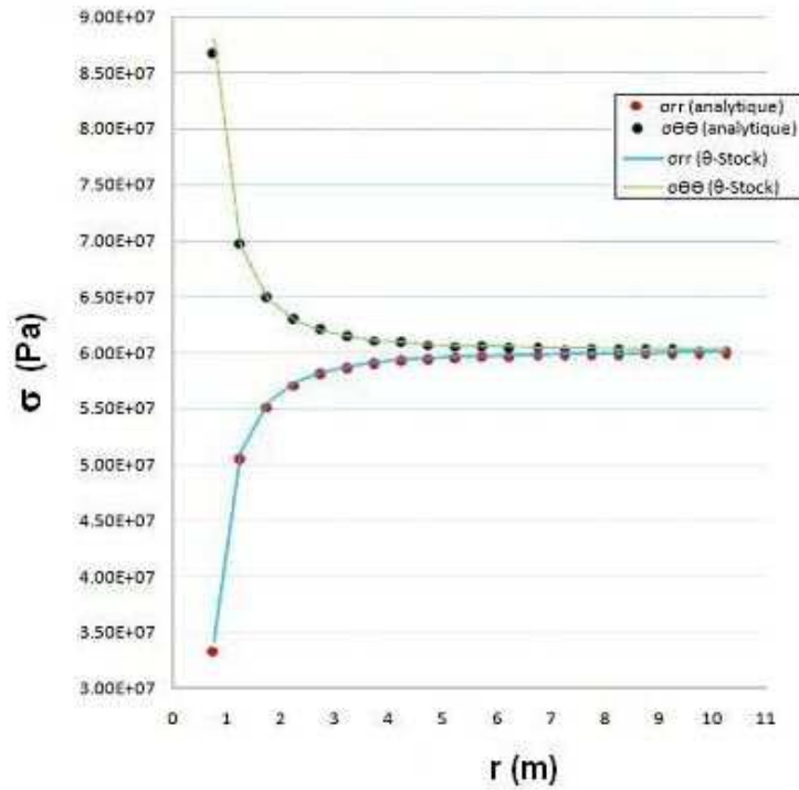
FIGURE 17.3 – Contraintes radiales et orthoradiales développées autour d'un tunnel en élasticité.
