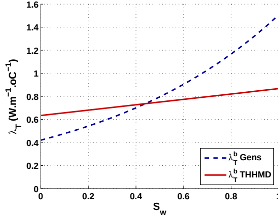
FIGURE 17.47 – Approximation du modèle de conductivité thermique de Gens [79] par le modèle THHMD pour la bentonite.
