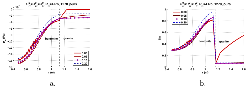
FIGURE 17.59 – Test in situ FEBEX. Influence de la présence d'endommagement initial isotrope dans la zone Rb \leq r \leq 4 Rb . Observations au voisinage de la frontière entre les barrières ouvragée (en bentonite) et géologique (en granite) après une phase de refroidissement (1278 jours). a. Pression d'eau interstitielle. b. Degré de saturation.
