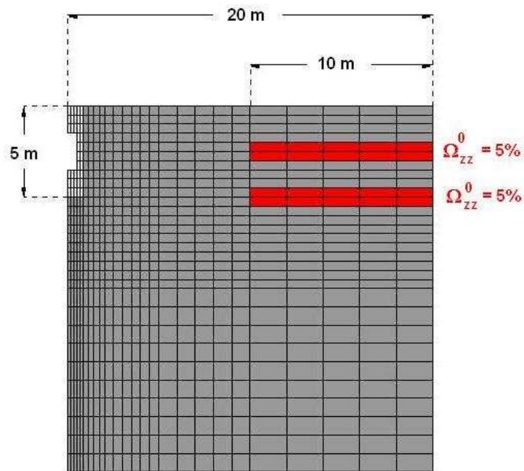
FIGURE 17.85 – Etude du problème de stockage de Kamaishi avec un massif granitique initialement endommagé. Cas n^o 1 : deux plans de fissuration horizontaux d’une étendue de 10 mètres.
