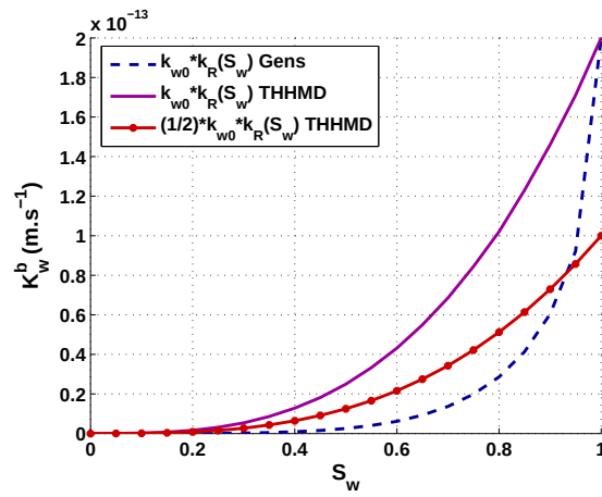
FIGURE 17.46 – Approximation du modèle de perméabilité de Gens [79] par le modèle THHMD pour la bentonite.
