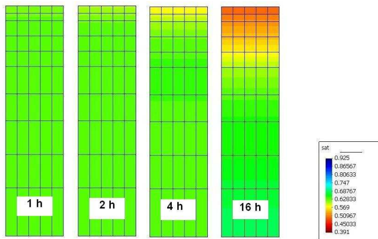
FIGURE 16.29 – Evolution du degré de saturation au début de l'essai de Pintado et al. [161]
