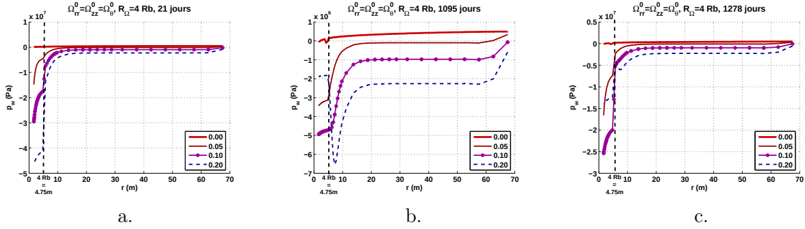
FIGURE 17.56 – Test in situ FEBEX. Influence de la présence d'endommagement initial isotrope dans la zone Rb \leq r \leq 4Rb . Evolution de la pression d'eau interstitielle dans le massif granitique. a. Fin de l'accroissement de température (21 jours). b. Après le plateau de température (1095 jours). c. Après refroidissement (1278 jours).
