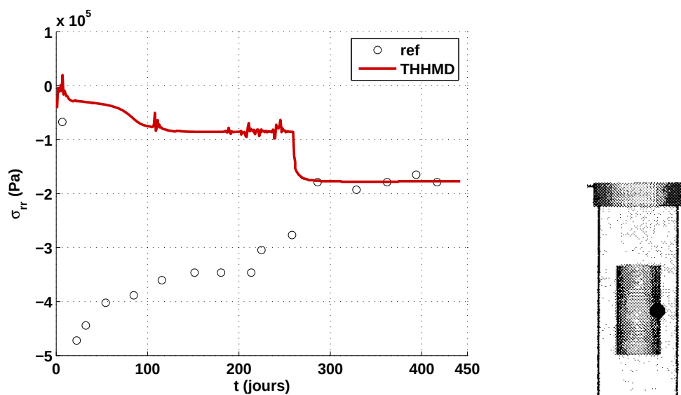
FIGURE 17.83 – Evolution de la contrainte radiale totale au point situé dans la zone de contact entre la source de chaleur et la barrière ouvragée, à mi-hauteur du dispositif de chauffage.
