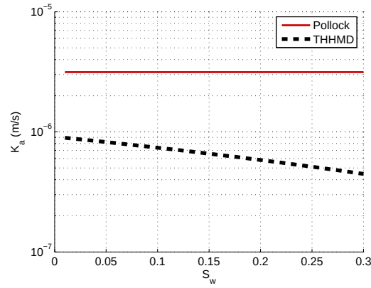
FIGURE 17.28 – Comparaison des perméabilités à l’air du modèle de Pollock [163] et du modèle THHMD ( c_a = 5 * 10^{-12} m^2 , \alpha_a = 2 ).
