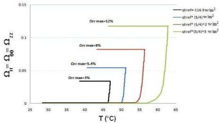
FIGURE 16.33 – Variations de l'endommagement avec le chargement thermique q_h , avec la même rigidité g_M = g_{Mref} = -1.414 \text{ Pa} . Résultats pour un élément en tête de l'échantillon.
