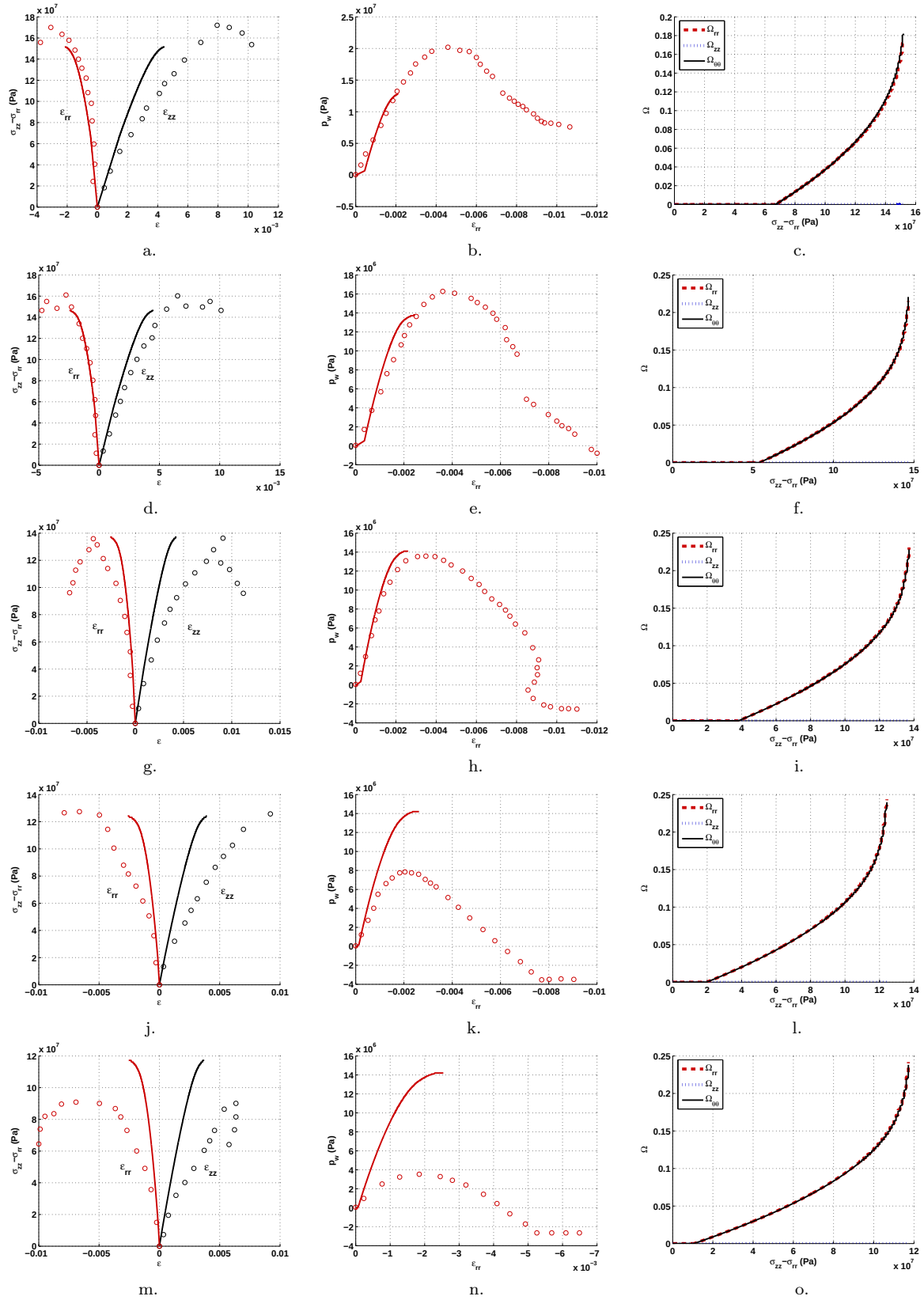
FIGURE 16.13 – Essais de compression triaxiale non drainés sur du grès de Fontainebleau saturé (points : mesures expérimentales [184]; lignes continues : résultats numériques). (a,b,c) p_c = 50 \text{ MPa} . (d,e,f) p_c = 40 \text{ MPa} . (g,h,i) p_c = 28 \text{ MPa} . (j,k,l) p_c = 14 \text{ MPa} . (m,n,o) p_c = 7 \text{ MPa} .
