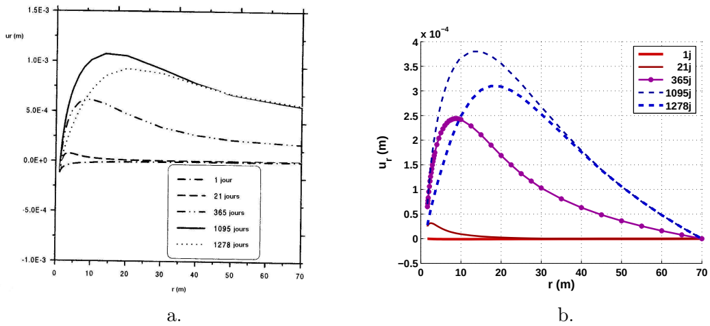
FIGURE 17.54 – Test in situ FEBEX. Evolution du déplacement radial dans la barrière géologique de granite. a. Résultats obtenus avec CODE BRIGHT par Gens et al. [79]. b. Résultats obtenus dans le domaine élastique du modèle THHMD avec \Theta -Stock.
