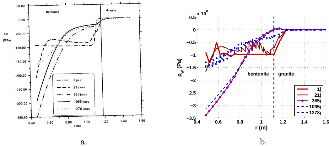
FIGURE 17.51 – Test in situ FEBEX. Evolution de la pression d’eau interstitielle dans la barrière ouvragée de bentonite. a. Résultats obtenus avec CODE BRIGHT par Gens et al. [79]. b. Résultats obtenus dans le domaine élastique du modèle THHMD avec \Theta -Stock.
