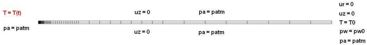
FIGURE 17.45 – Conditions aux limites imposées dans la simulation du test in situ FEBEX [79].
