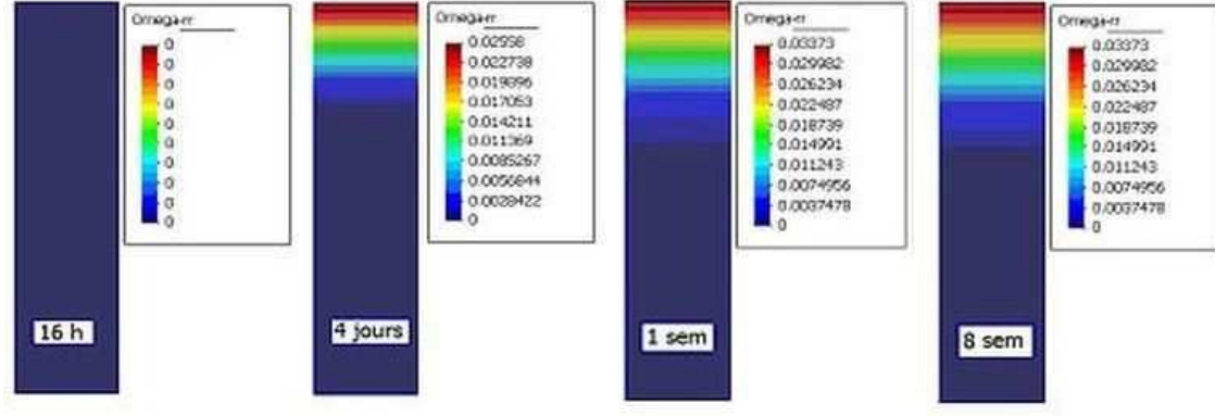
FIGURE 16.31 – Evolution spatio-temporelle de l'endommagement radial dans l'échantillon de bentonite pour g_M = g_{Mref} = -1.414 Pa et q_h = 116.9 W.m^{-2} .
