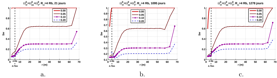
FIGURE 17.57 – Test in situ FEBEX. Influence de la présence d'endommagement initial isotrope dans la zone Rb \leq r \leq 4Rb . Evolution du degré de saturation dans le massif granitique. a. Fin de l'accroissement de température (21 jours). b. Après le plateau de température (1095 jours). c. Après refroidissement (1278 jours).
