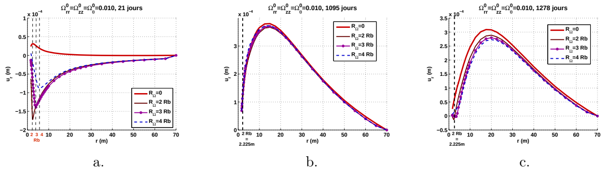
FIGURE 17.65 – Test in situ FEBEX. Influence de la présence d’un endommagement initial isotrope de 10 pour cent dans une zone d’étendue variable. Evolution du déplacement radial dans le massif granitique. a. Fin de l’accroissement de température (21 jours). b. Après le plateau de température (1095 jours). c. Après refroidissement (1278 jours).
