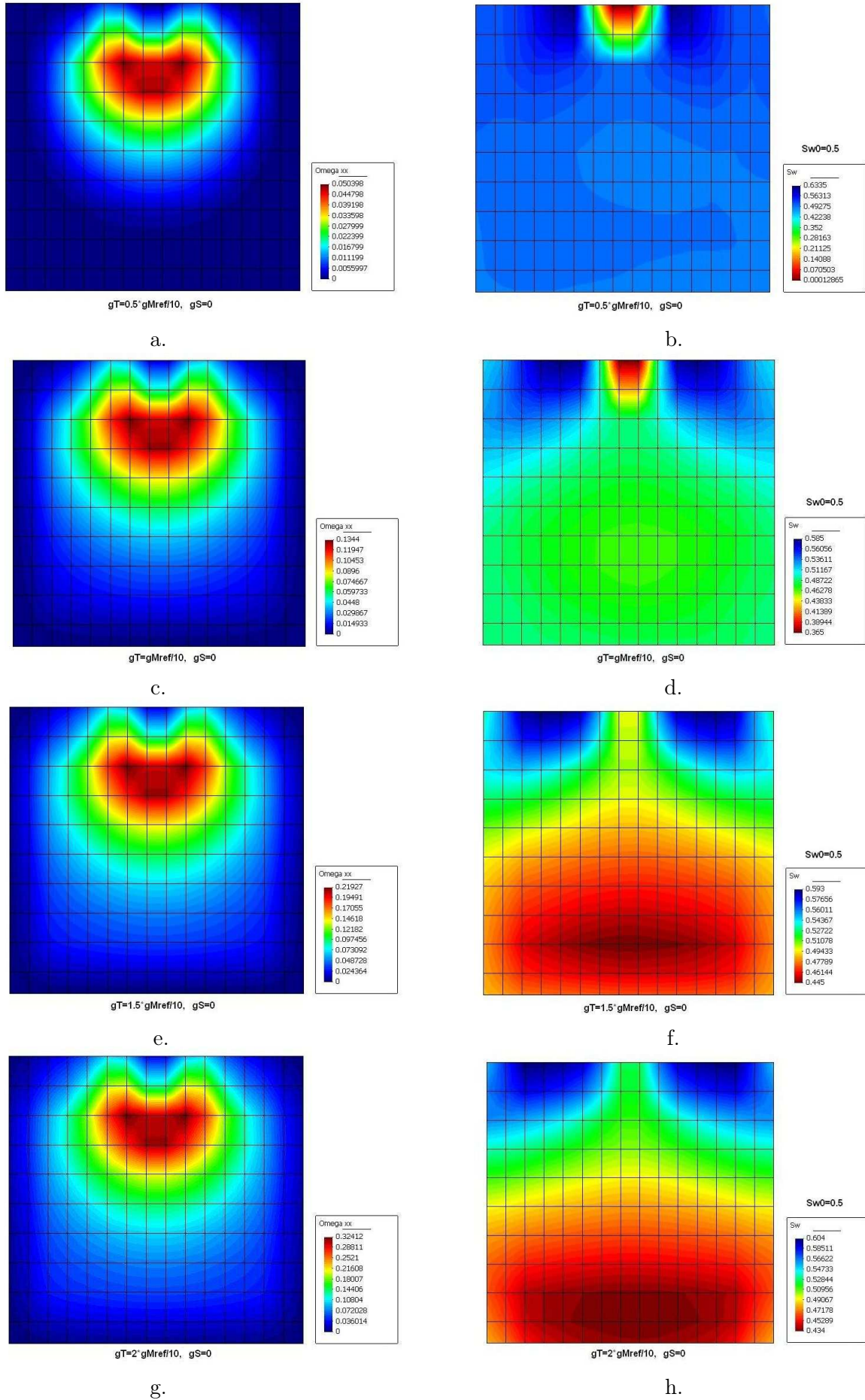
FIGURE 16.46 – Influence de g_T sur l'endommagement ( \Omega_{xx} = \Omega_{yy} ) et sur le degré de saturation, après 2h de chauffage. Fissuration thermique ( g_S = 0 ).
