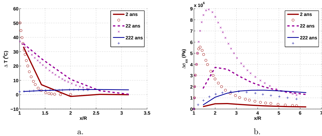
FIGURE 17.14 – Etat thermo-mécanique du massif à proximité du paquet radioactif. Etude en déformations planes. a. Evolution de la température. b. Variation de contrainte « radiale ». Points : résultats obtenus par Carter et Booker [32]. Lignes continues : résultats numériques obtenus avec \Theta -Stock dans le domaine élastique du modèle THMD sur les éléments situés à la base du modèle.
