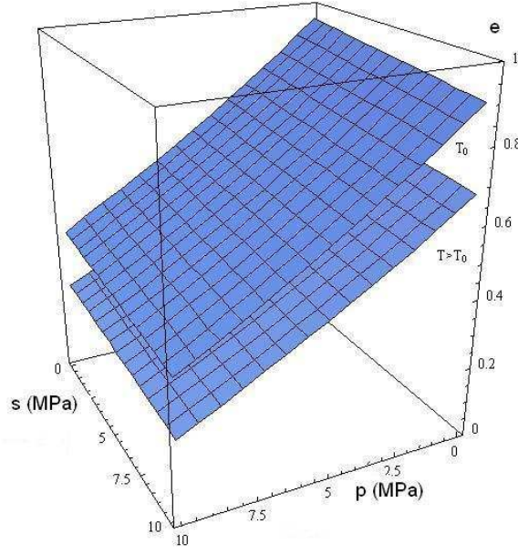
FIGURE 2.2 – Surface d'état thermique de l'indice des vides dans le modèle de Gatmiri [76, 70]. a_e = 1.5 , b_e = 0.15 , c_e = -3 \cdot 10^{-4} \text{ } ^\circ\text{C}^{-1} , \sigma_c = 800 \text{ kPa} .
