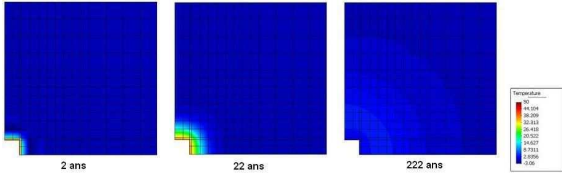
FIGURE 17.15 – Evolution spatio-temporelle de la température dans le problème de stockage des déchets radioactifs [32] traité en déformations planes.
