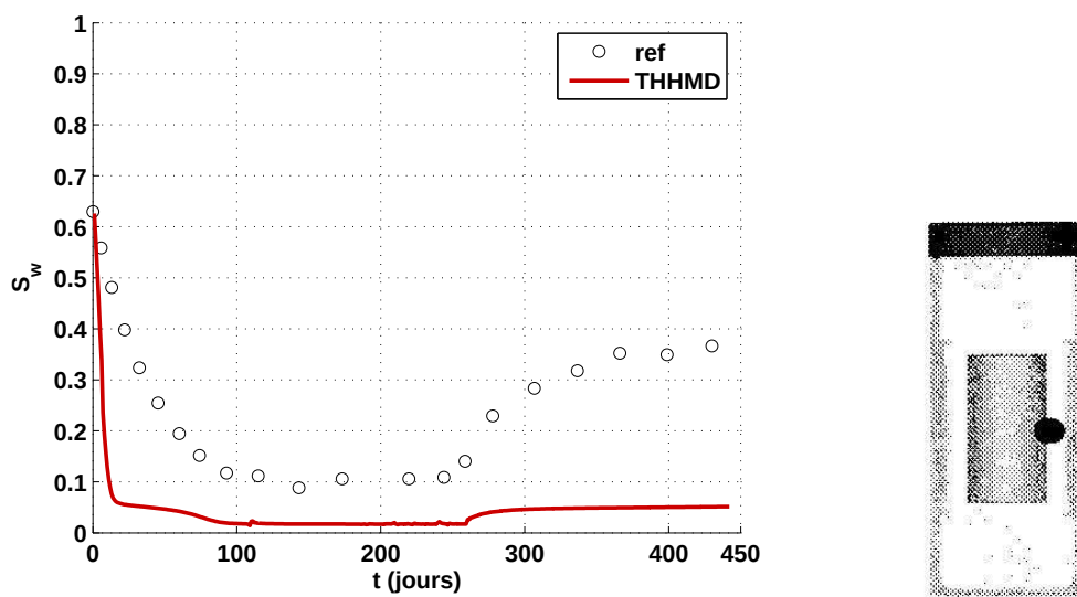
FIGURE 17.82 – Evolution du degré de saturation au point situé dans la zone de contact entre la source de chaleur et la barrière ouvragée, à mi-hauteur du dispositif de chauffage.
