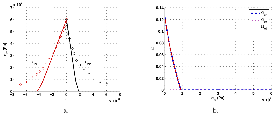
FIGURE 16.9 – Essai d'extension latérale effectué sur l'argilite de l'Est ( p_c^{init} = 60 \text{ MPa} ). a. Evolution des déformations (points : résultats expérimentaux ; lignes continues : résultats numériques). b. Evolution de l'endommagement.
