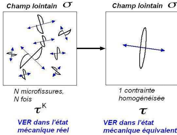
FIGURE 5.1 – Concept d'état mécanique équivalent.
