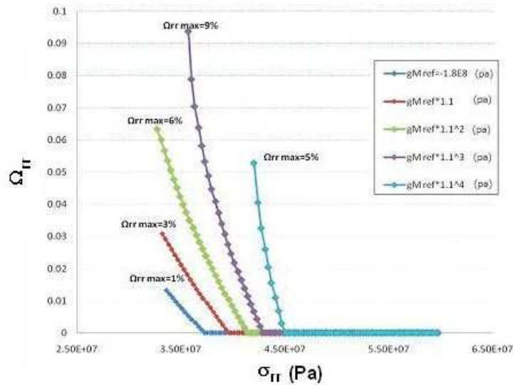
FIGURE 17.4 – Tendances de l'endommagement lors du déchargement mécanique de la paroi d'un tunnel creusé dans du granite sec.
