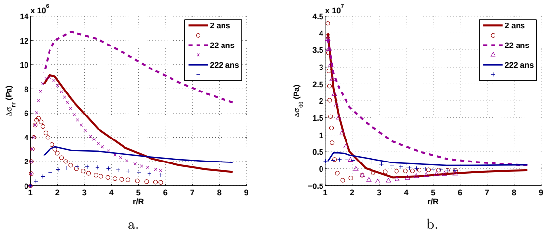
FIGURE 17.13 – Evolution des contraintes dans le massif à proximité du paquet radioactif. Etude axisymétrique pseudo-unidimensionnelle. a. Variation de contrainte radiale. b. Variation de contrainte circonférentielle. Points : résultats obtenus par Carter et Booker [32]. Lignes continues : résultats numériques obtenus avec \Theta -Stock dans le domaine élastique du modèle THHMD.
