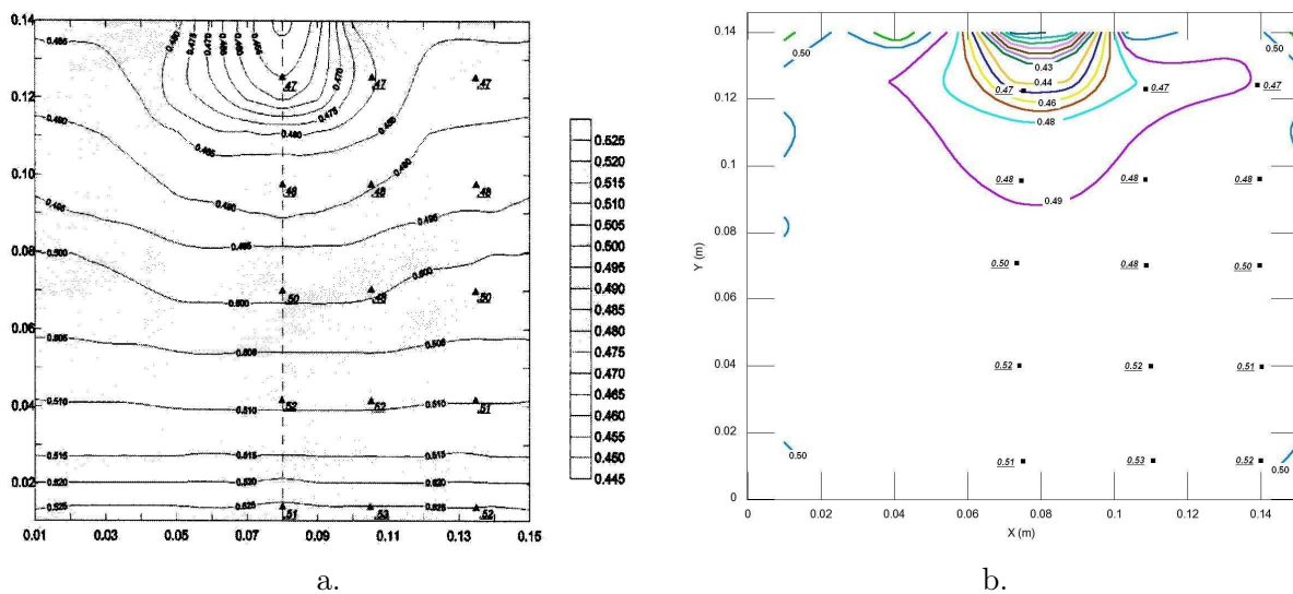
FIGURE 16.44 – Distribution spatiale du degré de saturation après 2h de chauffage (isochrones pour les résultats numériques, points pour les mesures expérimentales [201]). a. Modèle à surfaces d'état [102]. b. Modèle THHMD.
