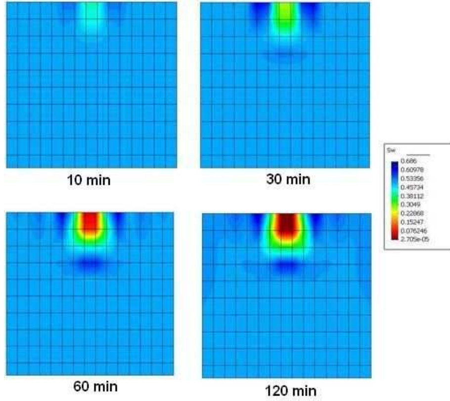
FIGURE 16.45 – Evolution spatio-temporelle du degré de saturation pendant la simulation de l'essai de chauffage de Villar et al. [201], dans le domaine élastique du modèle THHMD.
