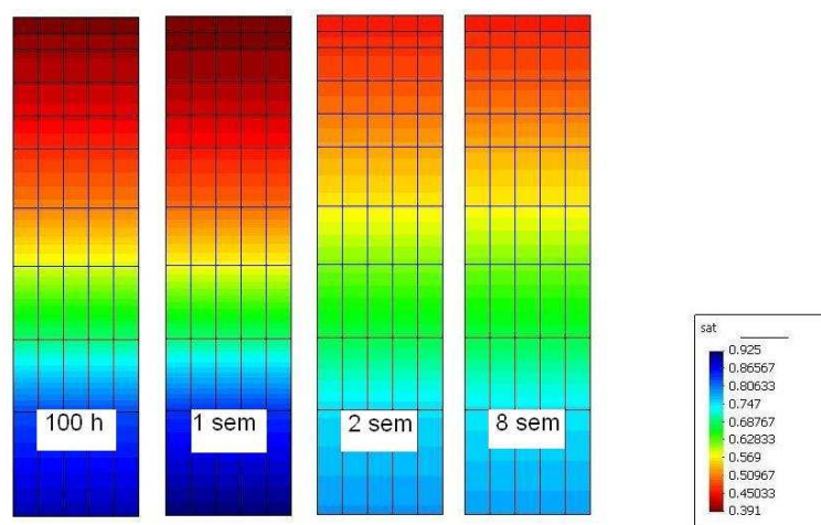
FIGURE 16.30 – Evolution du degré de saturation à la fin de l'essai de Pintado et al. [161]
