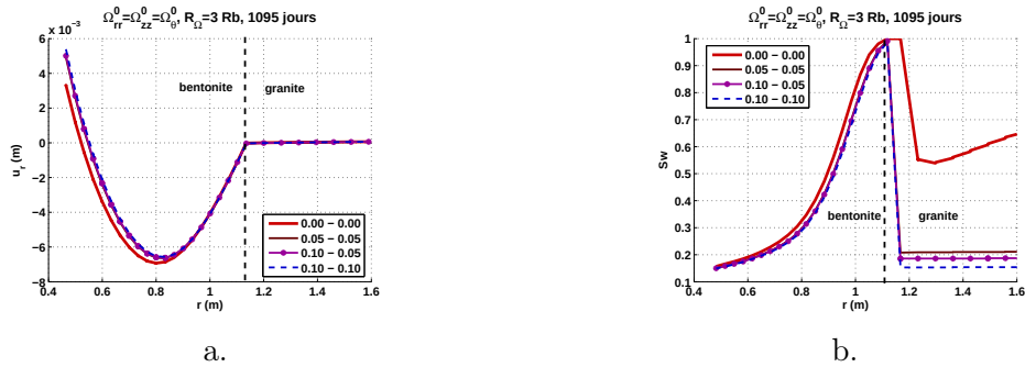
FIGURE 17.63 – Test in situ FEBEX. Influence de la présence d'endommagement initial isotrope dans la zone Rb \leq r \leq 3 Rb , avec deux zones d'endommagement : Rb \leq r \leq 2 Rb et 2 Rb \leq r \leq 3 Rb . Observations au voisinage de la frontière entre les barrières ouvragée (en bentonite) et géologique (en granite) après le plateau de température (1095 jours). a. Déplacement radial. b. Degré de saturation.
