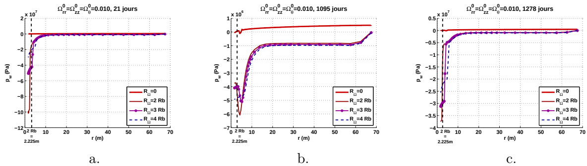
FIGURE 17.66 – Test in situ FEBEX. Influence de la présence d’un endommagement initial isotrope de 10 pour cent dans une zone d’étendue variable. Evolution de la pression d’eau interstitielle dans le massif granitique. a. Fin de l’accroissement de température (21 jours). b. Après le plateau de température (1095 jours). c. Après refroidissement (1278 jours).
