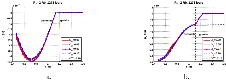
FIGURE 17.71 – Test in situ FEBEX. Influence de la présence d'un endommagement initial radial entre r = Rb et r = 2Rb sur le comportement de la bentonite. Etat de la barrière ouvragée après la phase de refroidissement (1278 jours). a. Déplacement radial. b. Pression d'eau interstitielle.
