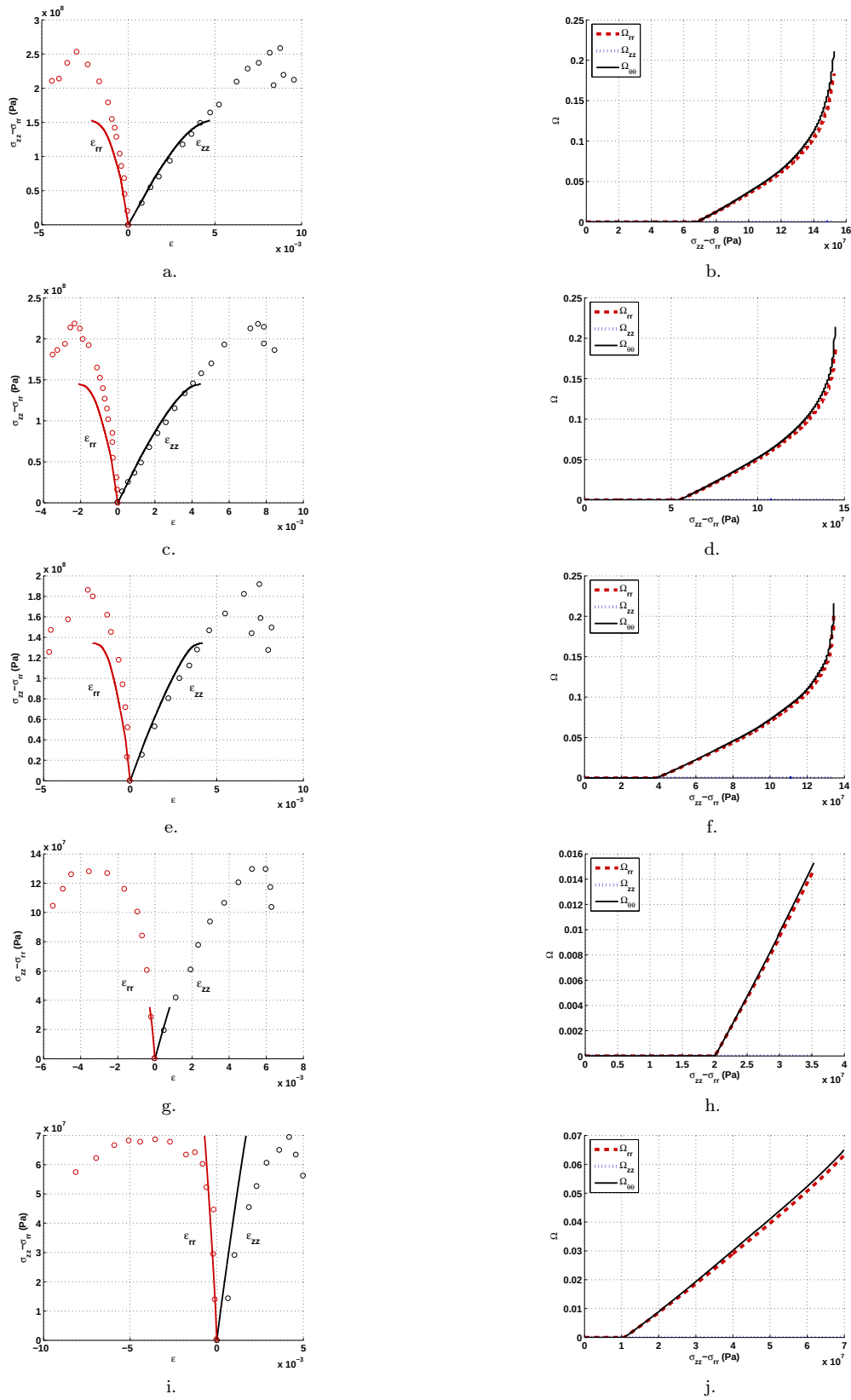
FIGURE 16.15 – Essais de compression triaxiale drainés sur du grès de Fontainebleau saturé (points : résultats expérimentaux [184]; lignes continues : résultats numériques). (a,b) p_c = 50 \text{ MPa} . (c,d) p_c = 40 \text{ MPa} . (e,f) p_c = 28 \text{ MPa} . (g,h) p_c = 14 \text{ MPa} . (i,j) p_c = 7 \text{ MPa} .
