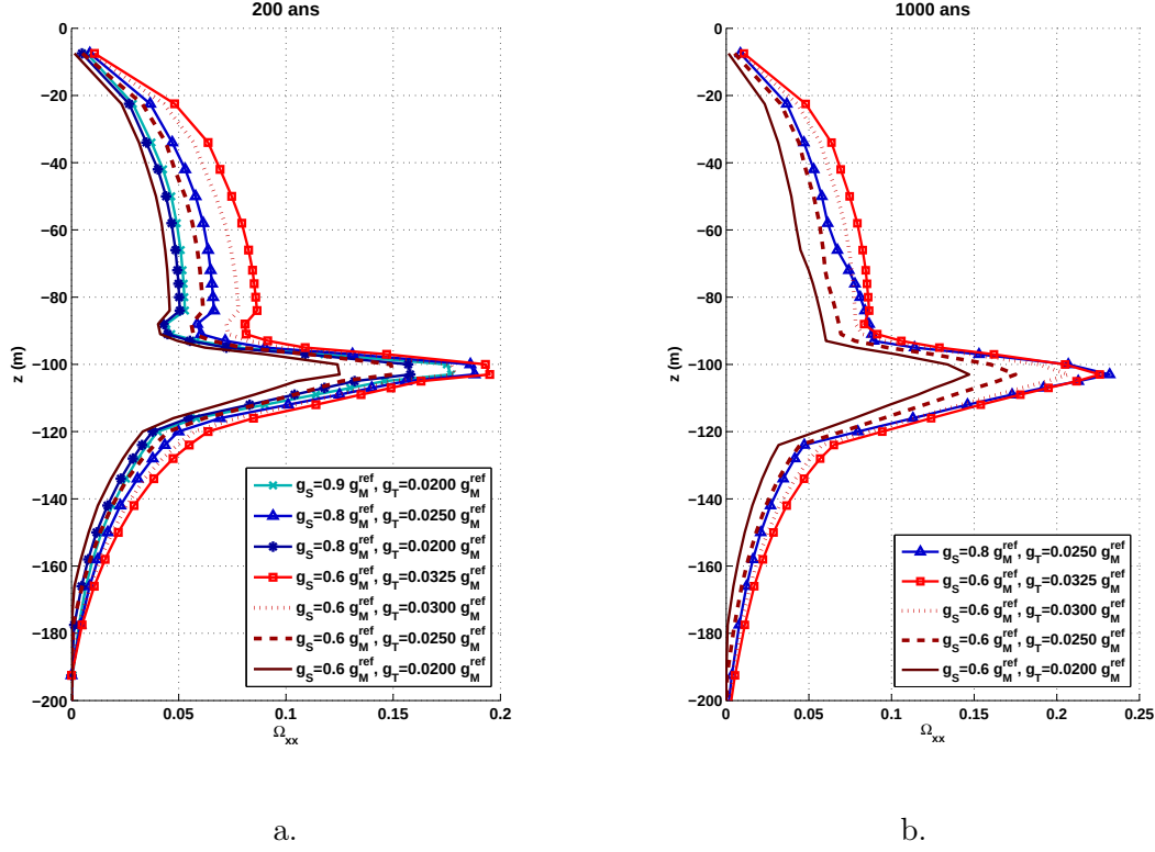
FIGURE 17.43 – Influence conjointe des rigidités g_S et g_T sur le développement de l'endommagement dans le problème de stockage des déchets radioactifs traité par Pollock [163]. a. Endommagement généré au bout de 200 ans de stockage ( \Omega_{xx} = \omega y y ). b. Endommagement généré au bout de 1000 ans de stockage ( \Omega_{xx} = \omega y y ).
