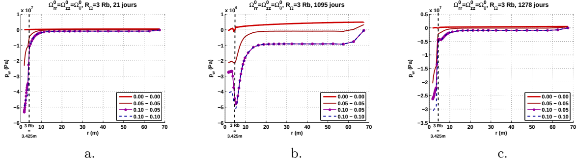
FIGURE 17.61 – Test in situ FEBEX. Influence de la présence d'endommagement initial isotrope dans la zone Rb \leq r \leq 3 Rb , avec deux zones d'endommagement : Rb \leq r \leq 2 Rb et 2 Rb \leq r \leq 3 Rb . Evolution de la pression d'eau interstitielle dans le massif granitique. a. Fin de l'accroissement de température (21 jours). b. Après le plateau de température (1095 jours). c. Après refroidissement (1278 jours).
