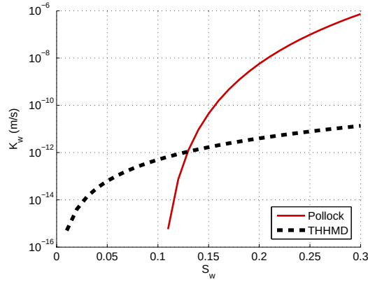
FIGURE 17.27 – Comparaison des perméabilités à l’eau du modèle de Pollock [163] et du modèle THHMD ( S_{w,r} = 0 , \alpha_w = 0 , k_{w0} = 5 * 10^{-10} m.s^{-1} ).
