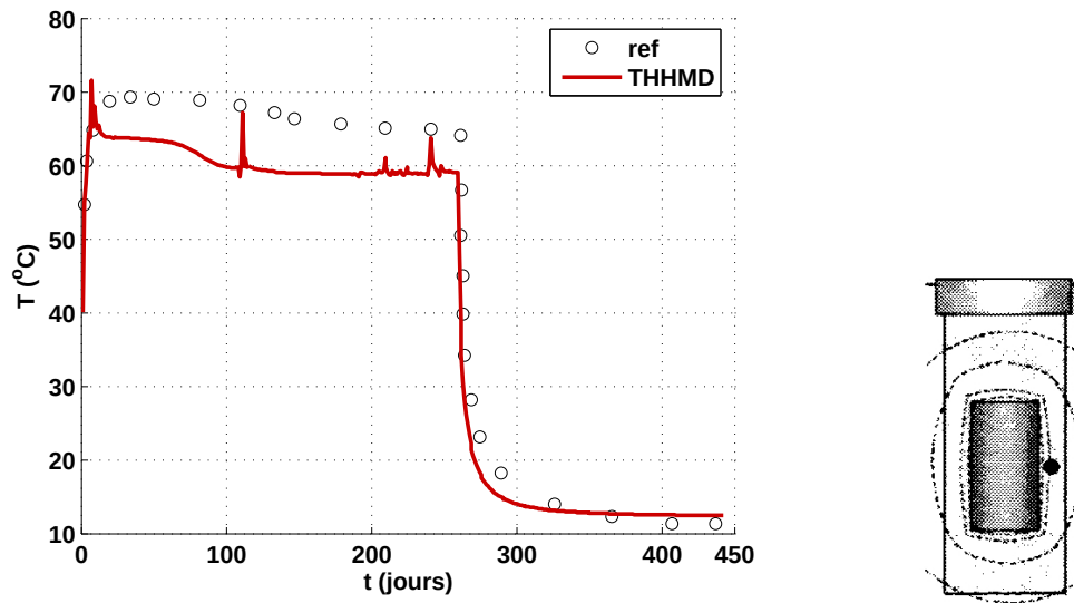
FIGURE 17.79 – Evolution de la température au point situé dans la bentonite, à mi-distance entre la source de chaleur et le massif granitique, à mi-hauteur du dispositif de chauffage.
