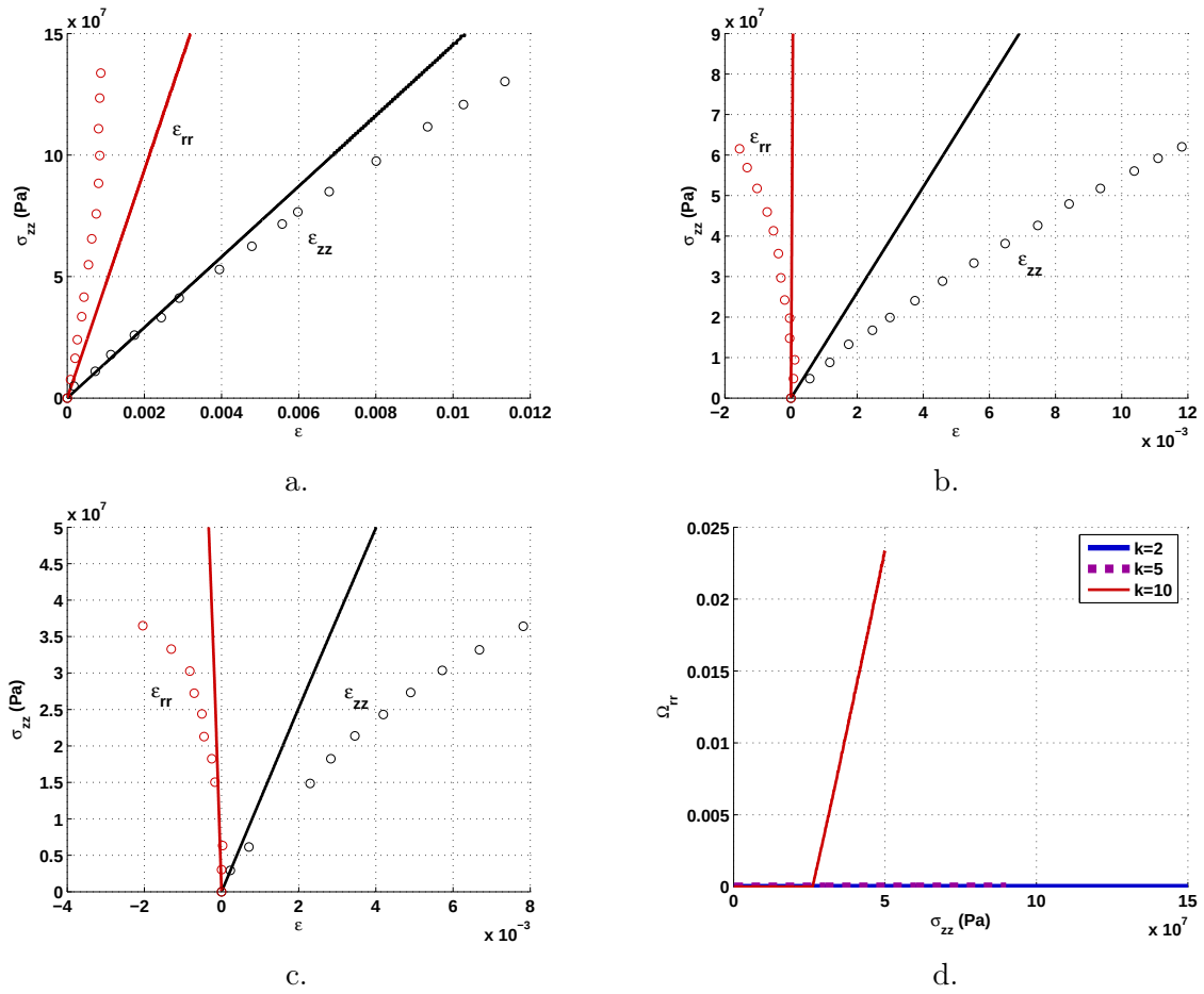
FIGURE 16.8 – Evolution des déformations lors des essais de compression proportionnelle effectués sur l'argilite de l'Est (points : résultats expérimentaux ; lignes continues : résultats numériques). a. k = 2 . b. k = 5 . c. k = 10 . d. Endommagement radial développé pendant les essais de compression proportionnelle.
