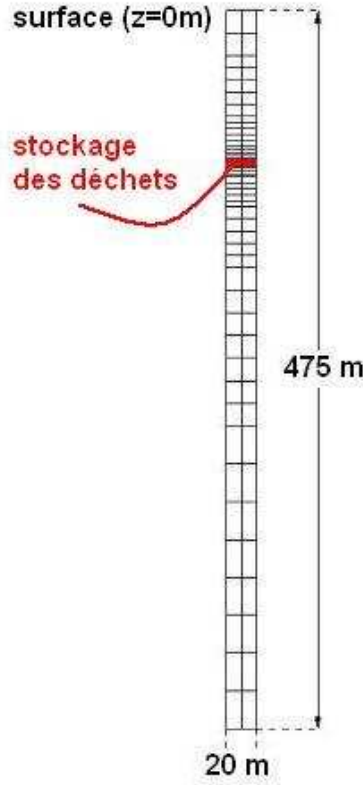
FIGURE 17.25 – Maillage adopté pour traiter le problème de stockage des déchets radioactifs étudié par Pollock [163].
