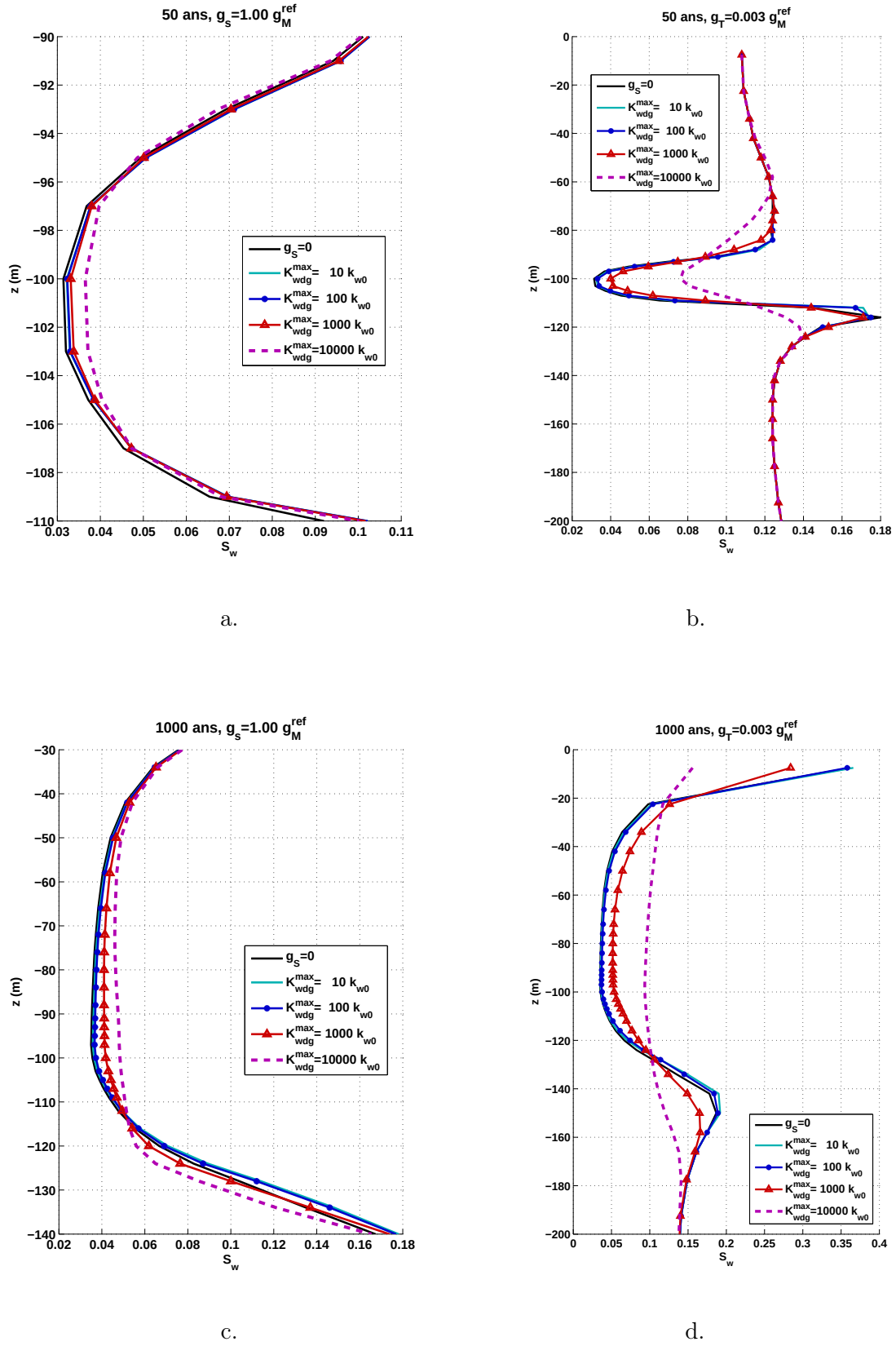
FIGURE 17.38 – Influence de la perméabilité intrinsèque endommagée maximale sur le degré de saturation dans le problème de stockage de déchets radioactifs de Pollock [163]. a,c. g_s = g_M^{ref} , g_T = 0 . b,d. g_T = 0.003 g_M^{ref} , g_s = 0 .
