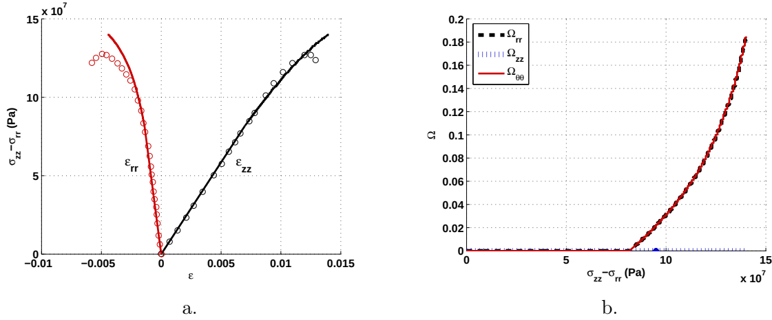
FIGURE 16.10 – Essai de compression triaxiale sur du grès des Vosges ( p_c = 15 \text{ MPa} ). a. Evolution des déformations (points : résultats expérimentaux ; lignes continues : résultats numériques). b. Evolution du tenseur d'endommagement.
