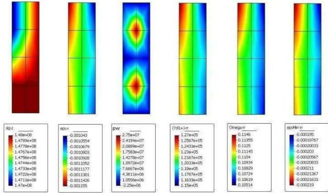
FIGURE 16.16 – Etat mécanique de l'échantillon de grès saturé drainé confiné à 28 MPa et soumis à \sigma_{zz} - \sigma_{rr} = 120 \text{ MPa} en tête.
