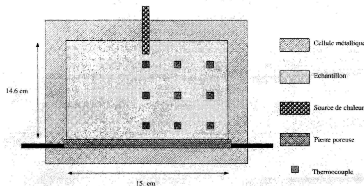
FIGURE 16.34 – Dispositif expérimental de Villar et al. [102, 201].
