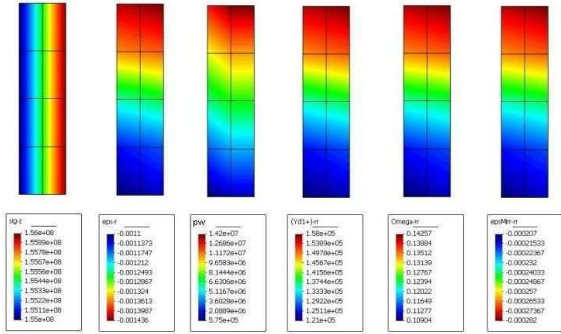
FIGURE 16.12 – Etat mécanique de l'échantillon de grès saturé non drainé confiné à 28 MPa et soumis à \sigma_{zz} - \sigma_{rr} = 127.5 \text{ MPa} en tête.
