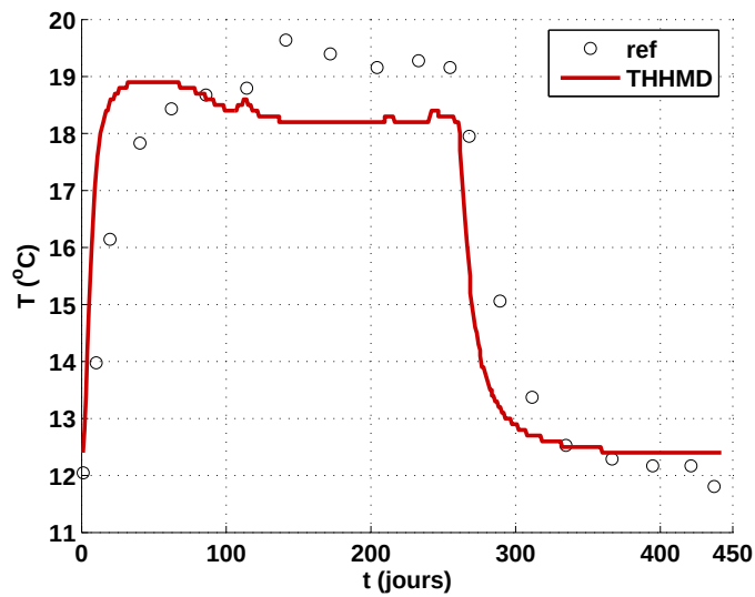
FIGURE 17.80 – Evolution de la température en un point situé dans le massif granitique, à proximité de la barrière ouvragée.
