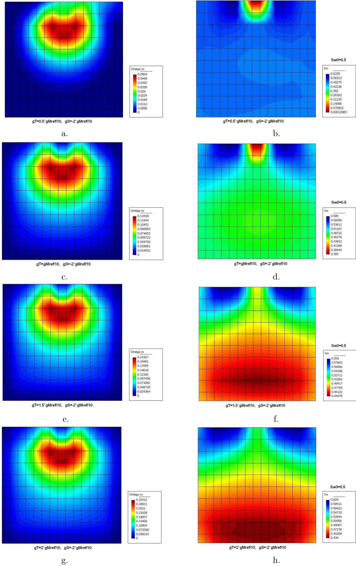
FIGURE 16.48 – Influence de g_T sur l'endommagement ( \Omega_{xx} = \Omega_{yy} ) et sur le degré de saturation, après 2h de chauffage. Fissuration thermo-capillaire ( g_S \neq 0 ).
