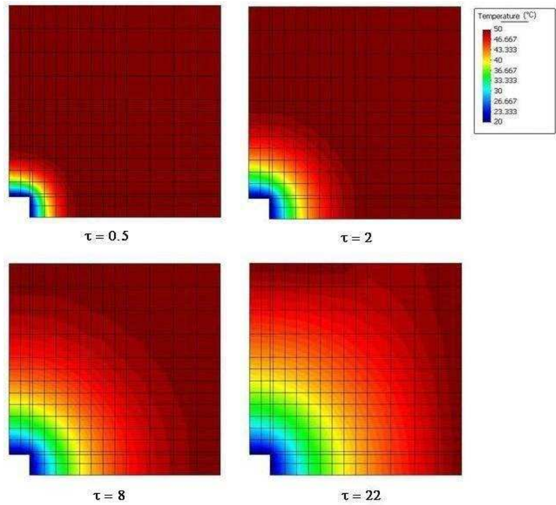
FIGURE 17.7 – Evolution spatio-temporelle des températures nodales calculées avec \Theta -Stock dans problème de refroidissement d'une galerie profonde de section carrée [32]. \tau = \frac{\lambda_s}{\rho_s C_{Ps}} \frac{t}{(a/2)^2} .
