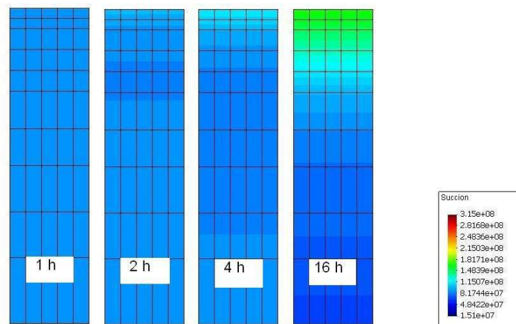
FIGURE 16.27 – Evolution de la succion au début de l'essai de Pintado et al. [161]
