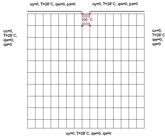
FIGURE 16.38 – Conditions aux limites adoptées pour reproduire l'essai de Villar et al. [201]
