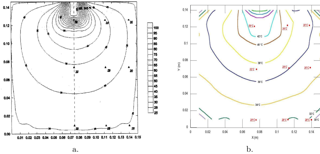
FIGURE 16.39 – Distribution spatiale de la température après 2h de chauffage (isochrones pour les résultats numériques, points pour les mesures expérimentales [201]). a. Modèle à surfaces d'état [102]. b. Modèle THHMD.
