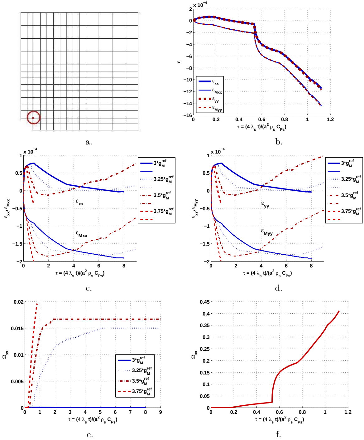
FIGURE 17.9 – Comportement fragile du massif dans le problème de refroidissement d'un tunnel de section carrée [32]. a. Elément choisi pour l'étude paramétrique. b. Déformations pour g_M = 4 g_M^{ref} . c. Déformations « horizontales » pour 3 g_M^{ref} \leq g_M \leq 3.75 g_M^{ref} . d. Déformations « verticales » pour 3 g_M^{ref} \leq g_M \leq 3.75 g_M^{ref} . e. Endommagement « horizontal » pour 3 g_M^{ref} \leq g_M \leq 3.75 g_M^{ref} . f. Endommagement « horizontal » pour g_M = 4 g_M^{ref} .
