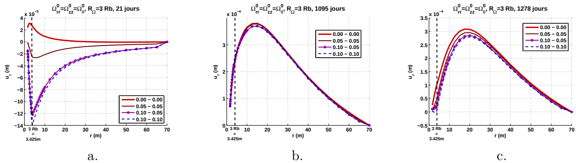
FIGURE 17.60 – Test in situ FEBEX. Influence de la présence d'endommagement initial isotrope dans la zone Rb \leq r \leq 3 Rb , avec deux zones d'endommagement : Rb \leq r \leq 2 Rb et 2 Rb \leq r \leq 3 Rb . Evolution du déplacement radial dans le massif granitique. a. Fin de l'accroissement de température (21 jours). b. Après le plateau de température (1095 jours). c. Après refroidissement (1278 jours).
