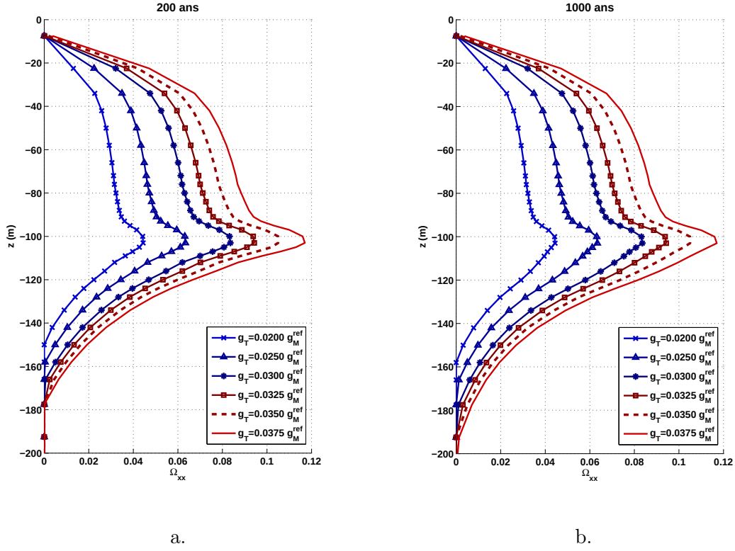
FIGURE 17.42 – Influence de la rigidité g_T sur le développement de l'endommagement dans le problème de stockage des déchets radioactifs traité par Pollock [163]. g_S = 0 . a. Endommagement généré au bout de 200 ans de stockage ( \Omega_{xx} = \omega yy ). b. Endommagement généré au bout de 1000 ans de stockage ( \Omega_{xx} = \omega yy ).
