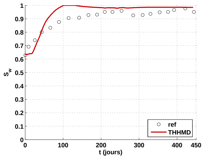
FIGURE 17.81 – Evolution du degré de saturation en un point situé dans la barrière ouvragée en bentonite, à environ un centimètre du massif géologique, au-dessus du dispositif de chauffage.
