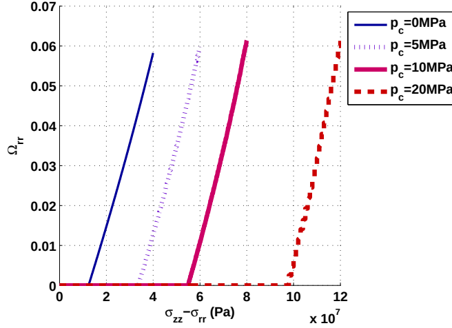
FIGURE 16.7 – Evolution de l'endommagement radial lors des essais de compression triaxiale réalisés sur l'argilite de l'Est.
