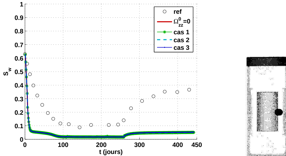
FIGURE 17.89 – Etude du problème de stockage de Kamaishi avec un massif granitique initialement endommagé. Evolution du degré de saturation au point situé dans la zone de contact entre la source de chaleur et la barrière ouvragée, à mi-hauteur du dispositif de chauffage.
