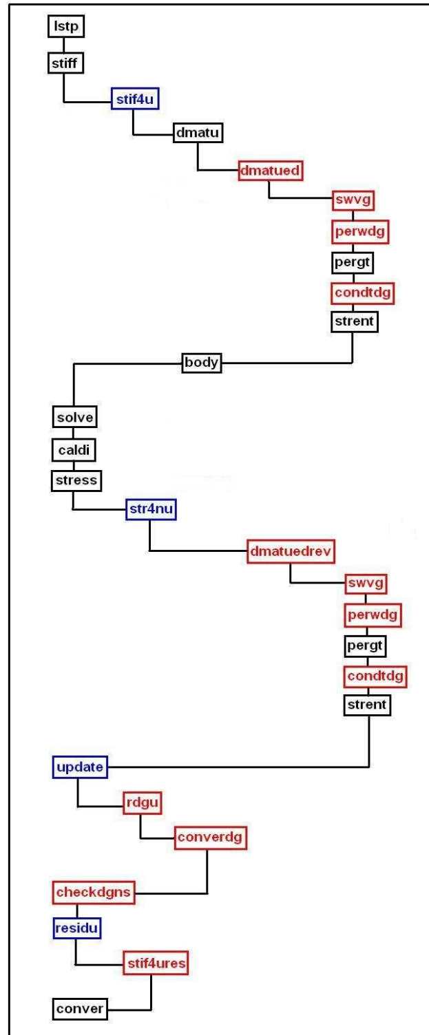
FIGURE 13.1 – Subroutines intervenant lors d’une simulation effectuée avec le modèle THHMD dans \Theta -Stock, pendant le calcul itératif. Un décalage vers la droite correspond à une servitude (les subroutines appelées sont plus à droite que leur subroutine mère). En rouge : les subroutines spécifiques au modèle THHMD. En bleu : les subroutines préexistantes fortement affectées par l’implantation du modèle THHMD. En noir : les subroutines peu ou pas affectées par l’intégration du modèle d’endommagement dans \Theta -Stock.
