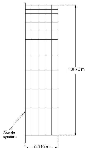
FIGURE 16.19 – Maillage adopté pour le test de chauffage de la bentonite de Pintado et al. [161]
