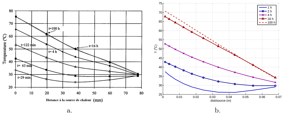
FIGURE 16.22 – Isochrones de température lors de l'essai de Pintado et al. a. Mesures expérimentales [161]. b. Résultats numériques.
