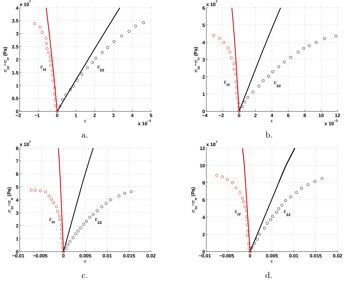
FIGURE 16.6 – Evolution des déformations lors des essais de compression triaxiale effectués sur l'argilite de l'Est (points : résultats expérimentaux ; lignes continues : résultats numériques). a. p_c = 0 \text{ MPa} . b. p_c = 5 \text{ MPa} . c. p_c = 10 \text{ MPa} . d. p_c = 20 \text{ MPa} .
