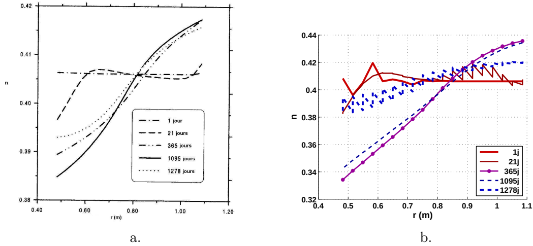
FIGURE 17.52 – Test in situ FEBEX. Evolution de la porosité dans la barrière ouvragée de bentonite. a. Résultats obtenus avec CODE BRIGHT par Gens et al. [79]. b. Résultats obtenus dans le domaine élastique du modèle THHMD avec \Theta -Stock.
