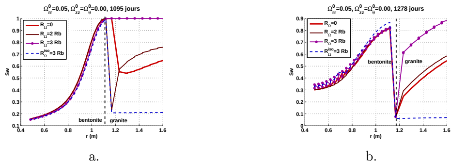
FIGURE 17.75 – Test in situ FEBEX. Influence de la présence d'un endommagement initial radial de 5 pour cent dans une zone d'étendue variable sur le degré de saturation de la barrière ouvragée en bentonite. a. Après le plateau de température (1095 jours). b. Après refroidissement (1278 jours).
