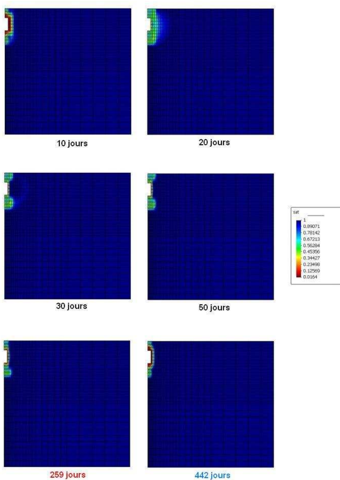
FIGURE 17.91 – Evolution spatio-temporelle du degré de saturation dans la simulation du test de Kamaishi. Cas n^{\circ} 1 (deux plans de fissuration horizontaux d’une étendue de 10 mètres).
