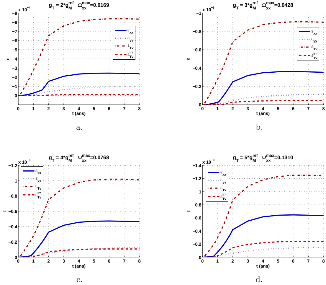
FIGURE 17.23 – Evolution temporelle des déformations dans le problème de stockage des déchets radioactifs en déformations planes. Elément endommagé jouxtant la paroi latérale de l'excavation.
