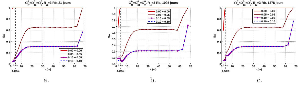
FIGURE 17.62 – Test in situ FEBEX. Influence de la présence d'endommagement initial isotrope dans la zone Rb \leq r \leq 3 Rb , avec deux zones d'endommagement : Rb \leq r \leq 2 Rb et 2 Rb \leq r \leq 3 Rb . Evolution du degré de saturation dans le massif granitique. a. Fin de l'accroissement de température (21 jours). b. Après le plateau de température (1095 jours). c. Après refroidissement (1278 jours).
