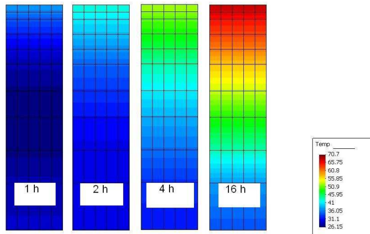
FIGURE 16.25 – Evolution de la température au début de l'essai de Pintado et al. [161]
