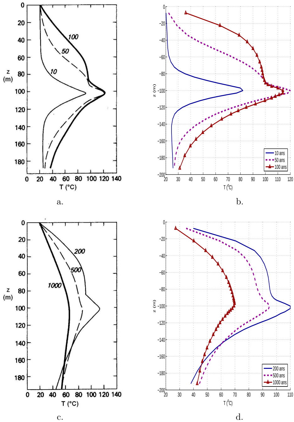
FIGURE 17.30 – Evolution spatio-temporelle de la température. a,c. Résultats de Pollock [163]. b,d. Résultats obtenus dans le domaine élastique du modèle THHMD.
