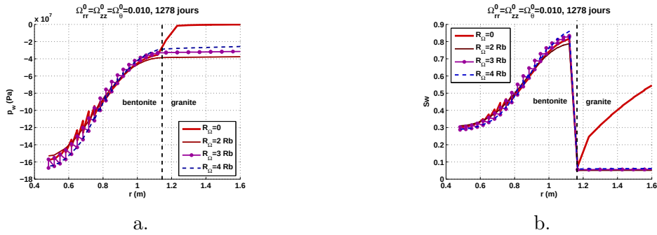
FIGURE 17.69 – Test in situ FEBEX. Influence de la présence d'un endommagement initial isotrope de 10 pour cent dans une zone d'étendue variable. Observations au voisinage de la frontière entre les barrières ouvragée (en bentonite) et géologique (en granite) après une phase de refroidissement (1278 jours). a. Pression d'eau interstitielle. b. Degré de saturation.
