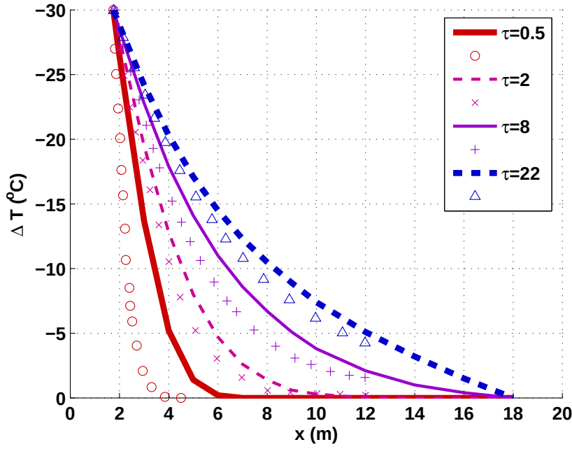
FIGURE 17.6 – Baisse de température observée dans le massif dans le problème de refroidissement d’une galerie profonde de section carrée (de côté a = 3.5m ). \tau = \frac{\lambda_s}{\rho_s C_{Ps}} \frac{t}{(a/2)^2} . Points : résultats obtenus numériquement par Carter et Booker [32]. Lignes continues : températures calculées aux noeuds situés sur le bord inférieur du maillage, dans le domaine élastique du modèle THHMD programmé dans \Theta -Stock.
