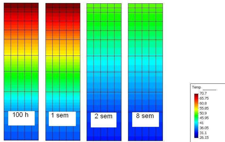
FIGURE 16.26 – Evolution de la température à la fin de l'essai de Pintado et al. [161]
