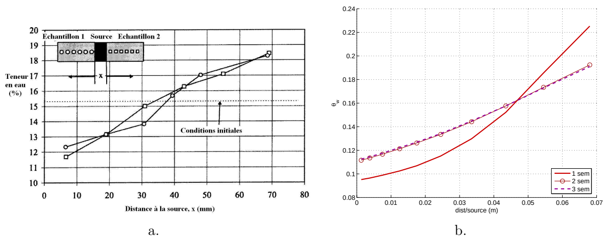
FIGURE 16.24 – Teneurs en eau volumiques après une semaine de chauffage pour l'essai de Pintado et al. a. Mesures expérimentales [161]. b. Résultats numériques.
