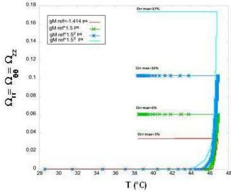
FIGURE 16.32 – Variations de l'endommagement avec la rigidité g_M , sous le même chargement thermique q_h = 116.9 \text{ W.m}^{-2} . Résultats pour un élément en tête de l'échantillon.
