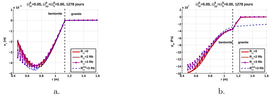
FIGURE 17.74 – Test in situ FEBEX. Influence de la présence d'un endommagement initial radial de 5 pour cent dans une zone d'étendue variable sur le comportement de la bentonite. Etat de la barrière ouvragée après la phase de refroidissement (1278 jours). a. Déplacement radial. b. Pression d'eau interstitielle.
