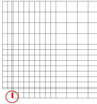
FIGURE 17.21 – Élément choisi pour représenter les résultats de l'étude paramétrique sur le comportement fragile d'un massif géologique sec avoisinant une zone de stockage de déchets radioactifs.
