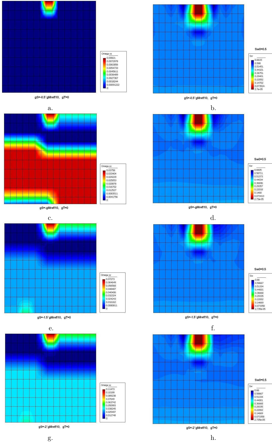
FIGURE 16.47 – Influence de g_S sur l'endommagement ( \Omega_{xx} = \Omega_{yy} ) et sur le degré de saturation, après 2h de chauffage. Fissuration capillaire ( g_T = 0 ).
