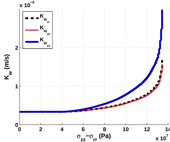
FIGURE 16.17 – Evolution des composantes de la perméabilité à l'eau liquide du grès de Fontainebleau pendant un essai de compression triaxiale drainé ( p_c = 28\text{MPa} ).
