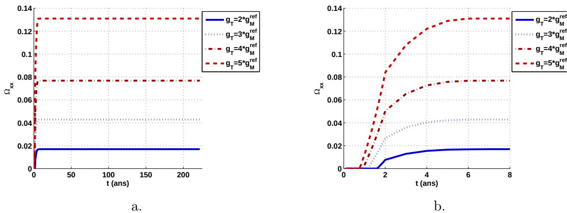
FIGURE 17.22 – Evolution temporelle de la composante horizontale de l'endommagement ( \Omega_{xx} = \Omega_{yy} ) dans le problème de stockage des déchets radioactifs en déformations planes. Élément jouxtant la paroi latérale de l'excavation.
