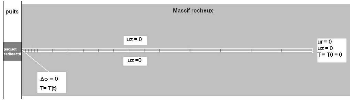
FIGURE 17.10 – Maillage et conditions aux limites pour le problème de stockage de déchets radioactifs dans un massif rocheux sec [32]. Analyse axisymétrique pseudo-unidimensionnelle.
