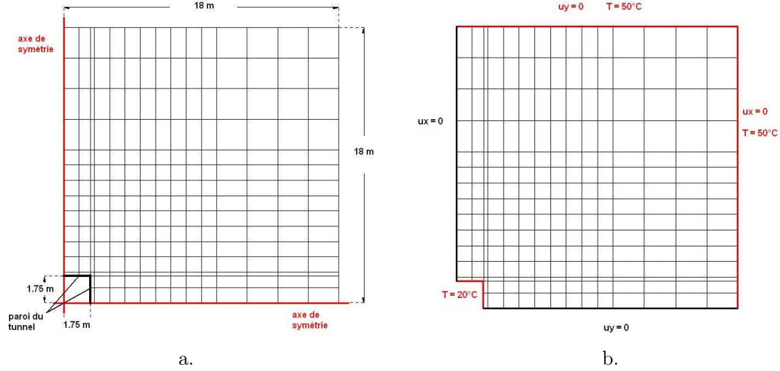
FIGURE 17.5 – Discretisation du problème de refroidissement d'une galerie profonde de section carrée [32]. a. Maillage. b. Conditions aux limites.
