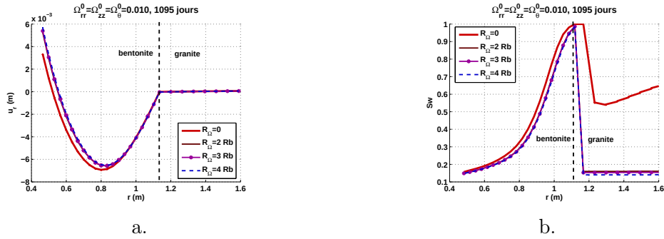
FIGURE 17.68 – Test in situ FEBEX. Influence de la présence d'un endommagement initial isotrope de 10 pour cent dans une zone d'étendue variable. Observations au voisinage de la frontière entre les barrières ouvragée (en bentonite) et géologique (en granite) après le plateau de température (1095 jours). a. Déplacement radial. b. Degré de saturation.
