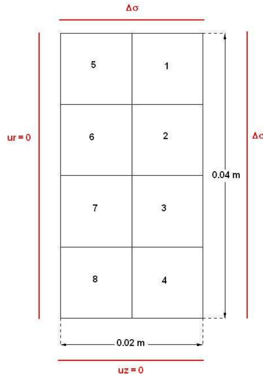
FIGURE 16.1 – Maillage et conditions aux limites adoptés pour les essais mécaniques simulés sur des géomatériaux secs.
