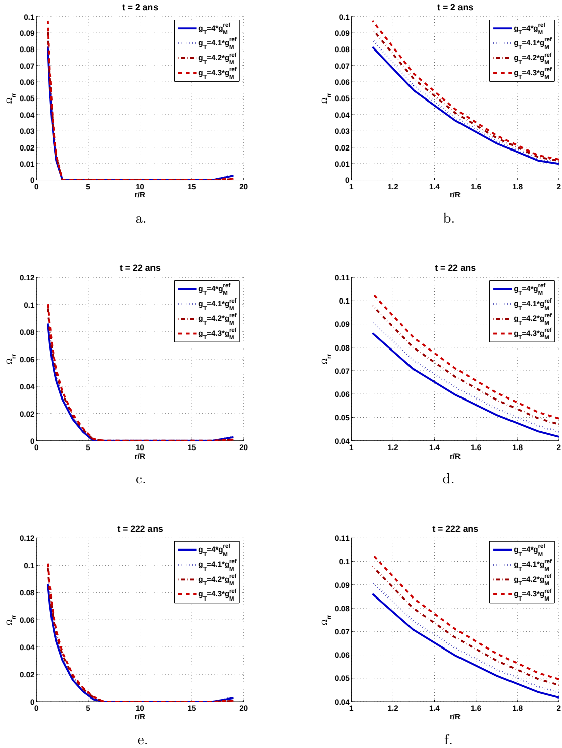
FIGURE 17.18 – Evolution spatiale de l'endommagement radial ( \Omega_{rr} = \Omega_{zz} = \Omega_{\theta\theta} ) dans le problème axisymétrique de stockage des déchets radioactifs, au bout de 2 ans (a,b), 22 ans (c,d) et 222 ans (e,f).
