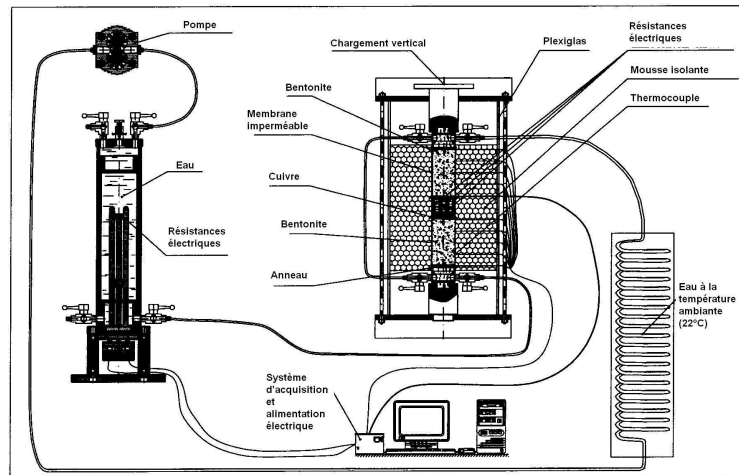
FIGURE 16.18 – Protocole expérimental adopté par Pintado et al. pour l'essai de chauffage de la bentonite [161].
