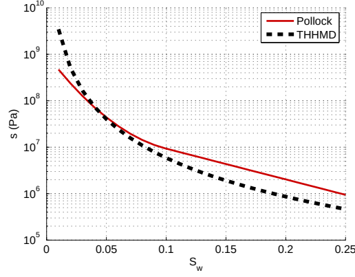
FIGURE 17.26 – Comparaison des courbes de rétention du modèle de Pollock [163] et du modèle THHMD ( S_{w,r} = 0 , \alpha_{VG} = 10^{-4} \text{ Pa}^{-1} , n_{VG} = 1.361 ).
