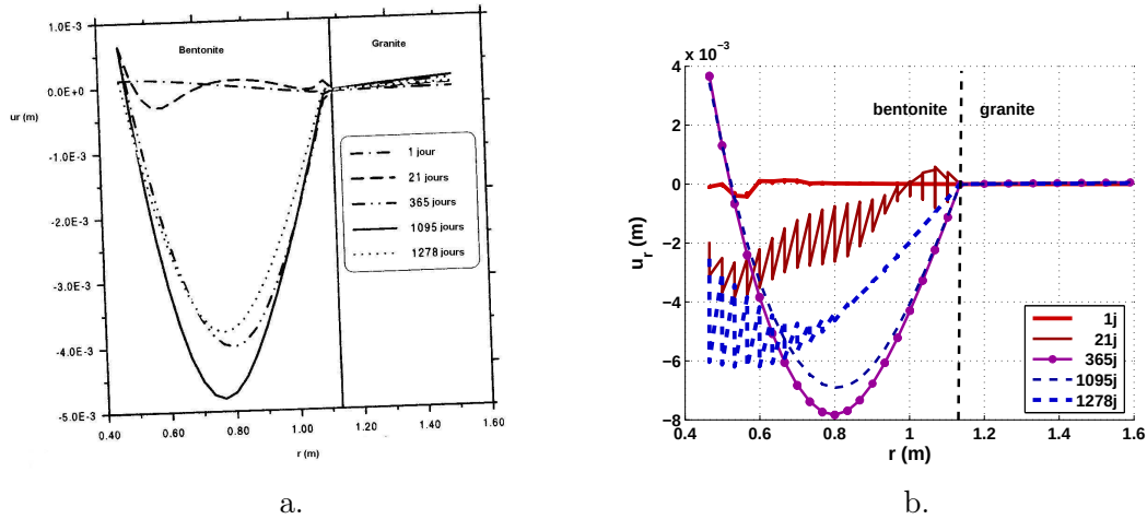
FIGURE 17.53 – Test in situ FEBEX. Evolution du déplacement radial dans la barrière ouvragée de bentonite. a. Résultats obtenus avec CODE BRIGHT par Gens et al. [79]. b. Résultats obtenus dans le domaine élastique du modèle THHMD avec \Theta -Stock.
