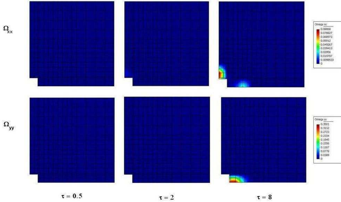
FIGURE 17.8 – Endommagement du massif dans le problème de refroidissement d'un tunnel de section carrée [32], avec g_M = 3.5 g_M^{ref} .
