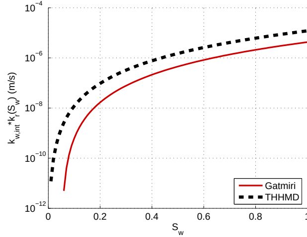
FIGURE 16.37 – Calage de la perméabilité intacte isotherme du modèle THHMD ( k_{w0} = 1.2 * 10^{-5} m.s^{-1} , \alpha_w = 0 , S_{w,r} = 0 ) sur celle du modèle élastique à surfaces d'état de Gatmiri ( k_{w0} = 1.2 * 10^{-9} m.s^{-1} , \alpha_w = 5 , e = e_0 et S_{w,r} = 0.05 ).
