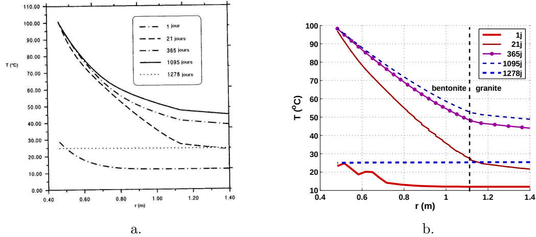
FIGURE 17.48 – Test in situ FEBEX. Evolution de la température dans la barrière ouvragée de bentonite. a. Résultats obtenus avec CODE BRIGHT par Gens et al. [79]. b. Résultats obtenus dans le domaine élastique du modèle THHMD avec \Theta -Stock.
