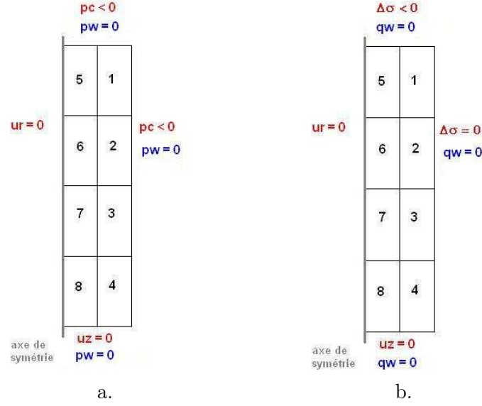
FIGURE 16.11 – Maillage et conditions aux limites adoptés pour simuler des essais de compression triaxiale non drainés sur du grès de Fontainebleau saturé. a. Phase de confinement. b. Phase de compression.
