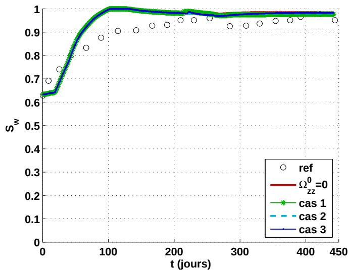
FIGURE 17.88 – Etude du problème de stockage de Kamaishi avec un massif granitique initialement endommagé. Evolution du degré de saturation en un point situé dans la barrière ouvragée en bentonite, à environ un centimètre du massif géologique, au-dessus du dispositif de chauffage.
