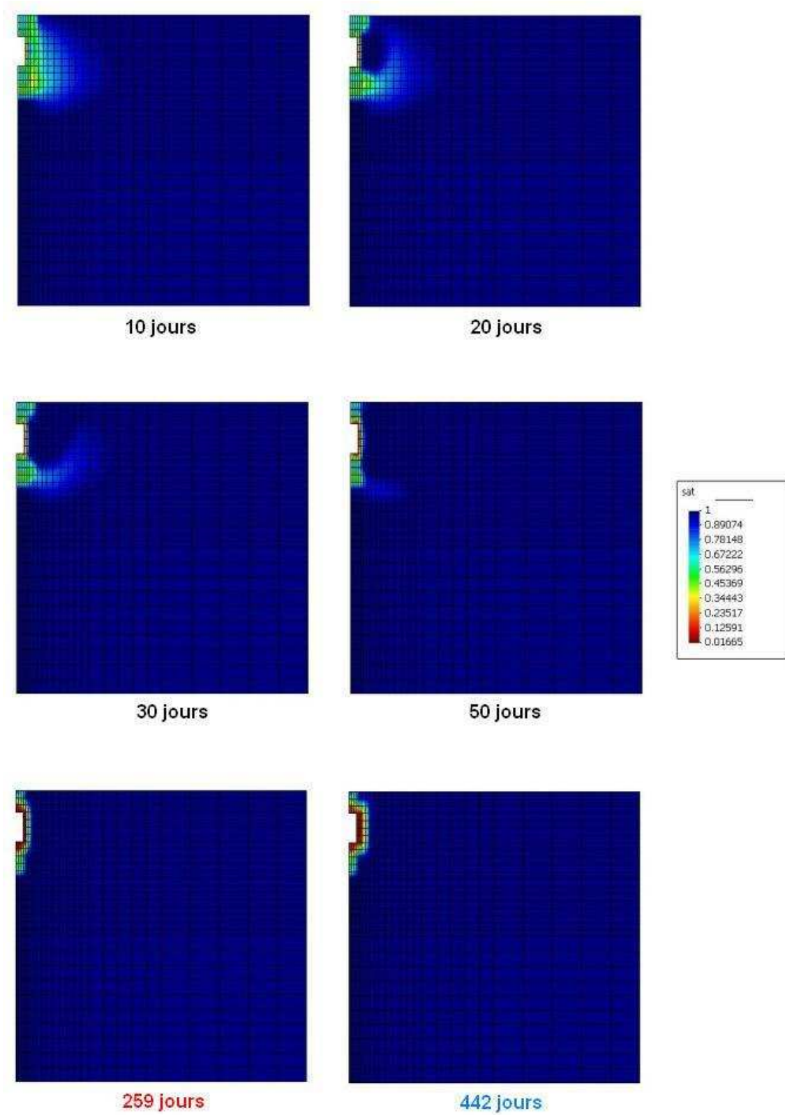
FIGURE 17.93 – Evolution spatio-temporelle du degré de saturation dans la simulation du test de Kamaishi. Cas n^{\circ} 3 (un plan de fissuration horizontal d’une étendue de 20 mètres).
