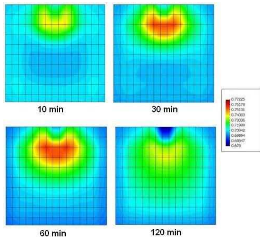
FIGURE 16.41 – Evolution spatio-temporelle de l'indice des vides pendant la simulation de l'essai de chauffage de Villar et al. [201], dans le domaine élastique du modèle THHMD.
