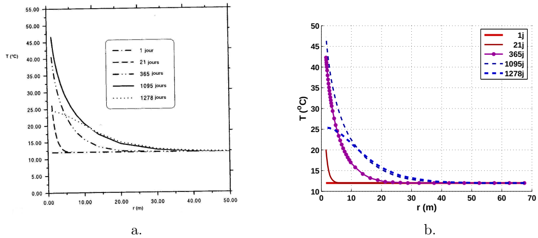
FIGURE 17.49 – Test in situ FEBEX. Evolution de la température dans la barrière géologique de granite. a. Résultats obtenus avec CODE BRIGHT par Gens et al. [79]. b. Résultats obtenus dans le domaine élastique du modèle THHMD avec \Theta -Stock.
