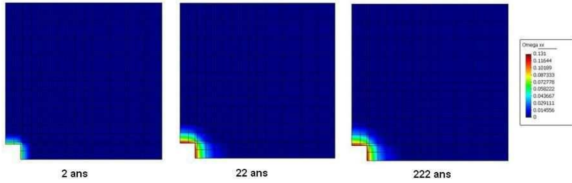
FIGURE 17.20 – Etude du comportement thermo-mécanique fragile d'un massif granitique en déformations planes. Evolution spatio-temporelle de la composante horizontale de l'endommagement ( \Omega_{xx} = \Omega_{yy} ) dans le problème de stockage des déchets radioactifs, avec g_T = 5 * g_M^{ref} .
