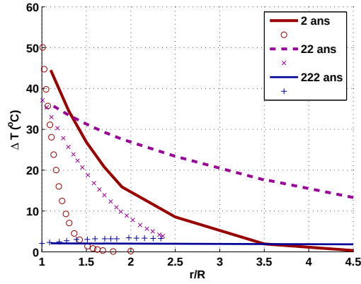
FIGURE 17.12 – Evolution de la température dans le massif à proximité du paquet radioactif. Etude axisymétrique pseudo-unidimensionnelle. Points : résultats obtenus par Carter et Booker [32]. Lignes continues : résultats numériques obtenus avec \Theta -Stock dans le domaine élastique du modèle THHMD.
