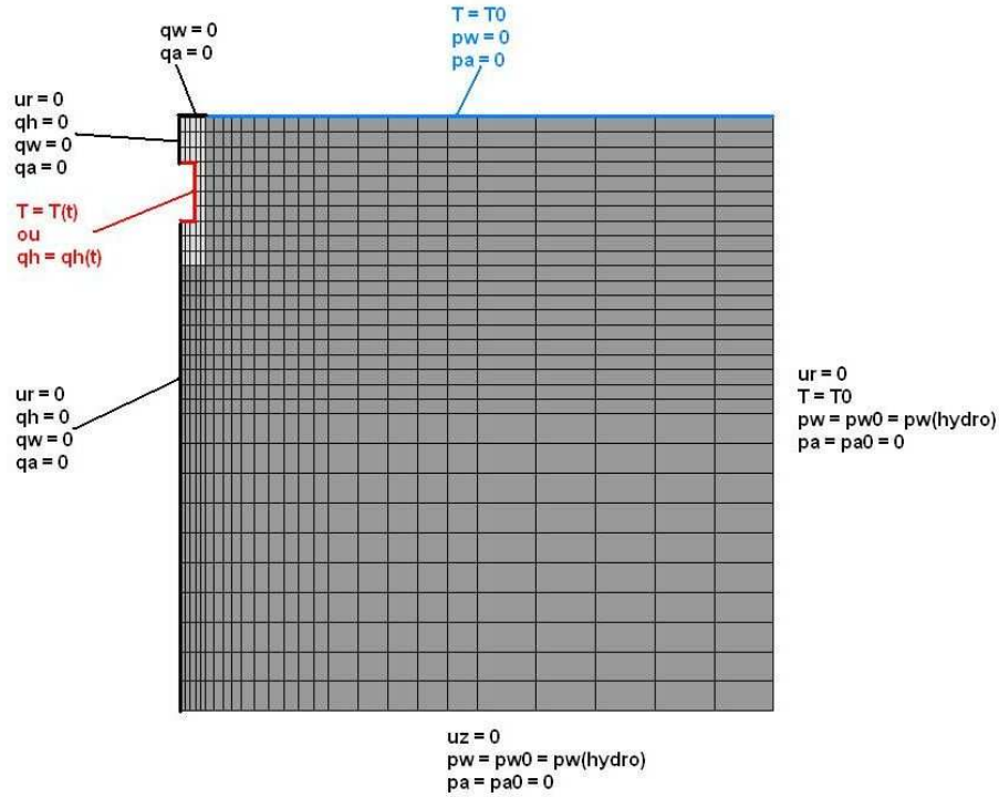
FIGURE 17.78 – Conditions aux limites adoptées dans la simulation de l’essai de chauffage réalisé à Kamaishi [173].
