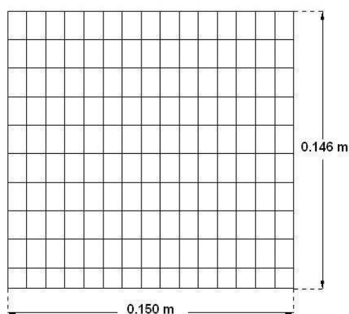
FIGURE 16.35 – Maillage adopté pour reproduire l'essai de Villar et al. [201]
