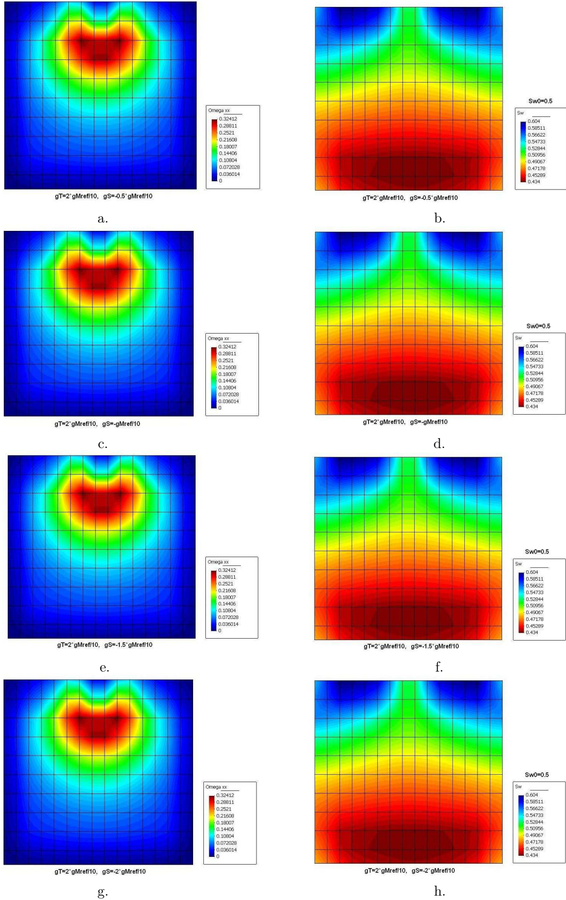
FIGURE 16.49 – Influence de g_S sur l'endommagement ( \Omega_{xx} = \Omega_{yy} ) et sur le degré de saturation, après 2h de chauffage. Fissuration thermo-capillaire ( g_T \neq 0 ).
