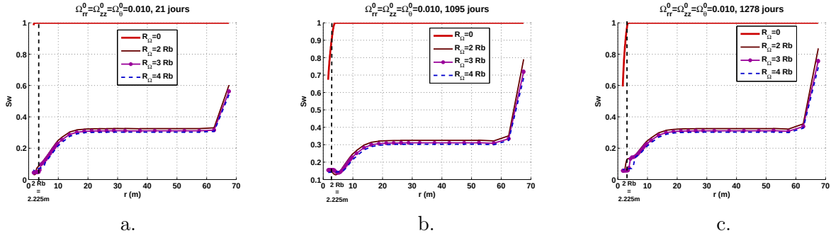
FIGURE 17.67 – Test in situ FEBEX. Influence de la présence d'un endommagement initial isotrope de 10 pour cent dans une zone d'étendue variable. Evolution du degré de saturation dans le massif granitique. a. Fin de l'accroissement de température (21 jours). b. Après le plateau de température (1095 jours). c. Après refroidissement (1278 jours).
