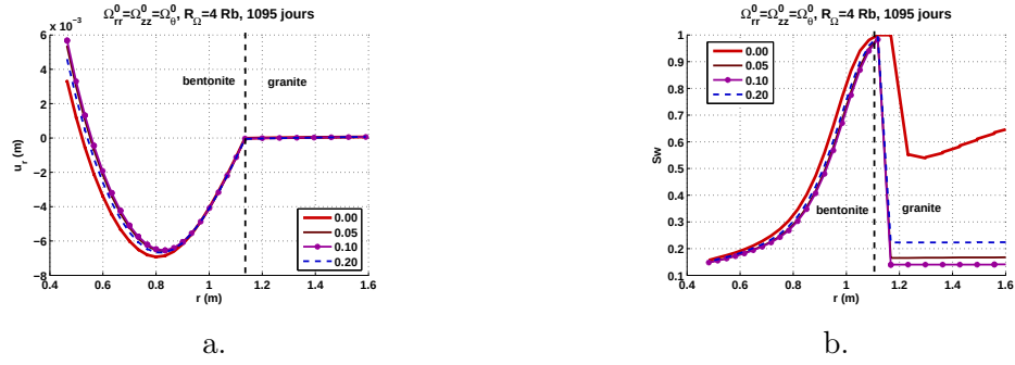
FIGURE 17.58 – Test in situ FEBEX. Influence de la présence d'endommagement initial isotrope dans la zone Rb \leq r \leq 4 Rb . Observations au voisinage de la frontière entre les barrières ouvragée (en bentonite) et géologique (en granite) après le plateau de température (1095 jours). a. Déplacement radial. b. Degré de saturation.
