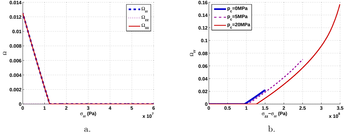
FIGURE 16.3 – Endommagement généré pendant les essais mécaniques simulés sur le granite de la Vienne. a. Essai d’extension latérale. b. Essai de compression triaxiale.
