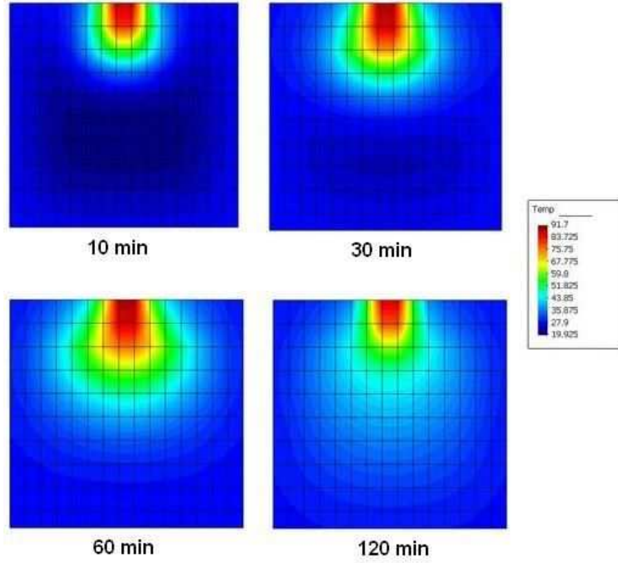
FIGURE 16.40 – Evolution spatio-temporelle de la température (en ^{\circ}\text{C} ) pendant la simulation de l'essai de chauffage de Villar et al. [201], dans le domaine élastique du modèle THHMD.
