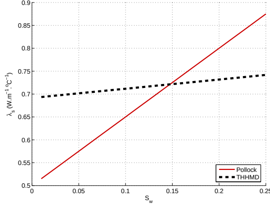
FIGURE 17.29 – Comparaison des conductivités thermiques du modèle de Pollock [163] et du modèle THHMD ( \lambda_s = 1.05 \text{ W.m}^{-1}.\text{°C}^{-1} ).
