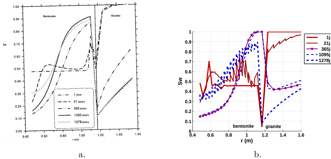
FIGURE 17.50 – Test in situ FEBEX. Evolution du degré de saturation dans la barrière ouvragée de bentonite. a. Résultats obtenus avec CODE BRIGHT par Gens et al. [79]. b. Résultats obtenus dans le domaine élastique du modèle THHMD avec \Theta -Stock.
