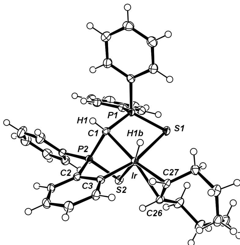
Figure 1: Molecular structure of II-27 . (ORTEP-plot, thermal ellipsoids, at a 50% probability level.) Selected bond distances ( \text{\AA} ) and angles ( ^\circ ): Ir(1)-S(1) 2.587(1); Ir(1)-S(2) 2.564(1); Ir(1)-C(3) 2.030(3); Ir(1)-C(1) 2.169(3); Ir(1)-H(1b) 1.46(4); Ir(1)-C(27) 2.209(4); Ir(1)-C(26) 2.210(3); S(1)-P(1) 1.996(1); S(2)-P(2) 2.002(1); P(1)-C(1) 1.785(3); P(1)-C(2) 1.794(4). P(1)-C(2)-C(3) 106.8(2); P(2)-C(1)-P(1) 124.7(2); P(1)-S(1)-Ir(1) 71.01(4); P(2)-S(2)-Ir(1) 78.62(4); C(1)-P(1)-S(1) 101.9(1); C(1)-P(2)-S(2) 106.8(1); C(3)-Ir(1)-C(1) 85.2(1); S(2)-Ir(1)-S(1) 86.34(3); S(2)-Ir(1)-H(1B) 87(2); S(1)-Ir(1)-H(1B) 163(2).
