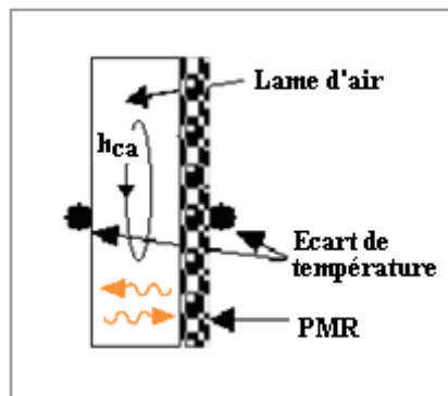
Figure 4.9 - Schéma du système modélisé (PMR couplé à une lame d'air)
