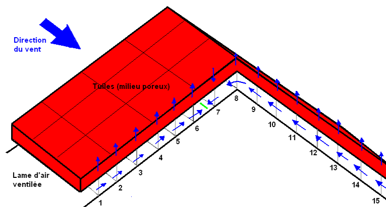
Figure 5.31 – Schéma représentant la direction du mouvement d'air dans le modèle (direction z)
