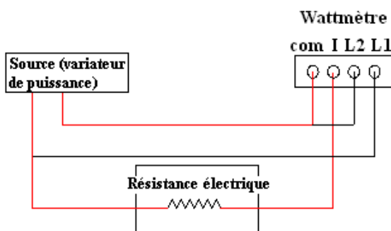
Figure 4.21 Installation électrique d'une cellule
