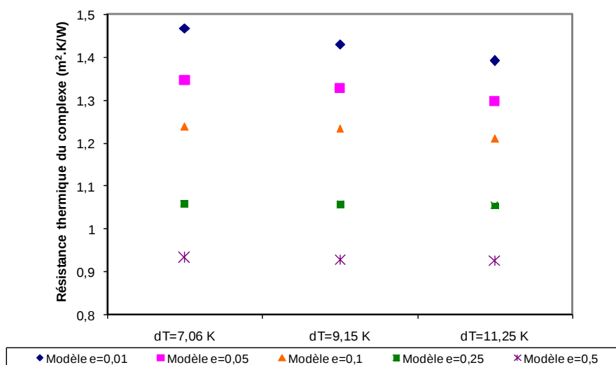
Figure 4.34 - Comparaison de la résistance thermique entre modèle et essais pour un complexe PMR et une lame d'air
