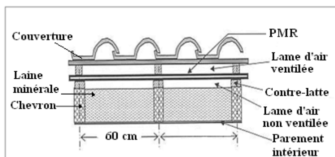
Figure 5.4 – Pose en écran de sous-toiture sur contre-latte (vue face aux chevrons)
