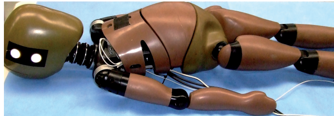
Figure 11 – LBMC – Mannequin de choc enfant Q3
