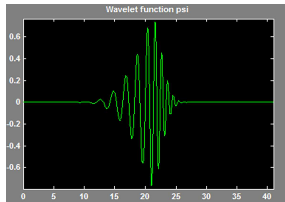
FIG. 8.7 – Ondelette de Daubechies d'ordre 19.
