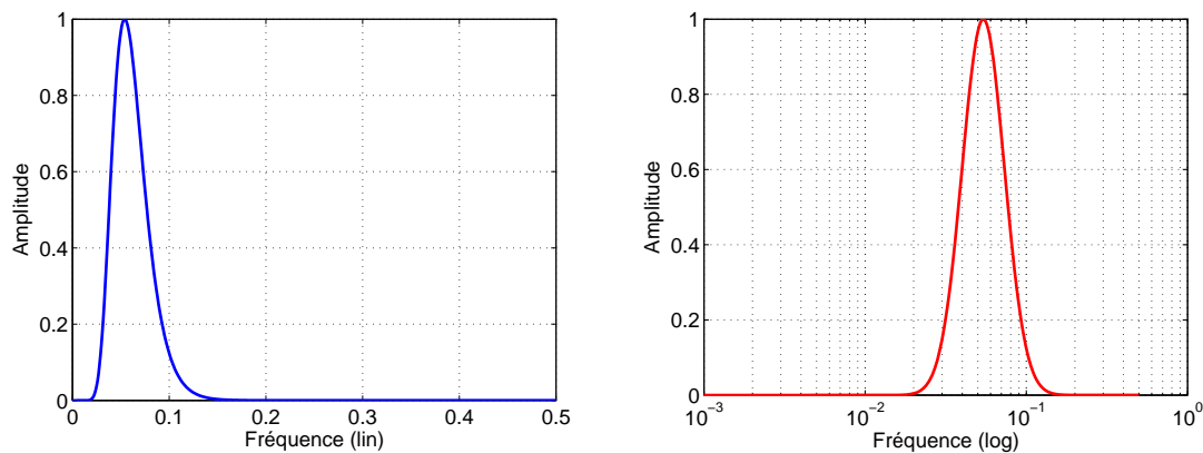
FIG. 3.12 – Fonction de transfert de Log-Gabor pour k = 0.04 (échelle fréquentielle linéaire à gauche, logarithmique à droite).
