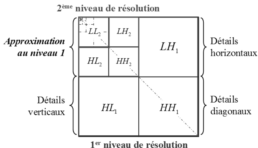
FIG. 6.10 – Analyse multirésolution.
