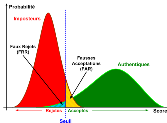
FIG. 7.1 – Illustration du FRR et du FAR.
