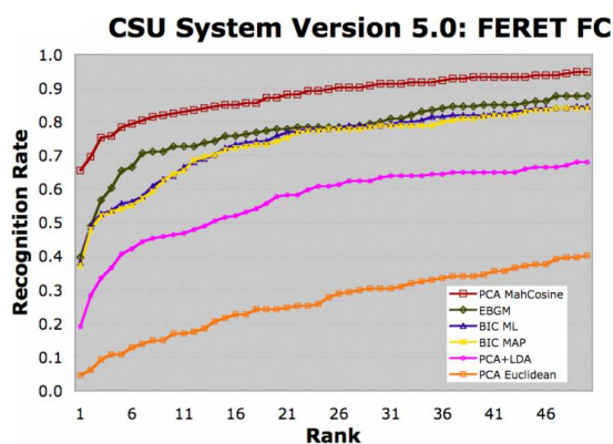
FIG. 1.8 – Courbes CMC du CSU System 5.0 pour le "FERET Probe Set FC" et pour différents algorithmes de reconnaissance faciale.
