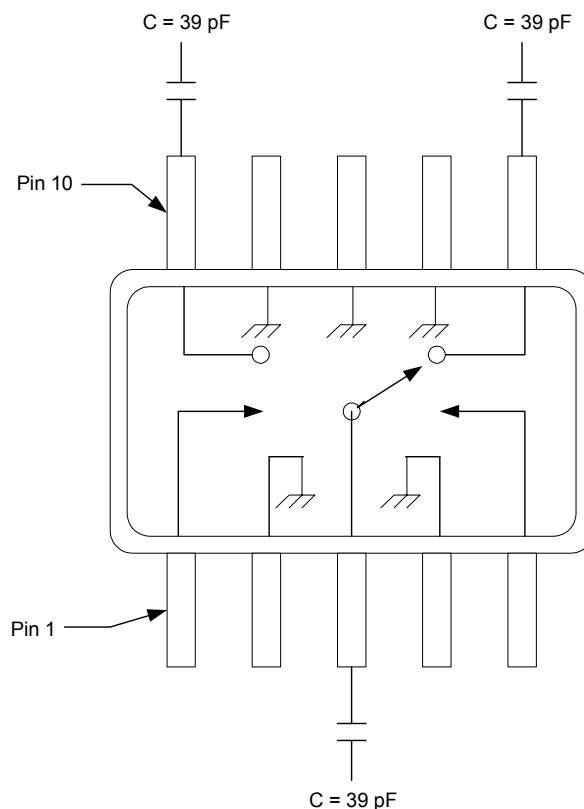
Fig. 2.15 : schéma fonctionnel de l'interrupteur SW439 de Tyco Electronics
