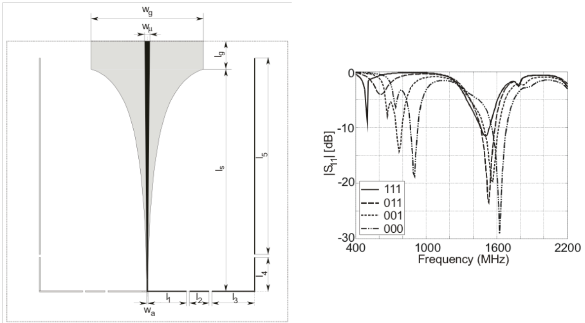
Fig. 1.6 : Une antenne quadri-bande reconfigurable
