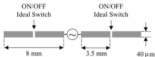
Fig. 1.5 : Un dipôle reconfigurable
