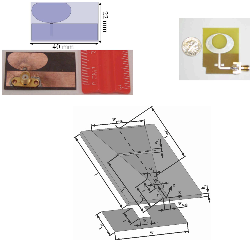
Fig. 2.5 : Exemple de monopoles UWB planaires
