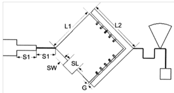
Fig. 1.7 : Antenne patch reconfigurable par MEMS
