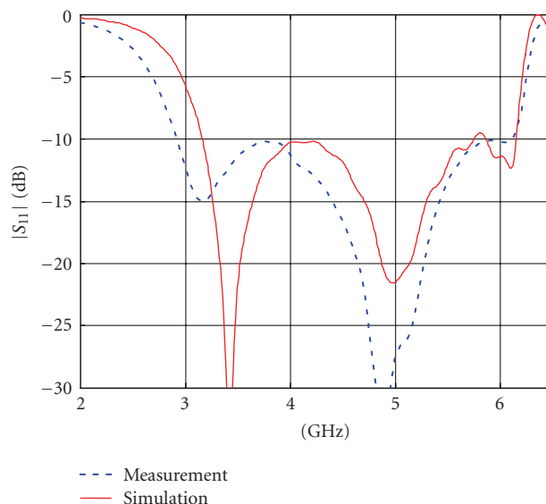
Fig. 4.2 : Courbe de S11 de l'antenne UWB de départ
