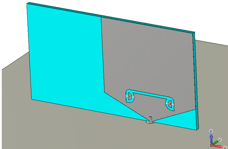
Fig. 4.17 : Vue en perspective de l'antenne proposée
