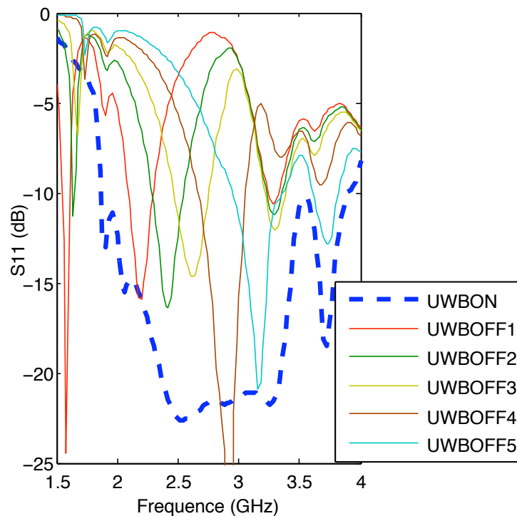
Fig. 4.30 : Courbe de S_{11} de l'antenne UWB reconfigurable proposée
