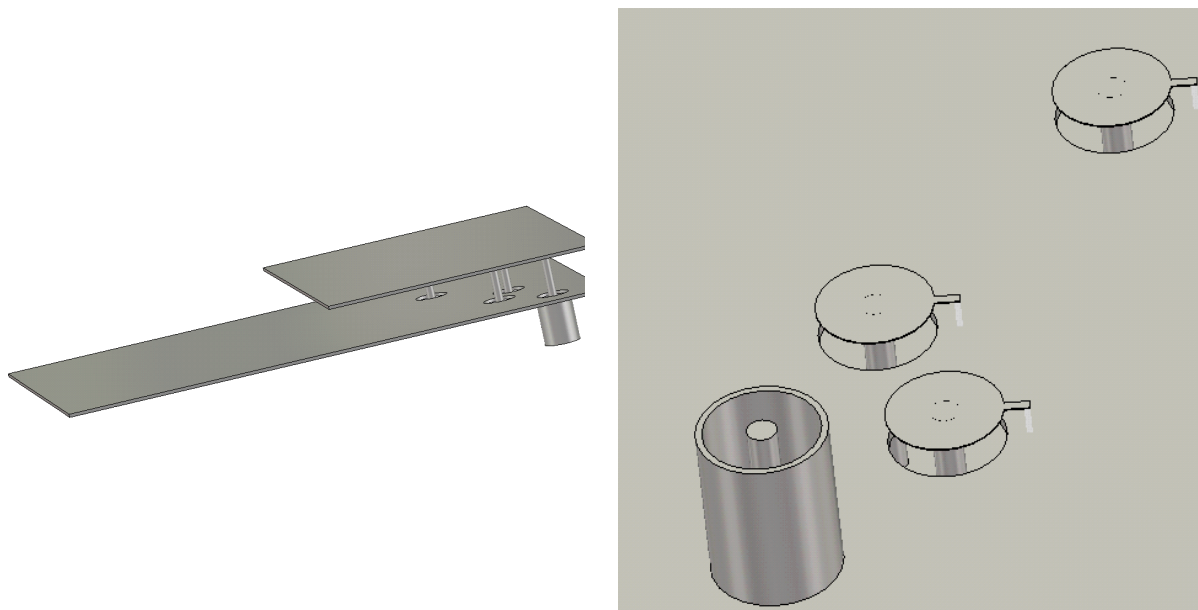
Fig. 3.27 : Géométrie de l'antenne PIFA comportant 3 diodes PIN et détail du positionnement des diodes
