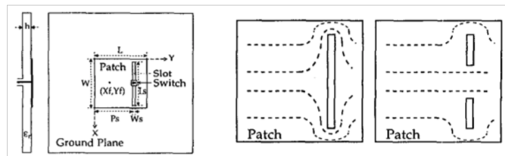
Fig. 1.11 : Fente commutable sur un patch rayonnant
