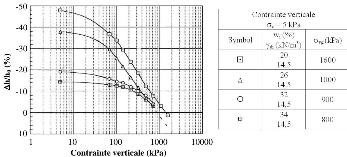
Figure 5.2.3 : Influence de la teneur en eau initiale sur la pression de gonflement mesurée par la méthode de gonflement libre ( \gamma_a moy = 14,5 kN.m -3 ) (Guiras-Skandaji, 1996)
