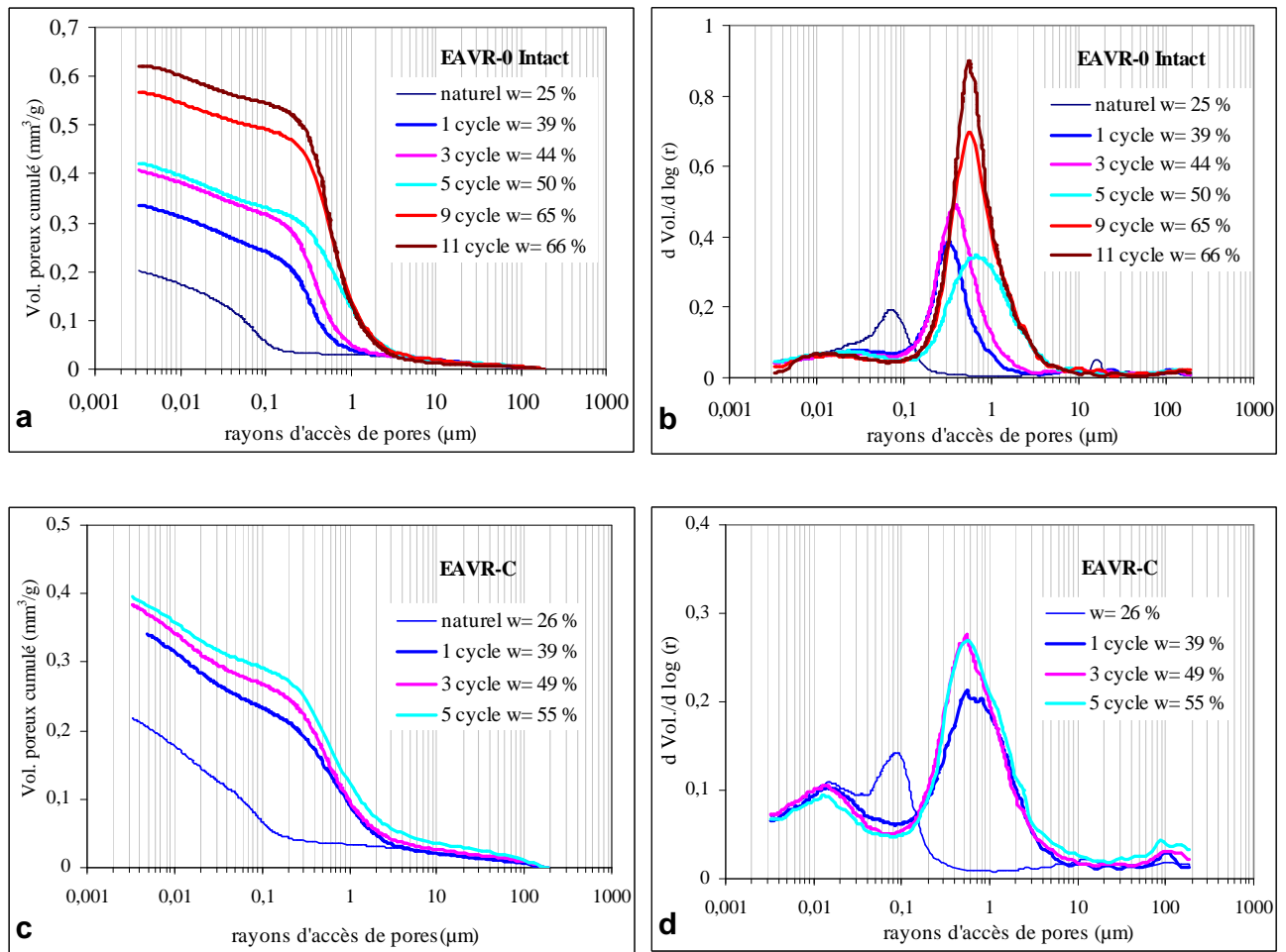
Figure 5.234 : Courbes cumulées (a) et dérivées (b) de distribution des rayons d'accès de pores de l'Argile verte de Romainville (EAVR-0) pour les cycles 1, 3, 5, 9 et 11. Courbes cumulées (c) et dérivées (d) de distribution des rayons d'accès de pores de l'Argile verte de Romainville (EAVR-C) pour les cycles 1, 3, 5
