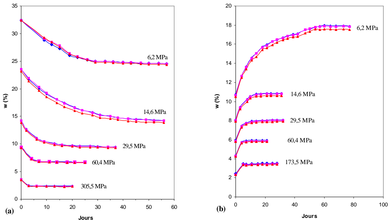
Figure 2.3.1 : Drainage (a) et humidification (b) par phase vapeur des échantillons d'Argile verte de l'Ouest
