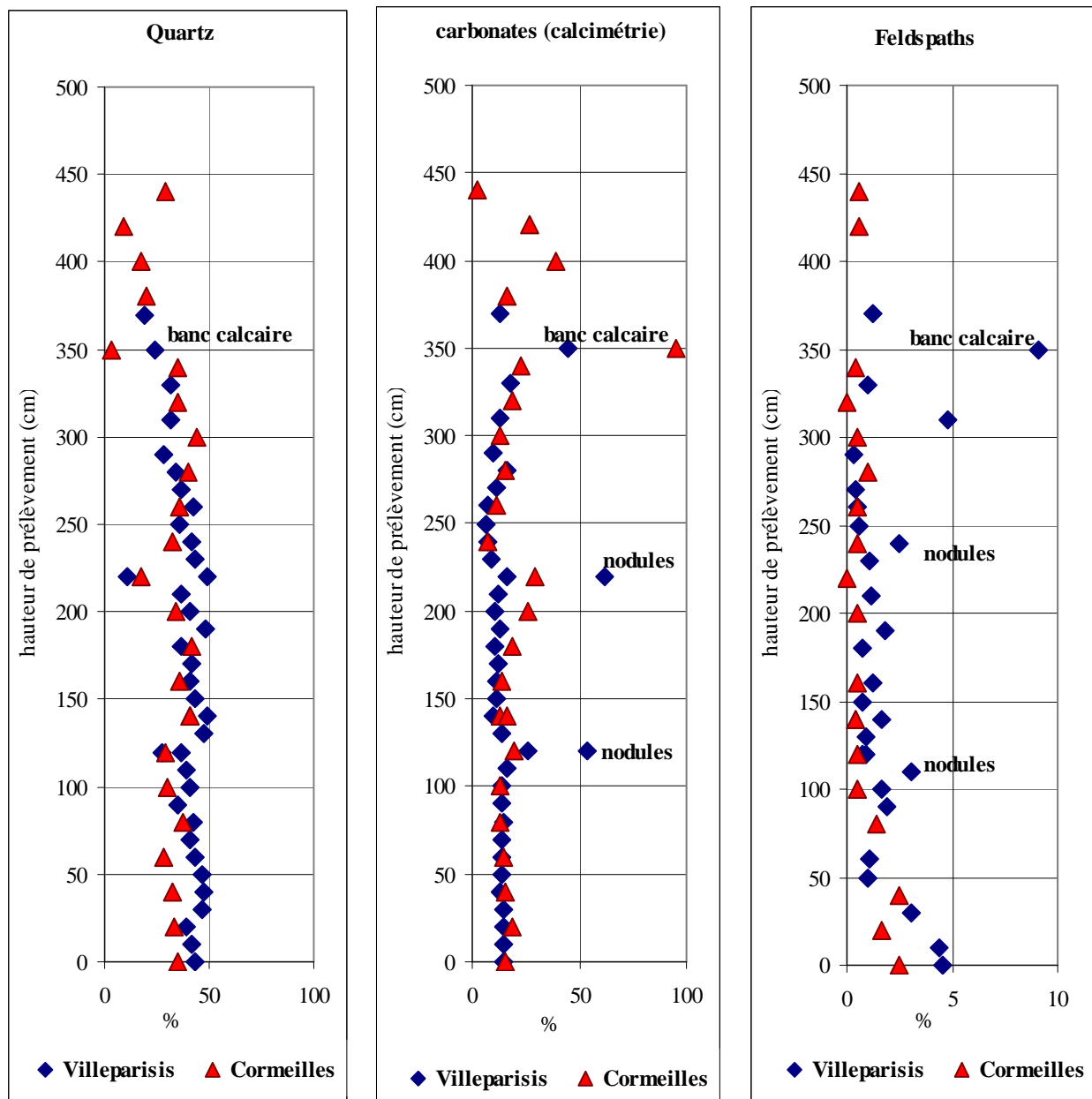
Figure 1.4.10 : Distribution du quartz (a) des carbonates dosés par calcimétrie (b) et des feldspaths (c) le long des profils de l'Argile verte de Romainville à l'Est (Villeparisis-Le Pin) et à l'Ouest (Cormeilles-en-Parisis)
