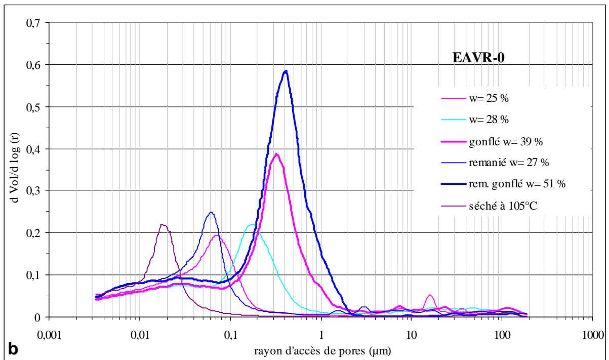
Figure 5.2.29 : Courbes cumulées (a) et dérivées (b) de distribution des rayons de pores de l'Argile verte de Romainville (EAVR-0) à l'état naturel, remanié, séché et après gonflement libre
