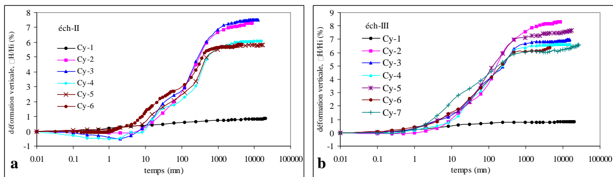
Figure 4.4.1 : Courbes de gonflement libre de la Marnes bleues d'Argenteuil (EMBA-1) au cours des cycles successifs imbibition-séchage complet a) échantillon Ech-II et b) échantillon Ech-III
