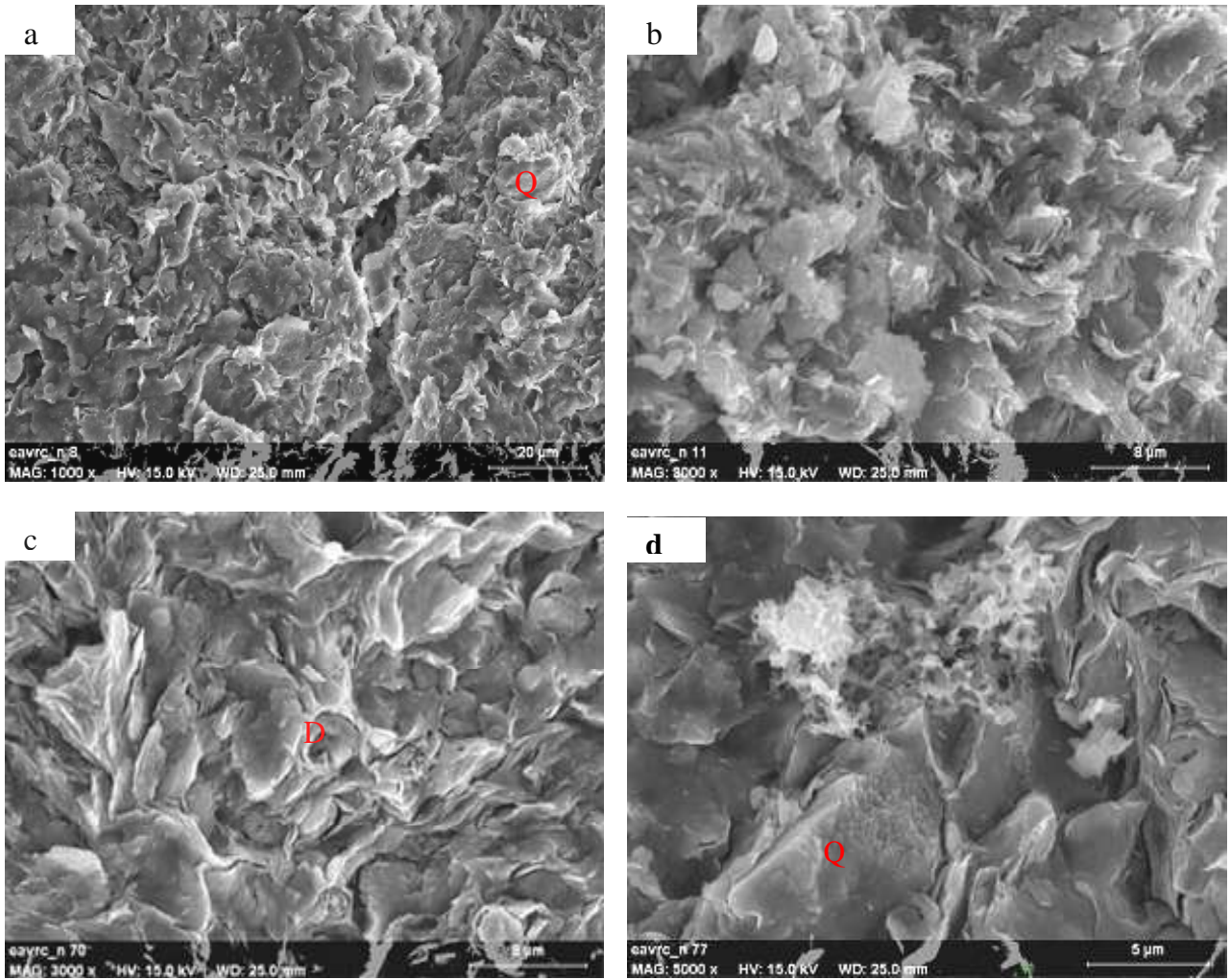
Figure 5.2.6 : Texture d'EAVR-C naturel (w= 24,9 %) dans le plan du litage : (a) vue globale, (b) texture à dominante argileuse, (c) présence des grains de dolomite, (d) présence de smectites et de grains de quartz
