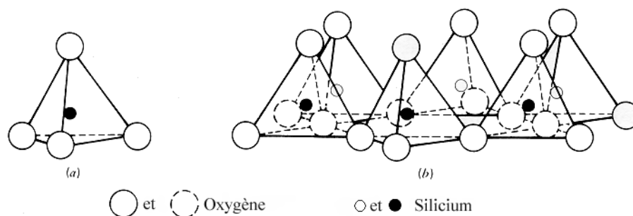
Figure 1.2.1 : Structure d'une couche tétraédrique : a) tétraèdre \text{SiO}_4 ; b) couche tétraédrique
