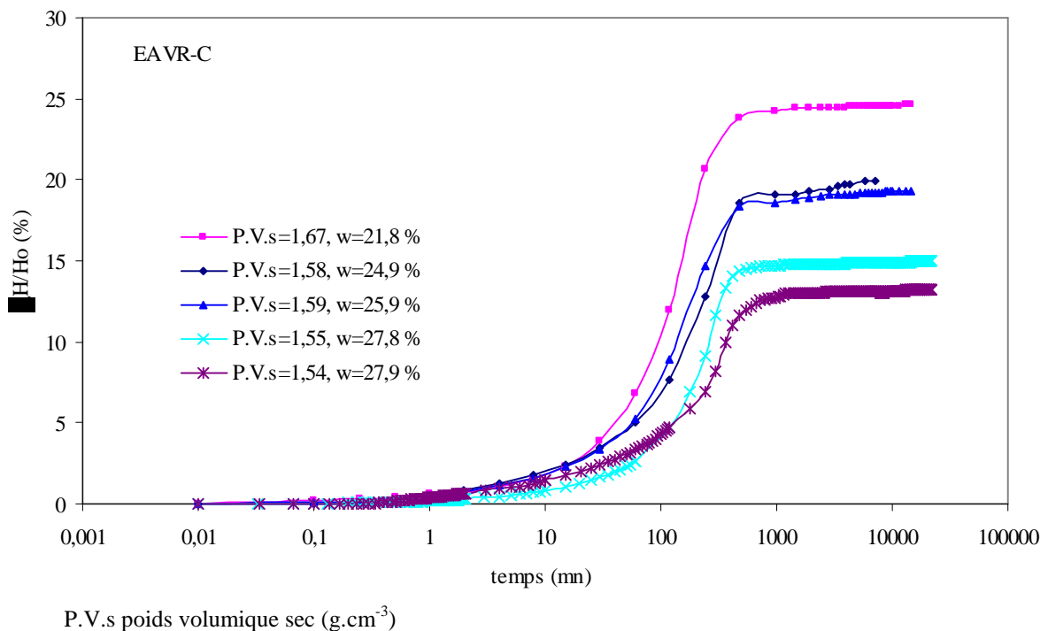
Figure 3.3.3 : Evolution des déformations verticales en fonction du temps (cinétique du gonflement) des échantillons EAVR-C testés à partir de leur état naturel, sous différentes charges verticales
