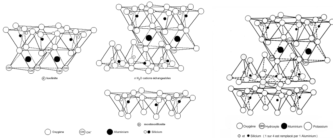
Figure 1.2.4 : Structures des feuillets de : a) kaolinite, b) smectite (montmorillonite) et c) illite (d'après Michell, 1993)
