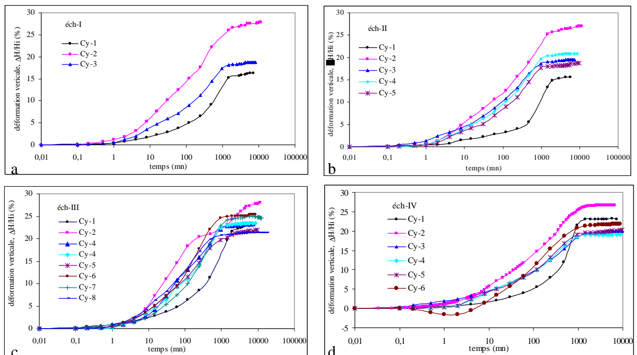
Figure 4.3.1 : Cinétique de gonflement de l'Argile verte de Romainville soumise alternativement à des phases d'imbibition totale et des phases de séchage complet a) Ech-I, b) Ech-II, c) Ech-III, d) Ech-IV
