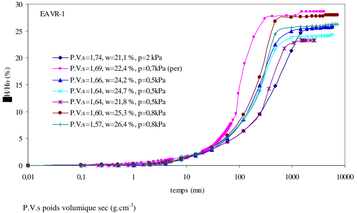
Figure 3.3.2 : Evolution des déformations verticales en fonction du temps (cinétique du gonflement) des échantillons EAVR-1 testés à partir de leur état naturel, sous différentes charges verticales
