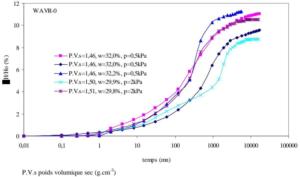
Figure 3.3.6 : Evolution des déformations verticales en fonction du temps (cinétique du gonflement) des échantillons WAVR-0 testés à partir de leur état naturel, sous différentes charges verticales
