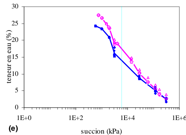
Figure 2.3.5 : Comportement global des Argiles vertes de Romainville de l'Est au cours d'un cycle de drainage-humidification, ( w_{Re} = limite de retrait effective, S_{wRe} = succion à la limite de retrait effective)
