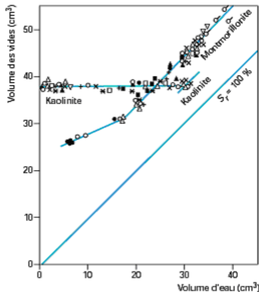
Figure 4.5.2 : Relation entre le volume des vides et le volume d'eau contenue dans deux argiles (d'après Delage et Cui, 2000)
