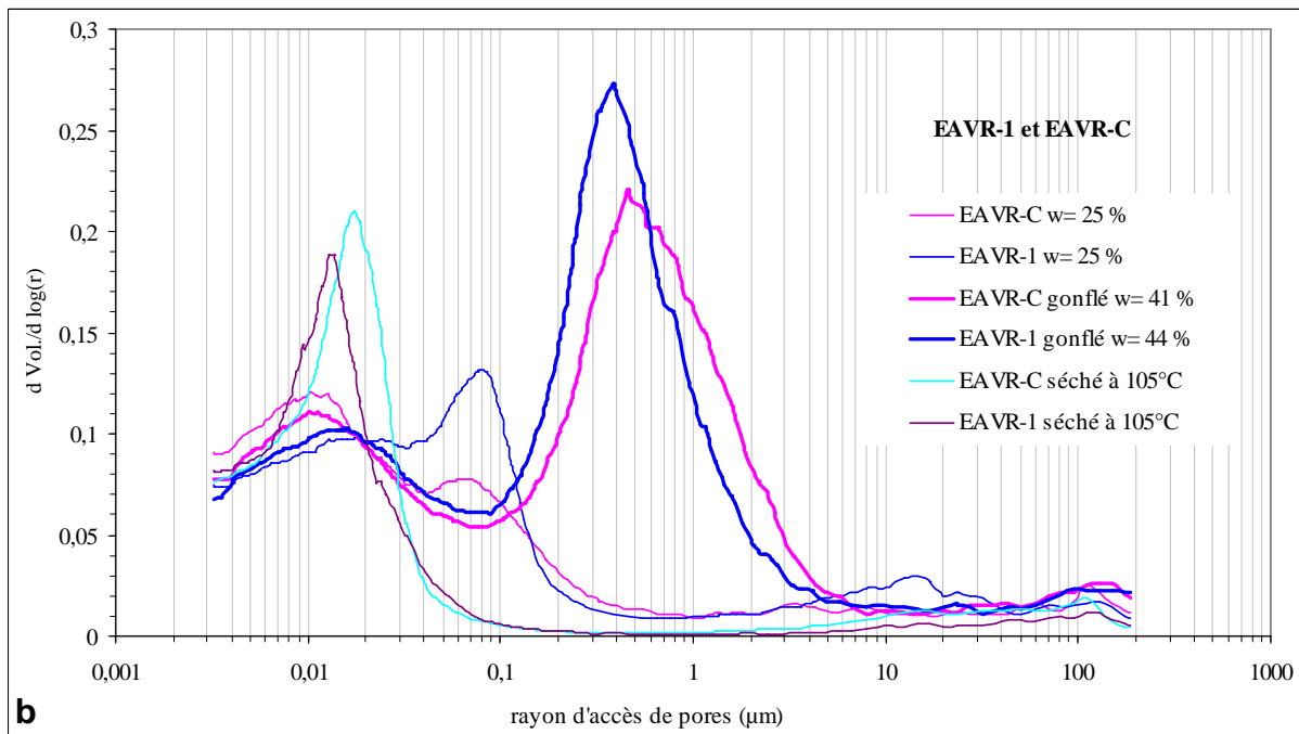
Figure 5.2.30 : Courbes cumulées (a) et dérivées (b) de distribution des rayons de pores de l'Argile verte de Romainville (EAVR-1 et EAVR-C) à l'état naturel, séché et après gonflement libre
