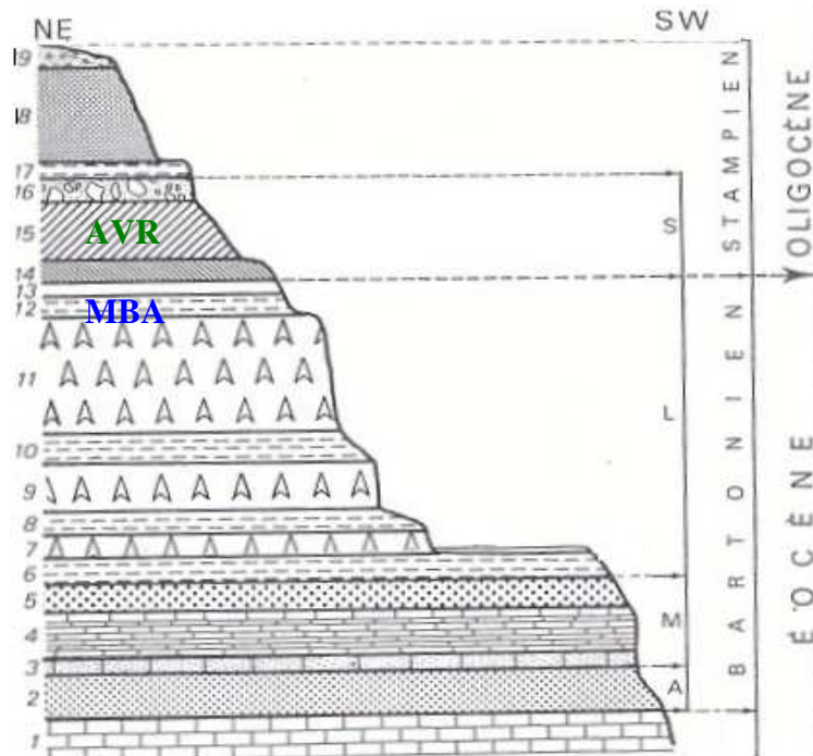
1) Calcaire Grossier, 2) Sables de Beauchamp, 3) Calcaire du Ducy et grès de Mortefontaine, 4) Calcaire de Saint-Ouen, 5) Sables de Monceau, 6) Marnes à Pholadomya ludensis , 7) Gypse, 3 e masse, 8) Marnes à Lucines, 9) Gypse pied-d'alouette (2 e masse), 10) Marnes d'Entre-deux-Masses, 11) Gypse saccharoïde (Haute-masse), 12) Marnes bleues d'Argenteuil, 13) Marnes blanches de Pantin, 14) Glaises brunes à Cyrènes, 15) Argiles vertes de Romainville, 16) Caillasses d'Orgemont et calcaire de Sannois, 17) Marnes à huîtres, 18) Sables de Fontainebleau, 19) Argiles à meulières de Montmorency et limon lœssique. A : Auversien, M : Marinésien, L : Ludien, S : Sannoisien
