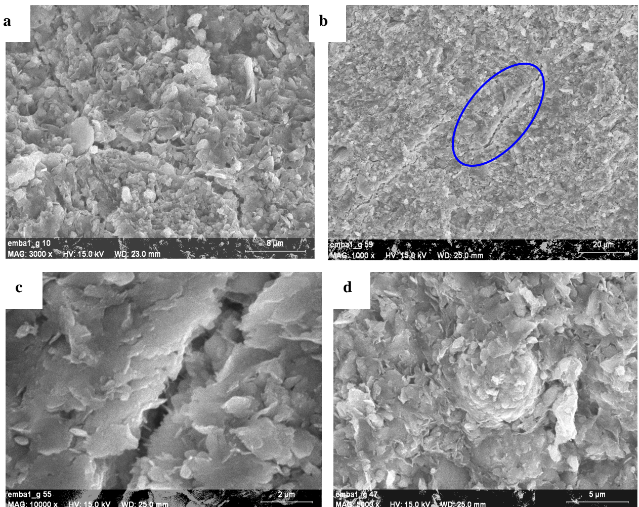
Figure 5.2.23 : Texture d'un échantillon d'EMBA-1 naturel après un cycle de gonflement: a) vue globale parallèle au plan du litage, b) vue globale perpendiculaire au plan du litage c) détail de microfissure observée sur l'image b, d) présence de pyrite framboïdale non altérée
