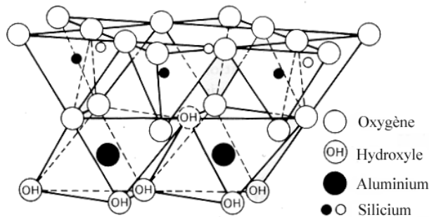
Figure 1.2.3 : Association d'une couche tétraédrique et d'une couche octaédrique
