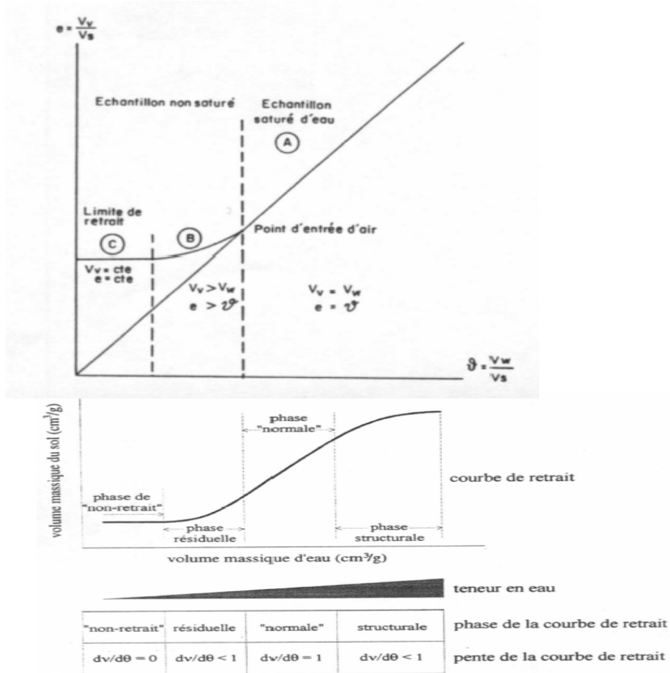
Figure 4.5.1 : Représentation schématique de la courbe de retrait d'une argile (d'après Tessier, 1984 ; Coquet, 1995 d'après Tessier et al, 2006)
