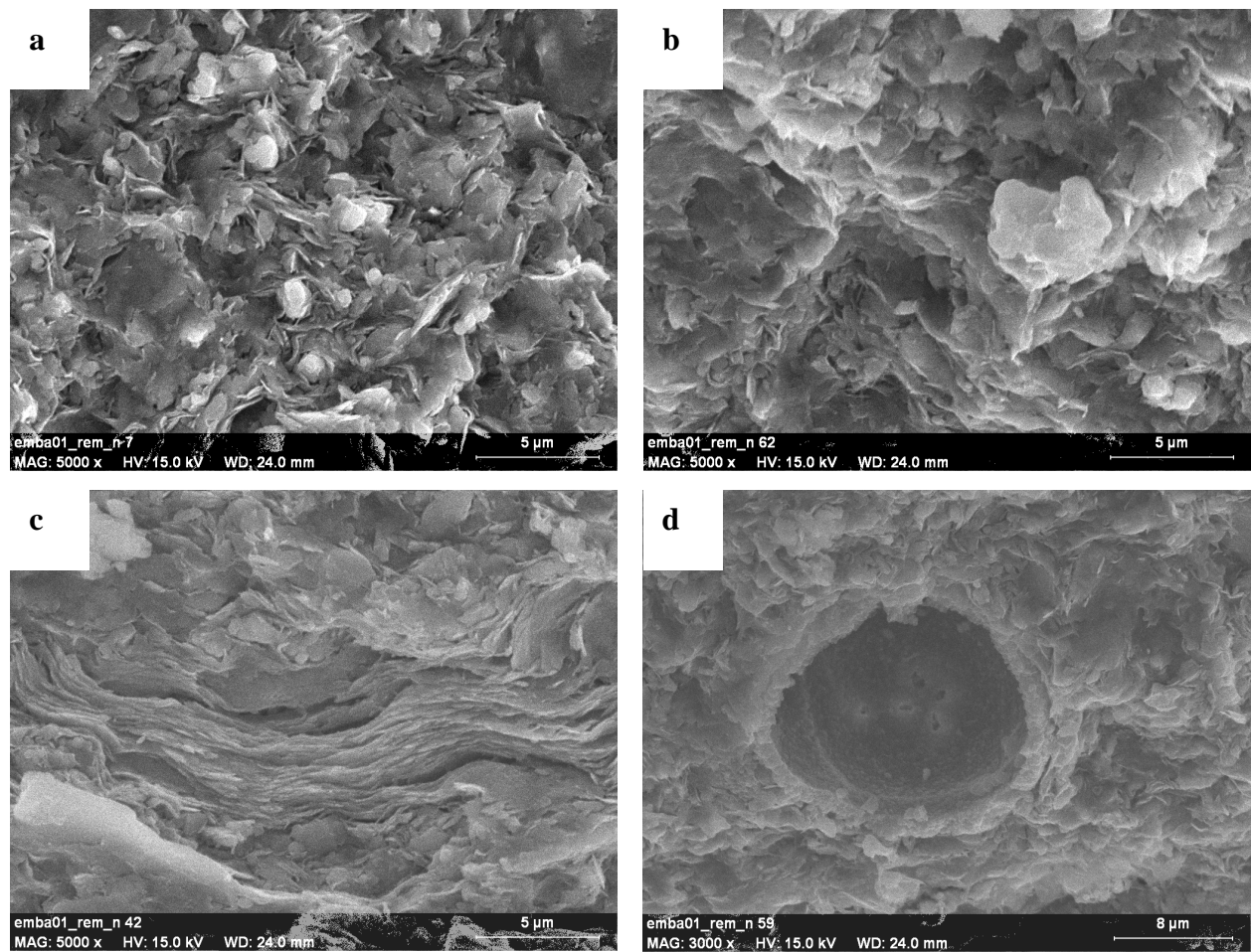
Figure 5.2.21 : Texture d'un échantillon d'EMBA-01 remanié avant essai de gonflement: a) vue globale dans le plan du dépôt, b) vue globale perpendiculaire au plan du dépôt c) amas d'argile d) fragments de tests d'animaux
