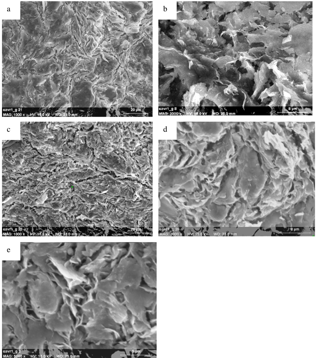
Figure 5.2.10 : Texture d'un Echantillon d'EAVR-1 après un cycle de gonflement libre : a) et b) dans le plan du litage ; c) d) et e) perpendiculaire au plan du litage
