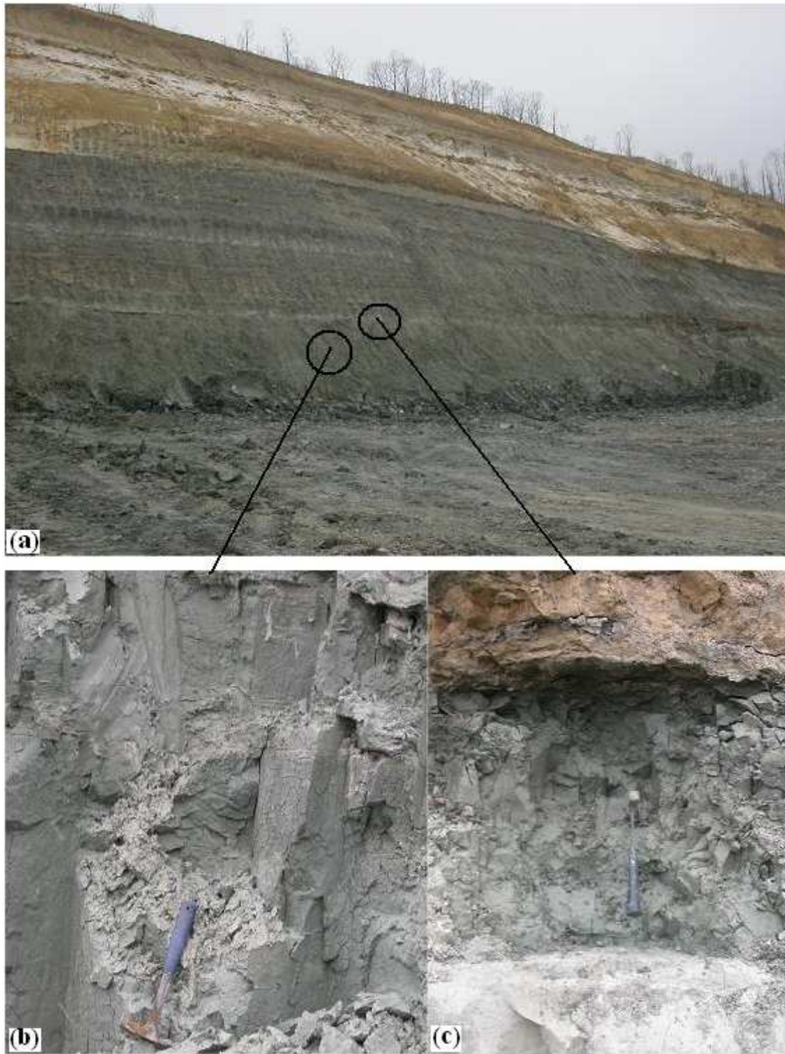
Figure 1.2.4 : (a) Front de taille de l'Argile verte de Romainville dans la carrière de Cormeilles-en-Parisis (avril 2008) ; (b) Partie inférieure du banc d'Argile verte de Romainville ; (c) partie supérieure du banc d'Argile verte de Romainville, avec à la base présence d'un banc calcaire décimétrique (partie blanche) et au sommet le contact avec le banc des caillasses d'Orgemont
