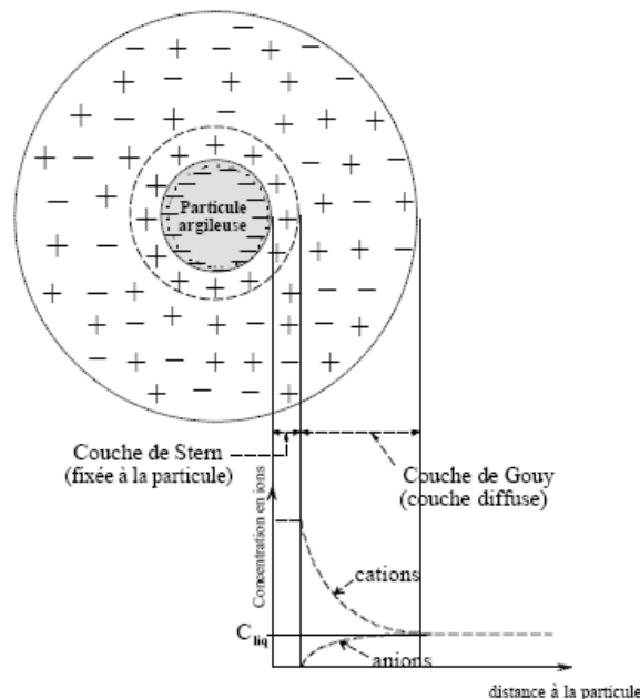
Figure 4.1.2 : Schéma de la double couche (d'après Bultel, 2001)
