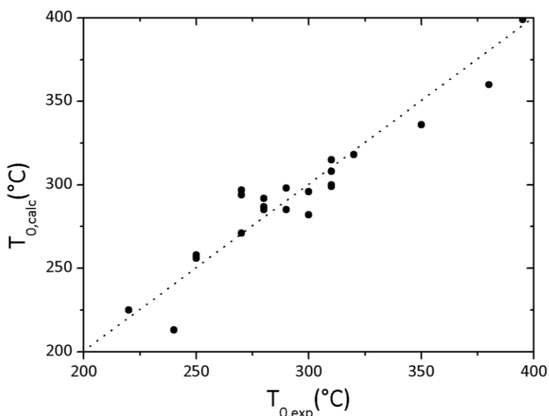
Figure 43 – Températures de décomposition (en °C) expérimentales et prédites par le modèle AM1 (Eq. 3.25)
