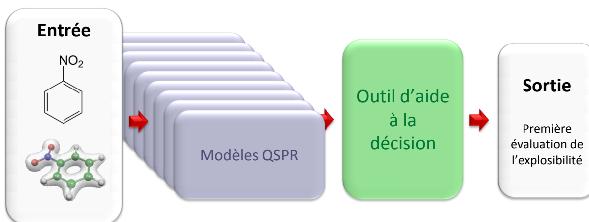
Figure 10 - Outil de prédiction des propriétés d'explosibilité
