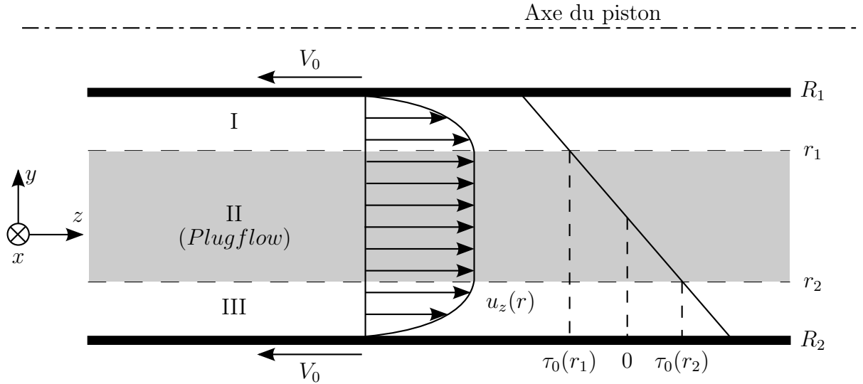
Figure 3.13 - Ecoulement plug flow d'après [Yang 02]. Dans la zone II, la contrainte de cisaillement n'est pas suffisante pour rompre les chaînes de particules, par conséquent dans cette zone le fluide se déplace en bloc.
