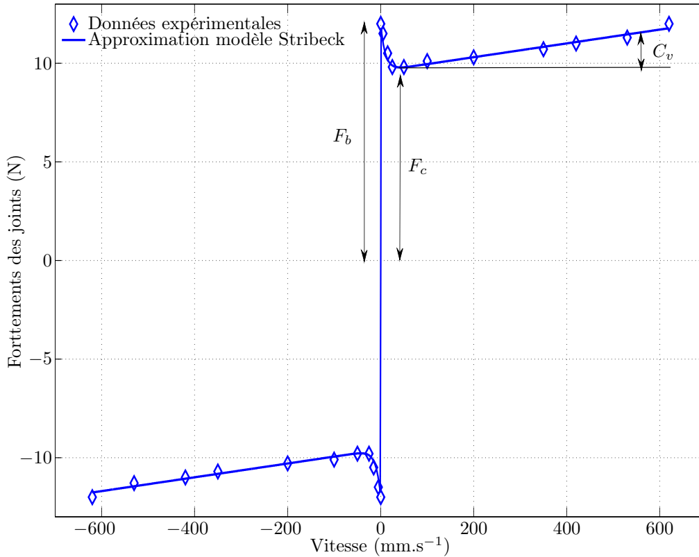
Figure 3.7 - Approximation de la force de frottements des joints quadrilobes par un modèle de Stribeck.
