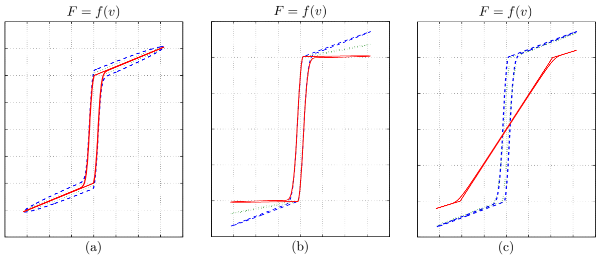
Figure 3.28 - (a) les paramètres k_0 ou k_1 agissent sur le seuil d'effort au-delà duquel l'amortisseur change de comportement; (b) le paramètre c_0 paramètre agit exclusivement sur la pente de l'effort à haute vitesse; (c) c_1 agit sur la première pente, pour les faibles vitesses.
