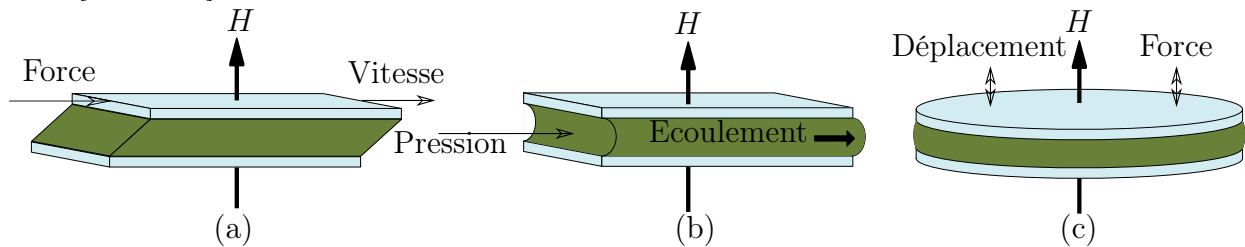
Figure 1.20 - Les modes d'utilisation des liquides MR : le mode cisaillement (a), le mode valve (b) et le mode compression (c).
