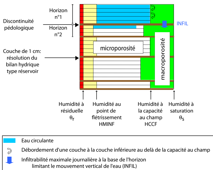
FIGURE 3.3 – Partition du sol et modélisation des transferts hydriques selon un modèle réservoir, d'après Brisson et al. [2008]
