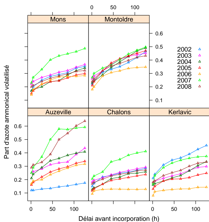
FIGURE 4.6 – Effet du délai d'enfouissement du lisier sur les émissions de NH_3 Dans toutes ces simulations, 80% du lisier est enfoui à 5 cm de profondeur
