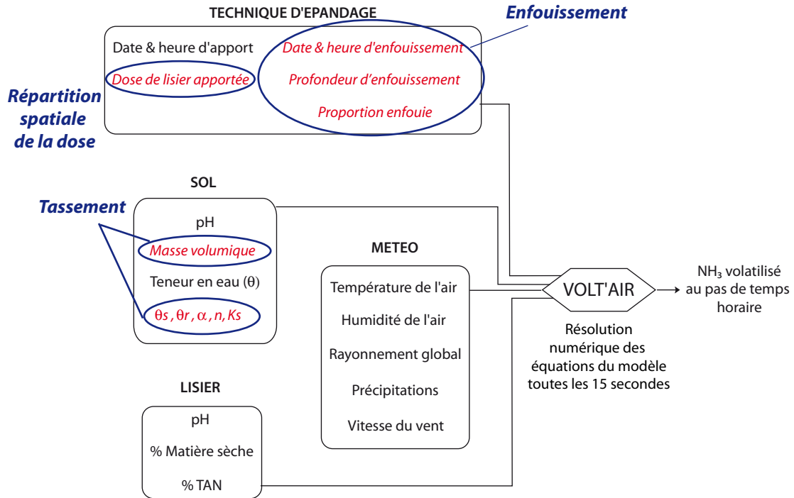
FIGURE 3.2 – Principaux paramètres d'entrée du modèle Volt'air
