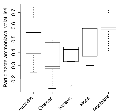
FIGURE 4.3 – Emissions de \text{NH}_3 simulées sur les 5 sites de 2002 à 2008 pour un épandage en plein homogène
