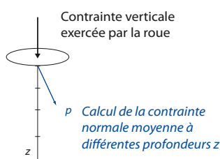
FIGURE 3.5 – Propagation de la contrainte verticale dans le sol
