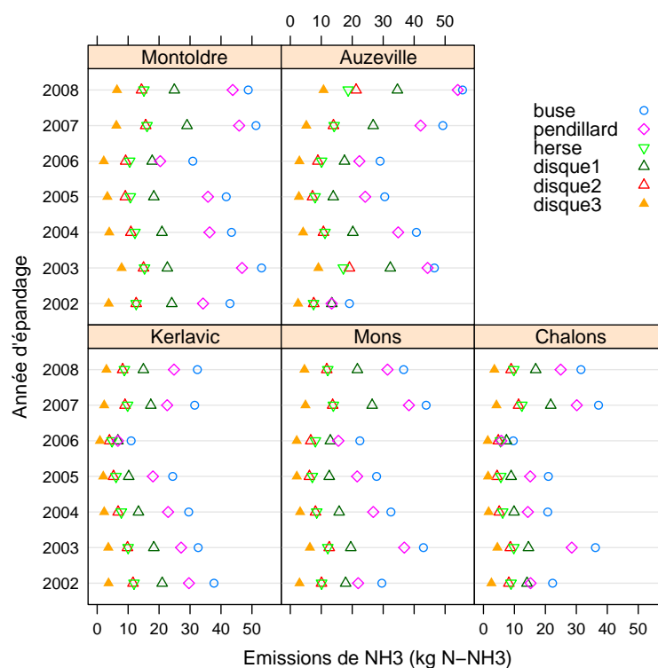
FIGURE 4.12 – Hiérarchie des épandeurs selon les émissions de \text{NH}_3 sur les cinq sites
