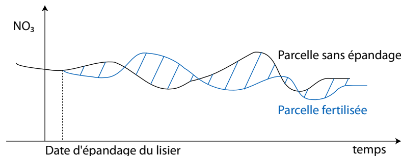
FIGURE 5.2 – Dynamique d'émission de \text{NO}_3^- pour une parcelle avec épandage de lisier et pour une parcelle sans épandage
