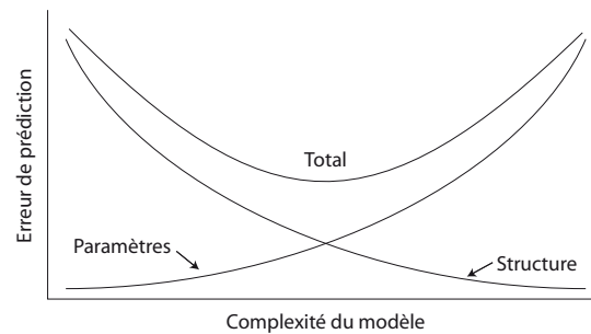
FIGURE 5.3 – Erreur prédictive des modèles selon leur niveau de complexité (d'après Passioura [1996])
