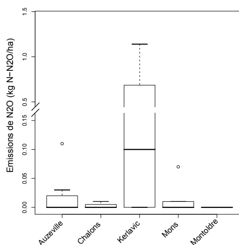
FIGURE 4.4 – Emissions de \text{N}_2\text{O} simulées sur les 5 sites de 2002 à 2008
