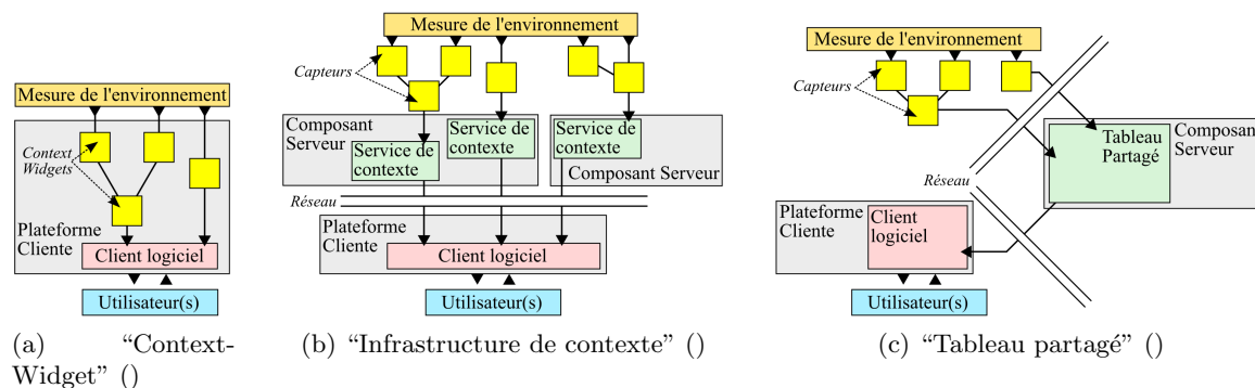
Figure II.6 – Architectures pour la perception du contexte à l'exécution
