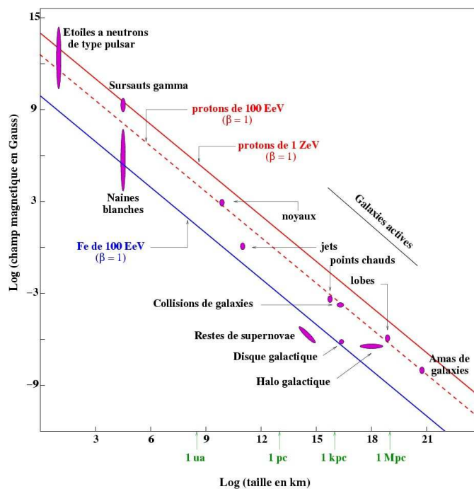
FIGURE 1.4 Diagramme de Hillas. La ligne pleine rouge représente la relation R-B pour un proton accéléré à 1 \text{ ZeV} = 1 \times 10^{21} \text{ eV} . La droite bleue est obtenue pour un atome de fer à 100 EeV, la ligne pointillée rouge pour un proton à la même énergie. Chaque type de source est repéré dans ce diagramme par une ellipse violette donnant les valeurs de B et R typiques de ces sources. Plus une source se situe vers le haut et la droite de cette figure, plus l'énergie maximale atteinte peut être grande.
