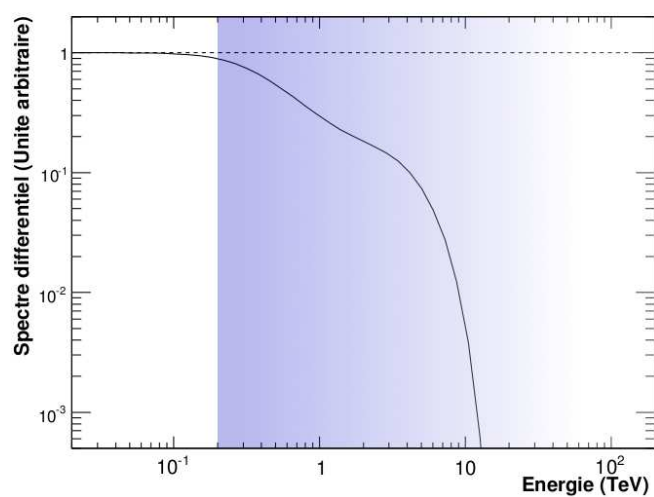
FIGURE C.3 Flux d'une source fictive à z=0.117 . En trait plein, le flux corrigé pour l'absorption due à l'EBL, en traits pointillés, le flux intrinsèque. La zone bleue présente la zone de sensibilité des expériences Tcherenkov.
