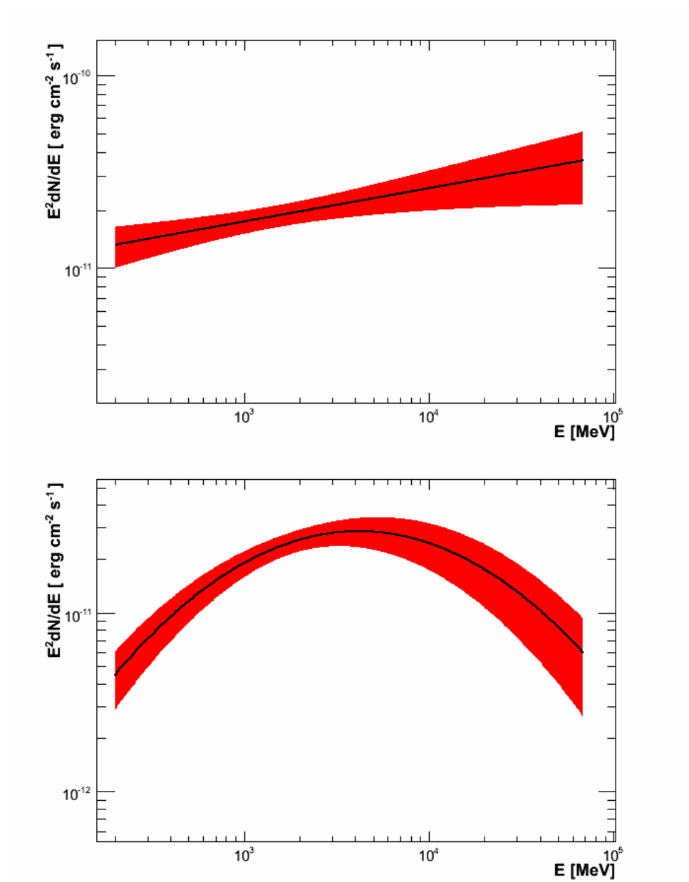
FIGURE B.1 Contour d'erreur pour une loi de puissance (en haut) et pour une log-parabole (en bas).
