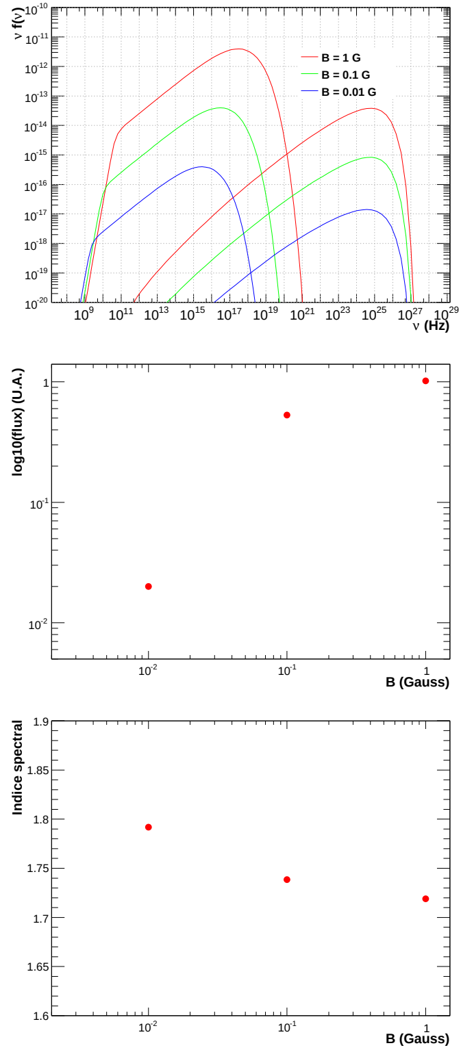
FIGURE 4.9 Effets de la variation des différents paramètres du modèle SSC. Pour chaque paramètre, les SED calculées sont présentées (en haut) ainsi que le flux normalisé entre 200 MeV et 10 GeV, soit entre 4.8 \times 10^{22} et 2.4 \times 10^{24} Hz, (au milieu) et l'indice spectral correspondant (en bas). Panel A
