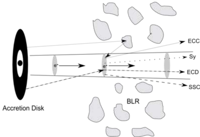
FIGURE 1.20 Schéma d'un jet. Les électrons sont accélérés proche du trou noir central. Ils émettent des photons par rayonnement synchrotron ou par interaction avec des photons cibles de différentes origines (disque, BLR ou même photons synchrotron).
