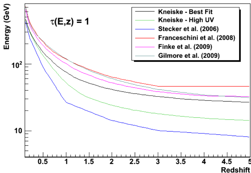
FIGURE 3.4 Énergie pour laquelle \tau = 1 en fonction du redshift z suivant les modèles de (Franceschini et al., 2008; Primack et al., 2005; Kneiske et al., 2004; Stecker et al., 2006; Finke et al., 2010; Gilmore et al., 2009).
