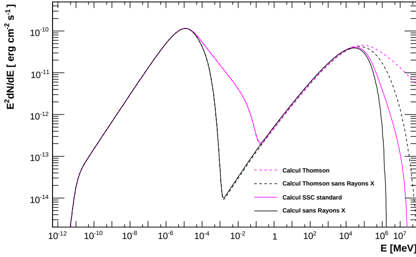
FIGURE 4.20 Résultats des différents calculs SSC. En magenta, le calcul avec les paramètres du modèle de base “ Swift -XRT magenta”. La ligne magenta pointillée donne le flux obtenu avec les mêmes paramètres mais dans l’approximation Thomson. La ligne noire est obtenue lorsque les électrons de plus haute énergie ( \gamma > \gamma_2 ) sont omis du calcul.
