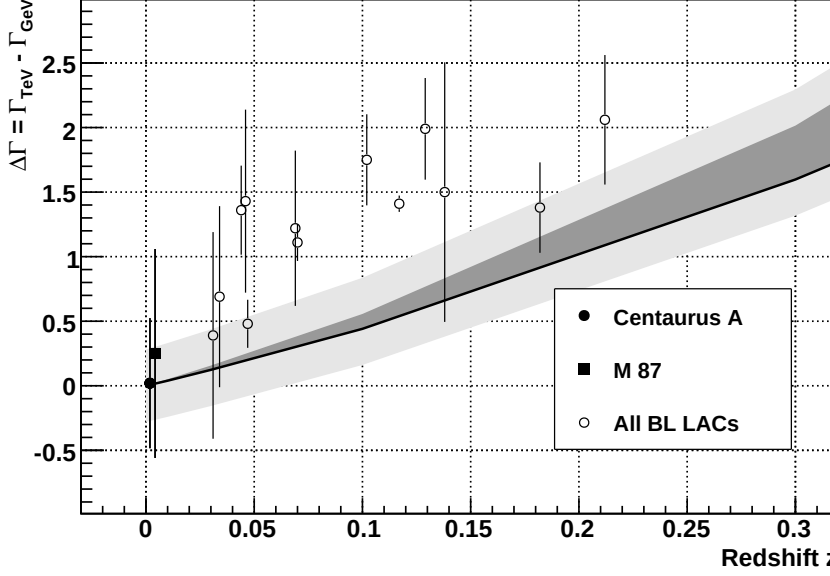
FIGURE 3.9 La différence \Delta\Gamma entre le spectre mesuré aux THE et celui mesuré aux HE en fonction de z . Les cercles vides sont les BL Lac, le cercle plein est Centaurus A et le carré noir M 87. Le spectre de Cen A a été obtenu sans prendre en compte l'extention de la source. Il apparaît une corrélation \rho = 0.76 \pm 0.16 . La ligne noire est la prédiction minimale des effets de l'EBL. La zone en gris sombre présente l'incertitude liée au calcul de cet effet. La zone gris clair est une représentation de l'erreur statistique ajoutée.
