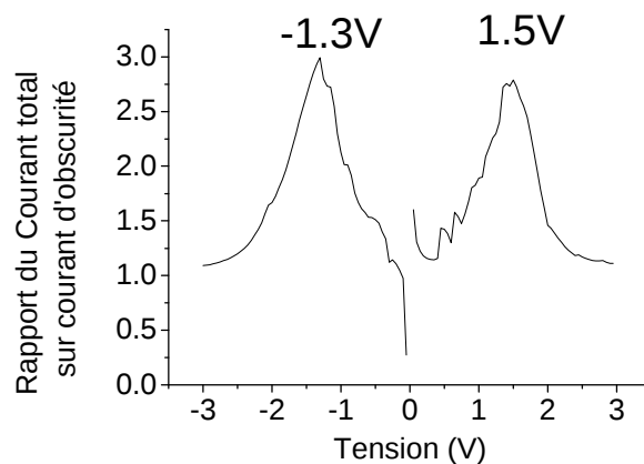
FIG. 2-18 Evolution du rapport entre le courant total et le courant d'obscurité en fonction de la tension. Ce graphe est utile à la détermination du point de fonctionnement en tension du détecteur.
