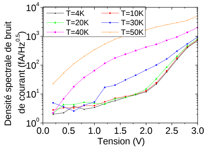
FIG. 2-10 Densité spectrale de bruit au niveau du plateau de courant tunnel, en fonction de la tension de polarisation pour différentes températures - pixel 100 \times 100 \mu m^2 .
