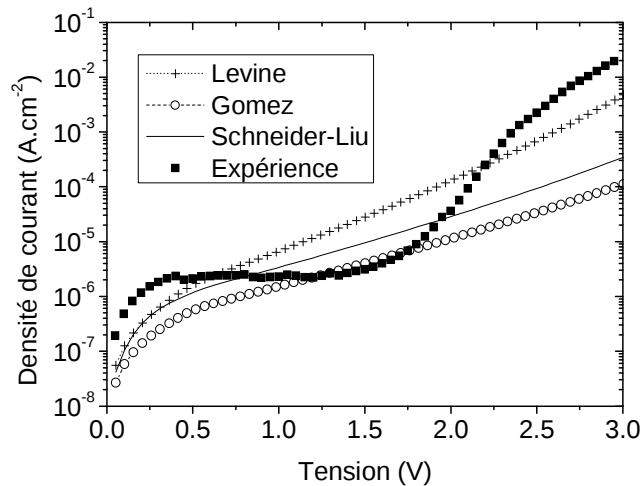
FIG. 3-3 : Comparaison des courbes I(V) expérimentales et théoriques issues du modèle WKB
