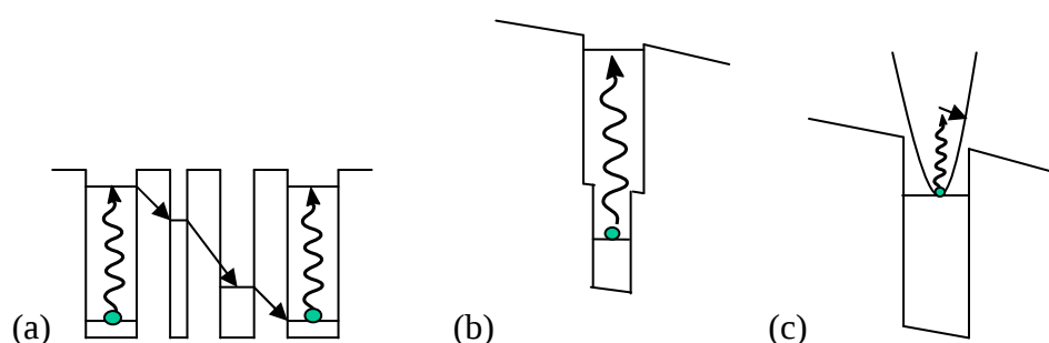
FIG. 1-10 (a) Détection dans un QCD. (b) QDIP en version DWELL. (c) QWISP.
