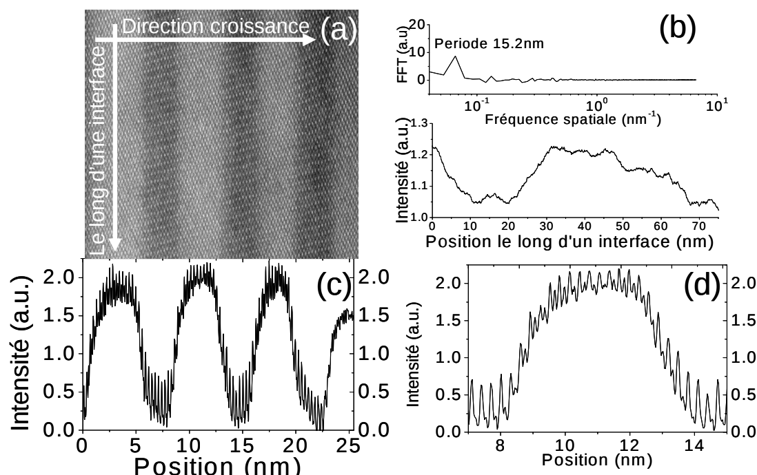
FIG. 5-11 : A gauche (a) Image STEM HAADF faite dans la direction 100 (b) en haut FFT de ce même profil, il est possible d'identifier deux pic de période 15 et 38 nm (c) Profil d'intensité fait le long de l'axe de croissance. (d) zoom sur le profil (c), chaque pic correspond à une colonne atomique.
