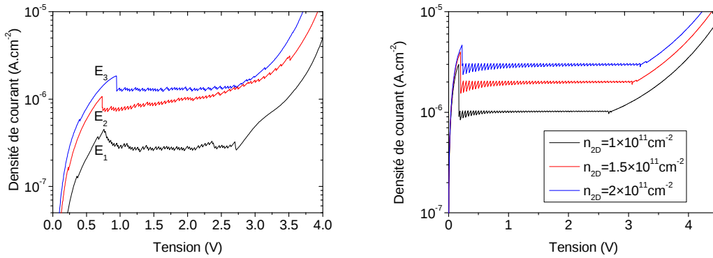
FIG. 6-12 : Courbe I(V) pour les composants de la série E. A gauche courbes expérimentales et à droite courbes simulées.
