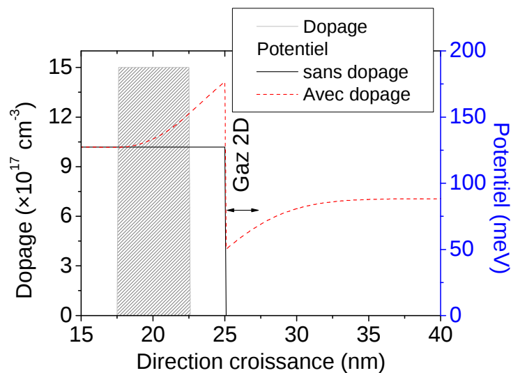
FIG. 1-4 : Profil de potentiel d'une interface de \text{Al}_{0.15}\text{Ga}_{0.85}\text{As}/\text{GaAs} en présence d'un fort dopage dans la barrière. Présence d'un gaz bidimensionnel d'électrons à l'interface entre GaAs et AlGaAs. De tels systèmes sont à présent disponibles de façon commerciale au prix de quelques centaines d'euros pour un wafer de trois pouces.
