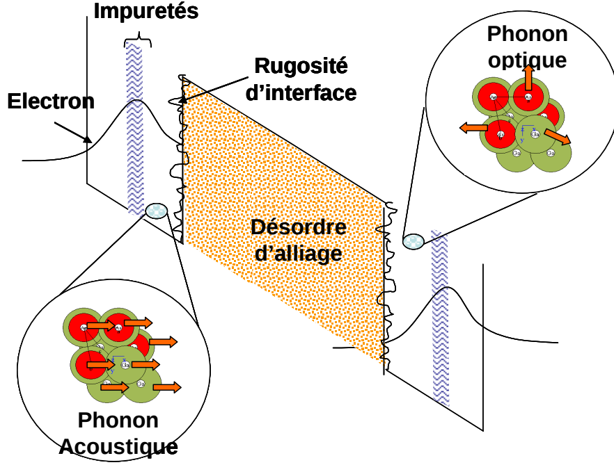
FIG. 4-5 : Schéma des interactions prises en compte par notre modélisation
