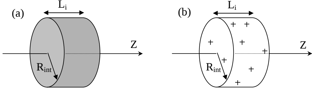
FIG. 5-14 (a) Volume d'intégration du potentiel écranté dans le cas d'une distribution homogène de charges. (b) Volume d'intégration du potentiel écranté dans le cas d'une distribution discrète de charges.
