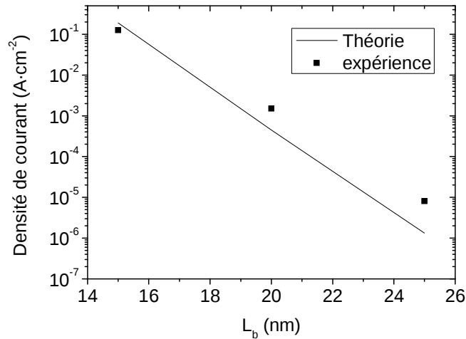
FIG. 4-13 Effet de la taille de barrière sur un QWIP 8.5\mu m ( L_w=49\text{\AA} , dopage 2 \times 10^{11} \text{cm}^{-2} ), sous un champ de 10 \text{kVcm}^{-1} et T \sim 40 \text{K} . Points expérimentaux fournis par Alcatel Thales 3-5 Lab.
