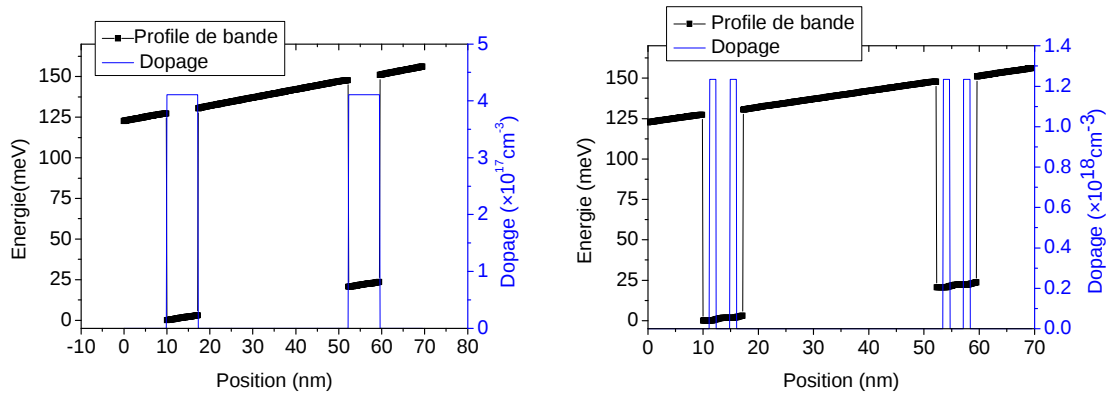
FIG. 5-9 : A gauche, Profil de bande sous un champ de 5\text{kVcm}^{-1} , dopage créneau sur toute la largeur du puits. A droite, Profil de bande sous un champ de 5\text{kVcm}^{-1} , double dopage créneaux entre le 1 er et le 2 ème sixième du puits, puis entre le 4 ème et le 5 ème sixième du puits
