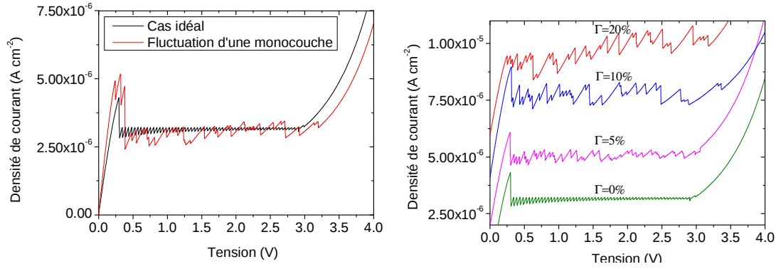
FIG. 6-14 : A gauche : effet des fluctuations de la taille (sans affecter le couplage) de la barrière sur la courbe I(V) . A droite : Effet de la fluctuation continue de la taille de la barrière sans changement du dopage, avec décalage des courbes de 2 \times 10^{-6} \text{ A cm}^{-2} entre chaque courbe.
