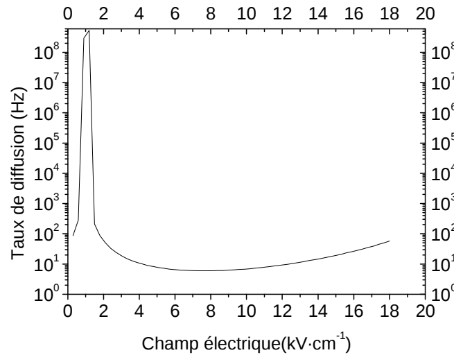
FIG. 4-9 Taux de diffusion en fonction du champ électrique pour une structure à deux puits asymétriques. Le puits amont passe de 73 Å à 80 Å et le puits aval est inchangé (73 Å). La mise en résonance des niveaux se produit pour F \approx 1 \text{ kVcm}^{-1} .
