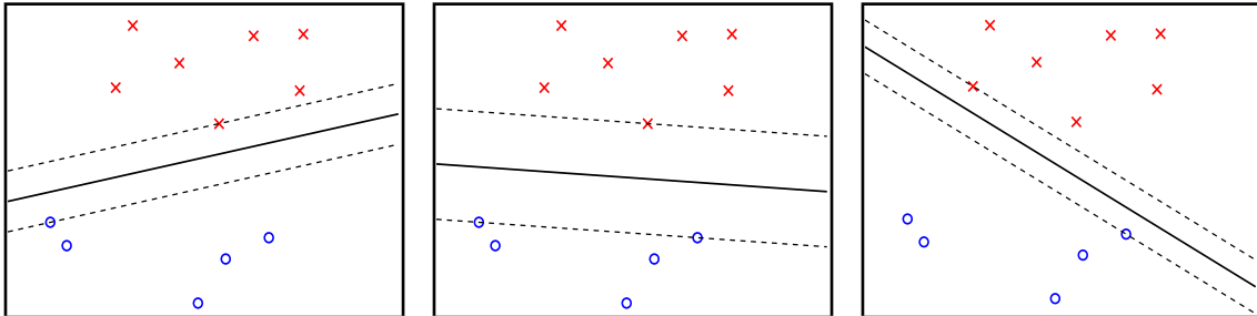
FIGURE 3.1 – Exemples d'hyperplans de séparation (en trait plein) et d'hyperplans de marge (en pointillés), entre deux classes dont les exemples sont respectivement représentés par des cercles et des croix.
