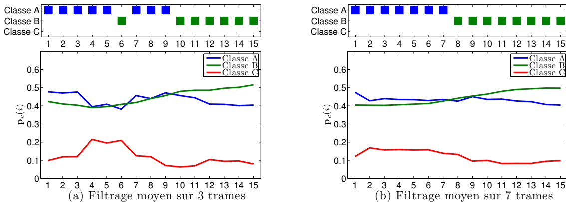
FIGURE 8.2 – Probabilités \tilde{p}_c(i) après filtrage moyen sur des fenêtres glissantes de (a) 3 et (b) 7 trames. Les labels des classes majoritaires sont indiqués dans le cadre supérieur.
