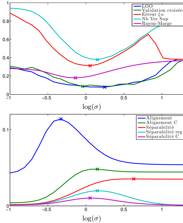
FIGURE 4.8 – Comparaison des valeurs optimales \hat{\sigma} du paramètre \sigma estimées par chaque critère sur la base Spambase , et de l'erreur Leave-One-Out pour ces valeurs, avec C = 1 .
