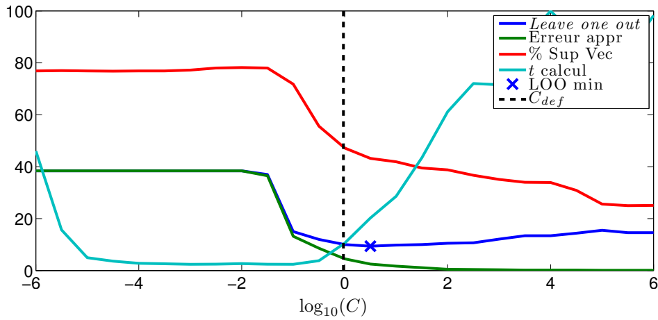
FIGURE 4.5 – Évolution des erreurs Leave-one-out et d'apprentissage, ainsi que du taux de vecteurs de support et du temps d'apprentissage (ici en pourcentage par rapport au temps maximal observé), par rapport aux variations du facteur C , sur la base Spambase . La ligne noire pointillée indique la valeur C_{def} définie par Joachims, et la croix bleue le minimum de l'erreur Leave-one-out . Le temps de calcul relatif ( t calcul) figure ici en pointillés à titre informatif.
