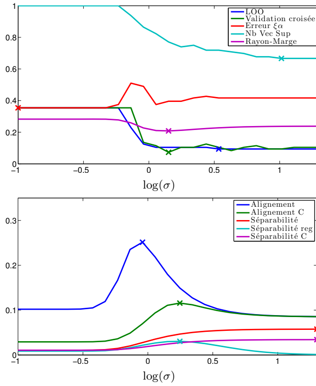
FIGURE 4.11 – Comparaison des valeurs optimales \hat{\sigma} du paramètre \sigma estimées par chaque critère sur la base Lymphoma , et de l'erreur Leave-One-Out pour ces valeurs, avec C = C_{def} .
