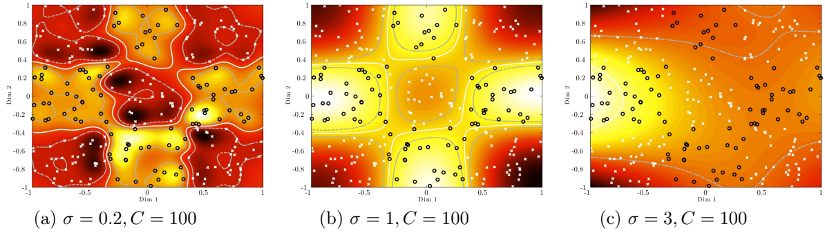
FIGURE 4.2 – Surfaces de décision obtenues par apprentissage SVM à noyau gaussien RBF pour différentes valeurs de \sigma sur la distribution Echiquier .
