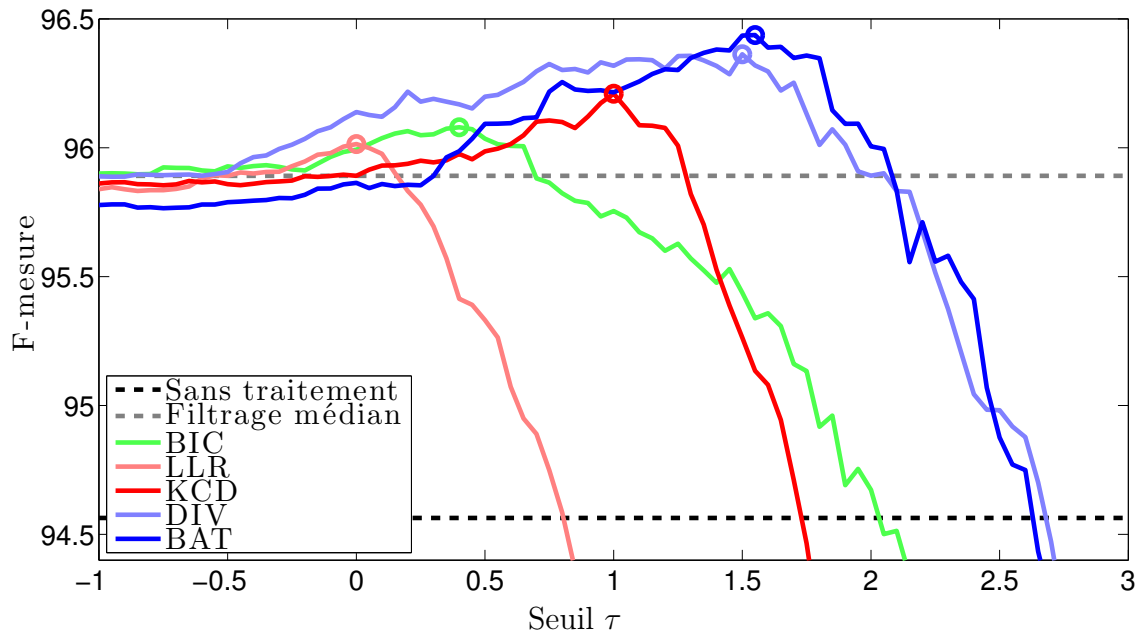
FIGURE 10.6 – Évolution de la F-mesure globale sur l'ensemble de validation par rapport au seuil \tau , pour chacune des mesures de détection de rupture.
