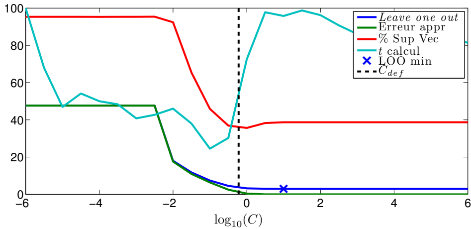
FIGURE 4.7 – Résultats de la même expérience sur la base parole/musique .
