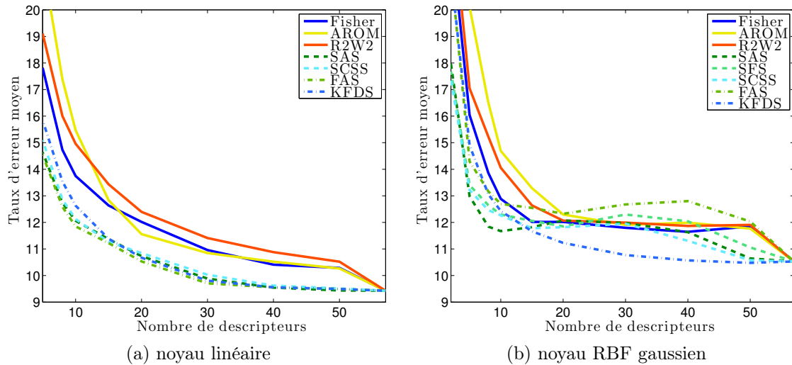
FIGURE 7.2 – Comparaison des performances entre les différentes méthodes sur la base Spambase .
