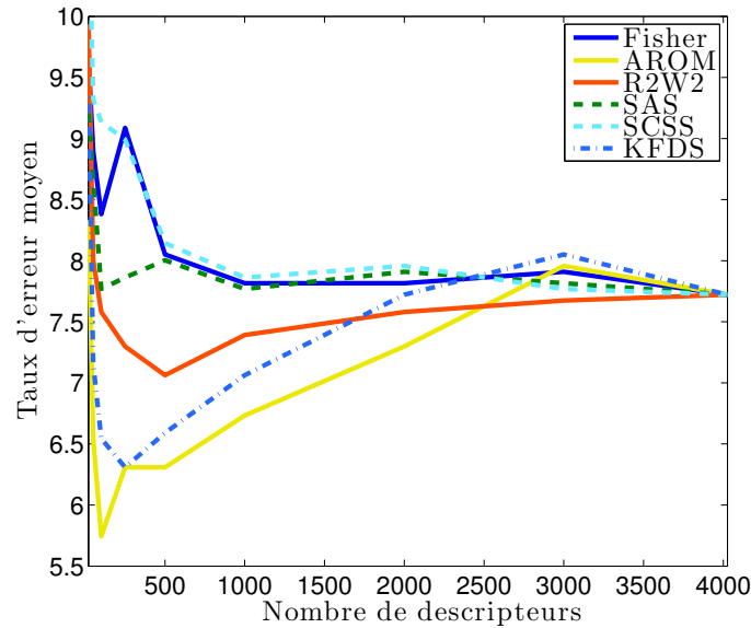
FIGURE 7.4 – Comparaison des performances entre les différentes méthodes sur la base Lymphoma .
