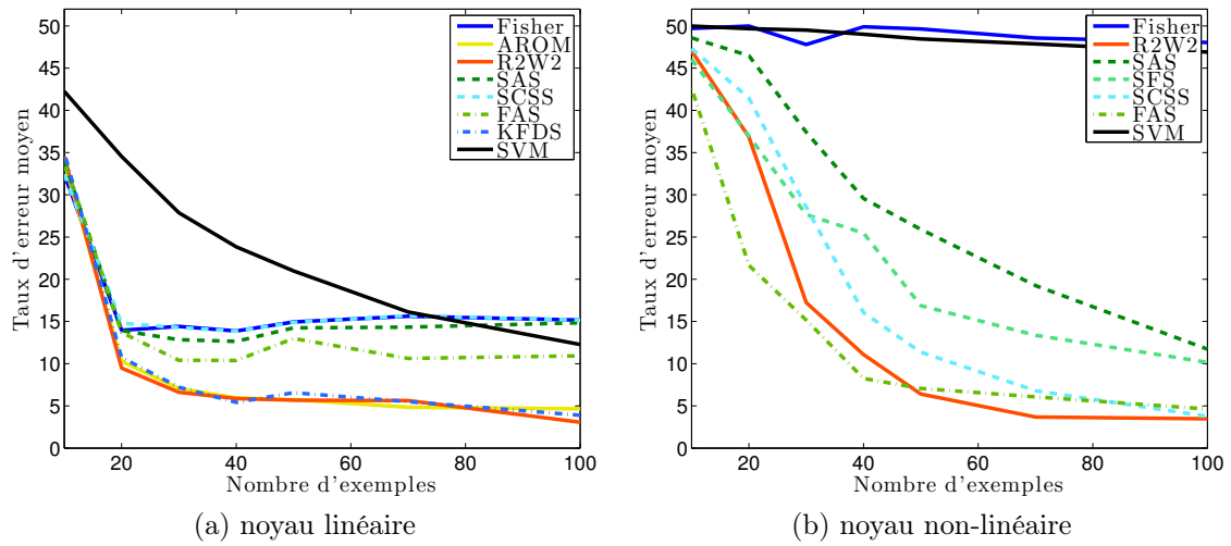
FIGURE 7.1 – Comparaison des performances sur un problème séparable linéaire (a) et un problème non-séparable linéaire (b), impliquant un grand nombre de descripteurs bruités.
