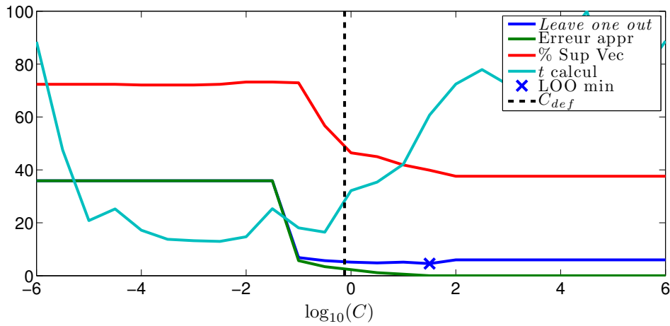
FIGURE 4.6 – Résultats de la même expérience sur la base Ionosphere .
