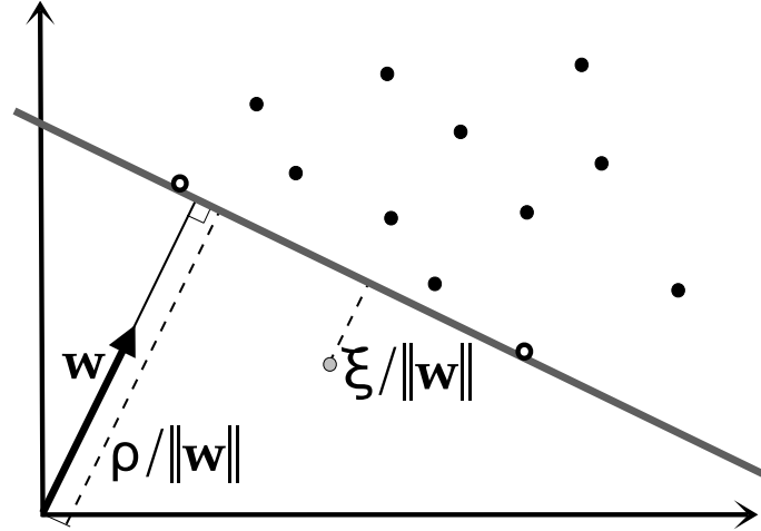
FIGURE 9.4 – Séparation des exemples avec l’origine par l’hyperplan (en gris foncé) défini par le vecteur normal \mathbf{w} , sur une projection schématisée en 2D de l’espace transformé. La figure montre trois vecteurs de support, dont deux à la marge (en blanc) et un autre mal classifié (en gris), dont la distance avec l’hyperplan définit la pénalité \xi .
