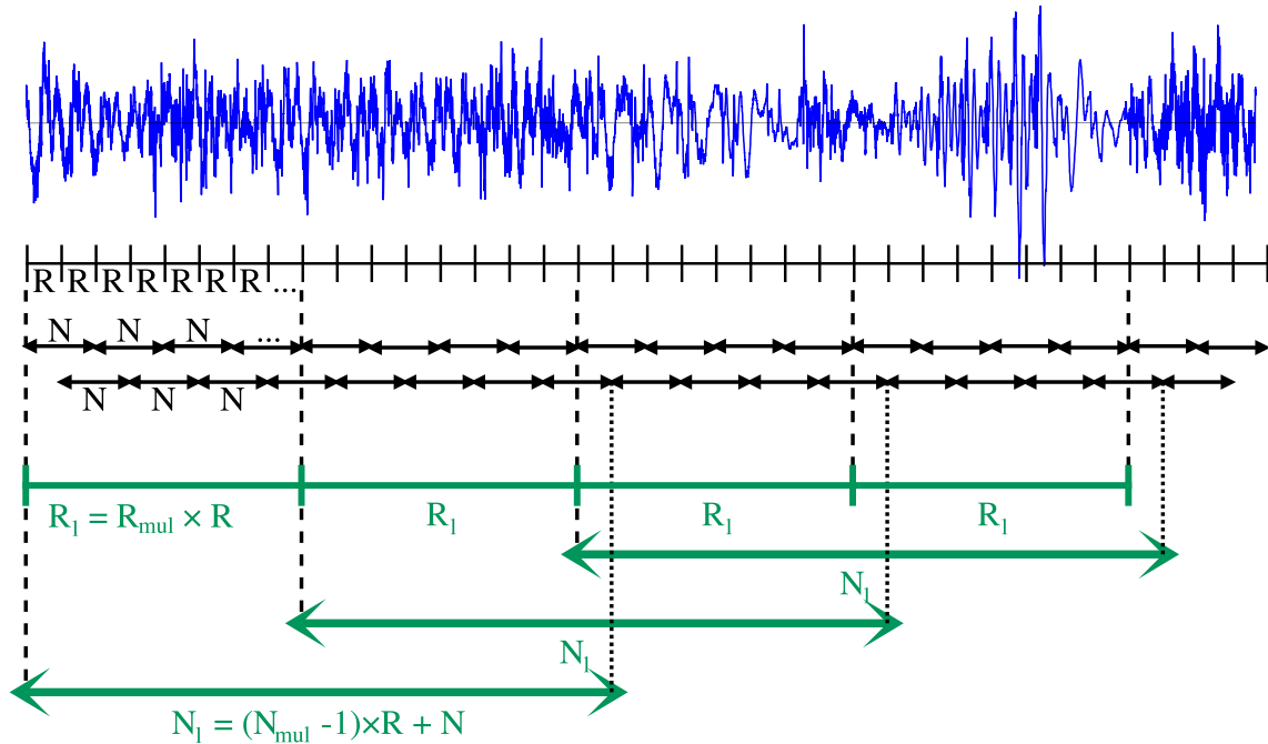
FIGURE 6.2 – Représentation de la synchronisation entre les frontières de trames courtes (segments fléchés en noir) et de trames longues (segments fléchés en vert).
