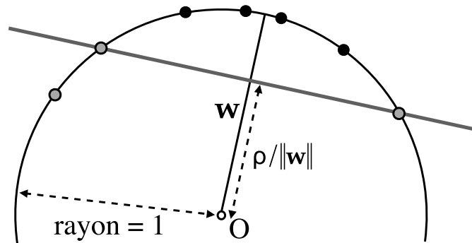
FIGURE 9.5 – La figure montre un exemple d'application de SVM à une classe. La contrainte de normalisation du noyau implique que, dans l'espace transformé, les exemples sont situés sur l'hypersphère de rayon 1. On peut y voir 3 vecteurs de support (en gris), dont deux sont à la marge, et le troisième mal classifié. Cette figure s'inspire d'une figure de l'article de Désobry et al. [63].
