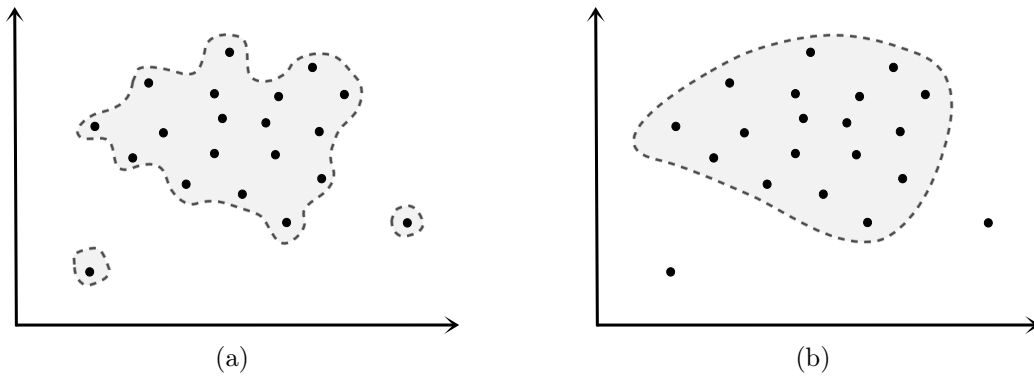
FIGURE 9.3 – Estimation du support d'une distribution sur un cas simple à deux dimensions, présentant deux exemples marginaux ( outliers ). Comparaison entre (a) un cas de sur-apprentissage, et (b) un cas correctement régularisé.
