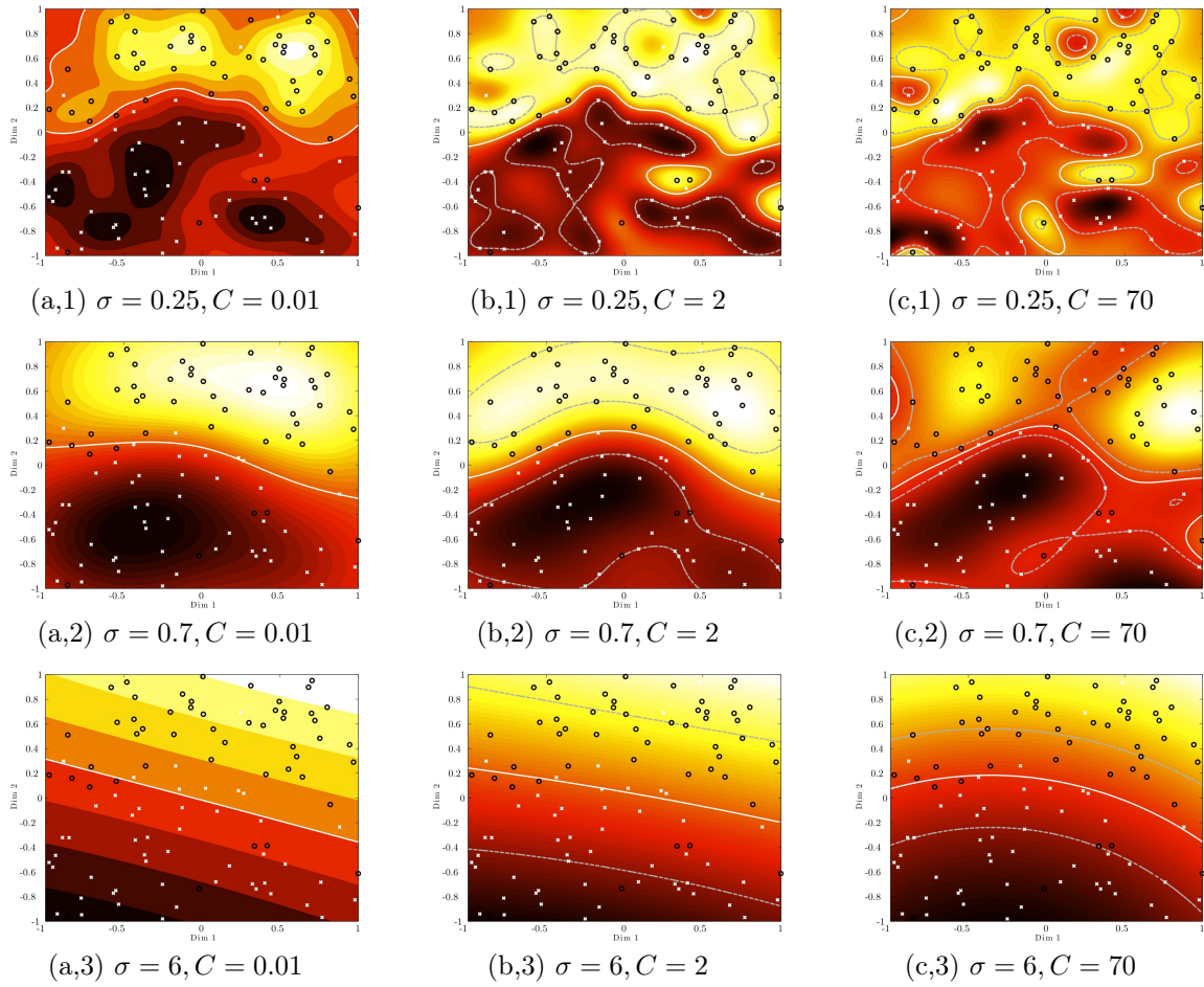
FIGURE 4.4 – Surfaces de décision obtenues par apprentissage SVM à noyau gaussien RBF pour différentes valeurs de \sigma et C sur la distribution Courbe .
