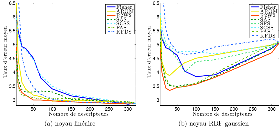
FIGURE 7.5 – Comparaison des performances entre les différentes méthodes sur la base parole/musique .
