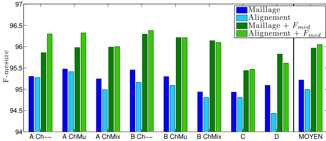
FIGURE 10.4 – Comparaison des résultats (en F-mesure) sur les différentes taxonomies après affinage des noyaux par recherche par maillage ou par optimisation de l’alignement, avec et sans filtrage médian.
