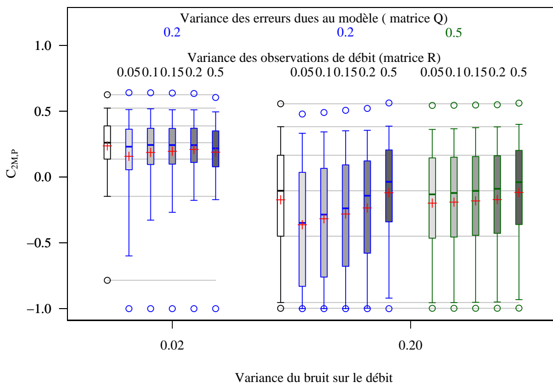
FIGURE 15.7 – Distributions (sur 178 bassins \times 2 périodes) des valeurs du critère de performance C_{2M,P} obtenues par le modèle GRP mis-à-jour par le filtre de Kálmán, quand le débit assimilé est perturbé par un bruit gaussien d'écart-type 0.02 \cdot Q_t (à gauche) ou 0.20 \cdot Q_t (à droite). L'horizon est de 6 heures. Pour chaque niveau de bruit, différentes paramétrisations des matrices de variance-covariance \mathbf{Q}_t et \mathbf{R}_t sont testées. Nous indiquons la valeur de la variance des erreurs d'observation (matrice \mathbf{R}_t ) en noir et la valeur de la variance des erreurs sur le niveau du réservoir de routage (matrice \mathbf{Q}_t ) en couleur. La boîte à moustache dessinée en noir correspond au cas où la mise-à-jour est complète.
