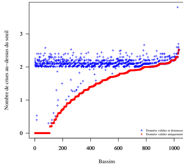
FIGURE H.1 – Nombre de pics de crues par an au dessus du débit de période de retour 6 mois Q^{[6 \text{ mois}]} , selon que les données douteuse sont prises en compte (+) ou non (×). Les débits Q^{[6 \text{ mois}]} ont été calculés par l’algorithme sup-seuil à partir de toutes les données disponibles pour chaque bassin. Les bassins sont classés par le nombre de pics au dessus du débit Q^{[6 \text{ mois}]} quand seules les données validées sont prises en compte.
