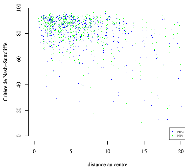
FIGURE G.15 – Distribution du critère de Nash-Sutcliffe ( \times 100 ) en contrôle représentée en fonction de la distance à l'origine dans l'espace des 6 indices décrivant le débit (en haut) et dans l'espace des 10 indices décrivant les régimes hydrographiques et pluvieux (en bas).
