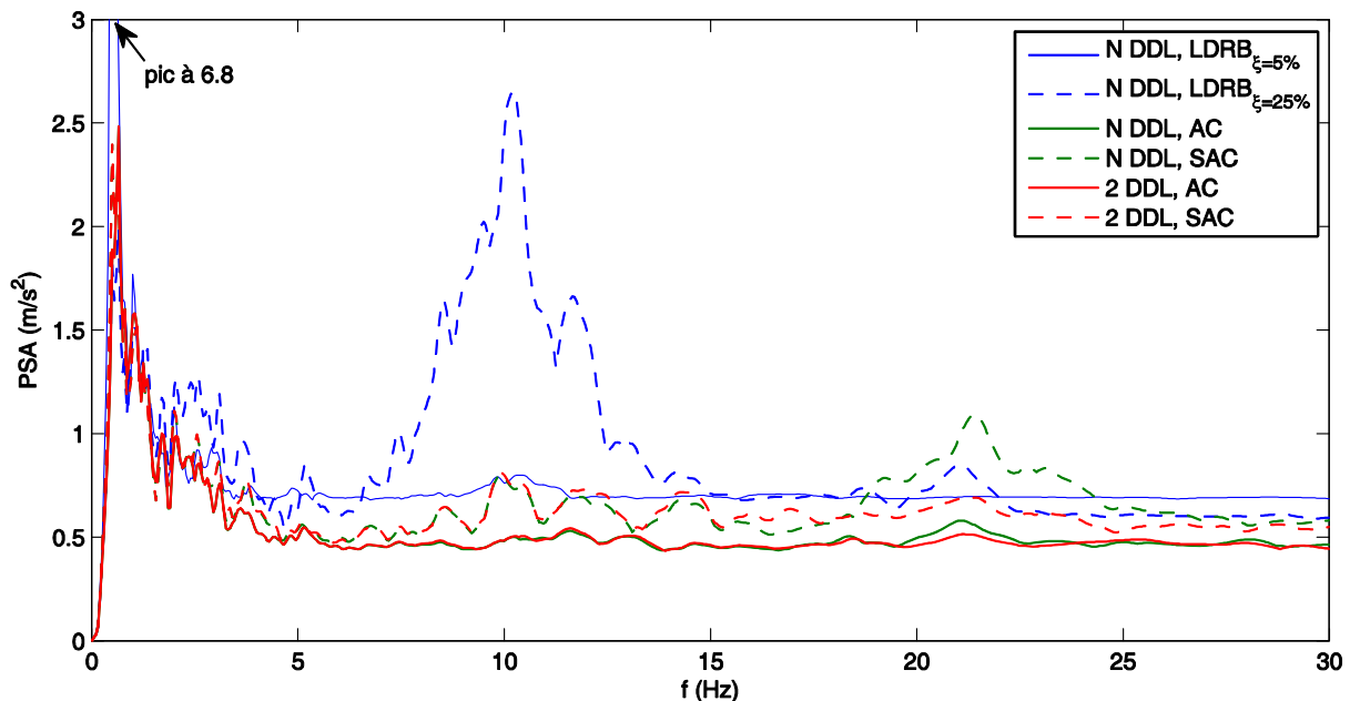
Figure 5.12. Spectres en pseudo-accélération (PSA) de la base du système à plusieurs DDL, pour un taux d'amortissement de 2%
