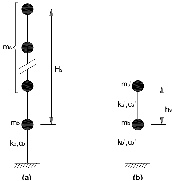
Figure 5.8. Modèles de structures : a) à plusieurs DDL ; b) à deux DDL
