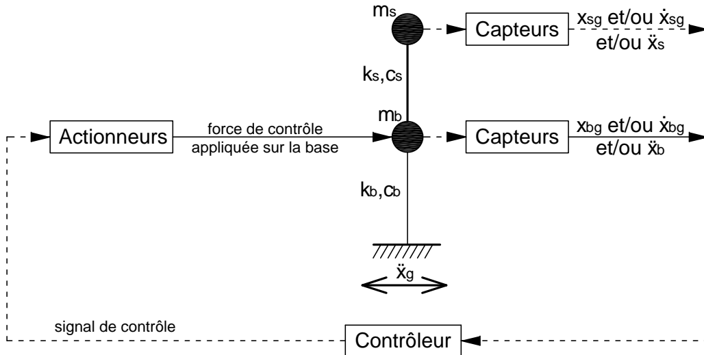
Figure 5.2. Modèle à deux DDL en boucle fermée
