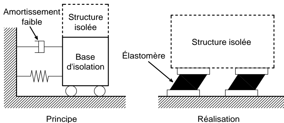
Figure 2.1. Appuis élastomères simples (LDRB – « Low Damping Rubber Bearings »)
