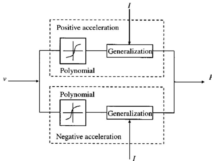
Figure 6.9. Modèle polynomial pour l'amortisseur MR [74]
