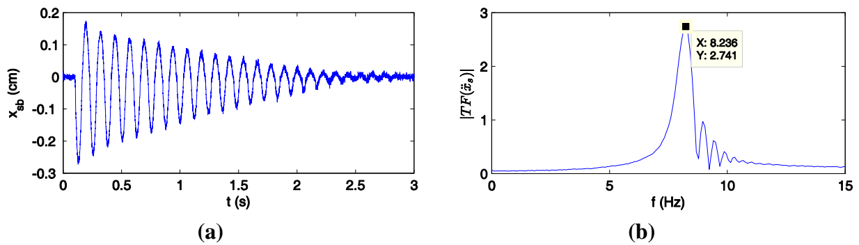
Figure 7.5. Essai de choc à base bloquée : a) déplacement relatif de la superstructure par rapport à la base ; b) module de la transformée de Fourier (TF) de l'accélération absolue de la superstructure
