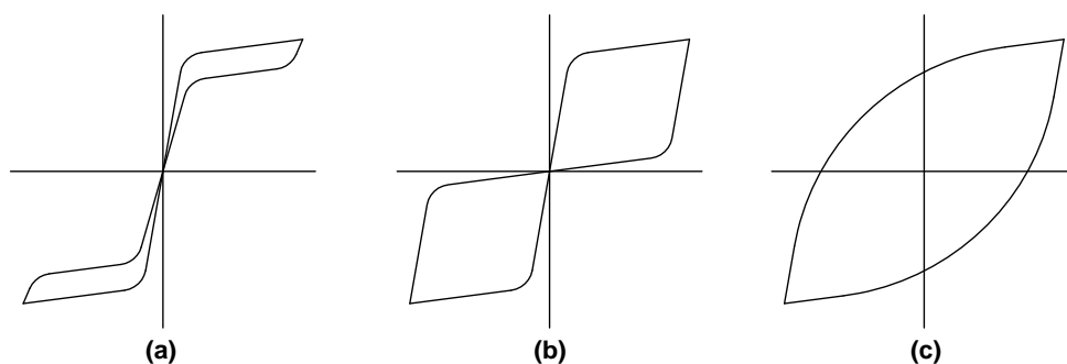
Figure 2.8. Comportements typiques des dispositifs d'isolation de SMA [17] : a) Dispositifs de recentrage supplémentaire ; b) Dispositifs de recentrage ; c) Sans dispositifs de recentrage
