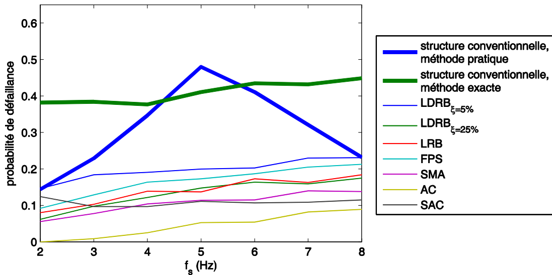
Figure 3.9. Probabilité de défaillance des superstructures élastiques bilinéaires en fonction du type d'appui
