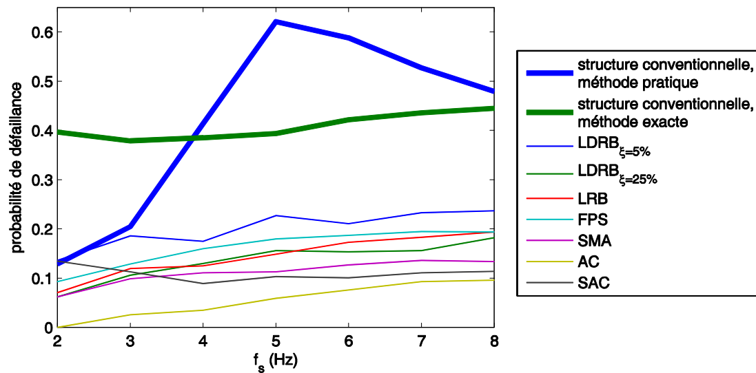
Figure 3.10. Probabilité de défaillance des superstructures OVO en fonction du type d'appui
