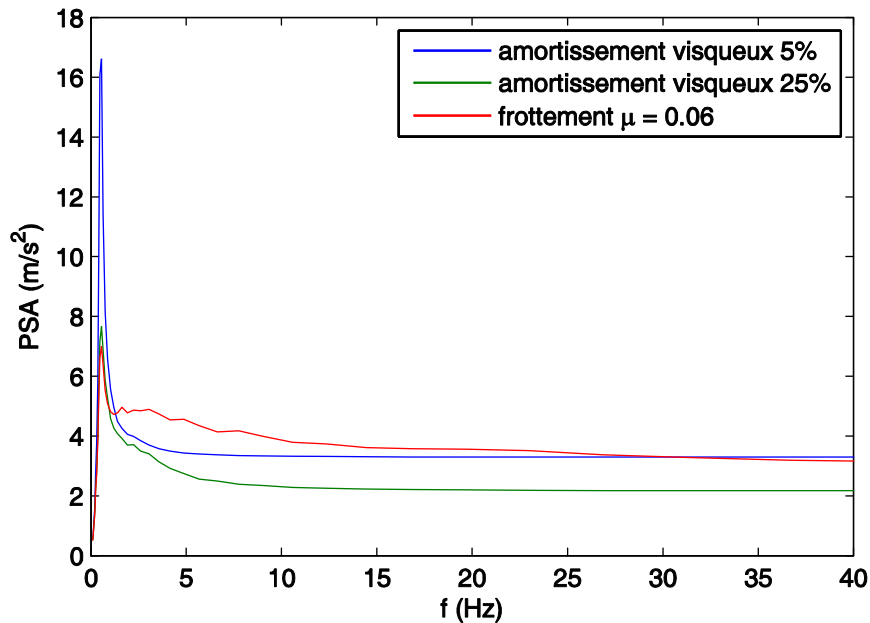
Figure 4.15. Spectre de plancher en pseudo-accelération (PSA) (2% amortissement, moyen de 100 signaux) du système à 1 DDL
