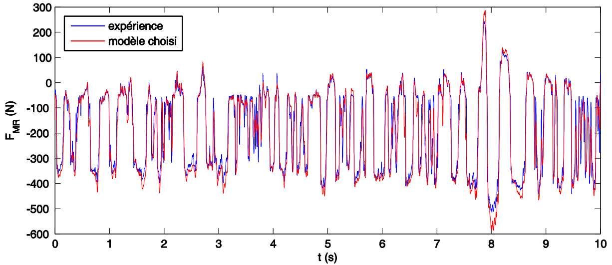
Figure 6.16. Comparaison entre la réponse de l'amortisseur MR et celle du modèle, soumis à un bruit blanc ( I = 0.05 A pour t < 5s , I = 0.1 A pour t > 5s )
