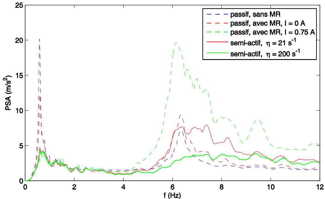
Figure 7.10. Spectre en pseudo-accélération (PSA) à la base d'une structure fictive
