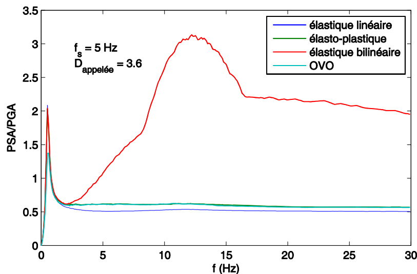
Figure 3.14. Spectres médians en pseudo-accelération normalisée à la base de la superstructure ( f_s = 5 Hz, D_{appelée} = 3.6 )
