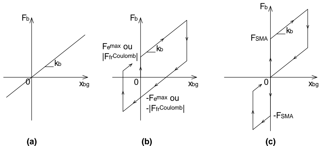
Figure 3.2. Comportements des appuis passifs utilisés dans le modèle : a) comportement linéaire des appuis LDRB \xi=5\% ou des LDRB \xi=25\% ; b) comportement des appuis LRB ou des FPS ; c) comportement des appuis SMA
