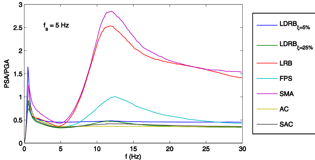
Figure 3.12. Spectres médians en pseudo-accélération (PSA) normalisée de la base d'une superstructure élasto-plastique ( f_s = 5 Hz)
