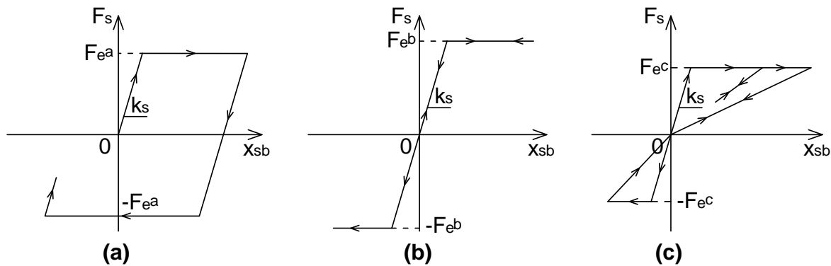
Figure 3.5. Comportements non-linéaires de la structure conventionnelle et de la superstructure : a) élasto-plastique ; b) élastique non-linéaire ; c) orienté-vers-l'origine (OVO)
