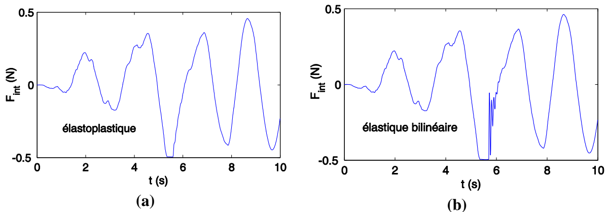
Figure 3.13. Évolution temporelle de la force interne F_{int} dans la superstructure ( f_s = 5 Hz, D_{appelée} = 3.6 ) : a) élasto-plastique ; b) élastique bilinéaire
