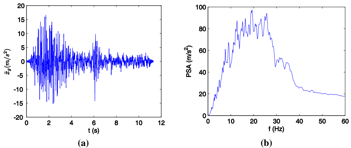
Figure 7.6. Signal d'accélération appliqué à la table vibrante : a) évolution temporelle ; b) spectre en pseudo-accelération (PSA) pour un taux d'amortissement de 2%
