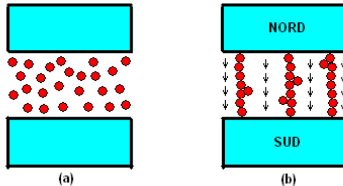
Figure 6.1. Formation des chaînes de particules ferromagnétiques dans un fluide MR : a) Sans champ magnétique ; b) Avec champ magnétique
