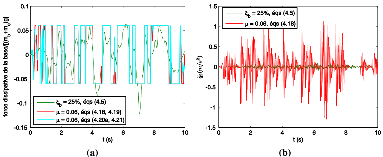
Figure 4.18. Évolution temporelle des forces dissipatives de la base et des accélérations modales : a) force visqueuse exacte, force de frottement exacte et approximative ; b) accélération du deuxième mode (amortissement et frottement)
