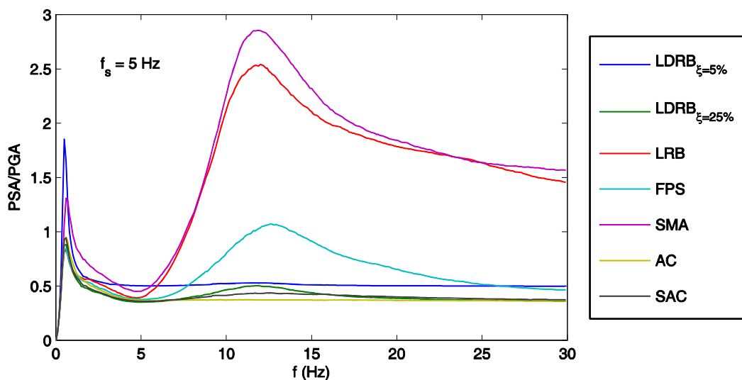
Figure 3.11. Spectres médians en pseudo-accélération (PSA) normalisée de la base d'une superstructure élastique linéaire ( f_s = 5\text{ Hz} )
