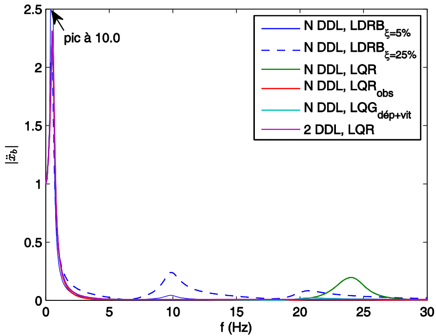
Figure 5.11. Amplitudes des fonctions de transfert de l'accélération absolue de la base du système à plusieurs DDL
