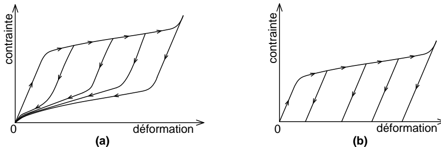
Figure 2.7. Comportement en tension uniaxiale des SMA : a) à température suffisamment élevée ; b) à température moins élevée
