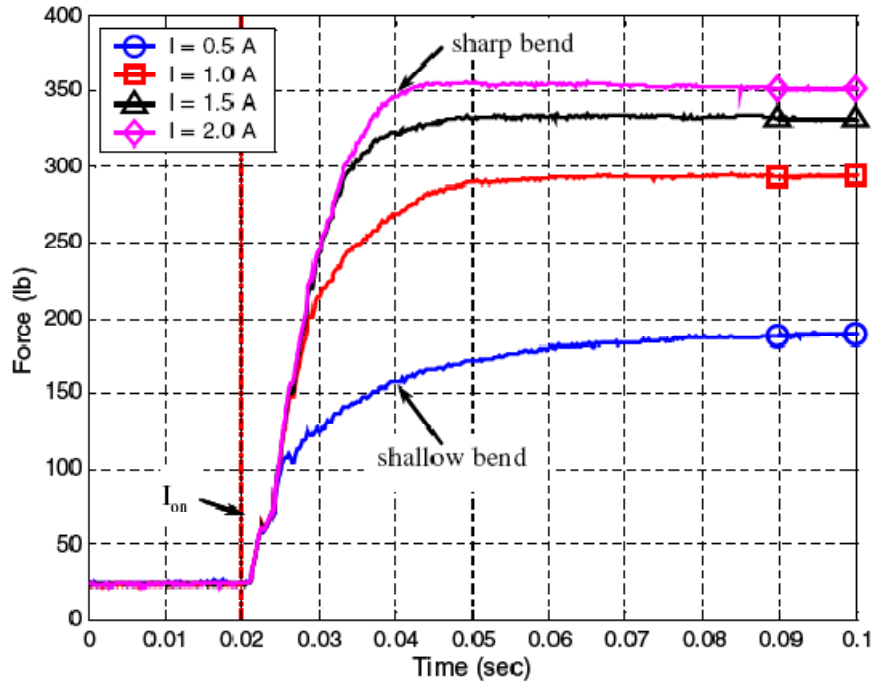
Figure 6.15. Temps de réponse de l'amortisseur MR pour différentes valeurs de courants [77]
