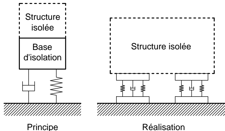
Figure 2.9. Boîtes à ressorts verticaux
