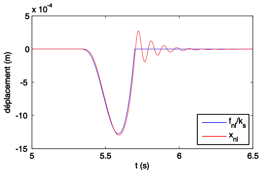
Figure 3.17. Évolution temporelle des forces non-linéaires et de la déformation due aux forces non-linéaires, pour une superstructure élastique bilinéaire ( f_s = 5 \text{ Hz} , D_{appelée} = 3.6 )
