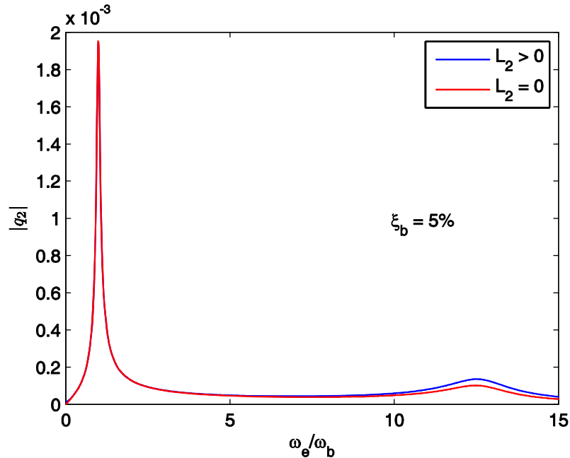
Figure 4.7. Module de la fonction de transfert de la réponse du deuxième mode
