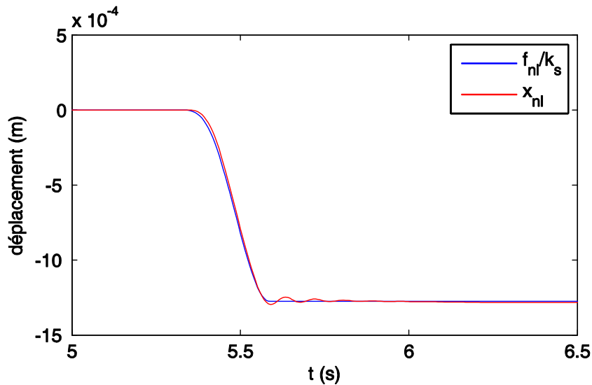
Figure 3.16. Évolution temporelle des forces non-linéaires et de la déformation due aux forces non-linéaires, pour une superstructure élasto-plastique ( f_s = 5 \text{ Hz} , D_{appelée} = 3.6 )
