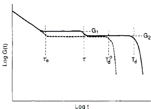
Figure 15 Comparaison schématique du module de relaxation en fonction du temps entre un polymère portant des groupes associatifs (ligne pleine) et un polymère non modifié (pointillés) ([32])
