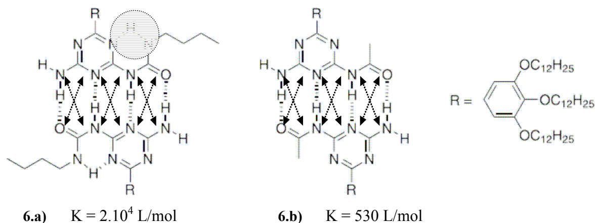
Figure 6 Structure de groupements auto-complémentaires proches de UPy, influence de la liaison hydrogène intramoléculaire. Cette comparaison montre que la séquence auto-complémentaire AADD (figure 3) est préférable à ADAD. Elle illustre aussi l'importance des liaisons hydrogène intramoléculaires.
