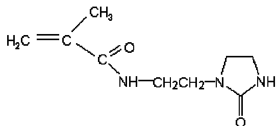
Figure 58 Monomère 2-méthyl-N-[2-(2-oxoimidazolidin-1-yl)éthyl]acrylamide utilisé dans la synthèse de PMMA porteurs de groupes associatifs
