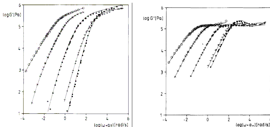
Figure 13 Modules élastiques ( G' ) et visqueux ( G'' ) pour un polybutadiène greffé par des groupes phényle-urazole à différentes concentrations : 0 % (●), 0,5 % (+), 2 % (*), 5 % (×) et 7,5 % (○). On s'aperçoit que plus le taux de greffage est élevé, plus la transition régime terminal/plateau caoutchoutique est déplacée vers les basses fréquences ([27]).
