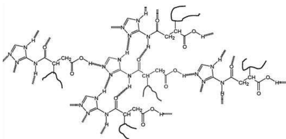
Figure 20 Association de stickers basés sur une triazole amide et un acide carboxylique ([42])
