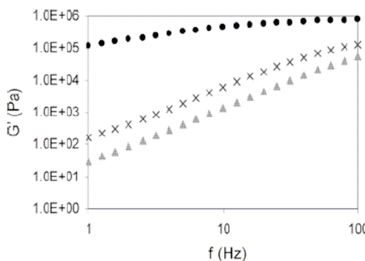
Figure 25 Module élastique en fonction de la fréquence à 100 °C pour des poly(éthylène-co-propylène) fonctionnalisés UPy : linéaire mono-fonctionnalisé (▲), linéaire di-fonctionnalisé (×) et étoile fonctionnalisée (●) ([58])
