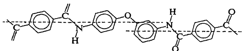
Figure 26 : Conformation de chaîne du 3,4'-POP-T [61]
