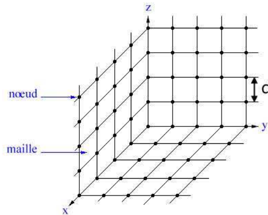
Figure 5 : Organisation tripériodique d'un cristal
