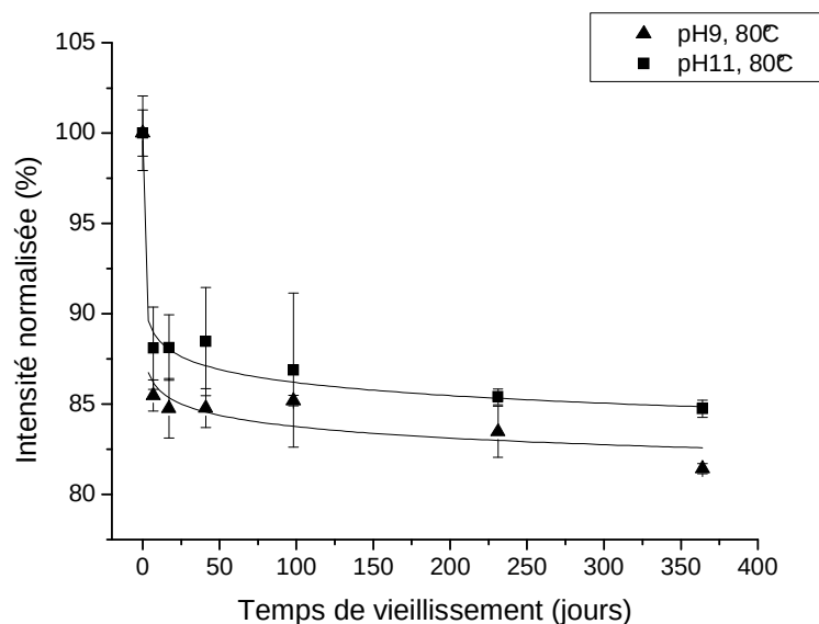
Figure 1 : Évolution de l'intensité normalisée du pic caractéristique de l'ensimage des fibres Twaron 1000 vieilles à pH9 et à pH11
