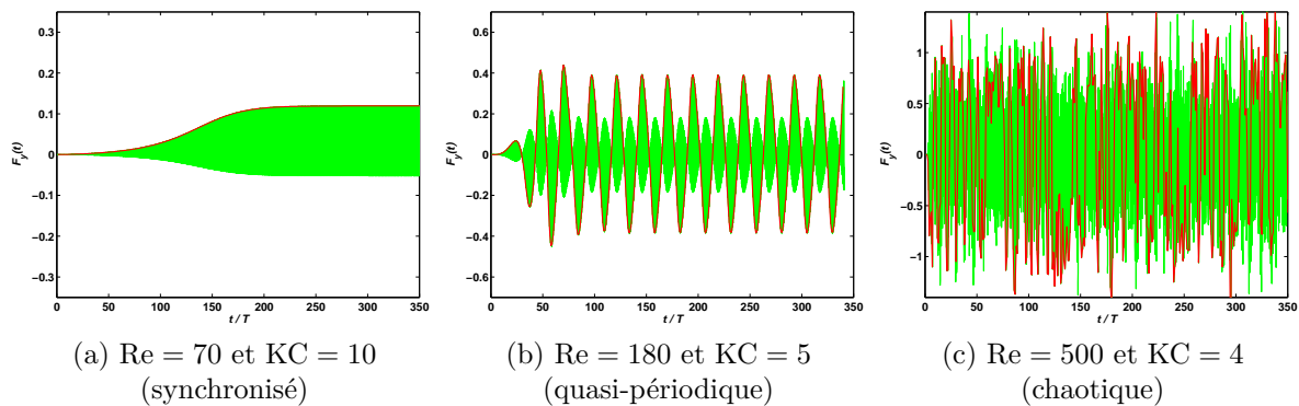
FIGURE 4.6 – Variations temporelles de la force de portance F_y(t) ( - ) et courbe constituée de son premier extremum à chaque période ( - ) pour trois couples (KC, Re) illustrant les trois types de régimes observés quand Re augmente le long de la frontière du régime A symétrique (voir la figure 4.5).
