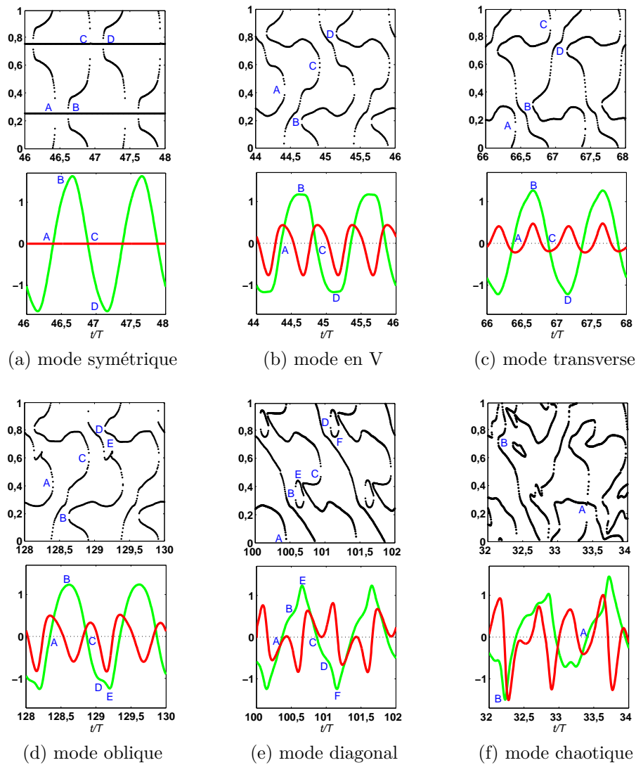
FIGURE 3.10 – Diagrammes spatio-temporels des points de vorticit   nulle sur le contour du cylindre (●) et variations temporelles de la force de tra  nee F_x(t) (—) et de la force de portance F_y(t) (—) sur deux p  riodes pour les six modes (a)-(f) d  finis par la figure 3.2.
