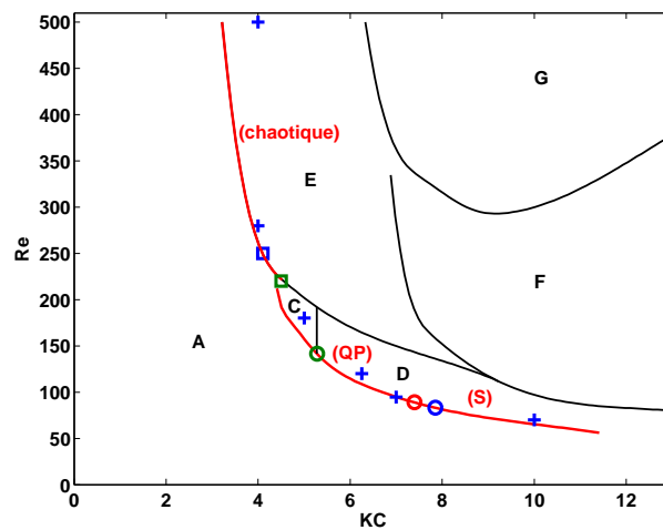
FIGURE 4.5 – Études de stabilité dans le plan ( KC , Re ) : — Frontières des régimes définis par Tatsuno & Bearman [7] ; — Courbe de stabilité marginale du régime symétrique d'après Elston [11, 70] ; + Points présentement étudiés (voir les figures 4.6 et 4.8) ; ○ Points critiques entre les régimes D synchronisé (S) et C quasi-périodique (QP) d'après [7] (○), d'après [70] (○), et d'après la formule (4.4) proposée (○) ; □ Points critiques entre les régimes C quasi-périodique et E chaotique d'après [7] (□) et d'après la formule (4.4) proposée (□).
