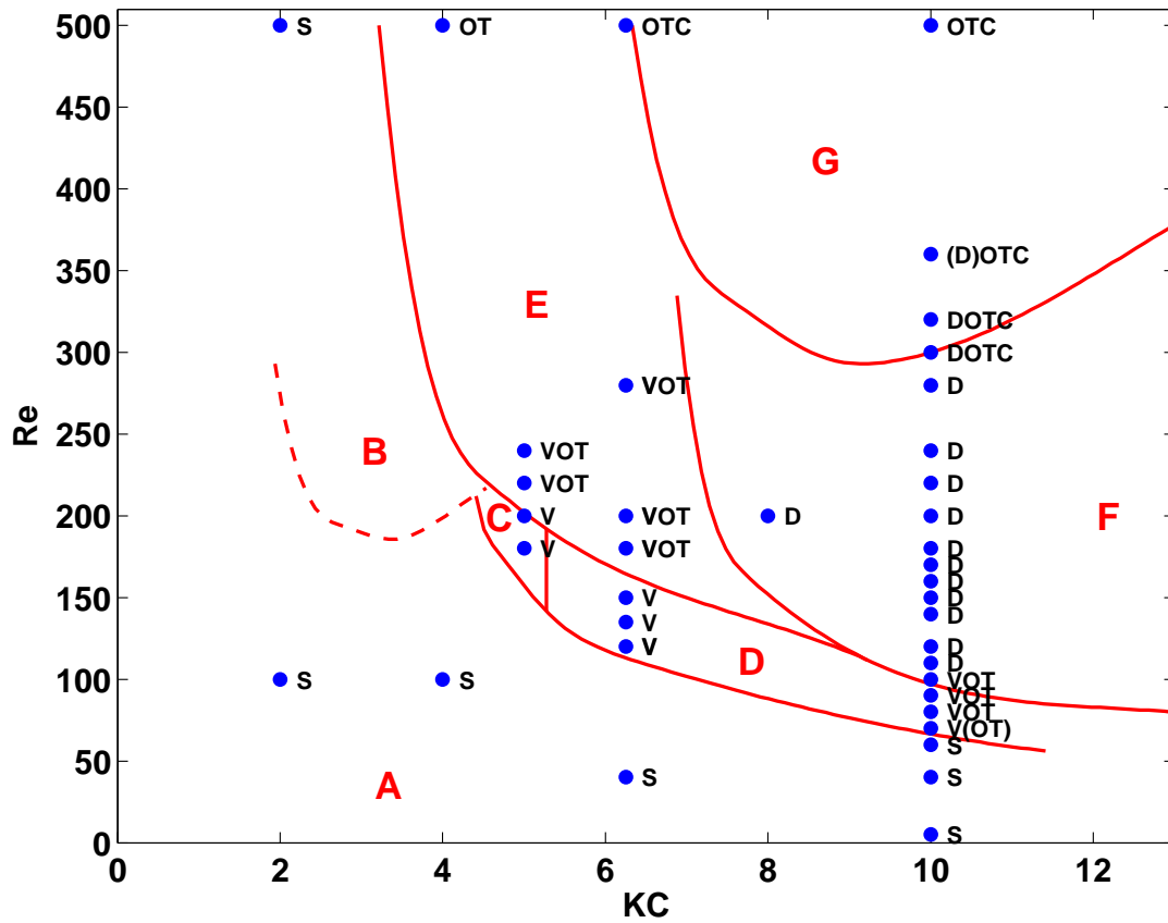
FIGURE 3.14 – Localisation des modes observés dans le plan (KC, Re) : (—) frontières des régimes de Tatsuno & Bearman [7], et (•) simulations numériques présentes. S : mode symétrique, V : mode en V, T : mode transverse, O : mode oblique, D : mode diagonal, C : mode chaotique.
