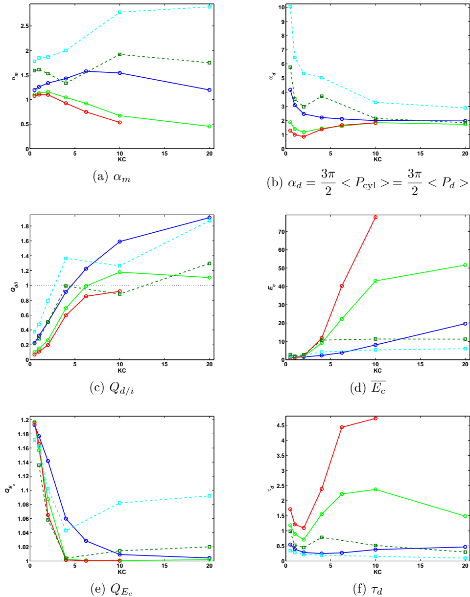
FIGURE 5.14 – Variations en fonction de KC des coefficients définis par les équations (1.13) et (5.5) à (5.8) pour le cylindre isolé à Re = 100 ( \bullet - \circ ), Re = 500 ( \bullet - \circ ) et Re = 1000 ( \bullet - \circ ), et pour le réseau de cylindres à Re = 100 ( \bullet - \square ) et Re = 500 ( \bullet - \square ).
