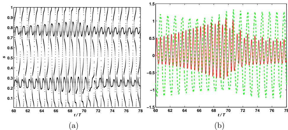
FIGURE 4.12 – (a) Diagramme spatio-temporel des points de vorticit   nulle sur le contour du cylindre et (b) forces de tra  n  e (---) et de portance (—) en fonction du temps pour KC = 10 et Re = 80 et 60T \leq t \leq 78T .
