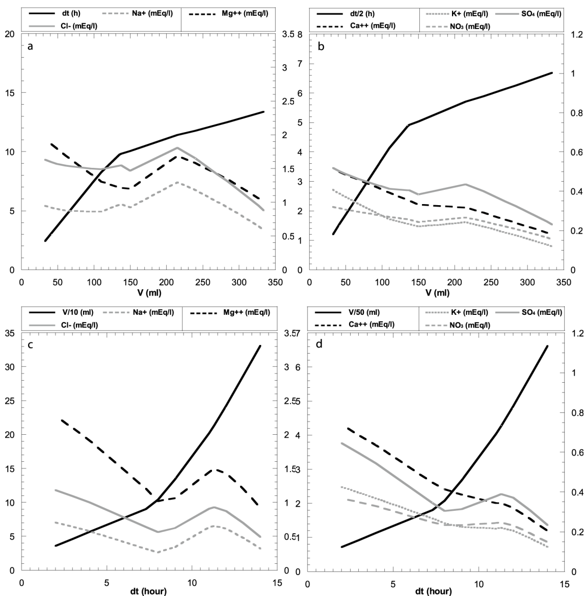
Figure V.11 : Corrélation entre les ions (mEq/l) avec le volume de rosée (V en ml) et le temps de condensation ( dt par heure). Les sels marins ( Na^+ , Cl^- : ordonnée gauche, Mg^{2+} : ordonnée droite) dans (a et c). Les espèces dérivés du sol ( Ca^{2+} : ordonnée gauche, K^+ : ordonnée droite) sont dans (b et d). Les ions ( NO_3^- , SO_4^{2-} , l'ordonnée droite) dans (b et d).
