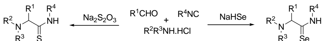
Schéma I.28 : Formation d' \alpha -aminothioamides et d' \alpha -aminosélénoamides
