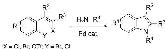
Schéma III.34 : Synthèse d'indole par double amination d'un dérivé du styrène
