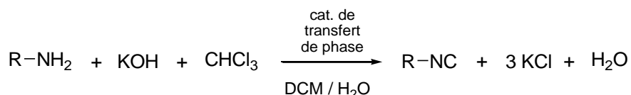
Schéma I.8 : Synthèse de Ugi à partir d'amines
