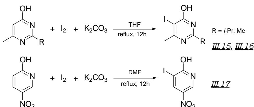
Schéma III.51 : Iodation de phénols hétérocycliques
