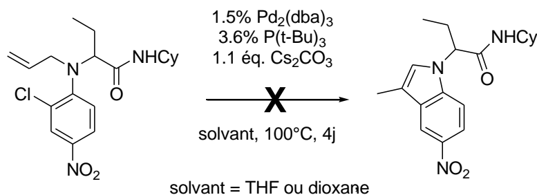
Schéma III.41 : Echec de la réaction de Heck avec un aryle chloré
