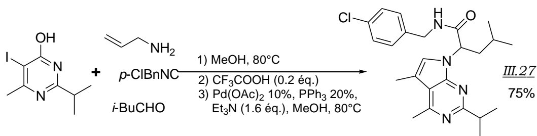
Schéma III.54 : Version one-pot du tandem Couplage Ugi-Smiles / Réaction de Heck
