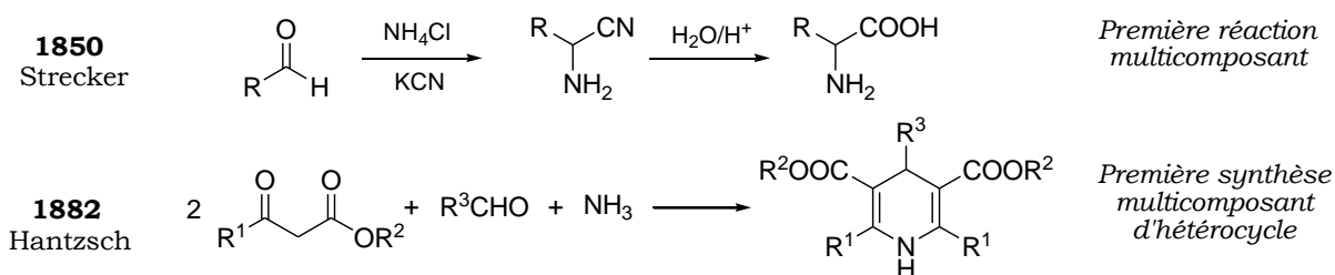
Schéma I.2 : Historique des réactions multicomposant
