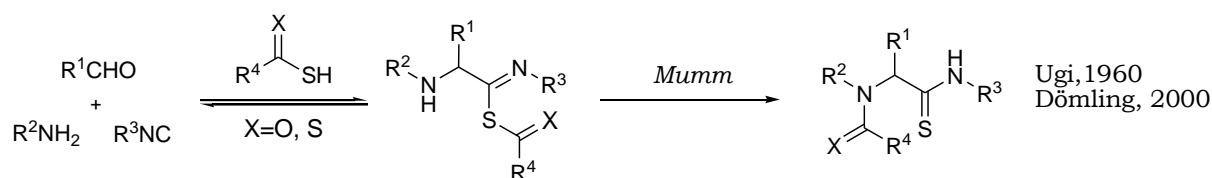
Schéma I.26 : Synthèse de dérivés de thioamides à partir d'acides thiocarboxyliques ou dithiocarboxyliques
