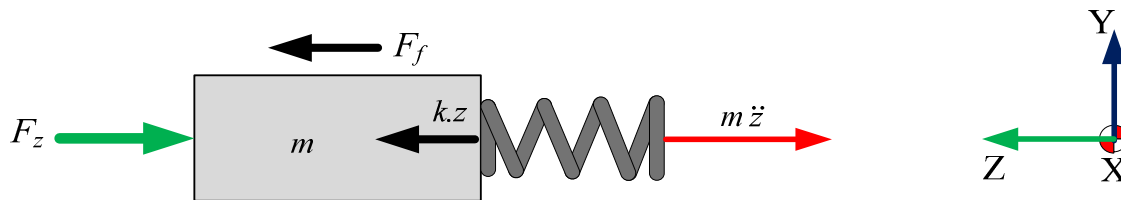
Figure 2.33 : Equilibre dynamique de la pièce au cours du test impulsionnel
