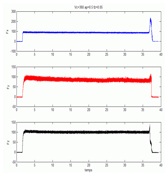
Essai 2 ( b=0.5\text{mm} , fz=0.05\text{mm/tr} )
