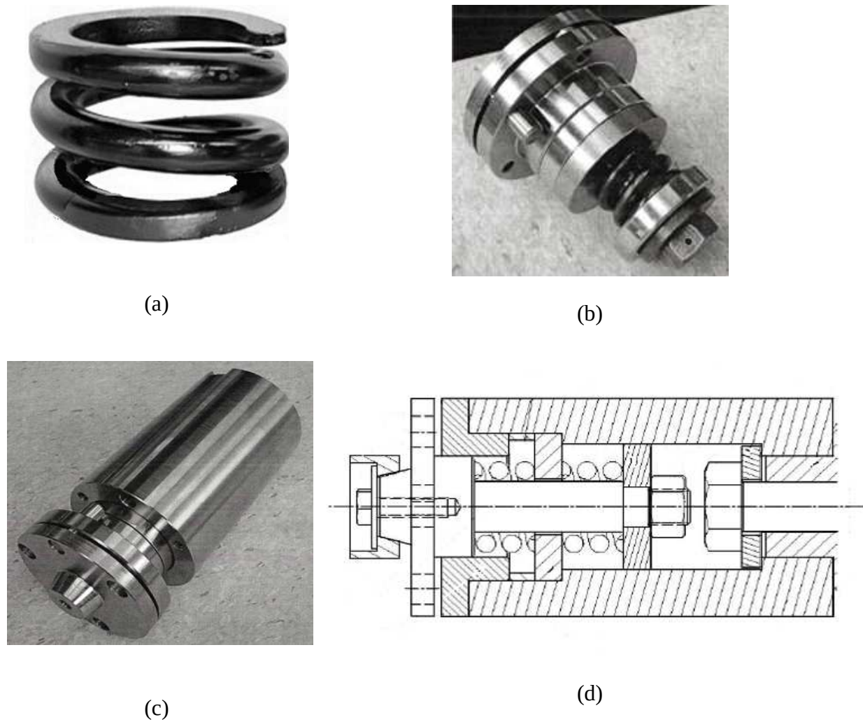
Figure 2.26 : Dispositif utilisant des ressorts hélicoïdaux, (a) ressort hélicoïdal, (b) masse vibrante, (c) dispositif démonté, (d) section du dispositif
