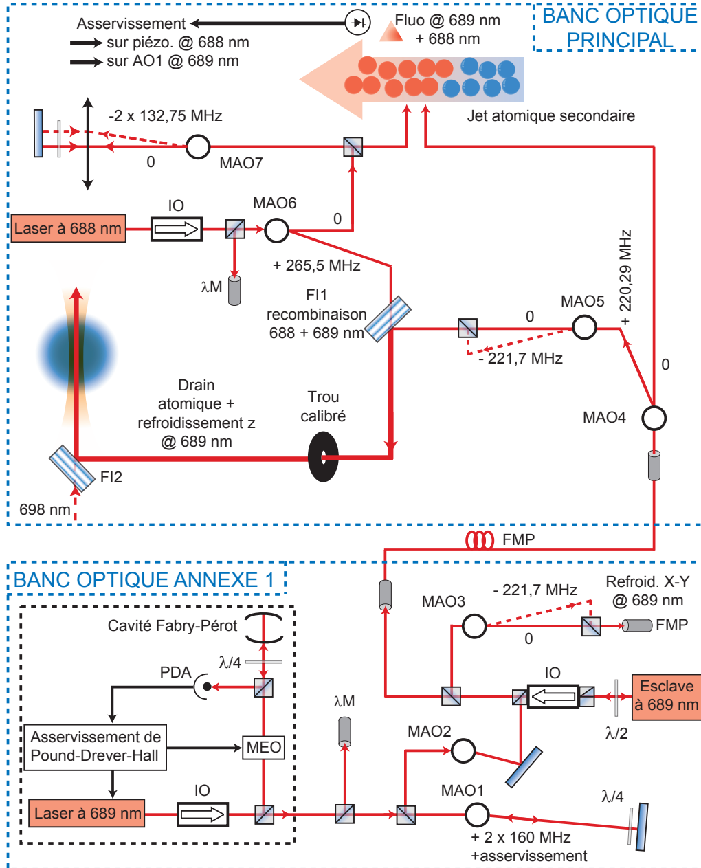
FIGURE 3.9 – Montage optique des lasers à 688 et 698 nm. FMP : Fibre à Maintien de Polarisation, MEO : Modulateur Electro-Optique, MAO : Modulateur Acousto-Optique, FI : Filtre Interférentiel, PDA : Photodiode à Avalanche, IO : Isolateur Optique, \lambda M : Lambdamètre. Les chemins en pointillés remplacent les chemins en trait plein lorsqu'on passe du ^{87}\text{Sr} au ^{88}\text{Sr} .
