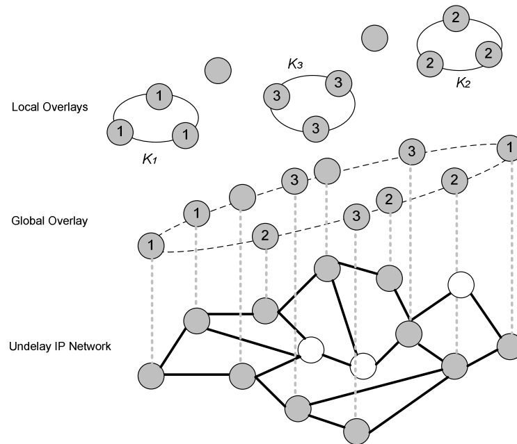
Figure 3. DHT sensible au contexte
