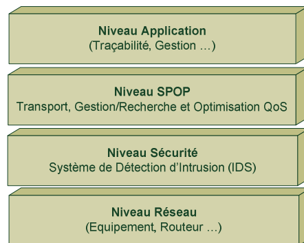
Figure 4. Les niveaux de l'architecture utilisée par l'application de sécurité intégrant SPOP
