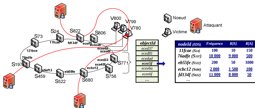
Figure 5. Distribution et Indexation avec Pastry
