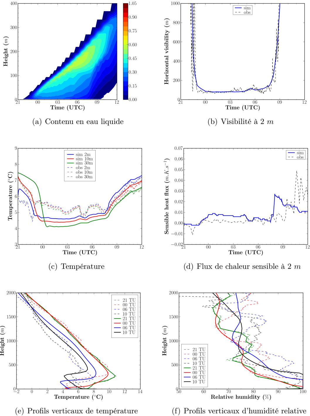
FIG. A.3 : Simulation démarrante à 21 TU avec le modèle diagnostique de Louis avec nudging ( C_n = 10^{-5} + 6.6 \cdot 10^{-3}(z) ). \mu_{min} = 0.05 \text{ m}^2 \cdot \text{s}^{-1} .
