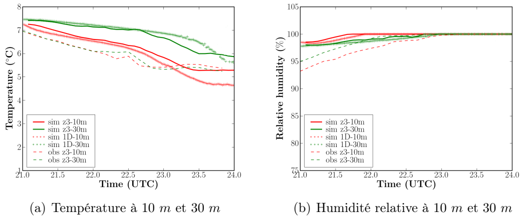
FIG. 5.7 : Phase de formation en cas homogène. Comparaison des observations et simulations pour la température et l'humidité relative en zone 3.
