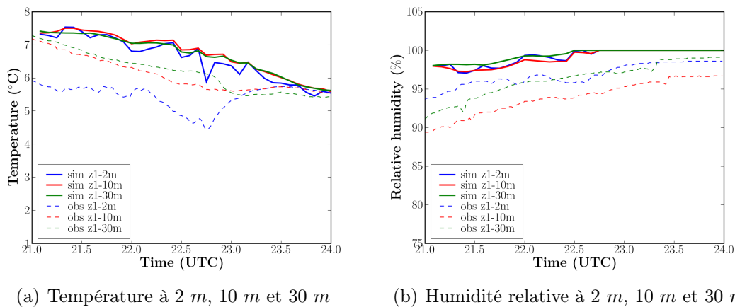
FIG. 5.27 : Phase de formation en cas avec le modèle de traînée. Comparaison des observations et simulations pour la température et l'humidité relative en zone 1.
