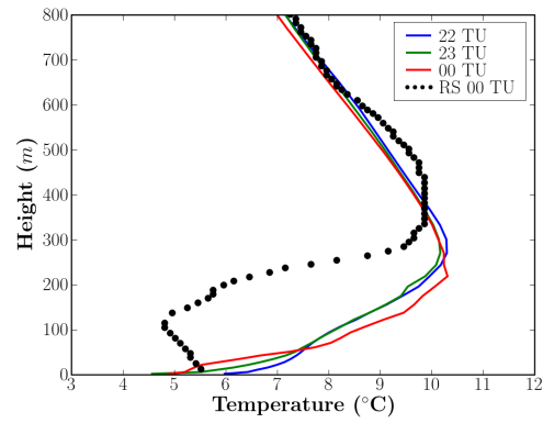
(b) Zone 3. Profils de température.
