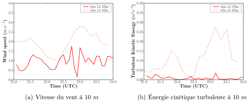
FIG. 5.26 : Phase de formation en cas avec le modèle de traînée. Comparaison des observations et simulations pour la vitesse du vent et l'énergie cinétique turbulente en zone 1.
