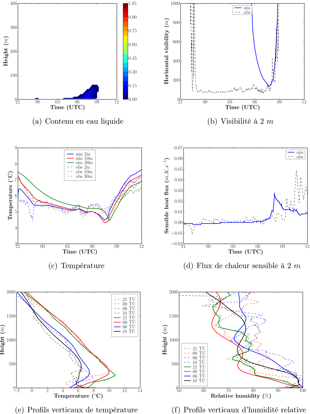
FIG. A.4 : Simulation démarrant à 21 TU avec le modèle diagnostique de Louis avec nudging ( C_n = 10^{-4} + 6.6 \cdot 10^{-3}(z) ). \mu_{min} = 0.05 \text{ m}^2 \cdot \text{s}^{-1} .
