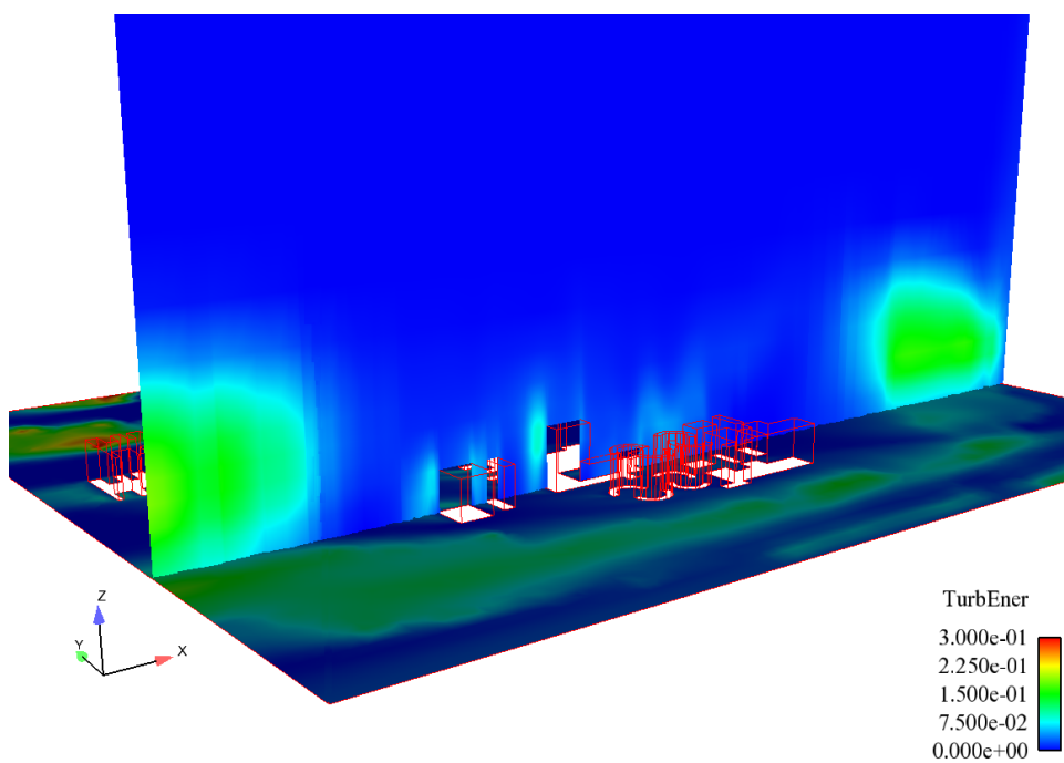
(b) TKE, 2400 TU, plan \vec{xz} , y = 575 m
