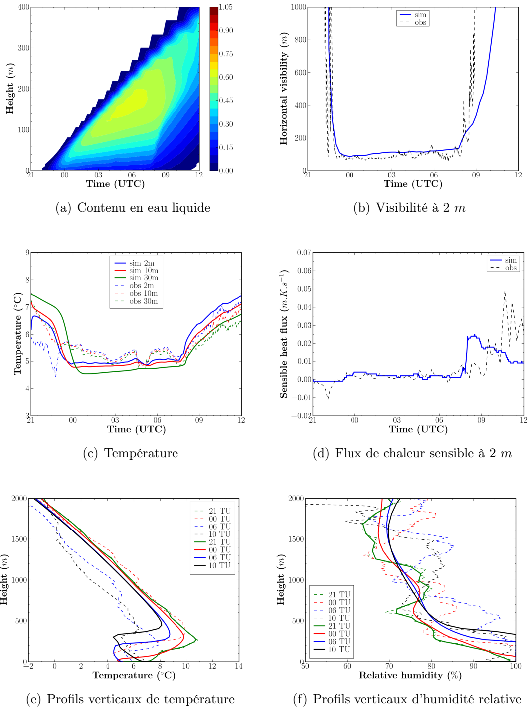
FIG. A.2 : Simulation démarrant à 21 TU avec le modèle diagnostique de Louis sans nudging. \mu_{min} = 0.05 \text{ m}^2 \cdot \text{s}^{-1} .
