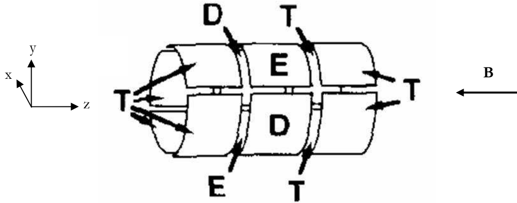
Figure 5 : Configuration d'une trappe d'ions à résonance cyclotronique ou piège de Penning. Elle est constituée de trois types d'électrodes. T : électrode de piégeage, E : électrode d'excitation, D : électrode de détection, B : champ magnétique. Figure d'après Guan et al. [64].
