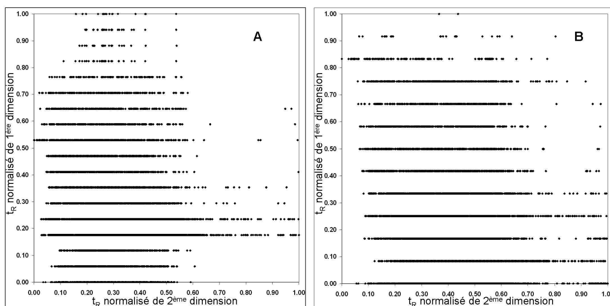
Figure 30 : Orthogonalité des deux dimensions en mode off-line (A) et en mode on-line (B).
