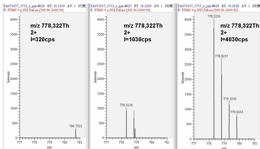
Figure 40 : Suivi dans 3 scans FTMS successifs de l'élution d'un peptide peu abondant de rapport m/z 778,322Th dans 20fmol de LCP.
