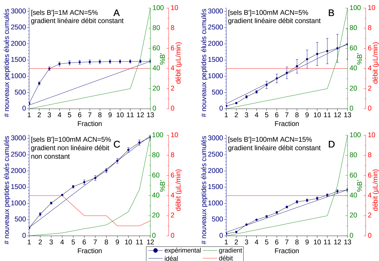
Figure 26 : Comparaison des différents protocoles sur un échantillon de cils digérés. Elution de nouveaux peptides cumulés en fonction des fractions SCX.
