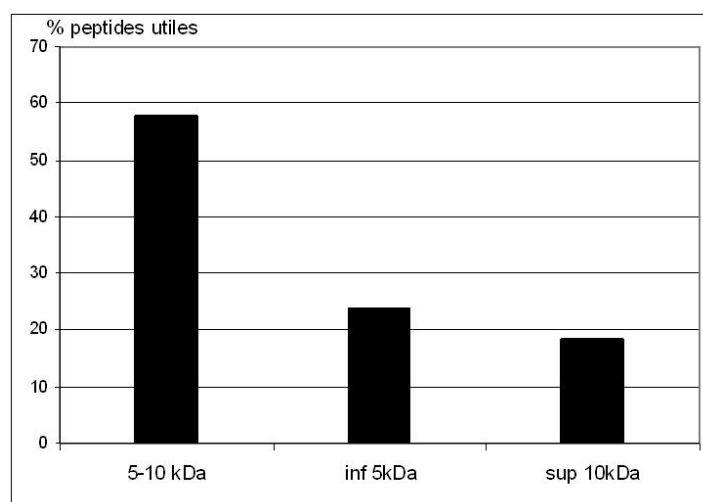
Figure 20 : Apport de chaque fraction dans les identifications.
