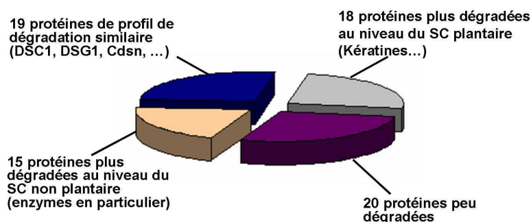
Figure 53 : Comparaison topologique des protéines identifiées dans le stratum corneum plantaire ou non.
