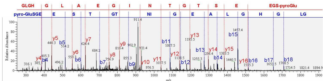
Figure 51 : Interprétation validée d'un spectre MS/MS lors de la confrontation dans la banque Swiss-Prot des données LC1D-FTMS obtenues sur un échantillon de SCP, avec l'hypothèse d'une pyroglutamination N-terminale.
