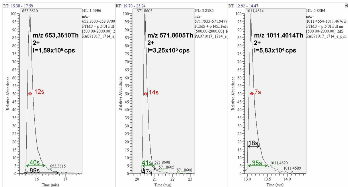
Figure 45 : Profils de différents peptides extraits d'une séparation de 20fmol de LCP.
