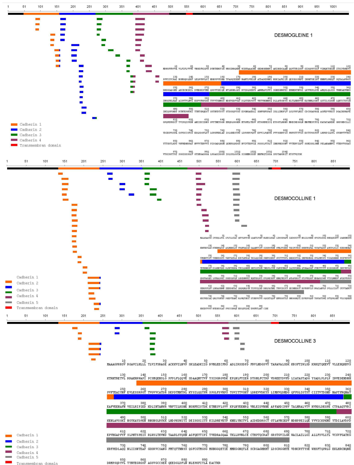
Figure 55 : Profil de dégradation des cadhérines identifiées. Les peptides identifiés dans les échantillons de stratum corneum plantaire et non plantaire ont été regroupés.
