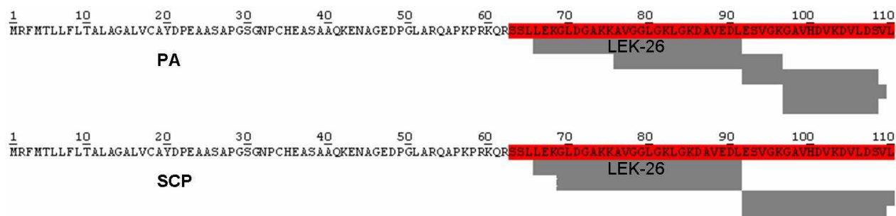
Figure 58 : Peptides dérivés de la DCD identifiés dans les échantillons de stratum corneum non plantaire (PA) et plantaire (SCP). En rouge est rappelé le peptide DCD-1.
