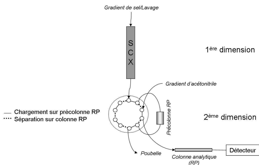
Figure 11 : Système de chromatographie multidimensionnelle on-line .
