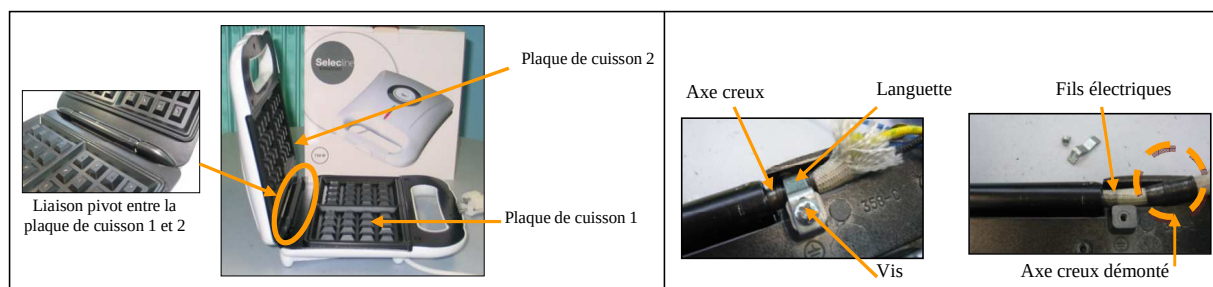
Figure 54 : Détail de l'articulation gaufrier (liaison annulaire démontable)
