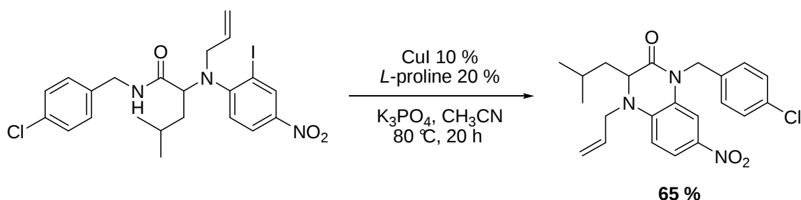
Figure 196 : Synthèse de quinoxalines
