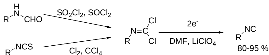
Figure 60 : Formation d'isonitriles par électrochimie
