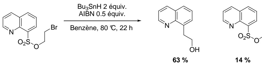
Figure 159 : Réarrangement radicalaire de Truce-Smiles
