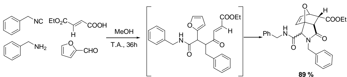
Figure 53 : Séquence Ugi-Diels Alder
