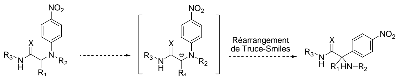
Figure 143 : Projet de r\u00e9arrangement de type Smiles
