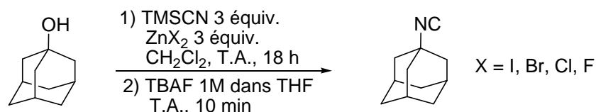
Figure 85 : Synthèse d'isonitrile à partir d'alcool d'adamantyle
