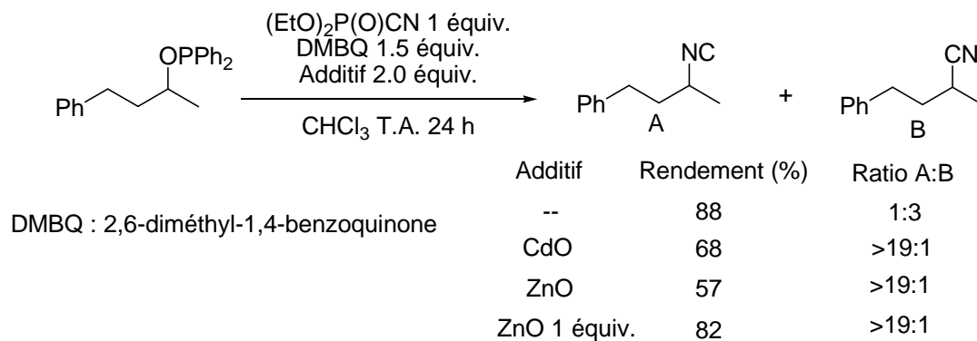
Figure 86: Synth\u00e8se d'isonitrile avec le cyanophosponate de di\u00e9thyle
