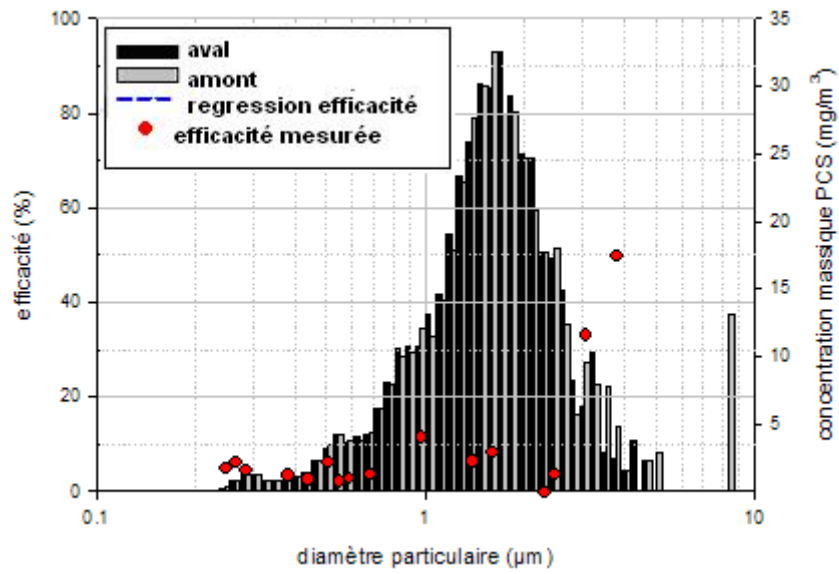
Figure 35 : M9R précécanteur-35l/min-D50>4 microns
