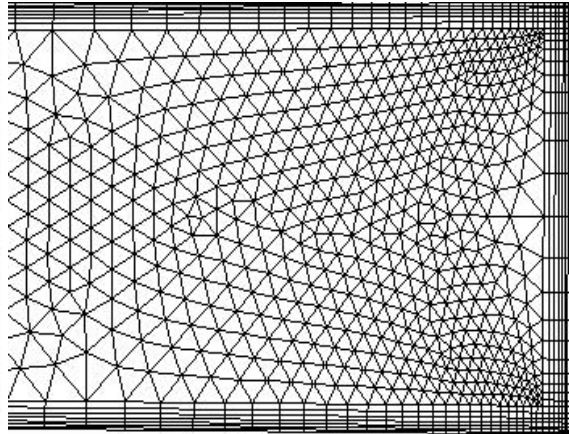
Figure 93: maillage constitué de prismes à la paroi puis de tétraèdres.
