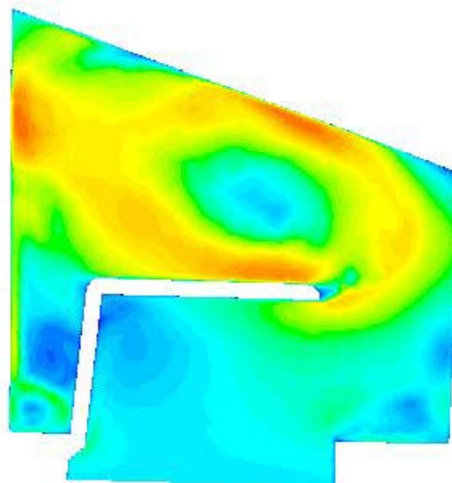
Figure 96: Vitesse moyennée, maillage 4 couches de prismes/tetra X=0.0141m
