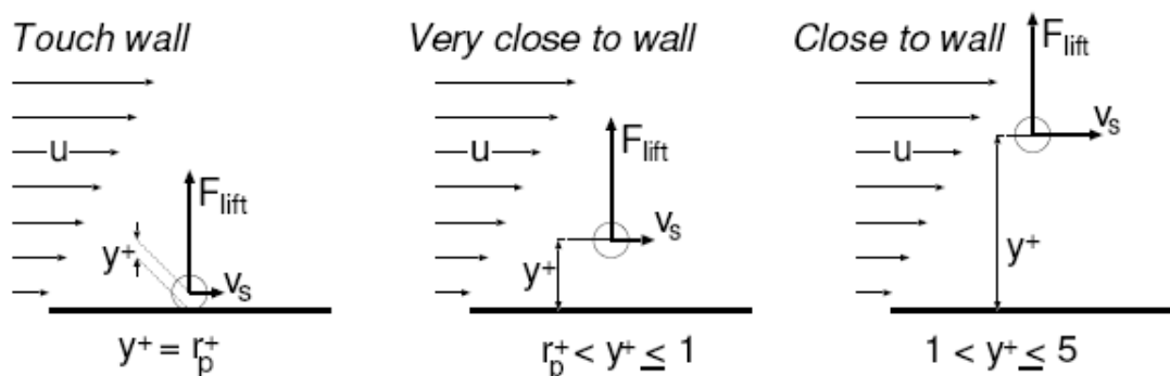
Figure 41 Zones de validité des expressions de la force de Saffman. D'après Van Wageningen (2005).
