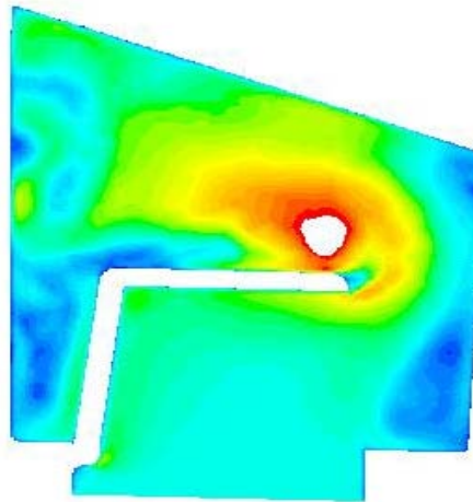
Figure 103 : Vitesse moyennée, maillage 10 couches de prismes/tetra X=0.0475m
