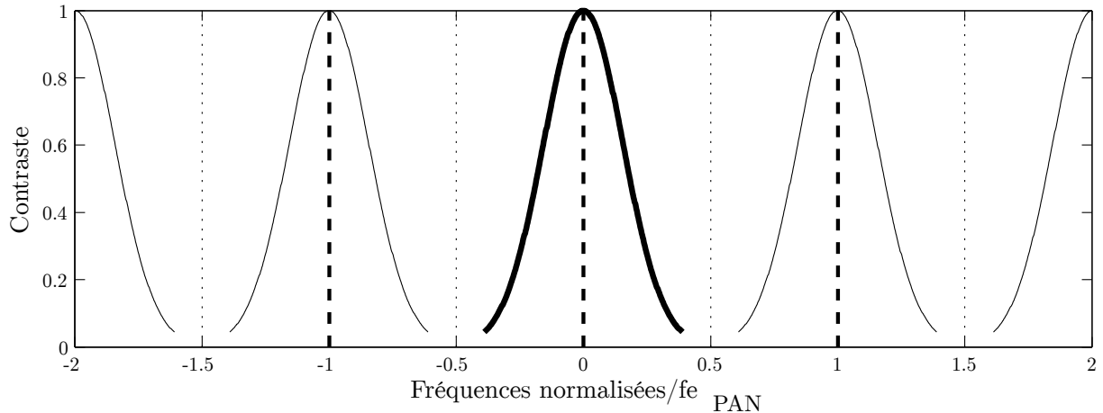
Figure 2.8 : échantillonnage et réplication du spectre
