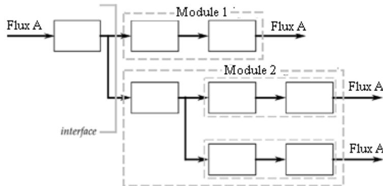
Figure 39. Représentation schématique de l'heuristique de la transmission de flux (Stone a & McAdams, 2004)
