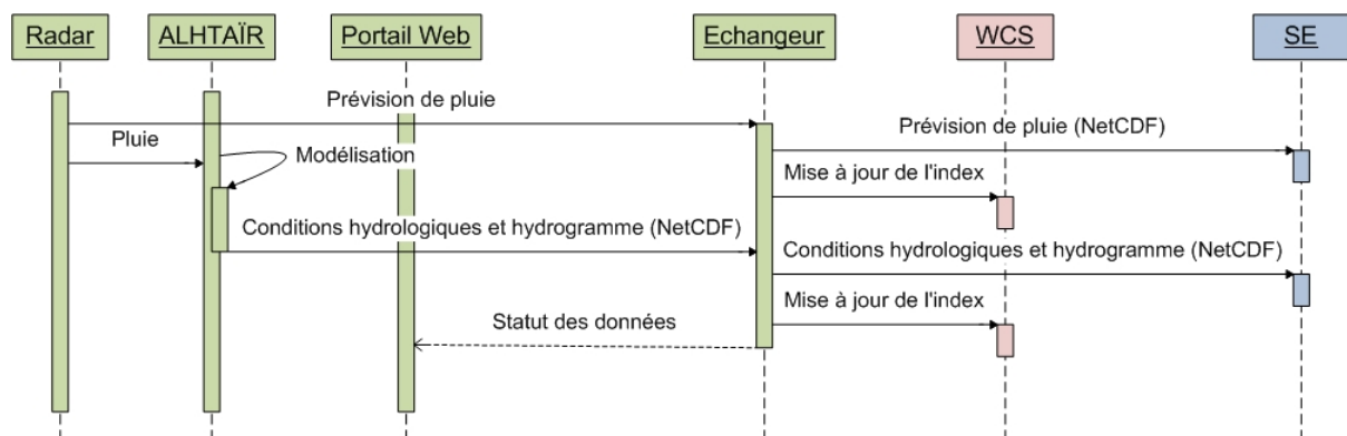
Figure 78 : Diagramme de séquence UML du rôle de l'échangeur, le vert représente le système d'information du SPC-GD, le rouge, le serveur OGC, et le bleu, les ressources de la grille EGEE
