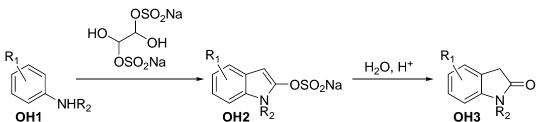
Schéma III-11 : Synthèse d'oxindoles par la réaction d'Hinsberg 132-136
