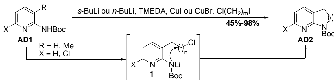
Schéma V-5 : Synthèse de 7-azaindolines par ortho-méallation dirigée 216
