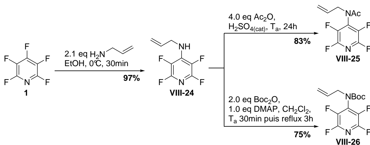
Schéma VIII-16 : Préparation des précurseurs oléfines
