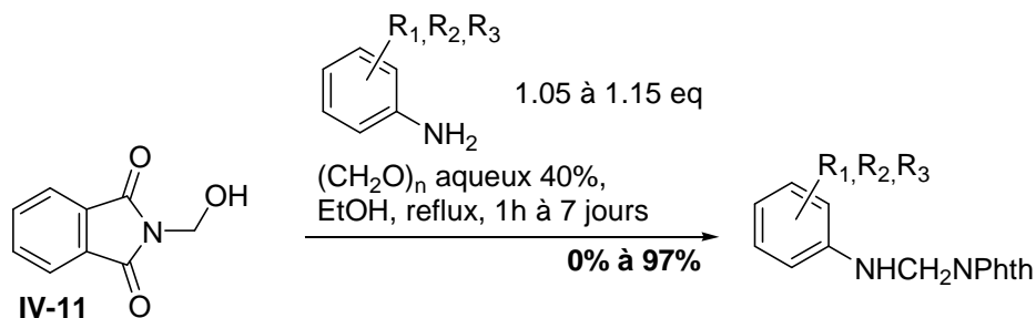
Schéma IV-9 : Formation d'anilines protégées à partir de l'intermédiaire IV-11
