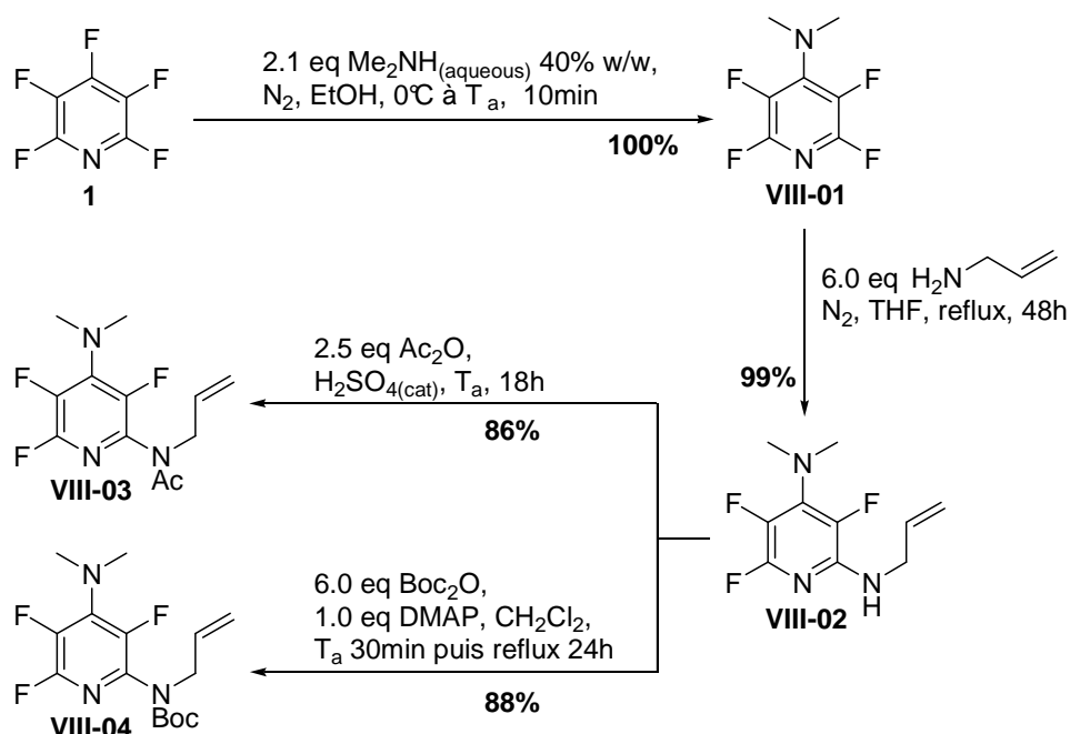
Schéma VIII-3 : Préparation des précurseurs oléfiniques VIII-03 et VIII-04
