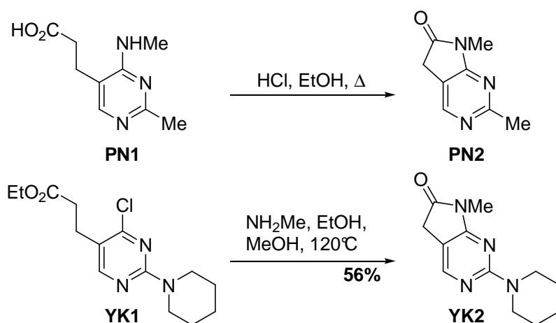
Schéma V-19 : Synthèse de dihydropyrrolopyrimidinones par lactamisation 248,249
