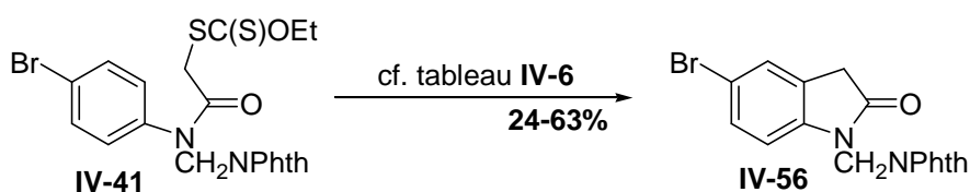
Schéma IV-12 : Tests de conditions de cyclisation radicalaire à partir du dérivé IV-41
