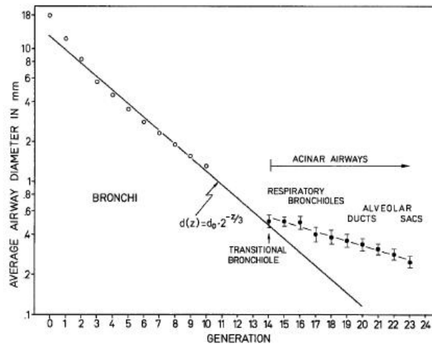
FIGURE 1.8 – Diamètre (sans les alvéoles) des branches dans le poumon en fonction de la génération (d'après Haefeli-Bleuer et Weibel, 1987 [7])
