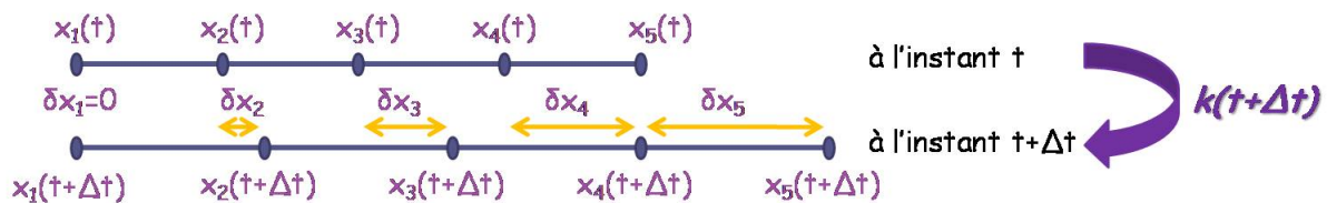
FIGURE 2.13 – Schéma du mouvement du maillage sur une branche
