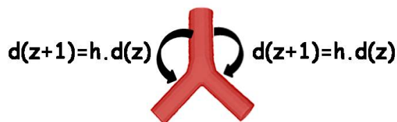
FIGURE 1.4 – Schéma du modèle A de Weibel. h est le facteur d'homothétie.
