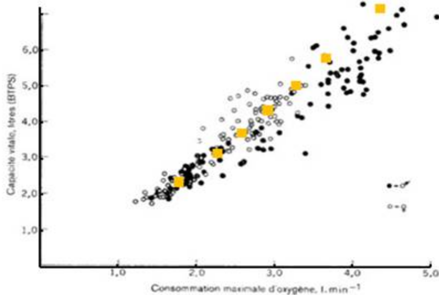
FIGURE 4.15 – Graphes de la capacité vitale en fonction de la consommation d'oxygène maximale \dot{V}_{O_2,max} (d'après Astrand, 1994 [21]). Nous avons superposé les résultats obtenus numériquement et les résultats expérimentaux de Astrand.
