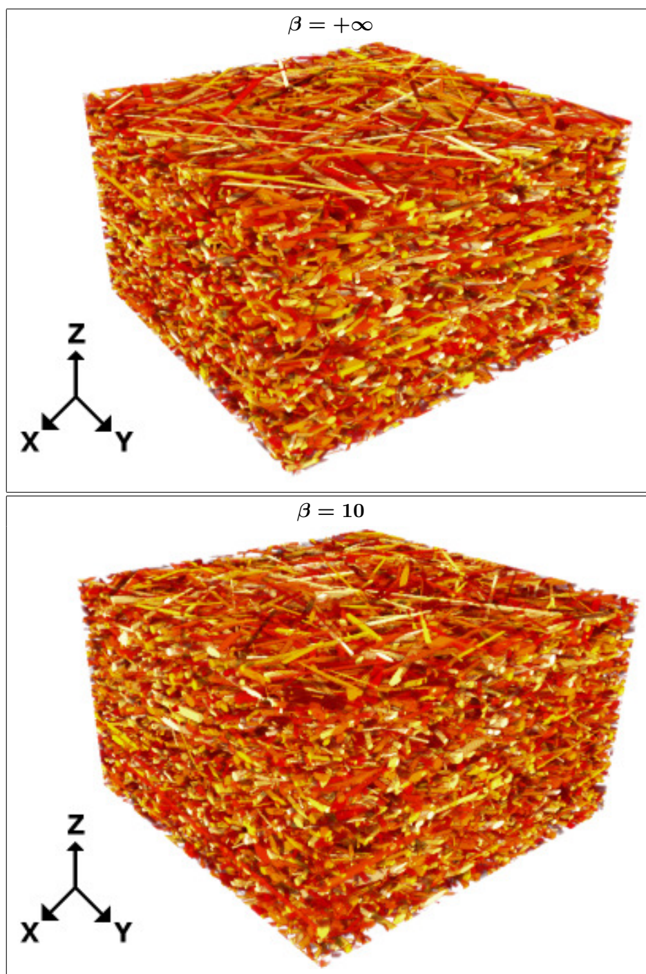
FIGURE 5.1 – Thermisorel™ réel et simulations 3D pour \beta = +\infty et \beta = 10 . Dimensions : 600 \times 600 \times 360 voxels, soit 5,6 \times 5,6 \times 3,4 \text{ mm}^3 ; résolution : 9,36 \mu\text{m}/\text{voxel} .
