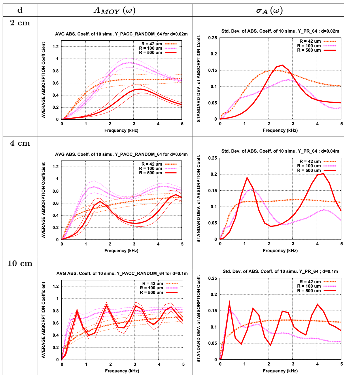
FIGURE 8.62 – Évolution en fonction de la fréquence (de 0 Hz à 5000 Hz) du coefficient d'absorption acoustique moyen A_{MOY}(\omega) avec ses intervalles de confiance à 95 % (traits fins), et évolution de l'écart-type \sigma_A(\omega) de l'ensemble des coefficients d'absorption acoustique, estimés pour 10 milieux homogènes d'épaisseurs d = 2\text{ cm} , 4\text{ cm} et 10\text{ cm} constitués des cellules périodiques élémentaires 2D PACC RANDOM64 correspondantes, en stimulation sonore selon l'axe vertical Oy . R_F = 42\ \mu\text{m} , 100\ \mu\text{m} , et 500\ \mu\text{m} .
