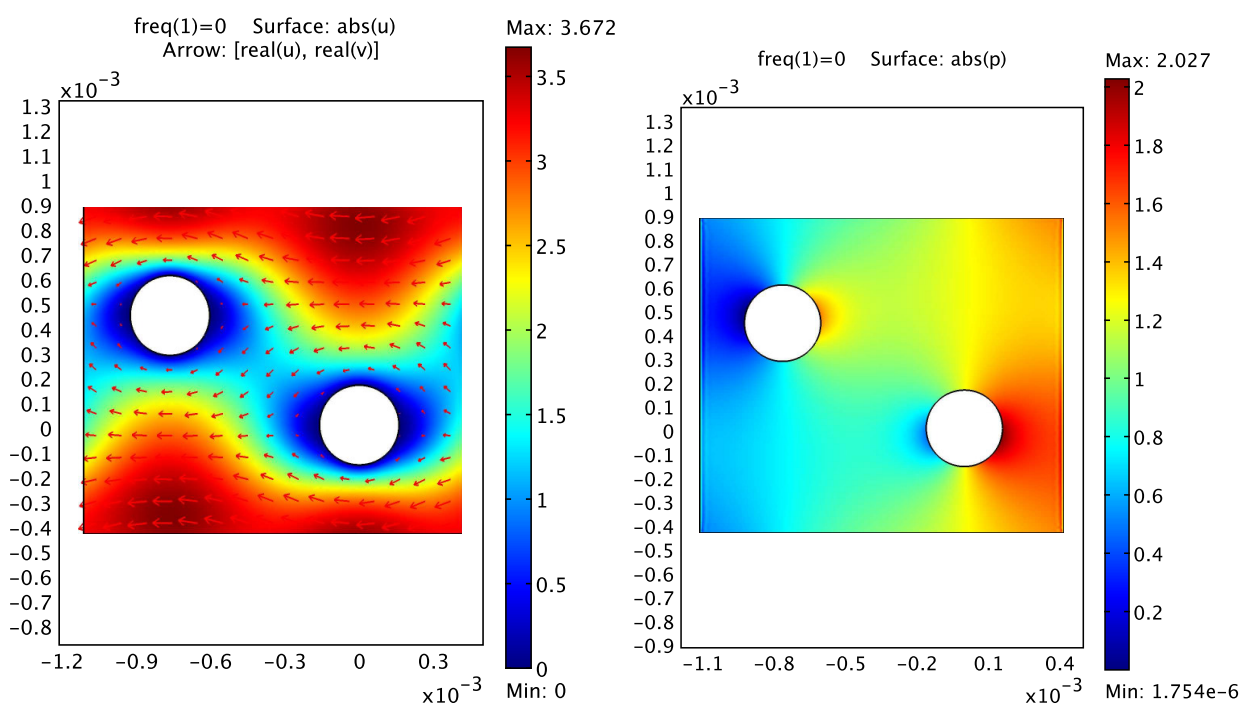
(a) Champ de vitesse acoustique \vec{u} ( m \cdot s^{-1} )
