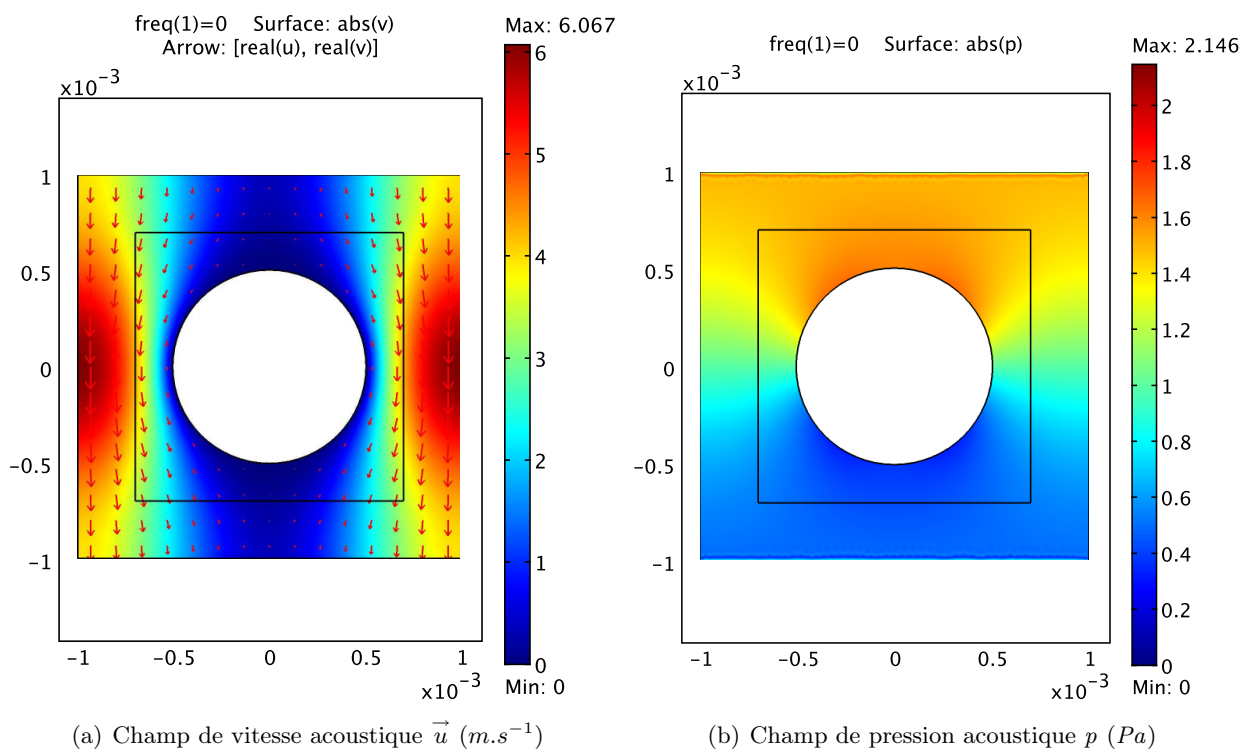
FIGURE 7.3 – Champs de vitesse (en m/s) et de pression (en Pa) acoustiques en régime statique ( f = 0 \text{ Hz} ) pour une cellule élémentaire 2D PACC (Fig. 7.2) en stimulation sonore selon l'axe vertical Oy , source en haut de la cellule élémentaire.
