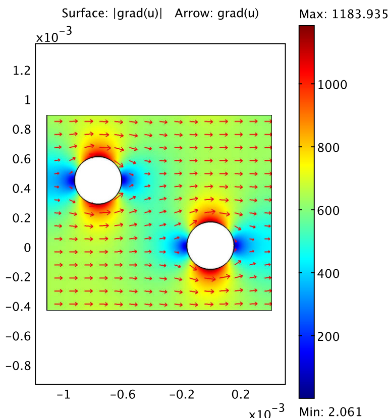
FIGURE F.4 – Champ électrique \vec{E} (en \text{V/m} ) pour une cellule élémentaire 2D Perrot RH (Fig. F.1), en stimulation électrique selon l'axe horizontal Ox , source à droite de la cellule élémentaire.
