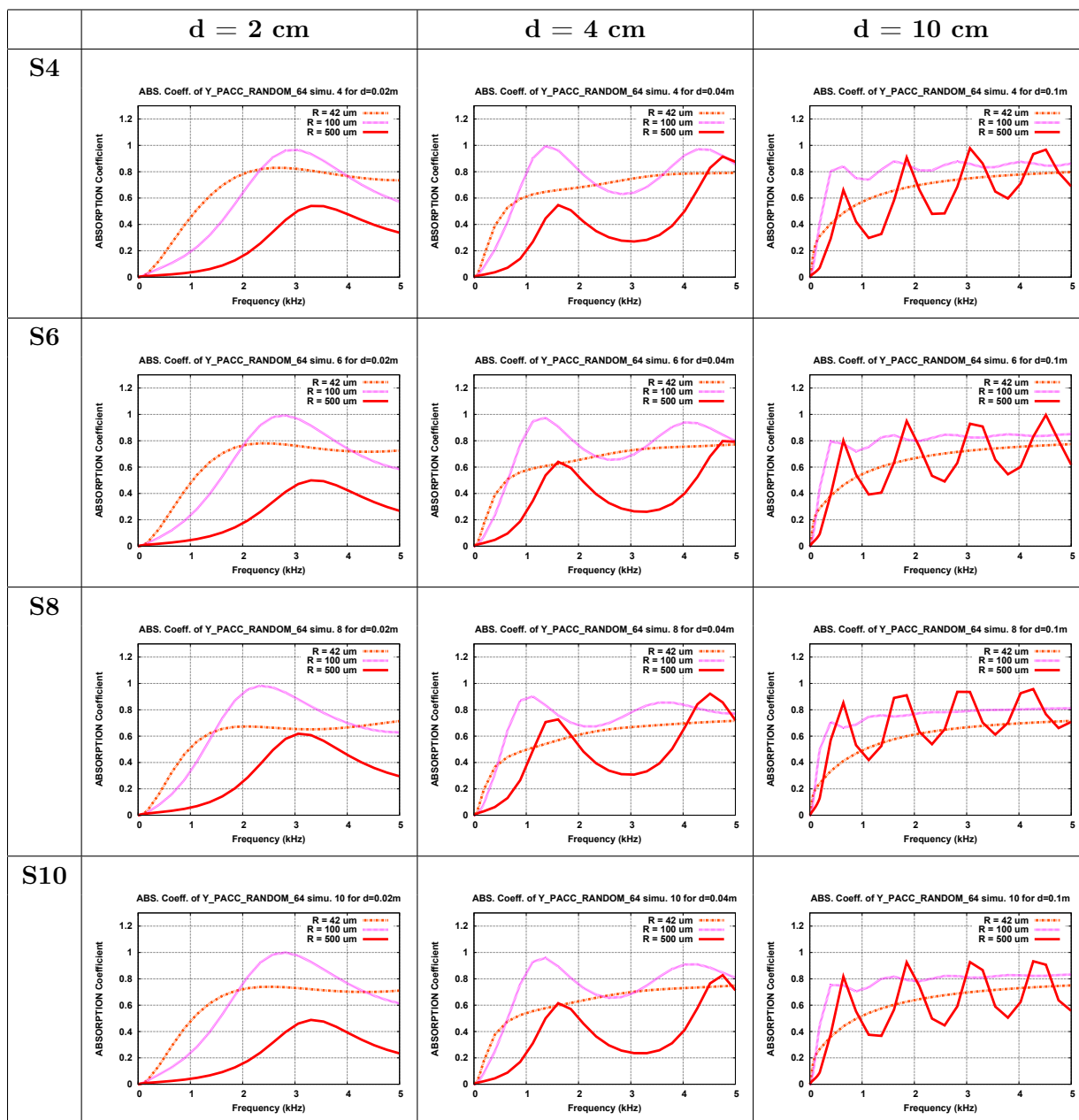
FIGURE 8.61 – Évolution en fonction de la fréquence (de 0 Hz à 5000 Hz) du coefficient d'absorption acoustique A(\omega) des milieux homogènes d'épaisseurs d = 2 \text{ cm} , 4 \text{ cm} et 10 \text{ cm} constitués de cellules périodiques élémentaires 2D PACC RANDOM64 4, 6, 8 et 10, en stimulation sonore selon l'axe vertical Oy . R_F = 42 \mu\text{m} , 100 \mu\text{m} , et 500 \mu\text{m} .
