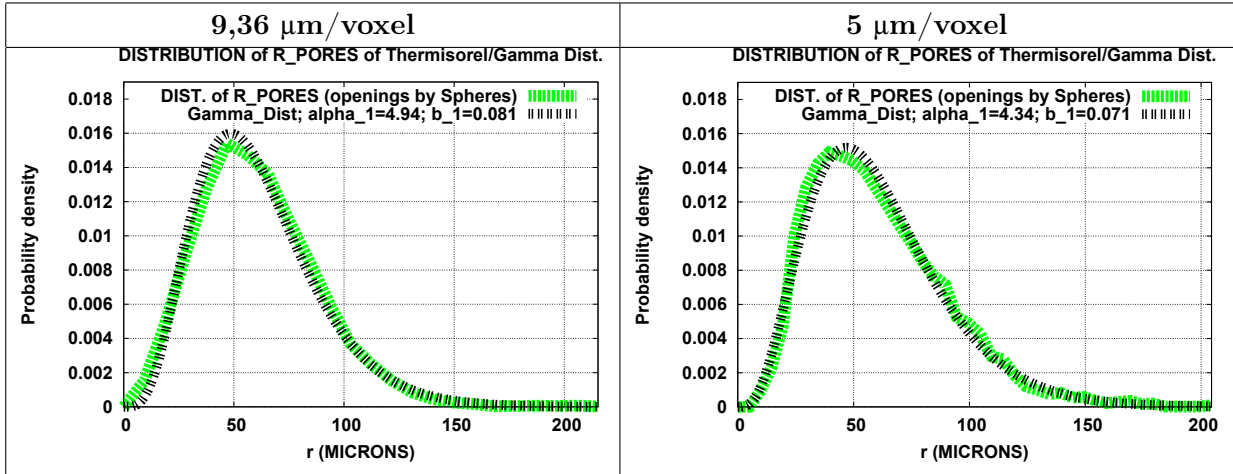
FIGURE 3.11 – Calage de lois gamma sur les distributions en volume des rayons de pores pour 4 échantillons de Thermisorel™ à 4 résolutions différentes : 15 μm, 10 μm, 9,36 μm et 5 μm/voxel (lumens rebouchés) (élément structurant Sphère FM).
