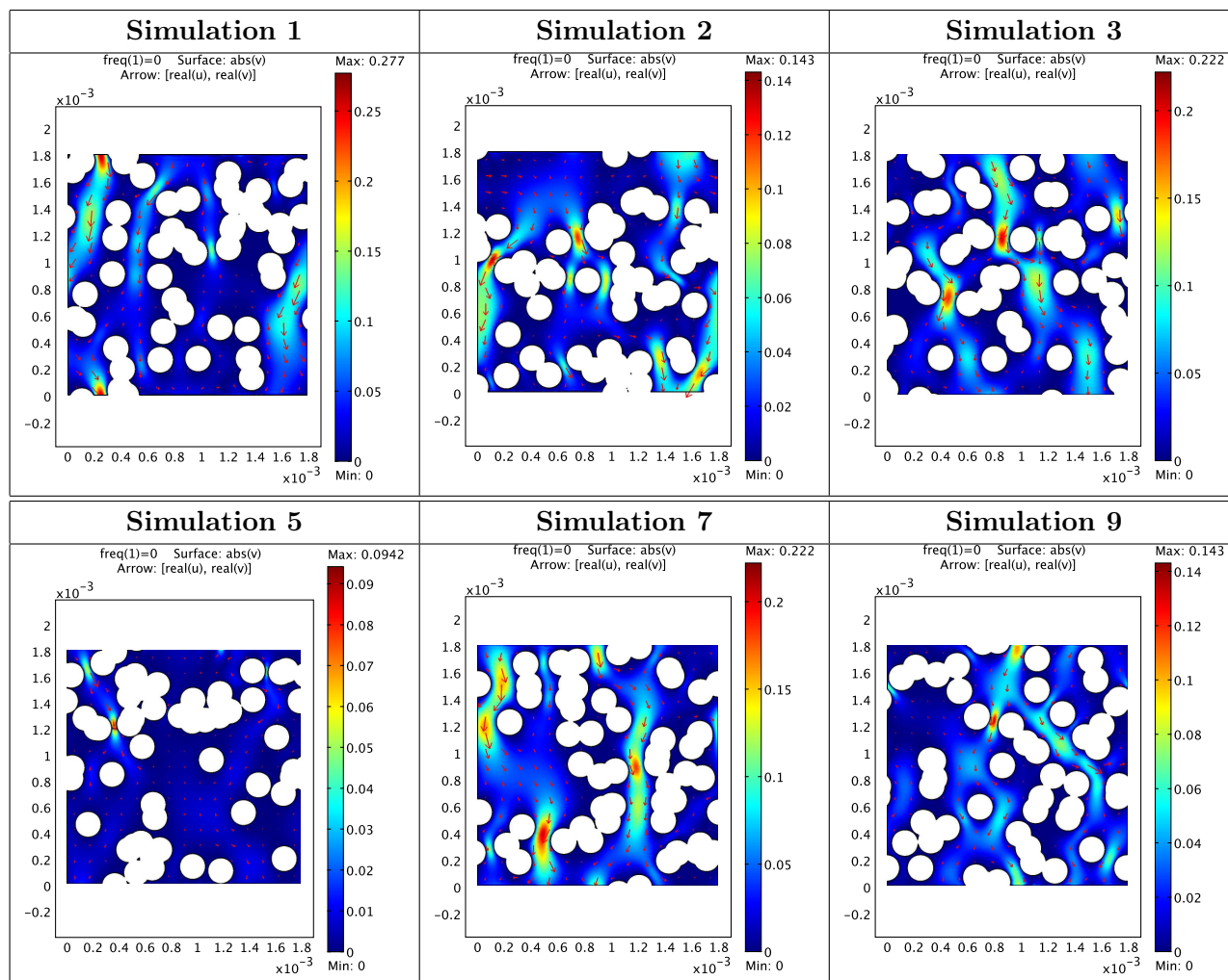
FIGURE 8.59 – Champs de vitesse acoustique (en m/s) en régime statique ( f = 0 Hz) pour les six cellules élémentaires 2D PACC RANDOM64 1, 2, 3, 5, 7 et 9 en stimulation sonore selon l'axe vertical Oy , sources en haut des cellules élémentaires. R_F = 100 \mu m .
