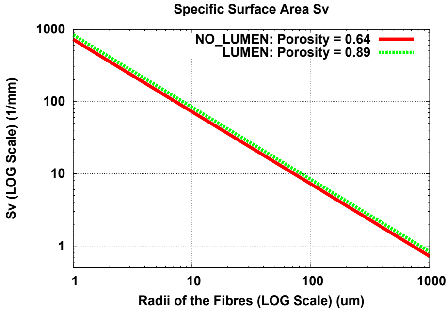
FIGURE 8.45 – Évolution de la surface spécifique S_v (en \text{mm}^{-1} ) des cellules élémentaires 2D PASC NO LUMEN et 2D PASC LUMEN en fonction des rayons de fibres R_F . Échelles logarithmiques.
