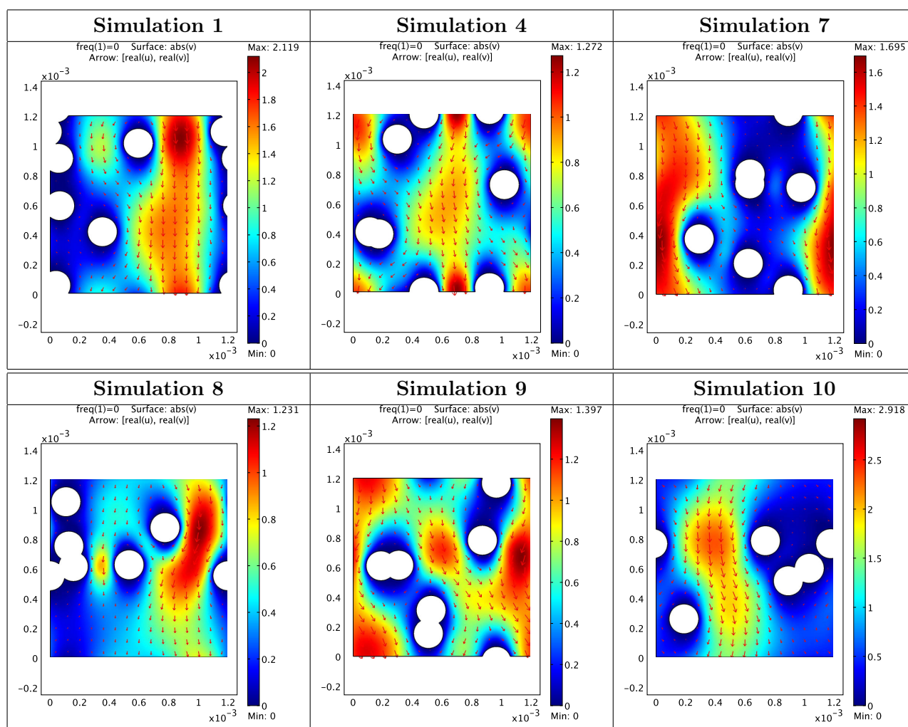
FIGURE 8.50 – Champs de vitesse acoustique (en m/s) en régime statique ( f = 0 Hz) pour les six cellules élémentaires 2D PACC RANDOM89 1, 4, 7, 8, 9 et 10 en stimulation sonore selon l'axe vertical Oy , sources en haut des cellules élémentaires. R_F = 100 \mu m .
