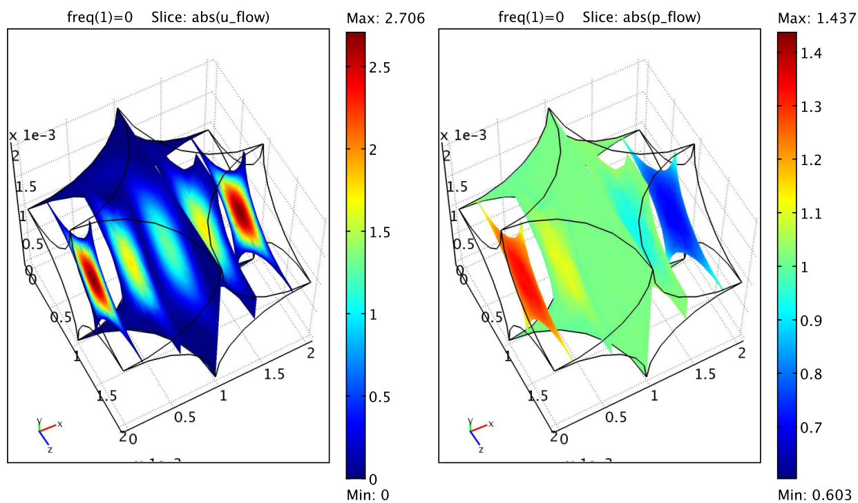
(a) Champ de vitesse acoustique \vec{u} ( m.s^{-1} )
