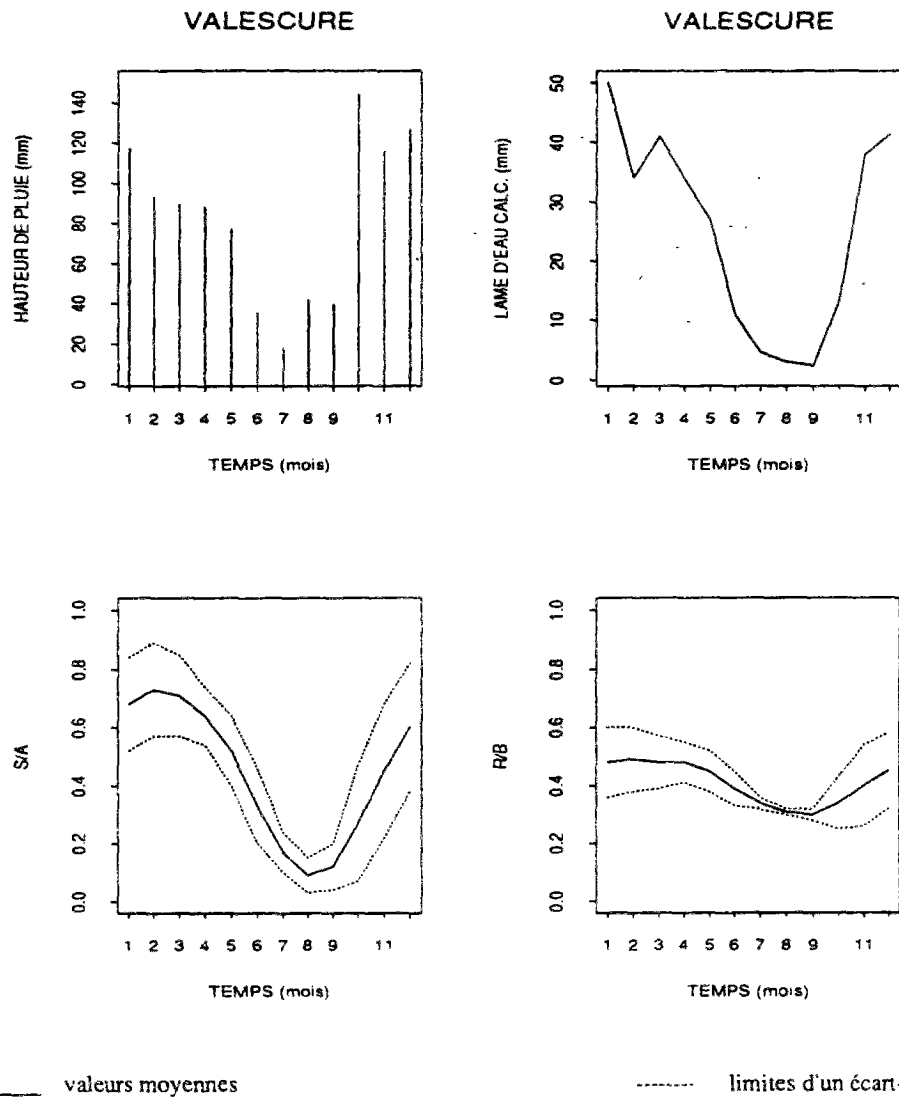
Fig. 3.12 b - Valeurs moyennes mensuelles de P , de Q_{calc} , de S/A et de R/B . Valescure au Bourdins caïage : 1981-1989
