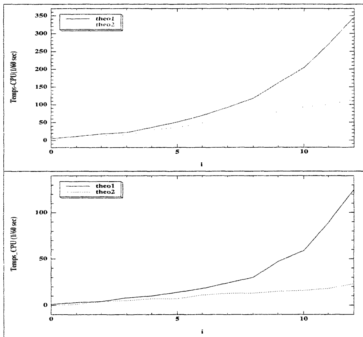
FIG. II.11 – Comparaison des temps CPU (en 1/60sec) pour le calcul de \langle f, \phi_M \rangle (courbe en haut) et \langle g, \phi_M \rangle (courbe en bas), respectivement donnés par les théorèmes 6 et 7, M = 2, 3, 4 et \varepsilon = 10^{-i} , i = 0, \dots, 12 .
