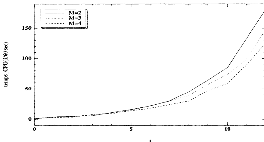
FIG. II.6 – Temps CPU pour le calcul par le théorème 6 de \langle g, \phi_M \rangle , M = 2, 3, 4 en fonction de \varepsilon = 10^{-i} .
