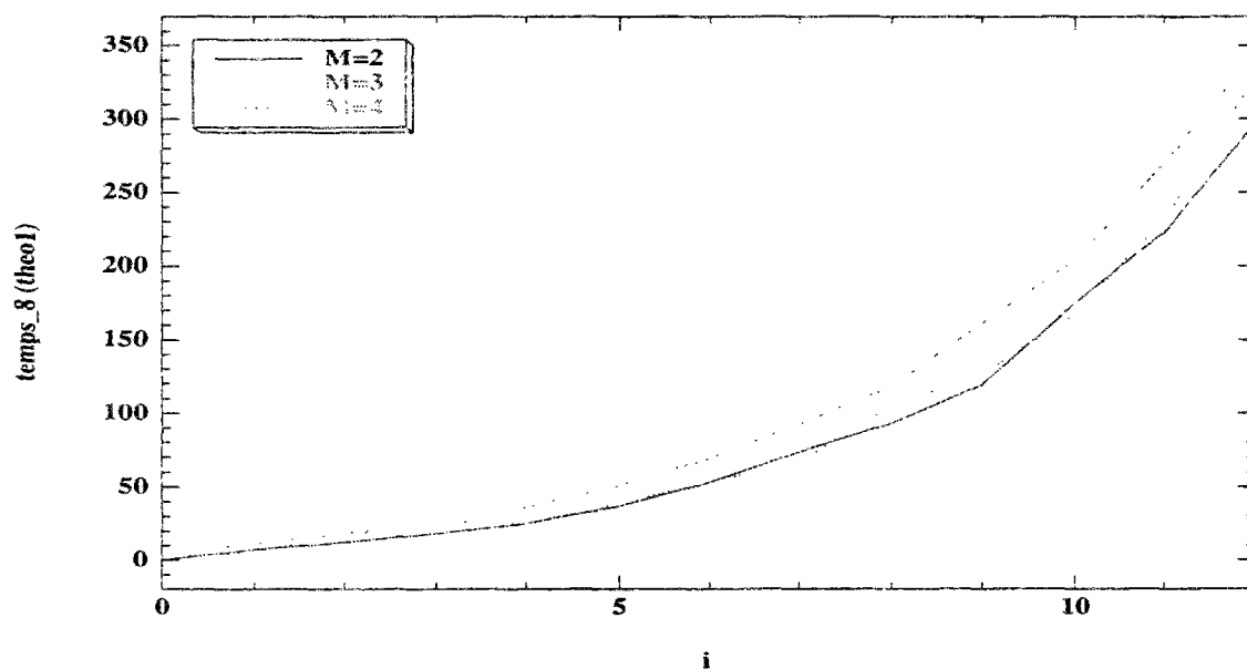
FIG. II.5 – Temps CPU pour le calcul par le théorème 6 de \langle f, \phi_M \rangle M = 2, 3, 4 en fonction de \varepsilon = 10^{-i} .
